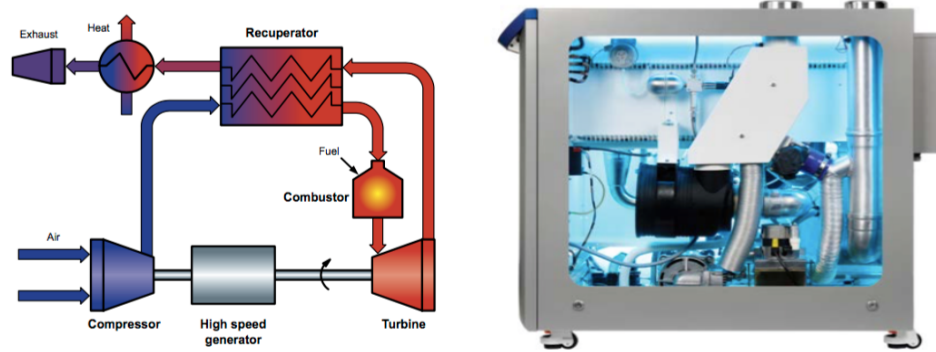
Şekil 2.1. Örnek bir mikro kojenerasyon ünitesi [27]
