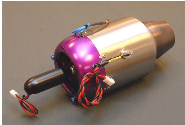
Şekil 4.1. AMT Titan turbojet motoru
