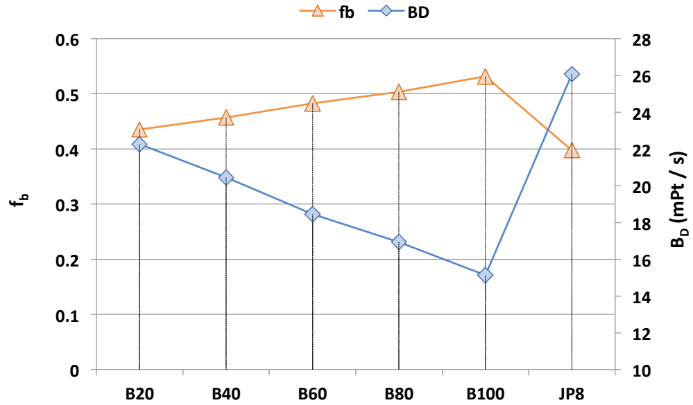
Şekil 4.45. 4.uçuş noktası için egzoz lülesi ekserji yıkım çevresel etkisi ve eksergoçevresel faktörün değişimi
