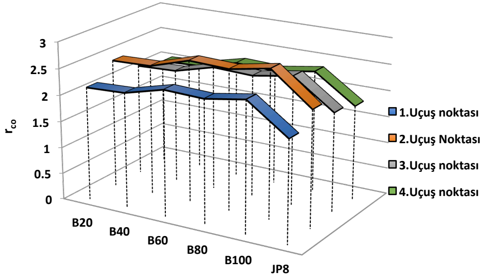
Şekil 4.28. Yanma odası için görece özgül maliyet farkı
