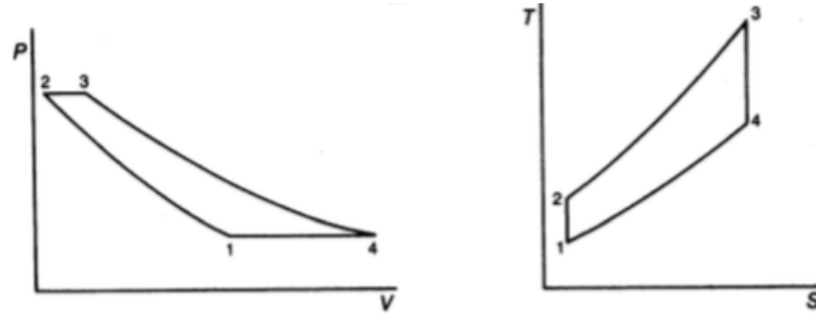
Şekil 3.1. İdeal Brayton çevrimi [31]
