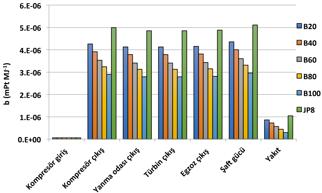
Şekil 4.41. 4. uçuş noktası için motor komponentleri özgül çevresel etki değerleri
