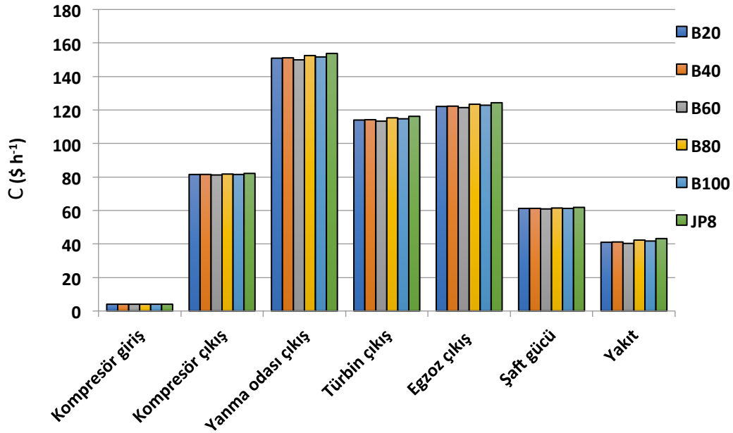
Şekil 4.24. 3. uçuş noktası için motor bileşenleri maliyet oranları
