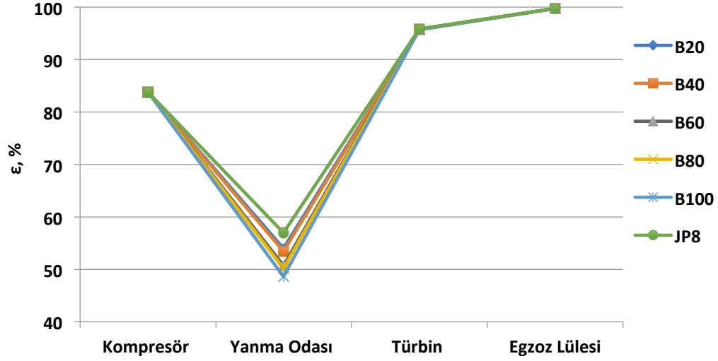
Şekil 4.17. 3. uçuş noktası için komponent ekserji verimlerinin yakıtlara göre değişimi
