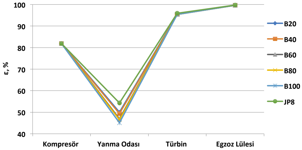
Şekil 4.15. 1.uçuş noktası için komponent ekserji verimlerinin yakıtlara göre değişimi
