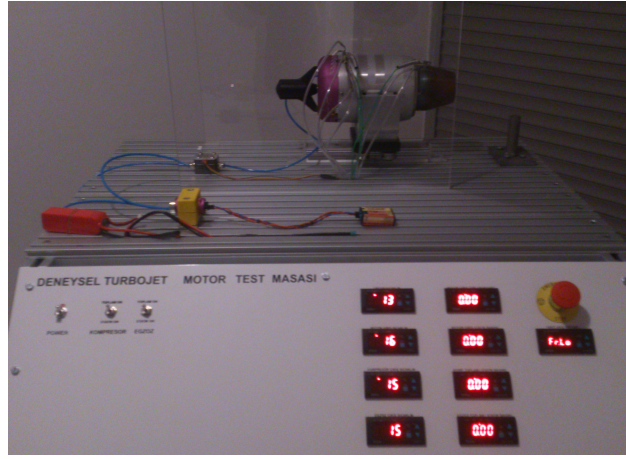
Şekil 4.8. Test düzeneği görünümü
