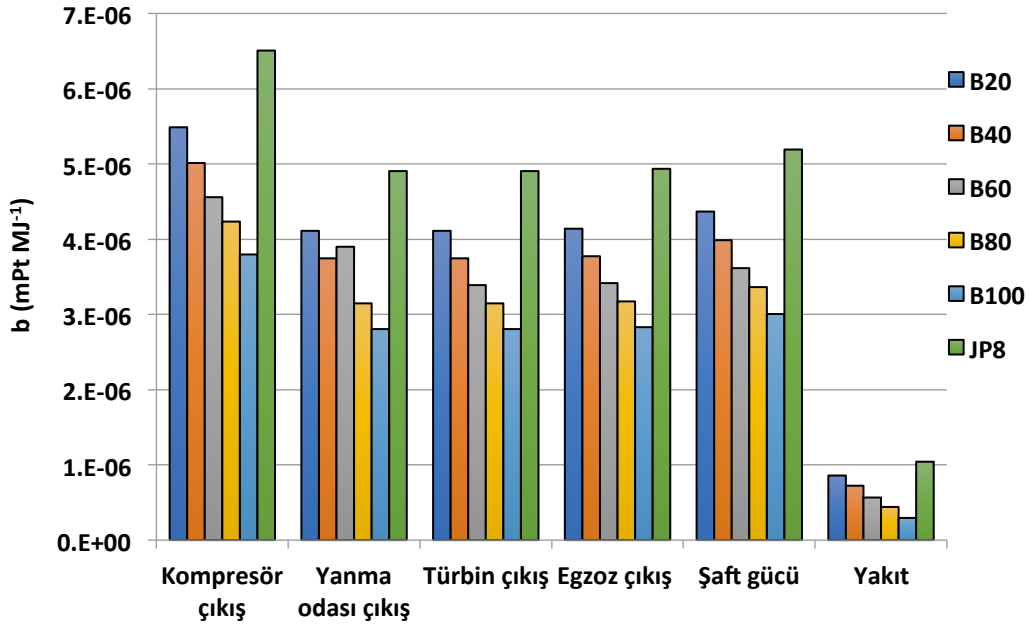
Şekil 4.37. 2.uçuş noktası için motor komponentleri özgül çevresel etki değerleri
