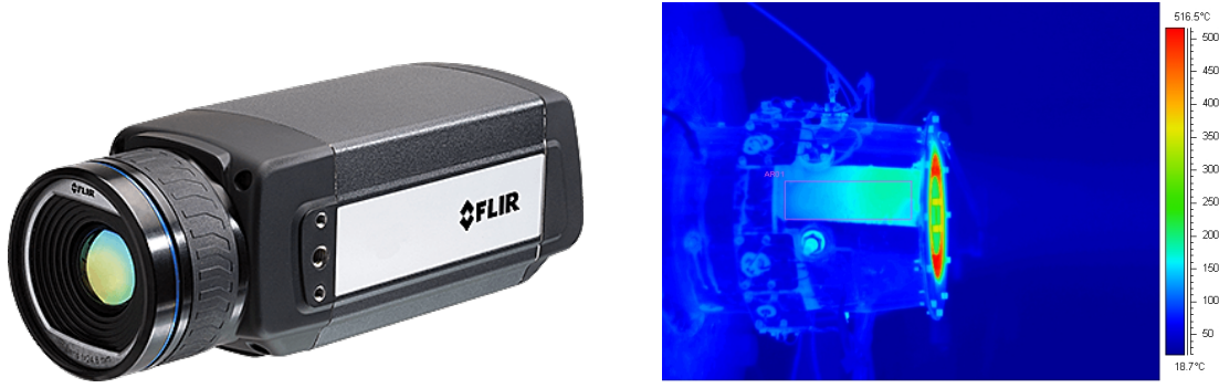
Şekil 4.13. Yüzey sıcaklık ölçümü
