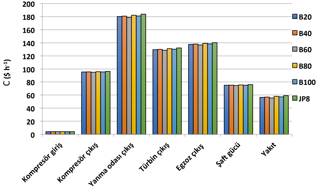
Şekil 4.26. 4.uçuş noktası için motor bileşenleri maliyet oranları
