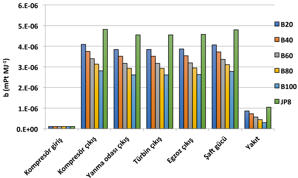
Şekil 4.39. 3.uçuş noktası için motor komponentleri özgül çevresel etki değerleri
