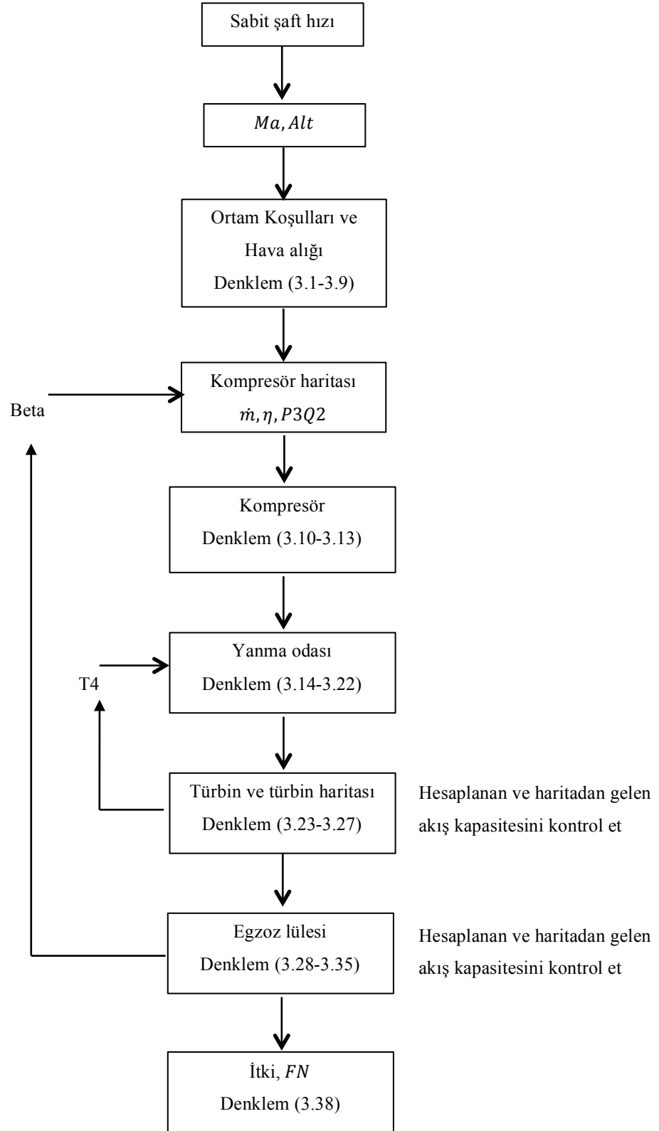
Şekil 3.3. Turbojet motor performans analizi (off-design) yöntemi
