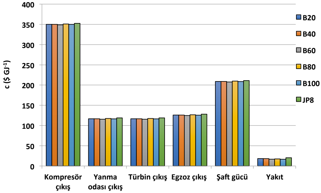
Şekil 4.23. 2. uçuş noktası için motor bileşenleri özgül maliyetleri
