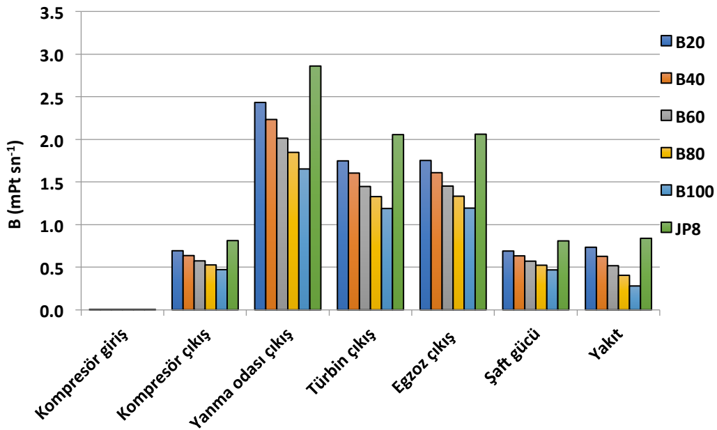
Şekil 4.40. 4. uçuş noktası için motor komponentleri çevresel etki değerleri
