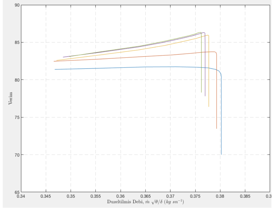
Şekil 4.5. Performans yazılımı ile elde edilen türbin haritası
