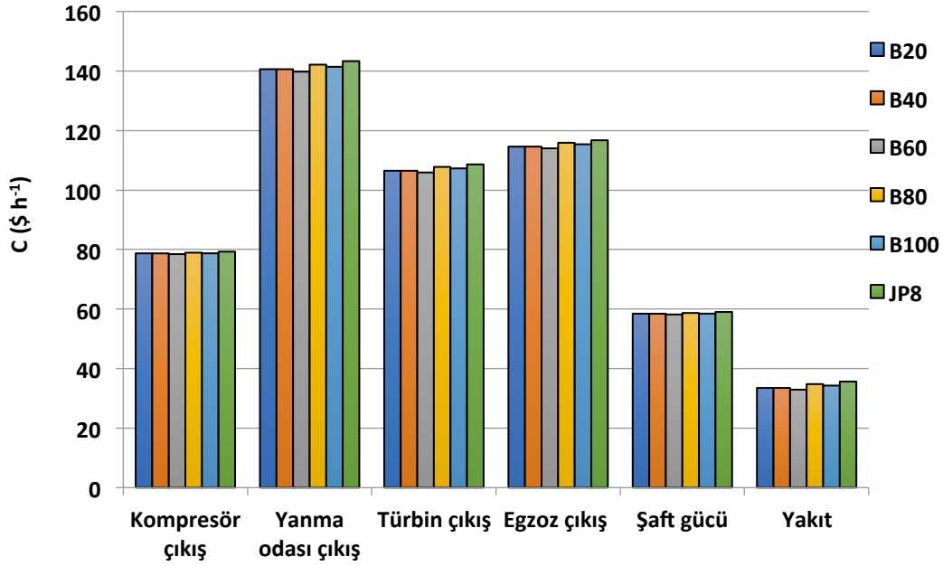
Şekil 4.22. 2.uçuş noktası için motor komponentleri maliyet oranları
