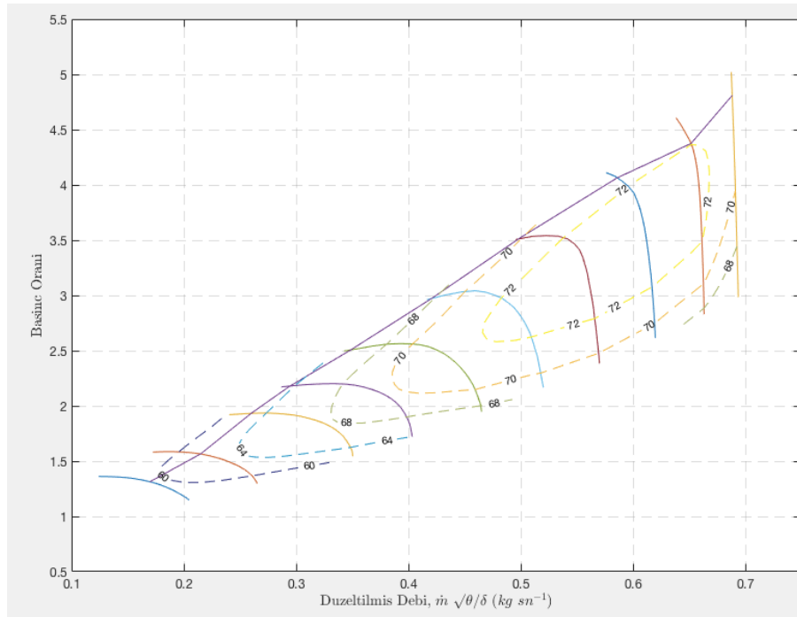
Şekil 4.4. Performans yazılımı ile elde edilen kompresör haritası
