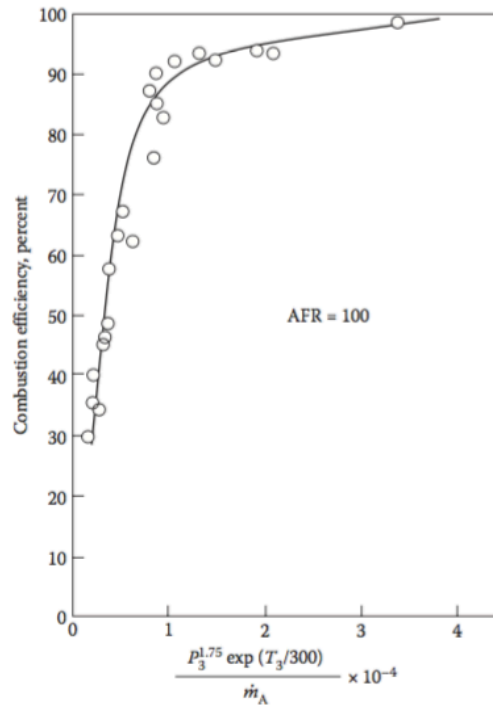
Şekil 4.10. Bir yanma odası için yanma verimi korelasyonu [50]
