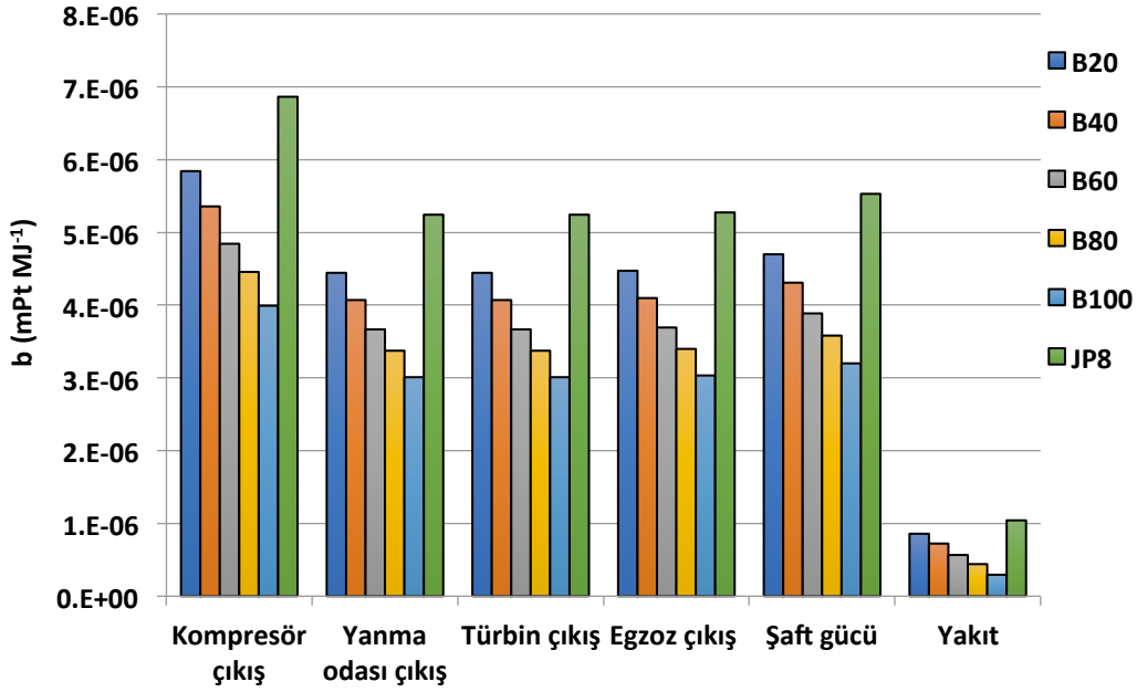
Şekil 4.35. 1.uçuş noktası için motor komponentleri özgül çevresel etki değerleri
