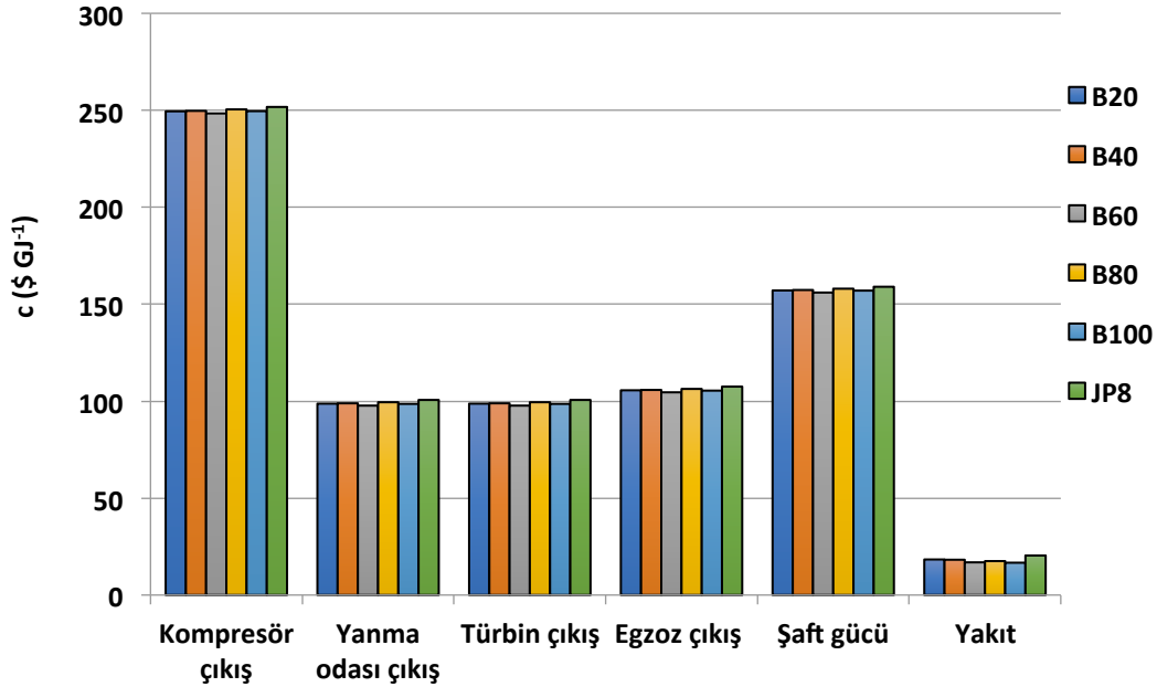
Şekil 4.21. 1. uçuş noktası için motor bileşenleri özgül maliyetleri
