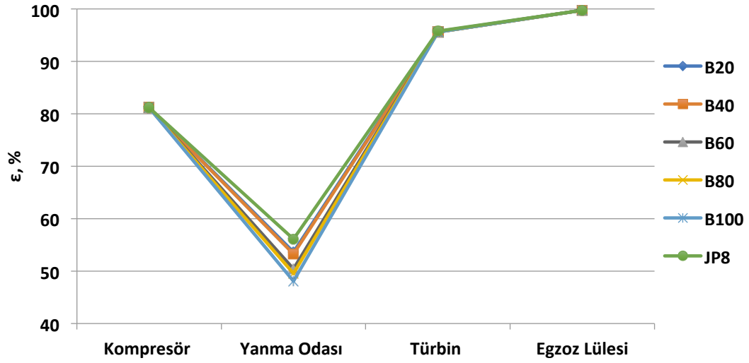
Şekil 4.16. 2.uçuş noktası için komponent ekserji verimlerinin yakıtlara göre değişimi
