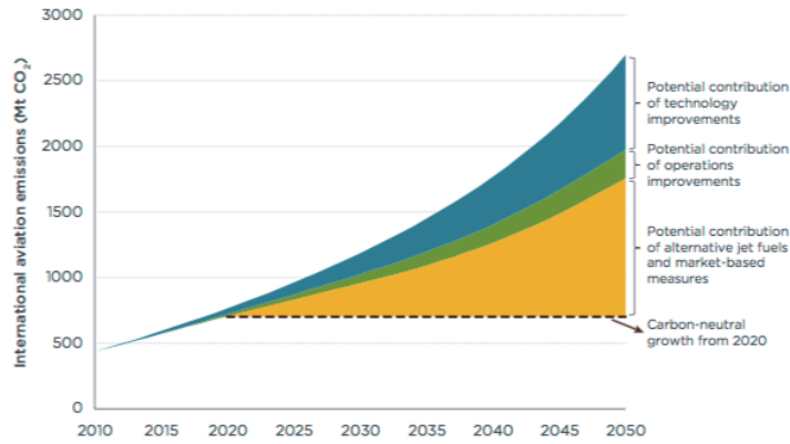
Şekil 1.3. Uluslararası sivil havacılık emisyonları ve azaltma stratejileri [5]
