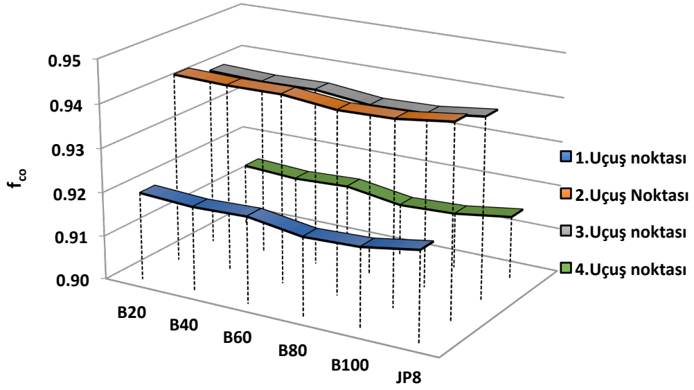
Şekil 4.29. Türbin için eksergoekonomik faktör parametresi
