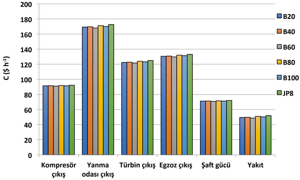
Şekil 4.20. 1. uçuş noktası için motor komponentleri maliyet oranları
