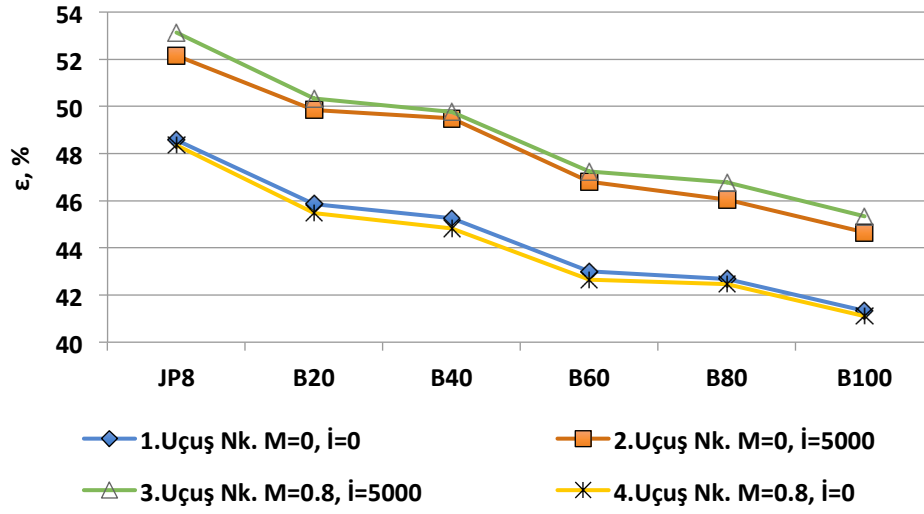
Şekil 4.19. Motor ekserji veriminin yakıtlara ve uçuş zarfına göre değişimi
