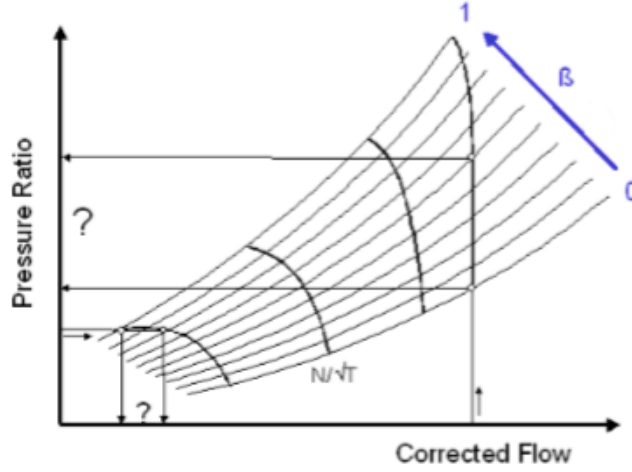
Şekil 3.4. Kompresör haritasında Beta çizgilerinin gösterimi [34]
