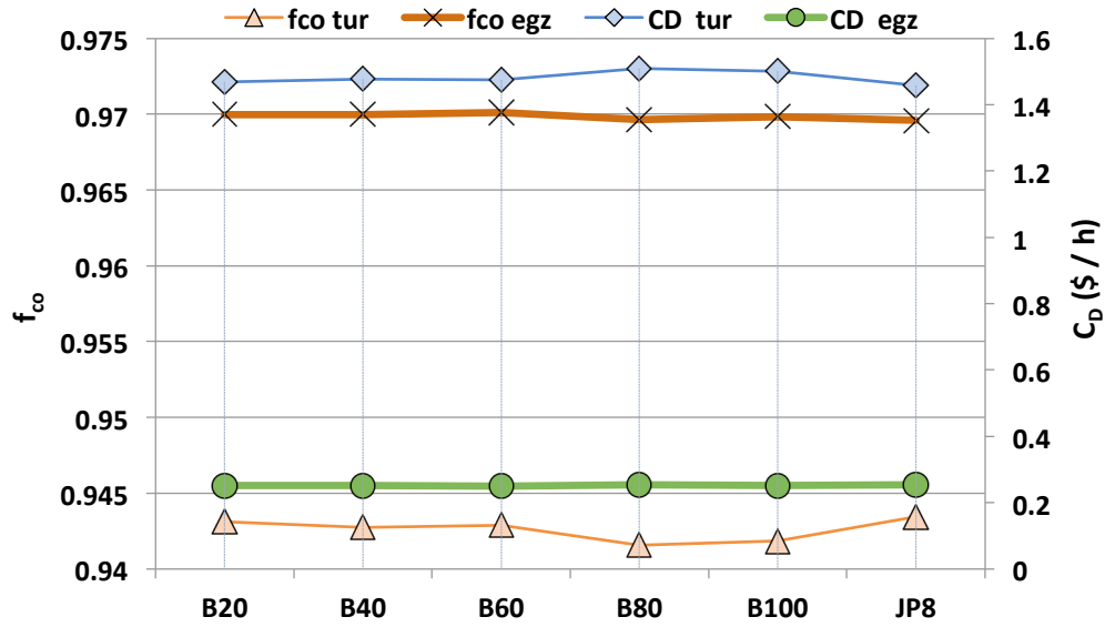
Şekil 4.31. 2.uçuş noktası için türbin ve egzoz lülesi ekserji yıkım maliyeti ve eksergoekonomik faktörün değişimi
