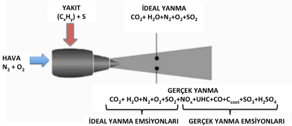
Şekil 1.4. Uçak jet motoru için ideal ve gerçek yanma işlemi [6]
