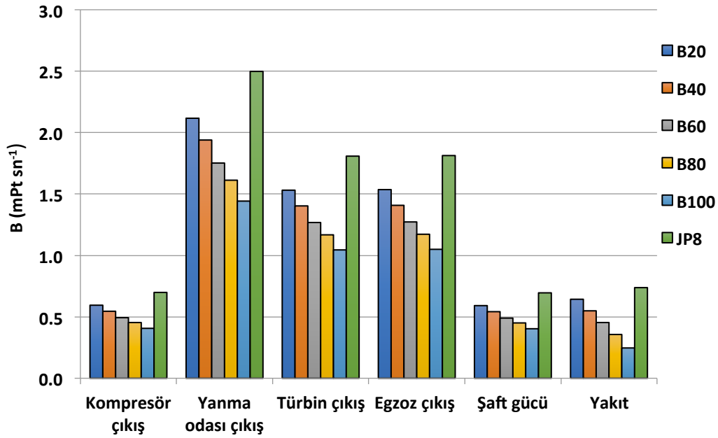
Şekil 4.34. 1.uçuş noktası için motor komponentleri çevresel etki değerleri
