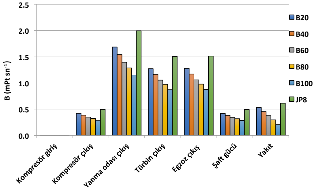
Şekil 4.38. 3.uçuş noktası için motor komponentleri çevresel etki değerleri
