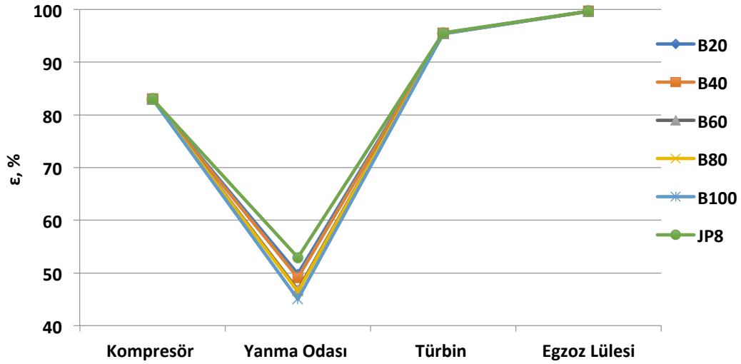
Şekil 4.18. 4.uçuş noktası için komponent ekserji verimlerinin yakıtlara göre değişimi
