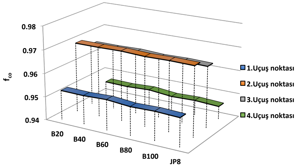
Şekil 4.30. Egzoz lülesi için eksergoekonomik faktör parametresi
