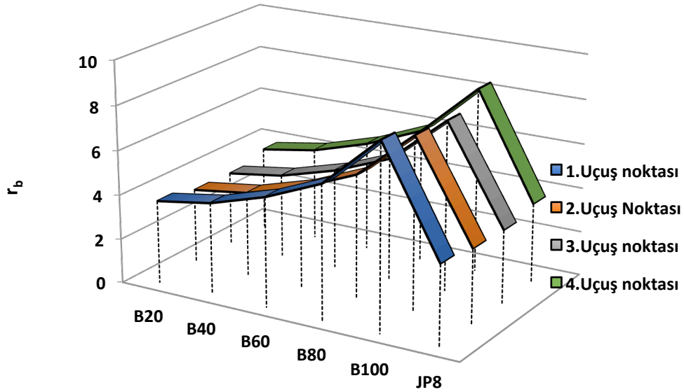
Şekil 4.42. Yanma odası için görece özgül çevre etkisi
