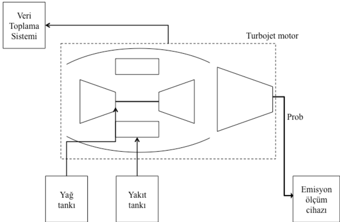
Şekil 4.9. Motor test düzeneği şematik gösterimi
