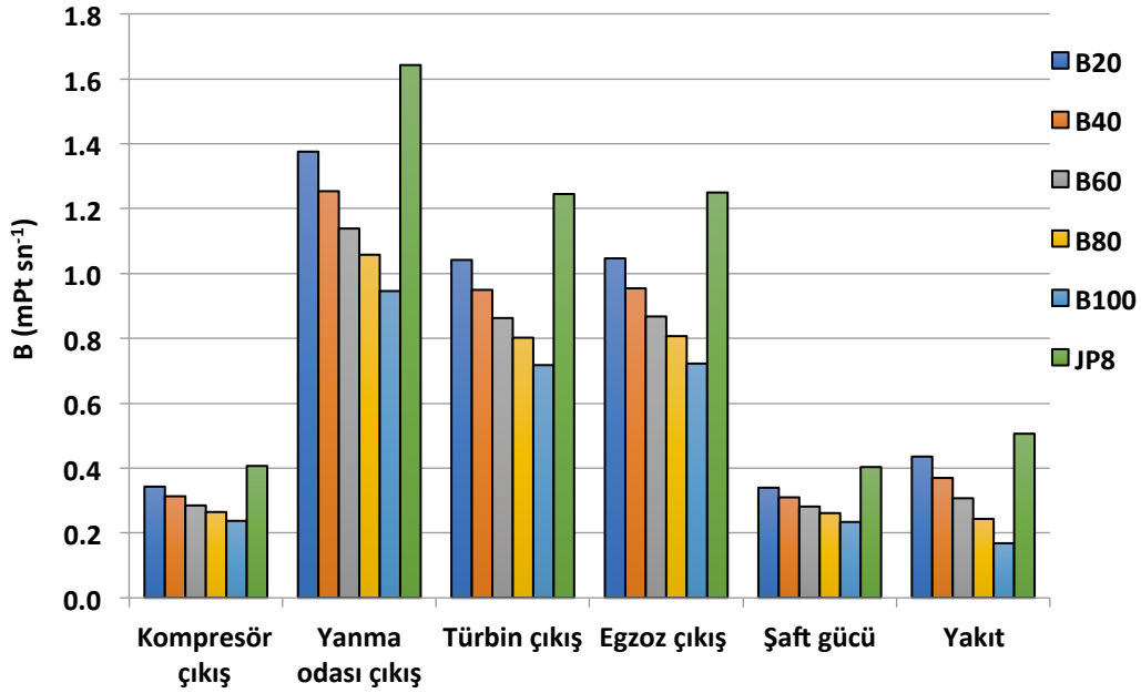
Şekil 4.36. 2.uçuş noktası için motor komponentleri çevresel etki değerleri
