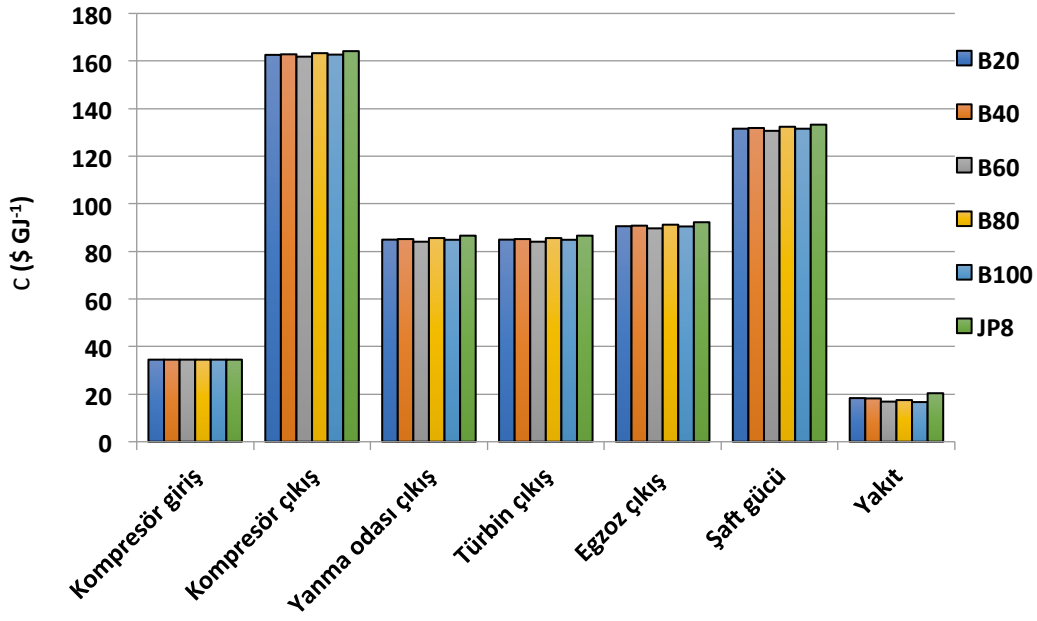
Şekil 4.27. 4.uçuş noktası için motor komponentleri özgül maliyetleri
