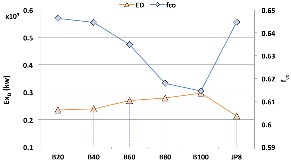
Şekil 4.33. 2. uçuş noktası için yanma odası ekserji yıkımı ve eksergoekonomik faktörün değişimi
