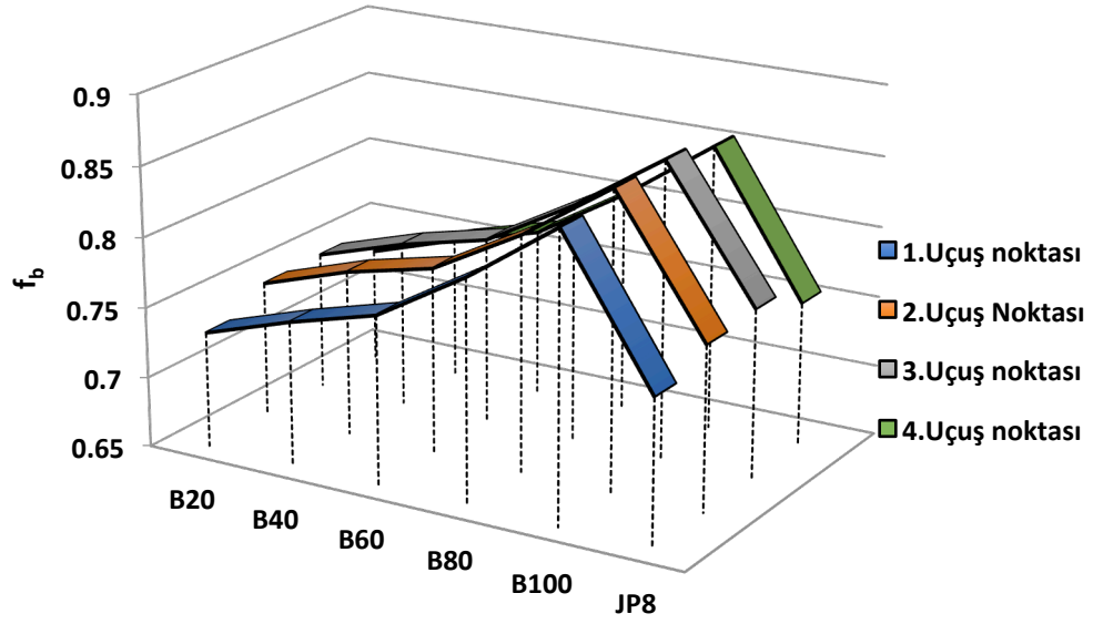
Şekil 4.43. Yanma odası için eksergoçevresel faktör parametresi
