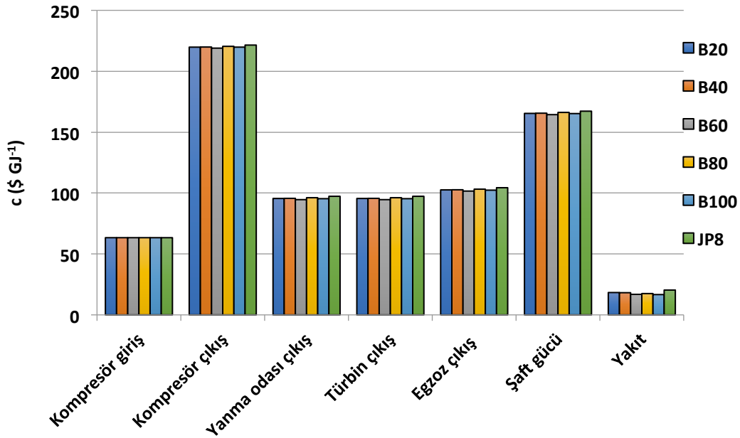
Şekil 4.25. 3.uçuş noktası için motor komponentleri özgül maliyetleri
