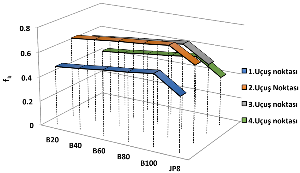
Şekil 4.44. Egzoz lülesi için eksergoçevresel faktör parametresi
