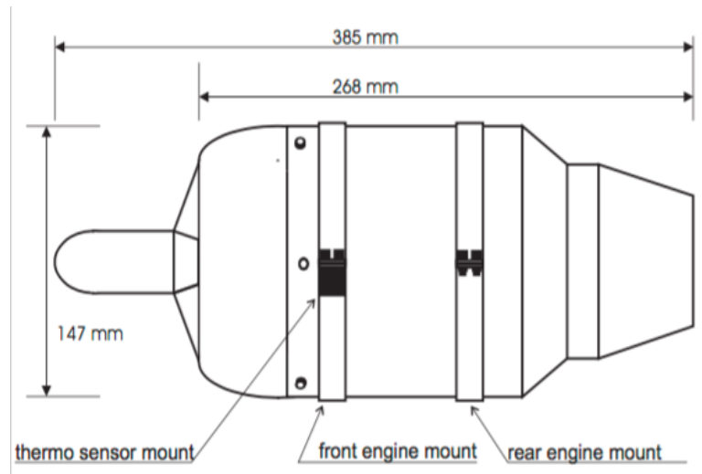
Şekil 4.2. AMT Titan turbojet motor boyutları [48]
