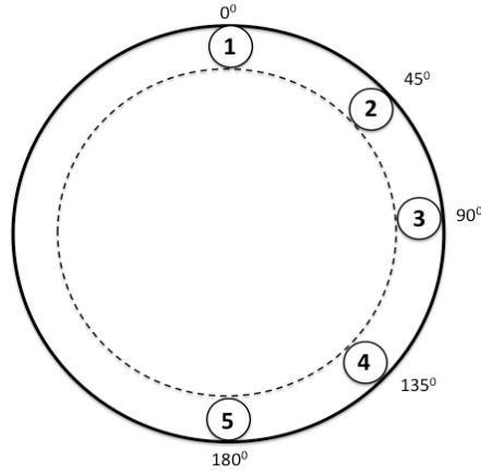
Şekil 4.11. Emisyon ölçüm noktaları (motor egzoz arkadan bakış)
