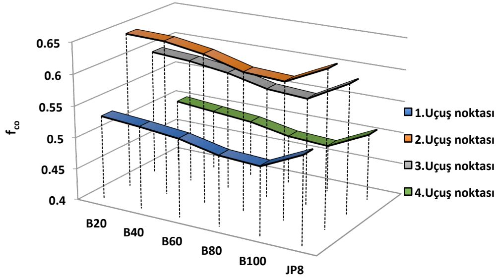
Şekil 4.32. Yanma odası için eksergoekonomik faktör parametresi
