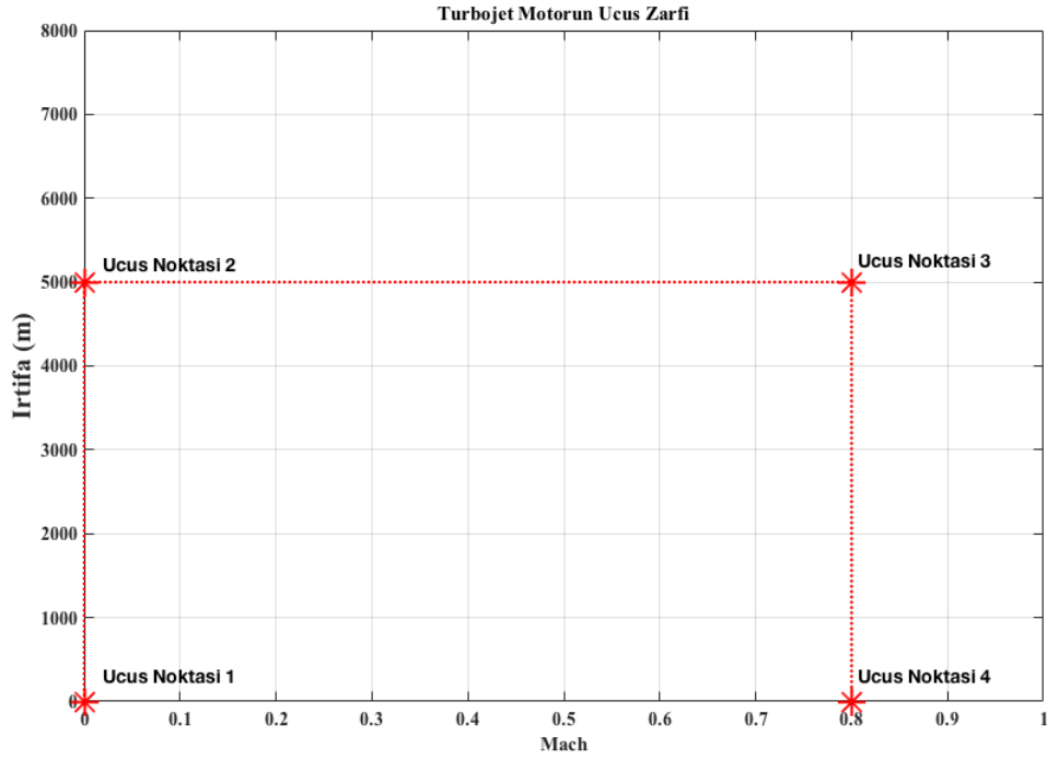
Şekil 4.14. Turbojet motor uçuş noktaları
