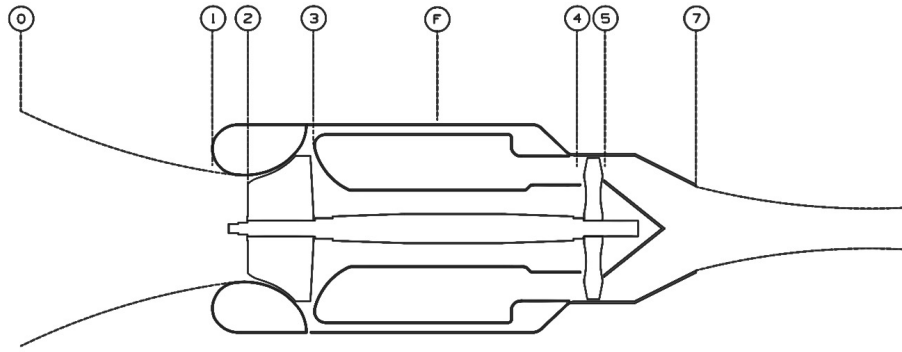
Şekil 3.2. Turbojet motor şematik gösterimi
