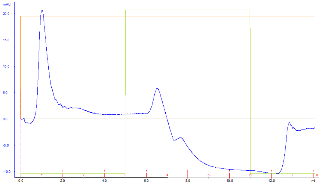
Şekil 3. 7. Poli(HEMA-ko-MATrp-Ru(bipyr) 2 -Biyotin) kriyojel kolonu ile Avidin saflaştırılmasına ait kromatogram
