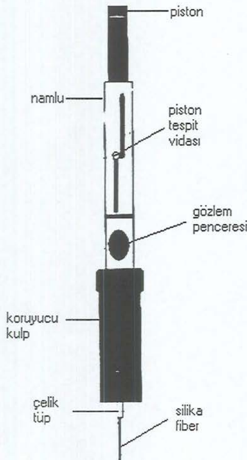
Şekil 1.1. KFME enjektörü
