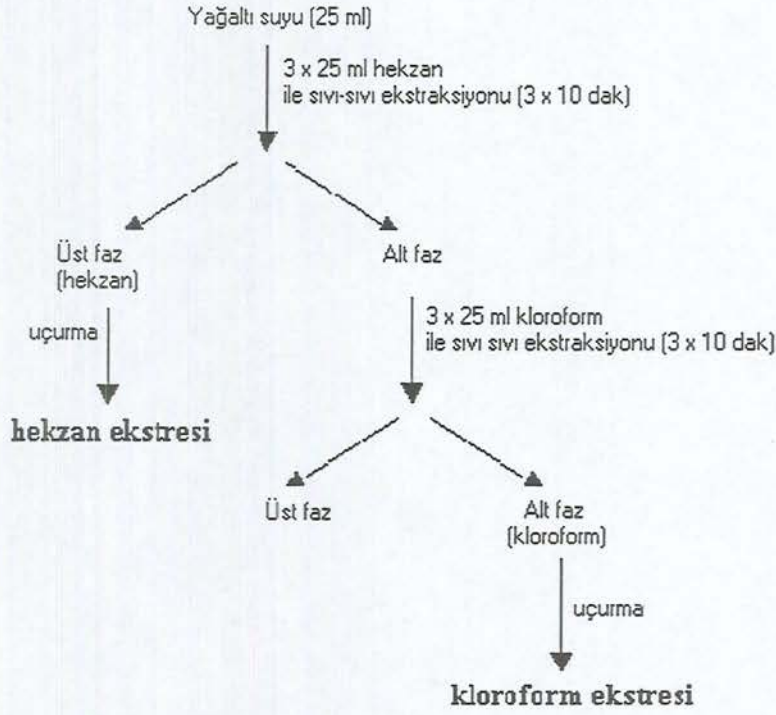
Şekil 2.1. Sıvı –Sıvı ekstraksiyonu şeması
