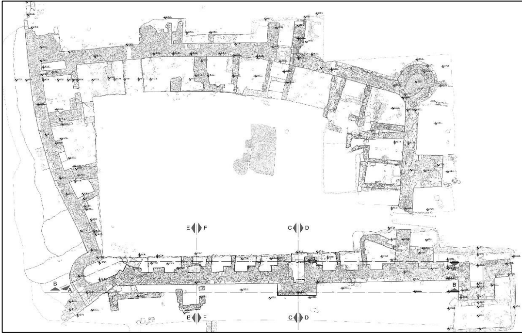
Şekil 8. İç Sur Alanı genel planı (Amorium Kazı Arşivi)
