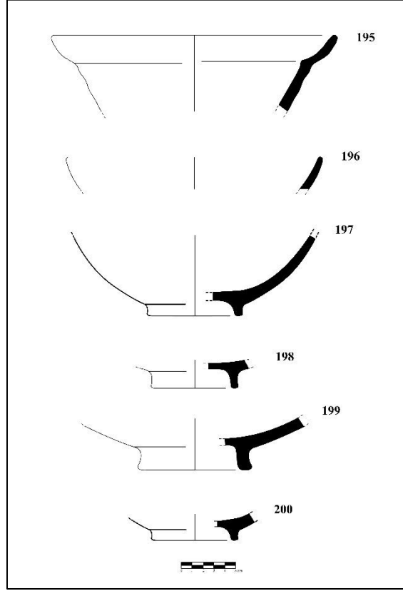
Çizim 26. Milet İşı yarı-küresel gövdeli ağız ve yüksek halka kaide örnekleri (Kat.195-200)
