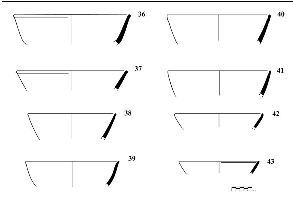
Çizim 6. Yeşil renk sırlı, yarı-küresel gövdeli hafif iç bükey ve dış bükey ağız profilli çanak örnekleri (Kat.25-35)
