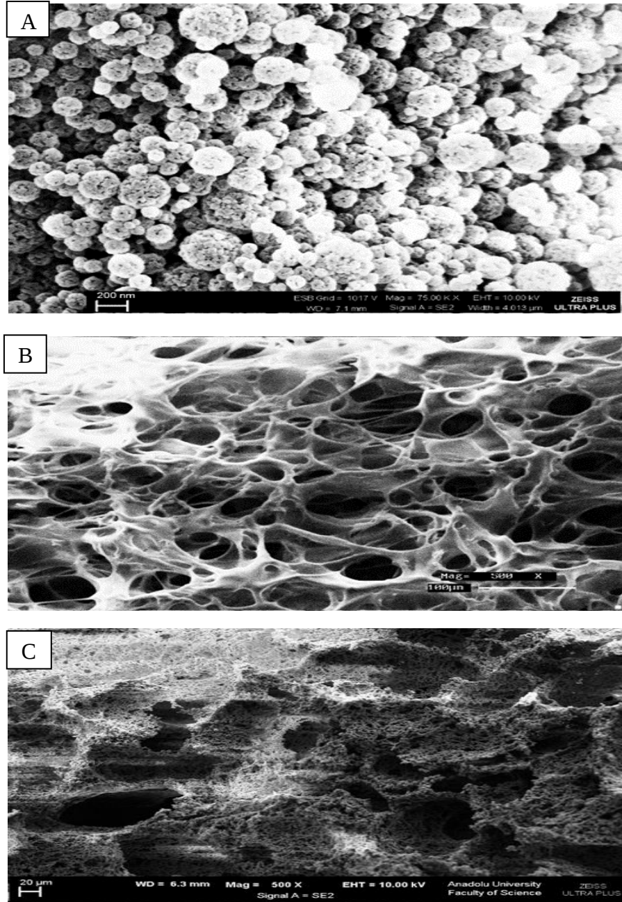
Şekil 4.2. (A) propaglor baskılı polimer, (B) boş kriyojel, (C) MIP gömülü kriyojelin SEM görüntüleri
