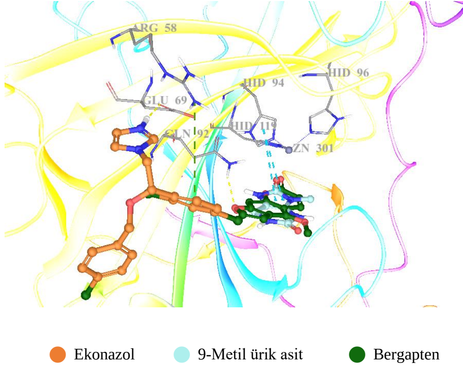
Şekil 5.19. Equisetum arvense ekstrelerinin içeriğinde tespit edilen başlıca etken maddelerin hCA II izoenzimi (PDB kodu: 5WLV) ile etkileşimi. A: Ekonazol'ün etkileşimi, B: 9-Metil ürik asit ve C: Bergapten'in etkileşimi.
