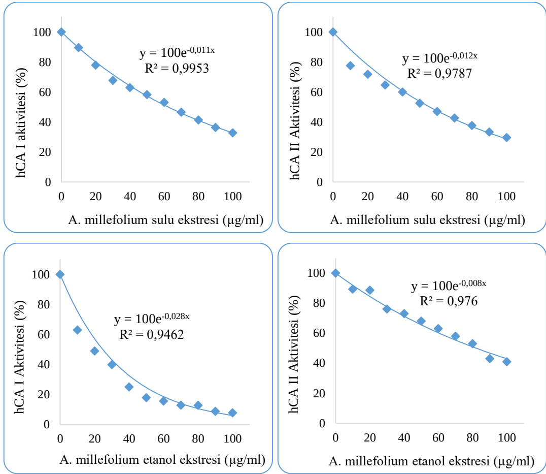
Şekil 5.42. hCA I ve II izoenzimlerinin CO 2 -Hidrataz aktivitesi üzerine A. millefolium bitki ekstraktlarının farklı konsantrasyonları kullanılarak IC 50 değerlerinin bulunması için çizilen [Aktivite(%)] – [İnhibitör] grafikleri
