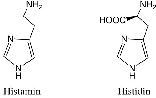
Şekil 1.12. CA I aktivatörleri (histamin ve histidin)
