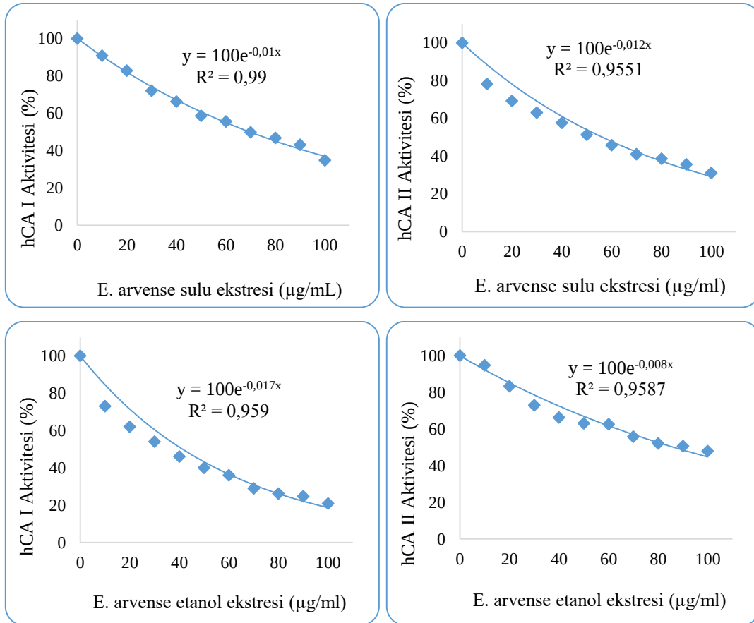
Şekil 5.40. hCA I ve II izoenzimlerinin CO 2 -Hidrataz aktivitesi üzerine E. arvense bitki ekstrelerinin farklı konsantrasyonları kullanılarak IC 50 değerlerinin bulunması için çizilen [Aktivite(%)] – [İnhibitör] grafikleri
