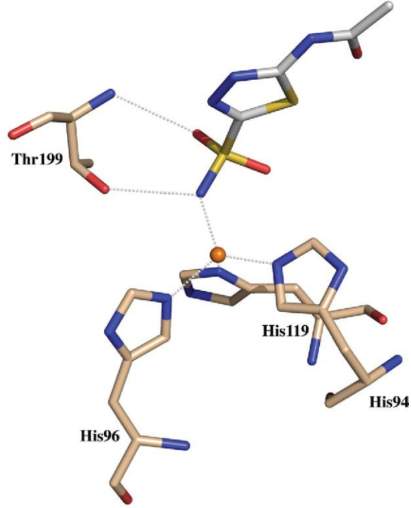
Şekil 1.11. Sülfonamidlerin CA I aktif bölgesine bağlanma şekli [33]
