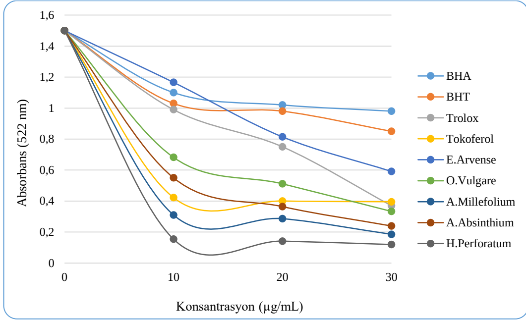
Şekil 5.76. Farklı konsantrasyonlardaki (10-30 µg/mL) su ile hazırlanan bitki ekstralarının metal şelatlama kapasitelerinin standart antioksidanlar olan BHA, BHT, Trolox ve α-Tokoferol ile karşılaştırılması
