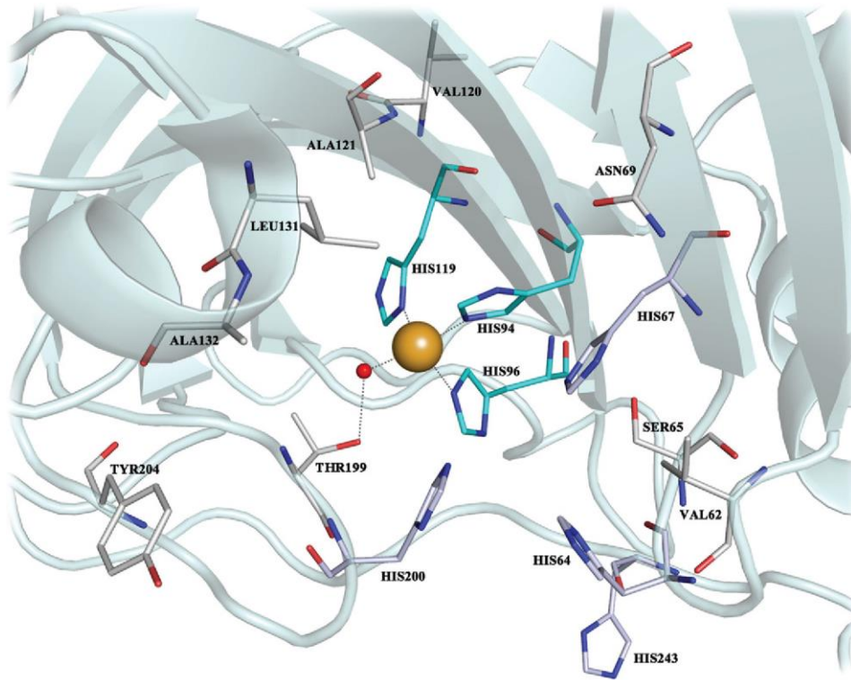
Şekil 1.9. CA I katalitik aktif bölgesi (PDB ID: 2FW4) [21]
