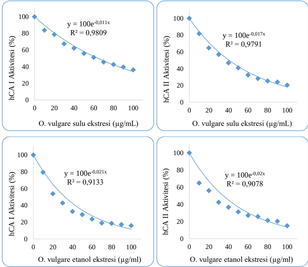
Şekil 5.41. hCA I ve II izoenzimlerinin CO_2 -Hidrataz aktivitesi üzerine O. vulgare bitki ekstralarının farklı konsantrasyonları kullanılarak IC_{50} değerlerinin bulunması için çizilen [Aktivite(%)] – [İnhibitör] grafikleri
