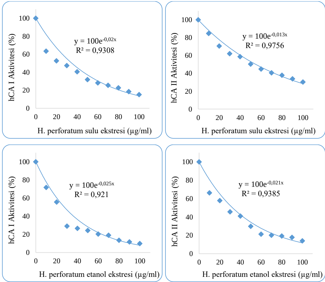
Şekil 5.44. hCA I ve II izoenzimlerinin CO 2 -Hidrataz aktivitesi üzerine H. perforatum bitki ekstraktlarının farklı konsantrasyonları kullanılarak IC 50 değerlerinin bulunması için çizilen [Aktivite(%)] – [İnhibitör] grafikleri
