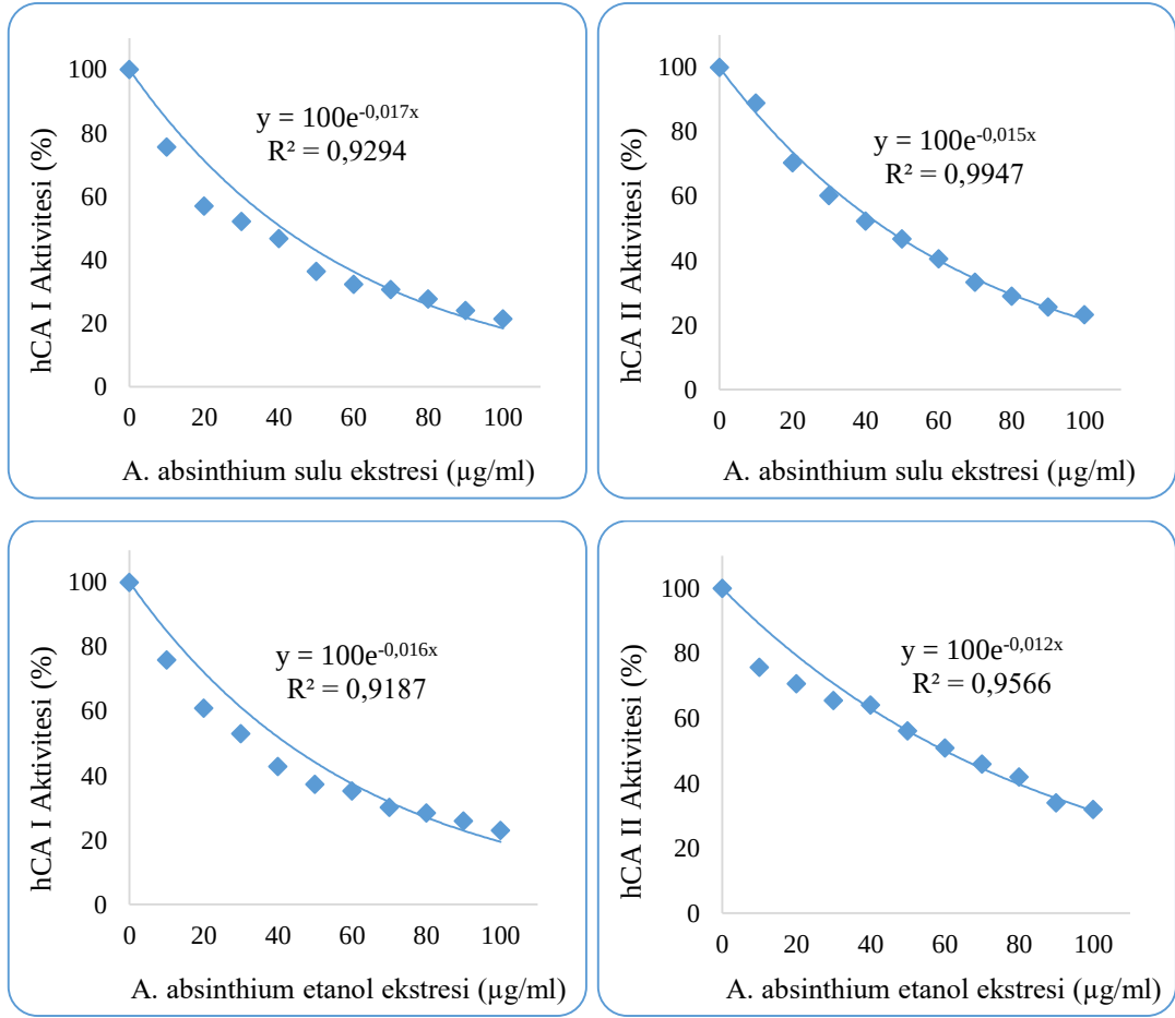
Şekil 5.43. hCA I ve II izoenzimlerinin CO 2 -Hidrataz aktivitesi üzerine A. absinthium bitki ekstralarının farklı konsantrasyonları kullanılarak IC 50 değerlerinin bulunması için çizilen [Aktivite(%)] – [İnhibitör] grafikleri
