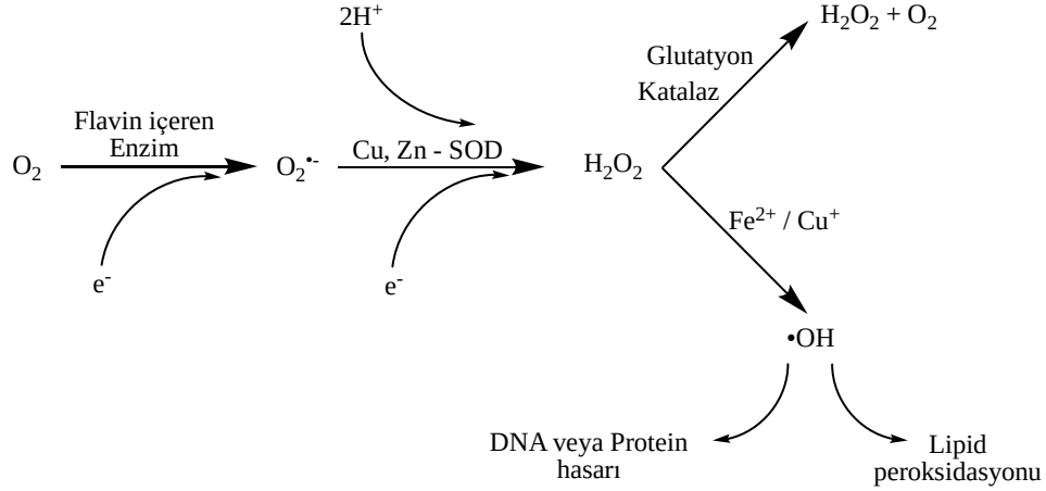
Şekil 1.21. ROS oluşumu ve hücre içi düzeyde metabolizma için basitleştirilmiş şeması [68]
