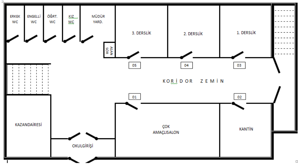
Görsel 2.3. Araştırma okulu zemin kat planı
