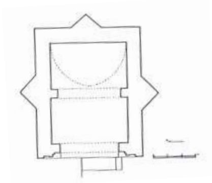
Çizim 3.7. Boyalıköy Eyvan Türbe planı (Önkal, 1996, )
