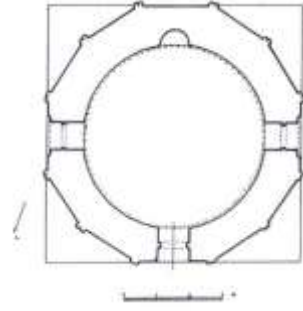
Çizim 3.27. Erzurum Gümüşlü Kümbet planı (Önkal, 1997, 206)
