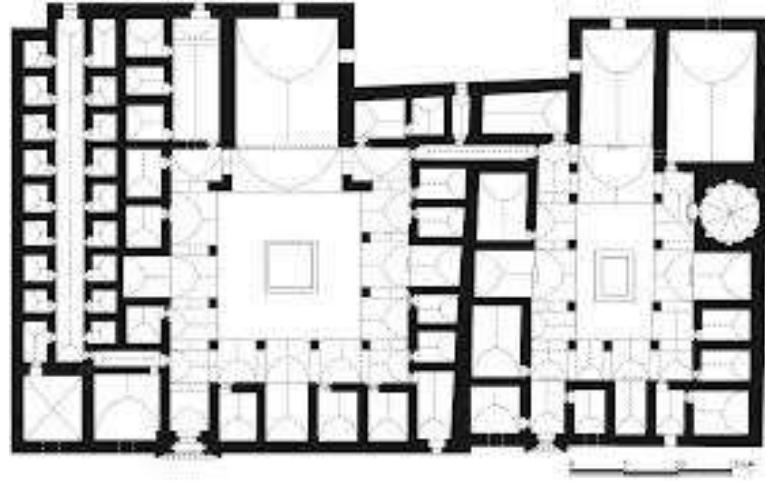
Çizim 2.7. Melike Gevher Nesibe Hatun Medrese ve Darüşşifası planı (Kutlu, 2017, 367)
