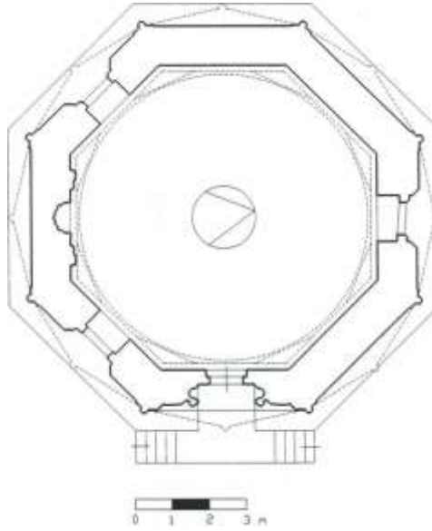
Çizim 2.13. Hüdevend Hatun Türbesi planı (Özkarıcı,1996, Çiz. 99)
