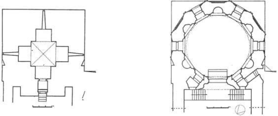
Çizim 2.16. Hatuniye Medresesi türbesi cenazelik ve mescit mekânı planı (Erzurum Vakıflar bölge müdürlüğü, 2017’de işlenerek düzenlenmiştir)
