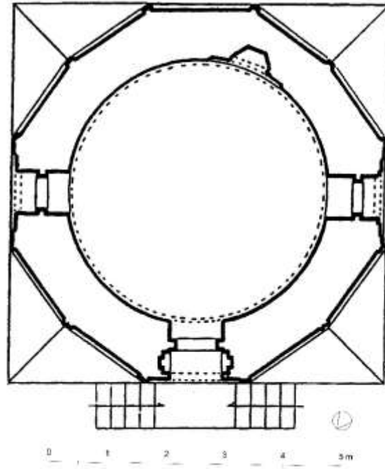
Çizim 2.17. Şah Cihan Hatun Türbesi planı (Önköl, 1996, 196)
