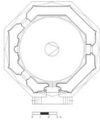
Çizim 3.23. Niğde Hüdavend Hatun Türbesi planı (Özkarıcı, 'üzerinden işlenerek düzenlenmiştir)
