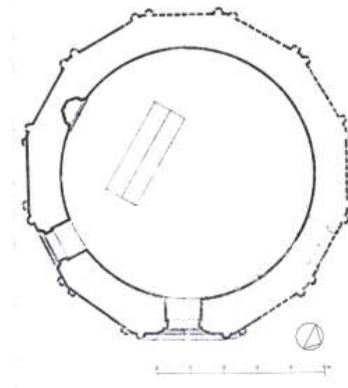
Çizim 2.18. Rabia Hatun Türbesi planı (Tuncer, 1991, 201'den işlenerek düzenlenmiştir)
