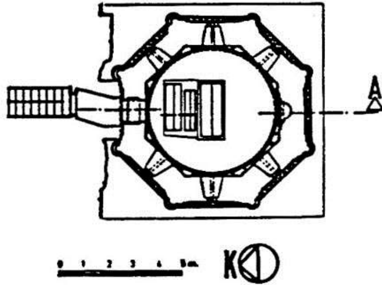
 izim 2.11. Mahperi Huand Hatun T rbesi planı (Parla,1997 , iz.97  zerinden  şlernerek d zenlenmiřtir)
