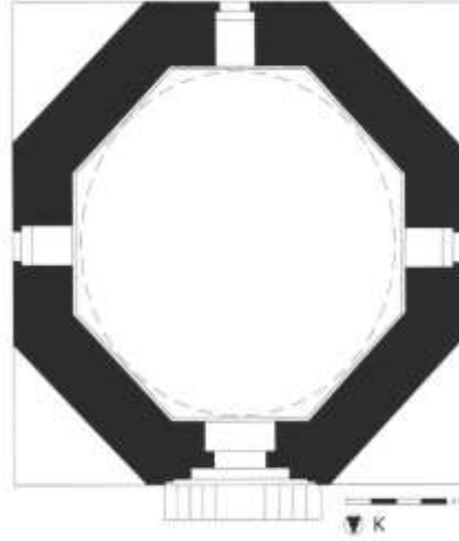
Çizim 2.12. Fatma Hatun Türbesi planı (Önkal, 1996, 162'den işlenerek düzenlenmiştir)
