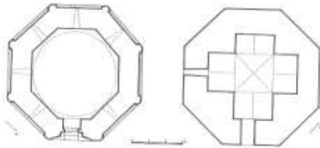
Çizim 3.28. Aksaray Selime Sultan Türbesi planı (Önkal, 1996, 90)
