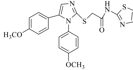
Şekil 5.9. Bileşik 8
