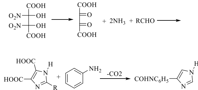
Şekil 2.12. Formaldehit ve tartarik asit dinitrattan hareketle imidazol sentez şeması
