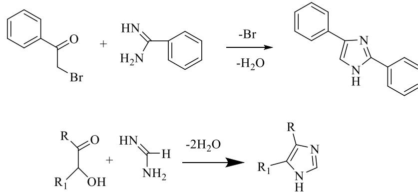
Şekil 2.8. Alfa haloketondan hareketle imidazol sentez şeması
