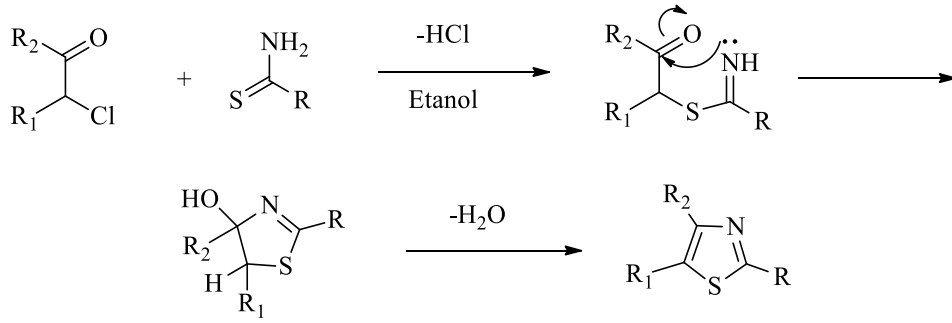
Şekil 2.23. Hantzsch tiyazol sentezinin genel gösterimi
