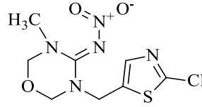
Şekil 2.31. Tiyametoksam molekülü
