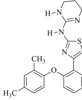
Şekil 2.30. Abafungin molekülü
