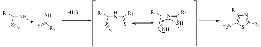
Şekil 2.25. Cook – Heilbron tiyazol sentez şeması
