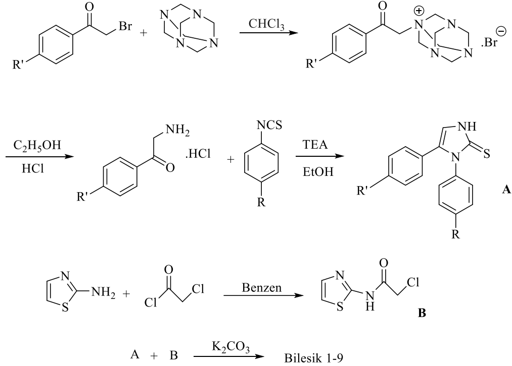
Şekil 5.11. 2-[(1,5-disübstitüe fenil-1 H -imidazol-2-il)tiyo]- N -(tiyazol-2-il)asetamid türevleri sentez şeması
