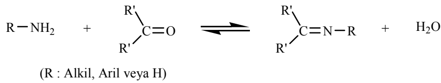
Şekil 2.1. Schiff baz oluşumuna ait genel reaksiyon
