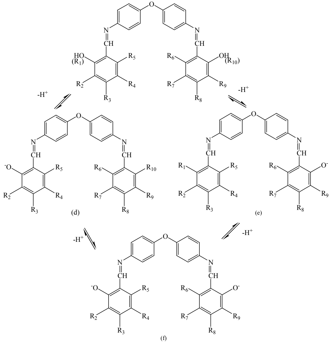
Şekil 6.7. Çalışılan 4,4'-oxydianilin türevleri için deprotonlanma şeması genel şeması
