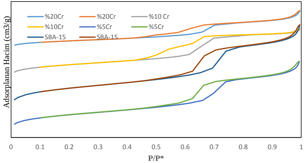
Şekil 8.17. %5, %10, %20 Cr_3(PW_{12}O_{40})_3 /SBA-15 ve SBA-15 katalizörlerinin N_2 Adsorpsiyon/Desorpsiyon izotermeleri
