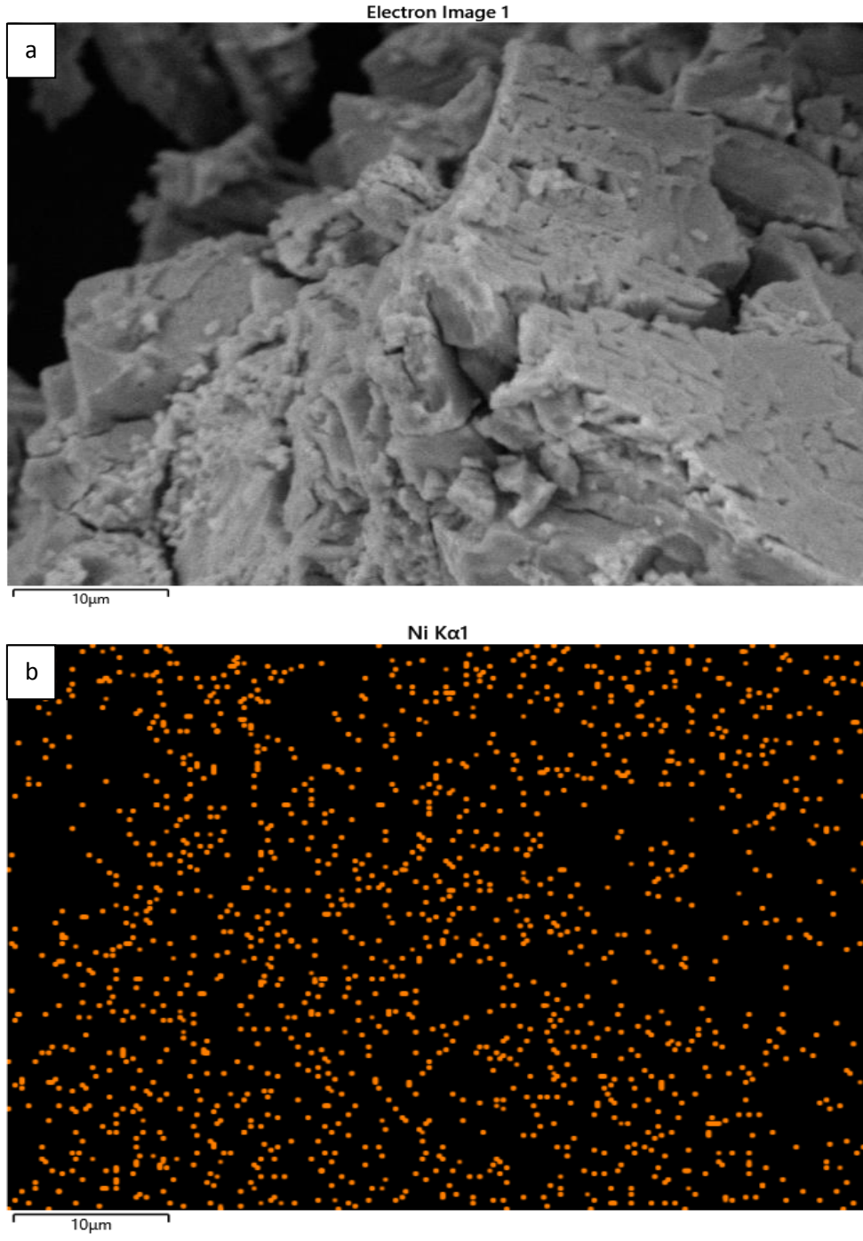
Şekil 8.5. \text{Ni}_3(\text{PW}_{12}\text{O}_{40})_2 katalizörünün, a-)SEM görüntüsü b-) SEM-EDX yüzey haritası c-)EDX spektrumu
