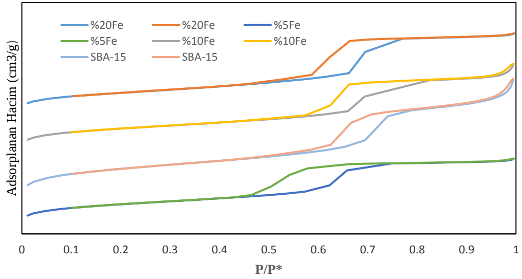
Şekil 8.16. %5, %10, %20 Fe_3(PW_{12}O_{40})_3 /SBA-15 ve SBA-15 katalizörlerinin N_2 Adsorpsiyon/Desorpsiyon izotermeleri
