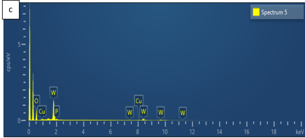
Şekil 8.4. (Devam) \text{Cu}_3(\text{PW}_{12}\text{O}_{40})_2 katalizörünün, a-)SEM görüntüsü b-) SEM-EDX yüzey haritası c-)EDX spektrumu
