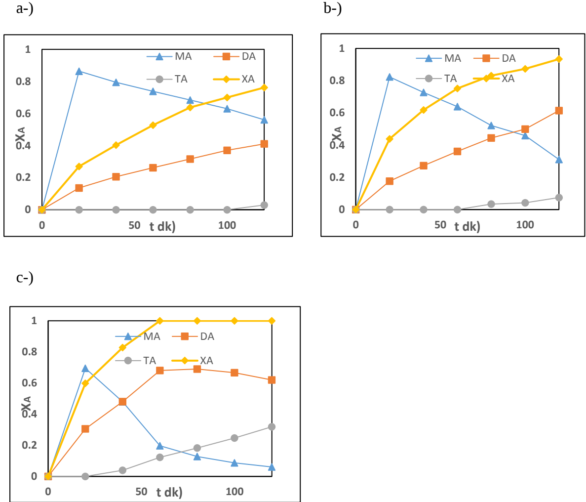
Şekil 8.27. Gliserol asetik asit reaksiyonu %20 \text{Fe}_3(\text{PW}_{12}\text{O}_{40})_3/\text{SBA-15} katalizörü'nün
