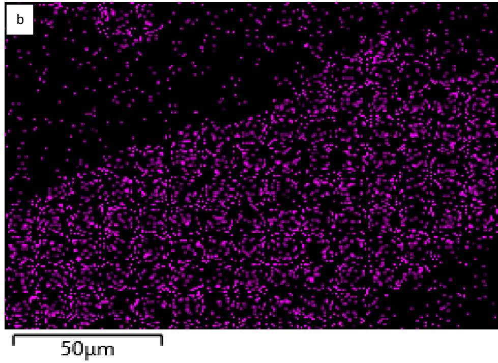
Şekil 8.3. \text{Cr}_3(\text{PW}_{12}\text{O}_{40})_3 katalizörünün, a-)SEM görüntüsü b-) SEM-EDX yüzey haritası c-)EDX spektrumu
