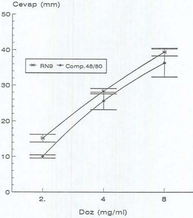
kil 4.11. Kobay ileumunda RN1 ve RN9'un kastırıcı etkisi üzerine 48/80 maddesinin etkisi (48/80 Maddesi: 3 \times 10^{-2} mg/L)
