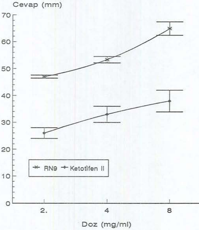
Şekil 4.9. Kobay ileumunda RN9'in kastırıcı etkisi üzerine ketotifenin etkisi (Ketotifen I: 3.09 \times 10^{-4} g/L ve ketotifen II: 3.09 \times 10^{-6} )
