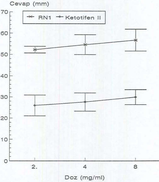
Şekil 4.8. Kobay ileumunda RN1'in kastırıcı etkisi üzerine ketotifenin etkisi (Ketotifen I: 3.09 \times 10^{-4} g/L ve ketotifen II: 3.09 \times 10^{-6} g/L)
