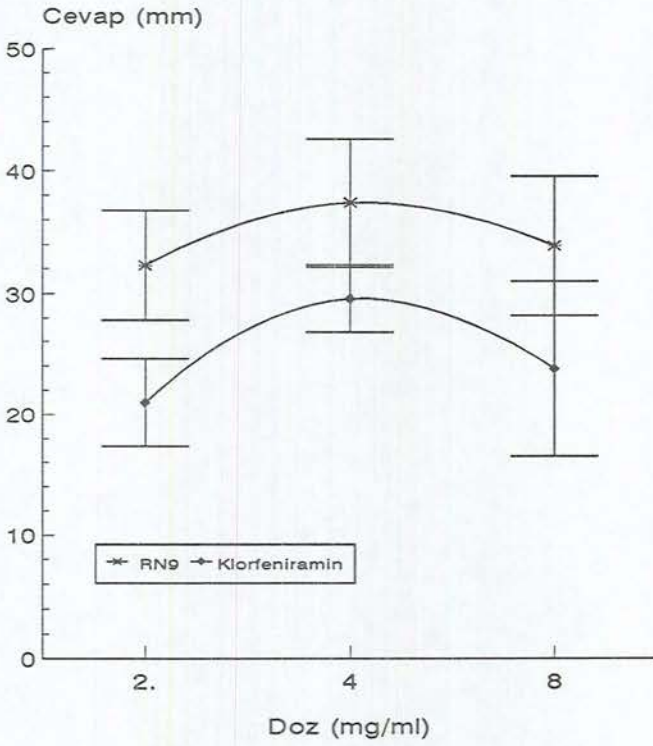
ekil 4.6. Kobay ileumunda RN1 ve RN9'un kastırıcı etkisi üzerine klorfeniraminin etkisi (Klorfeniramin 2 \times 10^{-6} g/L)
