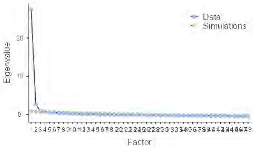
Şekil 3.8. Öğretmenlerin mesleki ve teknik eğitim kurumlarında endüstri 4.0 uygulamalarının kullanımına ilişkin algı ölçeği (ED 4.0-ÖAÖ)'nin faktör analizine ilişkin yamaç birikinti (scree plot) grafiği
