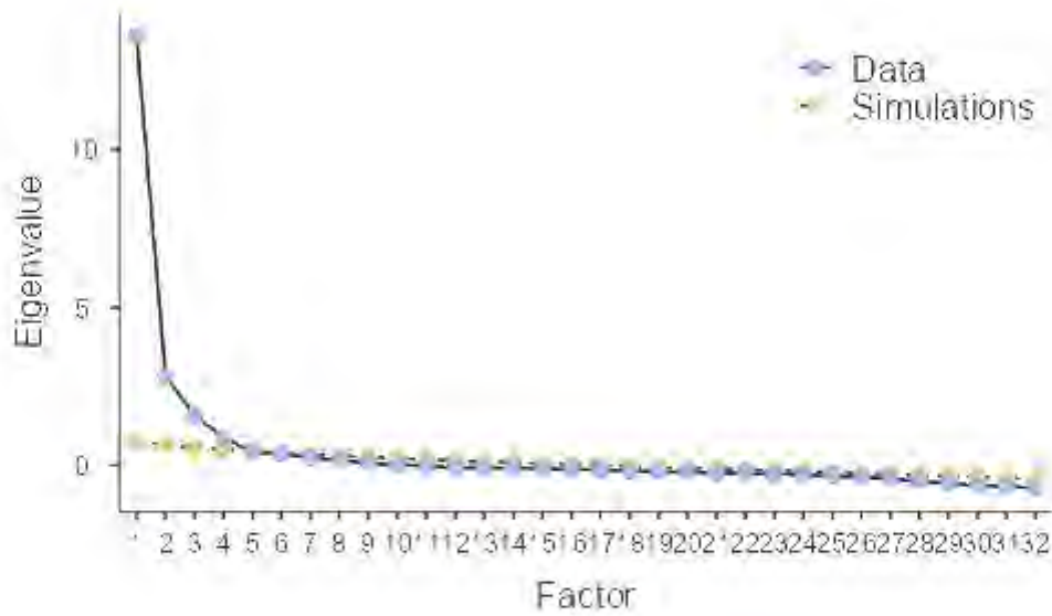
Şekil 3.5. Mesleki ve teknik anadolu liselerindeki öğretmenlerin endüstri 4.0 uygulamalarını kabul ve kullanım niyeti ölçeği (ED 4.0-ÖKKNÖ)'nin faktör analizine ilişkin yamaç birikinti (scree plot) grafiği
