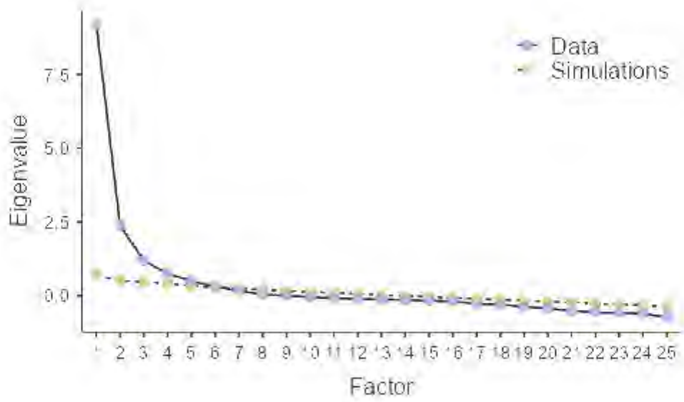
Şekil 3.2. Mesleki ve teknik eğitim öğretmenlerinin endüstri 4.0'a ilişkin hazırbulunuşluk ölçeği (ED 4.0-ÖHÖ)'nin faktör analizine ilişkin yamaç birikinti (scree plot) grafiği
