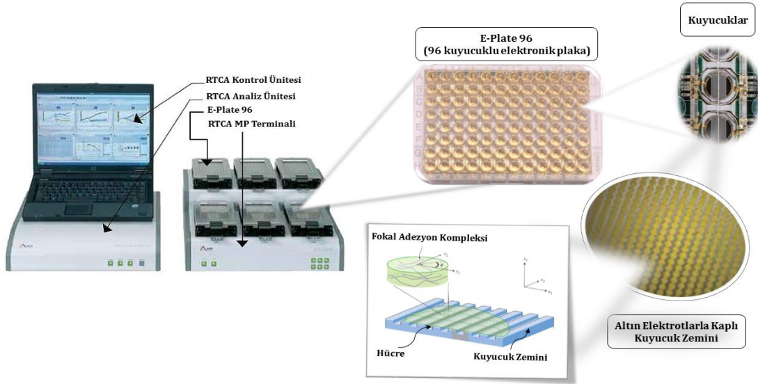
Şekil 2.3. Gerçek zamanlı hücre analiz sistemi (RTCA) MP modeli tanıtımı ve çalışma prensibi
