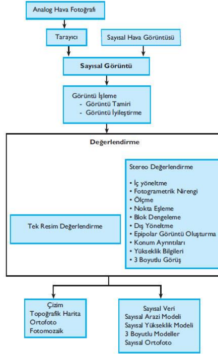
Şekil 4. 4. Fotogrametrik iş akış planı
