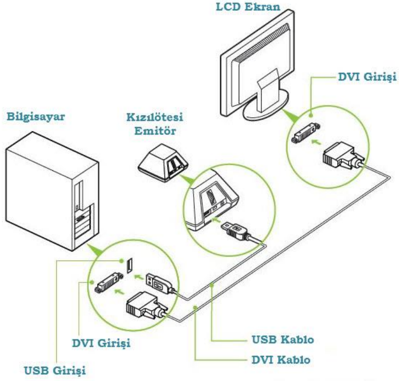
Şekil 5. 4. Stereo sistem donanımları ve bağlantıları (Http-8)
