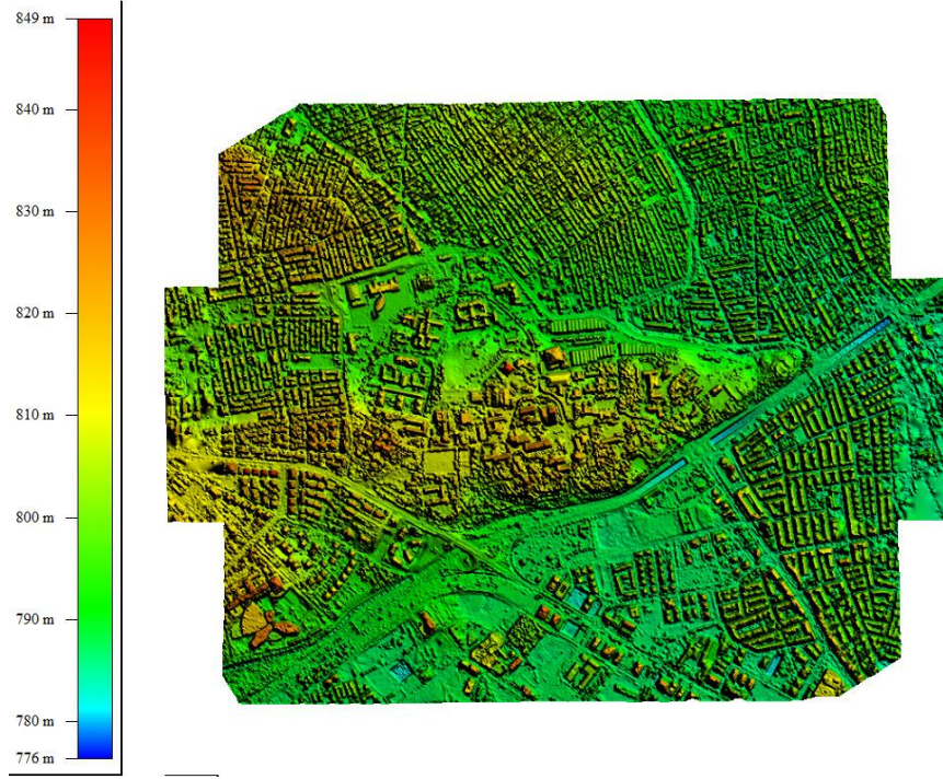
Şekil 6. 6. Agisoft Photoscan ile üretilen SYM verisi örneği (Kaynak: Yazar tarafından üretilmiştir.)
