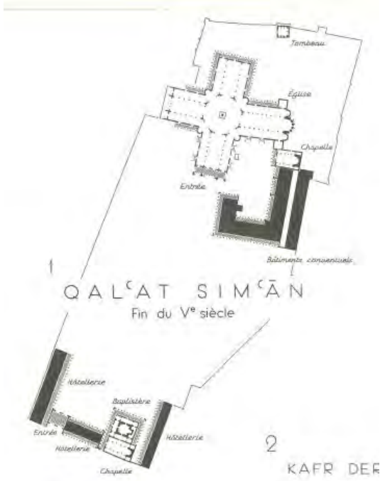
Çizim 61. Qal'at Sem'an Kilisesi Vaftizhanesi, (Tchalenko, G. (1953).
