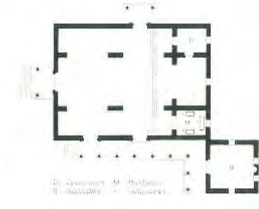
Çizim 53. Bamugga Vaftizhanesi (VI-VII. Yüzyıl), Tchalenko, G. (1953).
