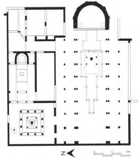
Çizim 70. Kartaca Dermech I Nolu Bazilikası Vaftizhanesi, Burns J. Patout - Jensen M. Robin. (2014).
