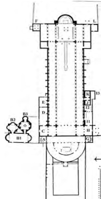
Çizim 48. Lechaion Bazilikası
