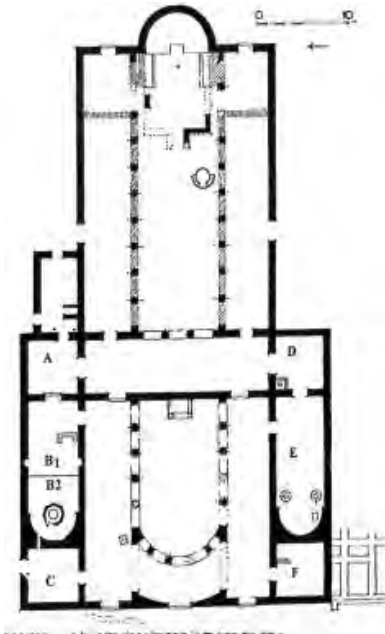
Çizim 46. Nea Anchialos A Bazilikası
