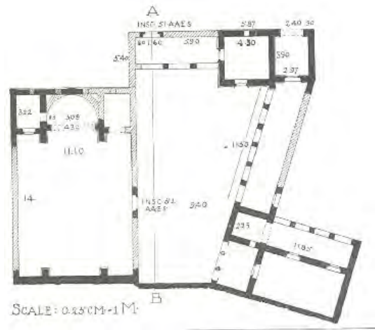
Çizim 56. Bâkirhâ Vaftizhanesi, H. C. Butler, (1929).
