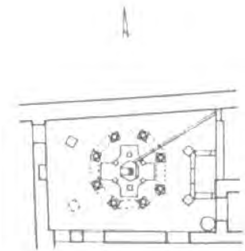
Çizim 82. Lucca Vaftizhanesi ve Vaftiz Havuzu (500)
