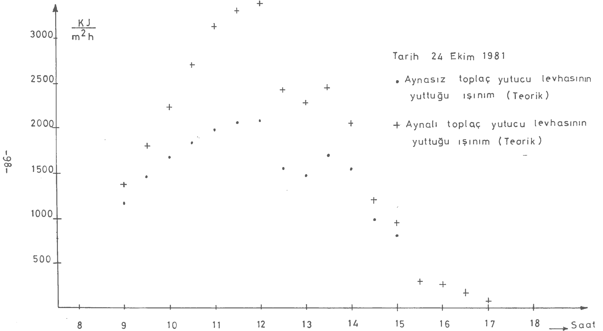
Şekil (4.17) Aynalı ve Aynasız toplaç yutucu levhalarının yuttuğu ışıınımların
