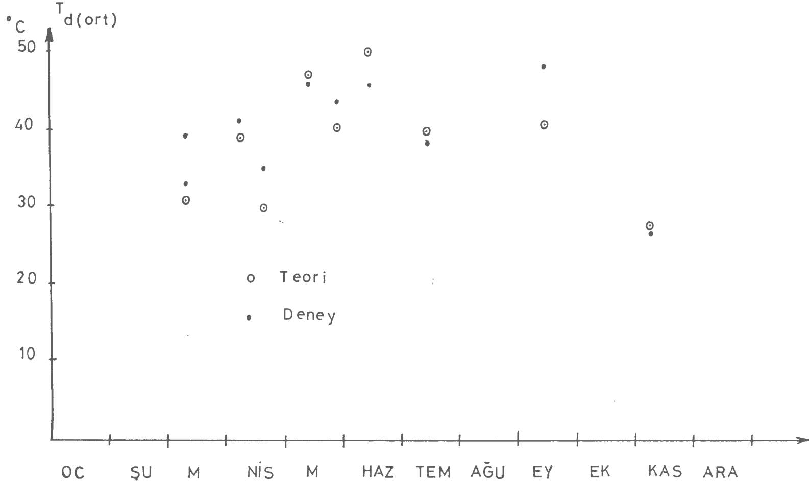
Şekil (4.14) Sene boyunca (Ekim 1981 - Ekim 1982) depo deney sonu sıcaklığının Doğal akış formülasyonunu (Program III) sonuçları ile karşılaştırılması
