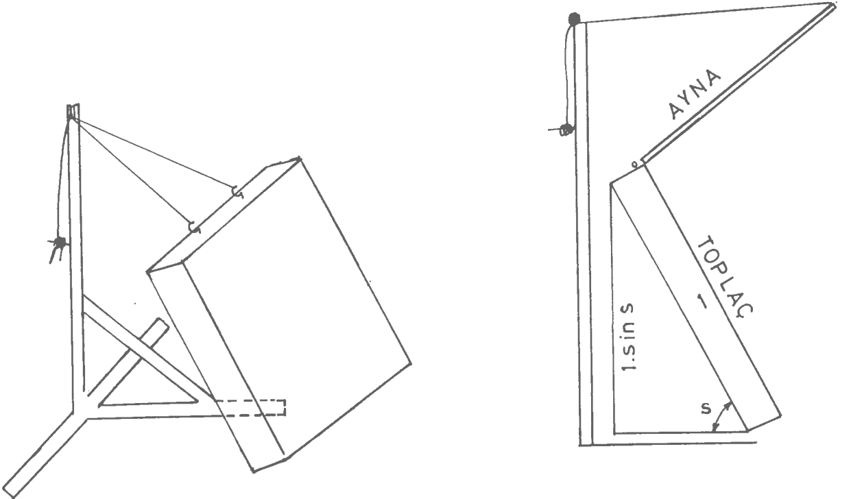
Sekil (4.11) Toplaç perspektif ve aynalı toplaçın yandan görünüş resmi
