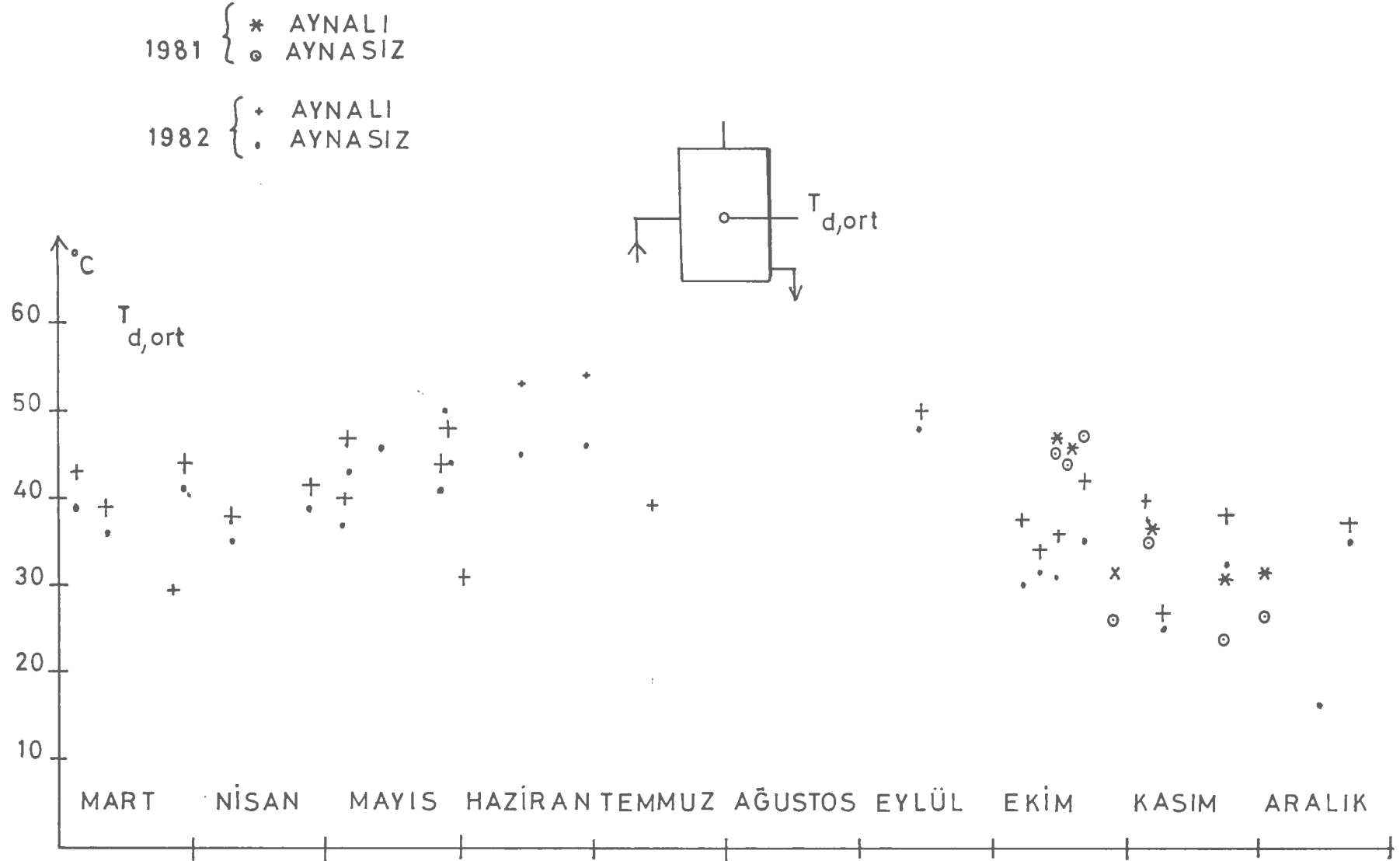
Şekil (4.20) 1981 ve 82 senesinde Aynasız ve Aynalı Toplaç depolarının elde edilen maksimum ortalama sıcaklıkları ( m_{\text{ort}} = 0 )
