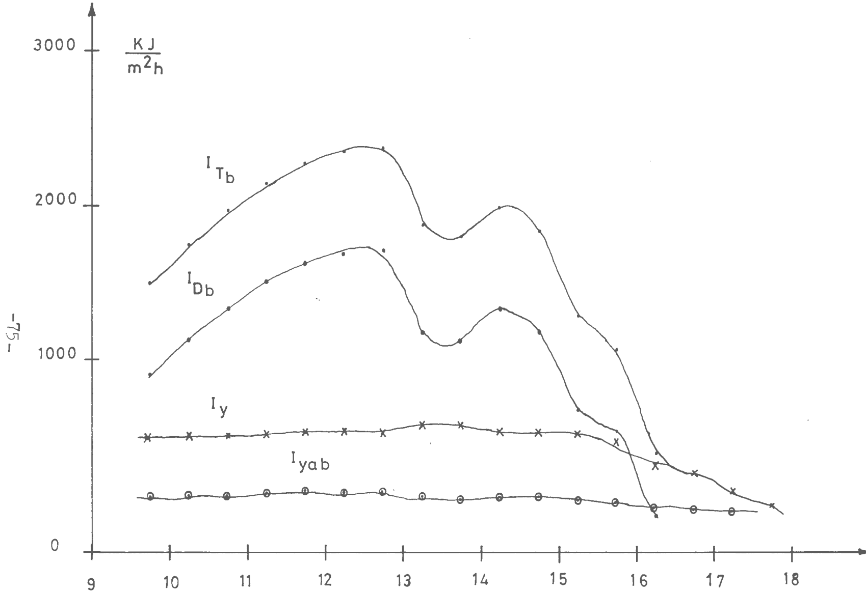
Şekil(4.3) 24.10.1981 Tarihinde Bulutlu halde yansıyan I_{yab} , yayılı I_y , Direkt I_{Db} ve Toplam I_{Tb} ışınım şiddetlerinin gün boyunca değişimi (Eskişehir)
