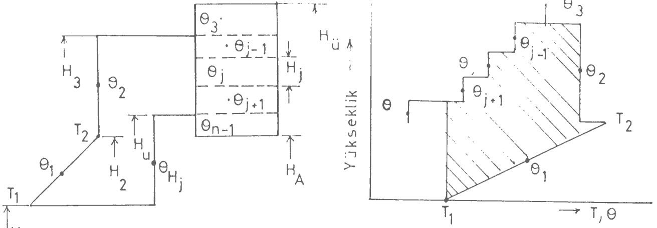
Şekil (2.4) Toplaç ve depo sisteminin parçalara Bölünmüş sekli bu halde yükseklik sıcaklık diyagramı
