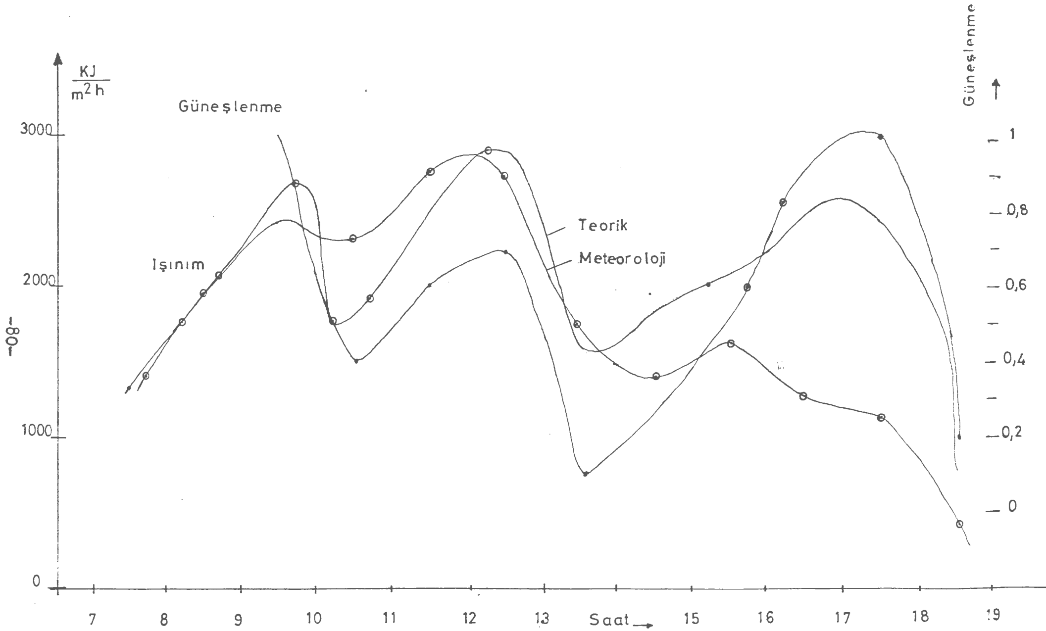
Sekil(47) 14.7.1982 Tarihinde Güneş ışınlm siddeti ve Güneşlenmenin günlük değışimleri
