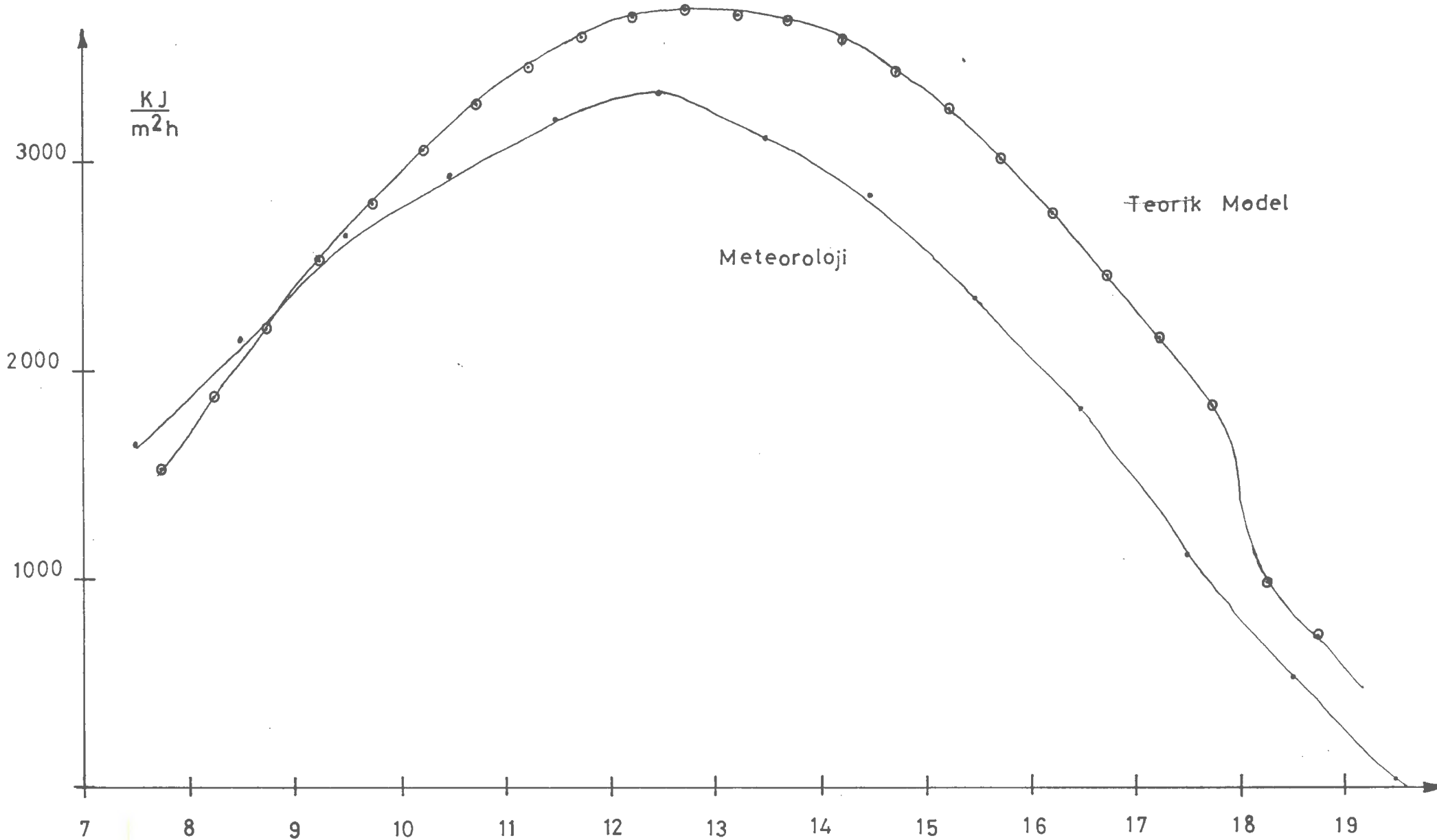
Şekil (46) 14.6.1982 Tarihinde teorik model ile Meteoroloji ölçümlerinin karşılaştırılması
