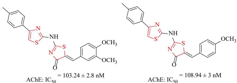
Figure 2.27. (Z)-5-(3,4-Dimethoxybenzylidene)-2-[(4-(p-tolyl)thiazol-2-yl)amino]thiazol-4(5H)-one (left) (Z)-5-(4-Methoxybenzylidene)-2-[(4-(p-tolyl)thiazol-2-yl)amino]thiazol-4(5H)-one (Right)
