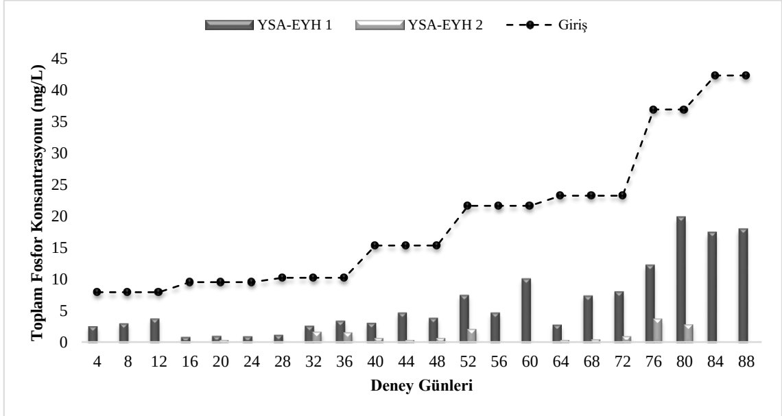
Şekil 3. 39. Yapay sulak alan ekolojik yakıt hücresi 2 modülünün çıkış suyunun araştırma periyodu içerisindeki giriş ve yapay sulak alan ekolojik yakıt hücresi 1 modülünün çıkış suyuna göre ortalama toplam fosfor konsantrasyonu (mg/L) değişimi
