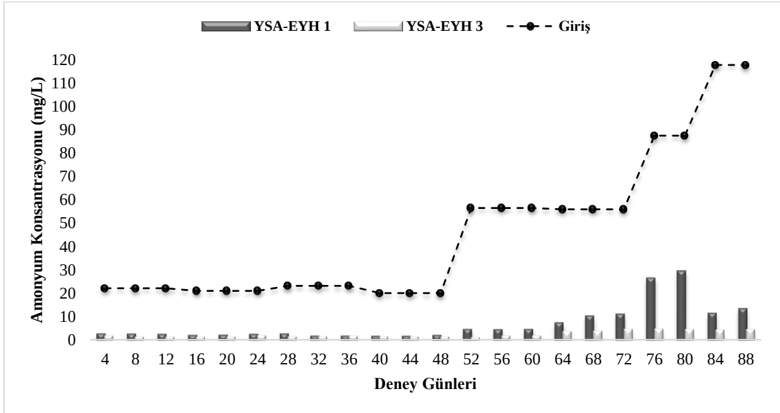
Şekil 3. 28. Yapay sulak alan ekolojik yakıt hücresi 3 modülünün çıkış suyunun araştırma periyodu içerisindeki giriş ve yapay sulak alan ekolojik yakıt hücresi 1 modülünün çıkış suyuna göre ortalama amonyum konsantrasyonu (mg/L) değişimi
