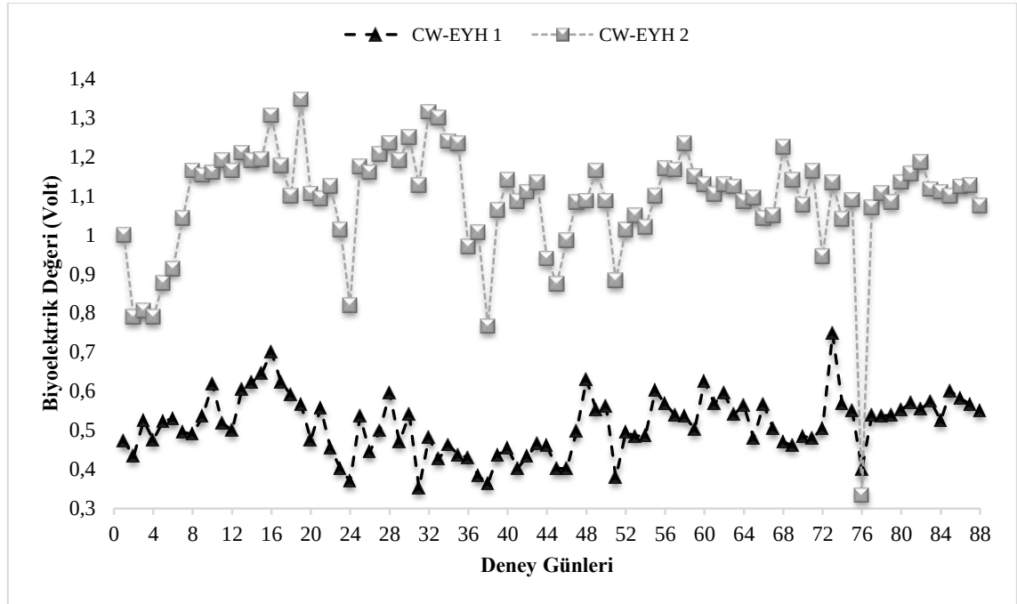
Şekil 3. 52. Araştırma periyodu içerisinde yapay sulak alan ekolojik yakıt hücresi 1 modülü ve yapay sulak alan ekolojik yakıt hücresi 2 modülünün biyoelektrik üretim değerleri(mV) değişimi
