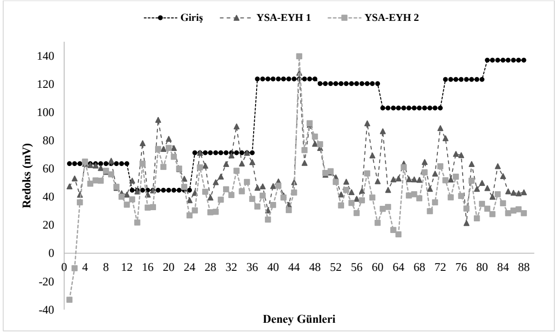
Şekil 3. 13. Yapay sulak alan ekolojik yakıt hücresi 2 modülünün çıkış suyunun araştırma periyodu içerisindeki giriş ve yapay sulak alan ekolojik yakıt hücresi 1 modülünün çıkış suyuna göre redoks (mV) değişimi
