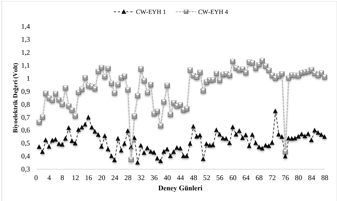
Şekil 3. 54. Araştırma periyodu içerisinde yapay sulak alan ekolojik yakıt hücresi 1 modülü ve yapay sulak alan ekolojik yakıt hücresi 4 modülününün biyo elektrik üretim değerleri(mV) değişimi
