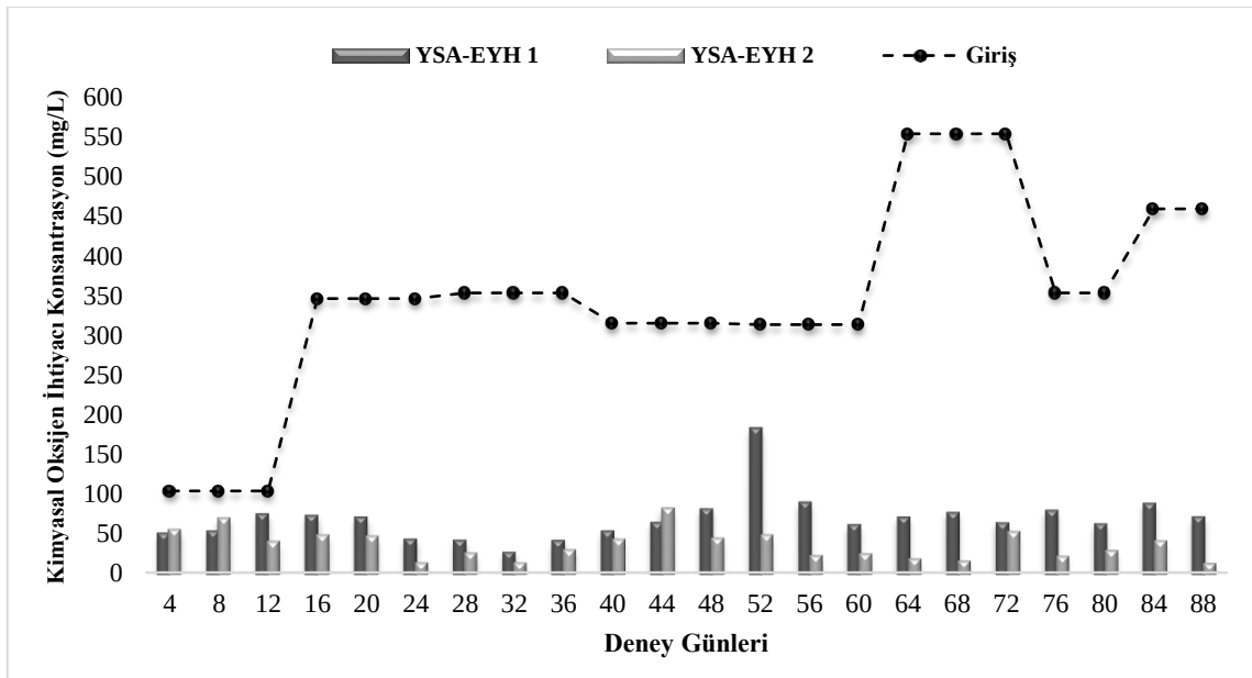
Şekil 3. 21. Yapay sulak alan ekolojik yakıt hücresi 2 modülünün çıkış suyunun araştırma periyodu içerisindeki giriş ve yapay sulak alan ekolojik yakıt hücresi 1 modülünün çıkış suyuna göre kimyasal oksijen ihtiyacı konsantrasyonu (mg/L) değişimi
