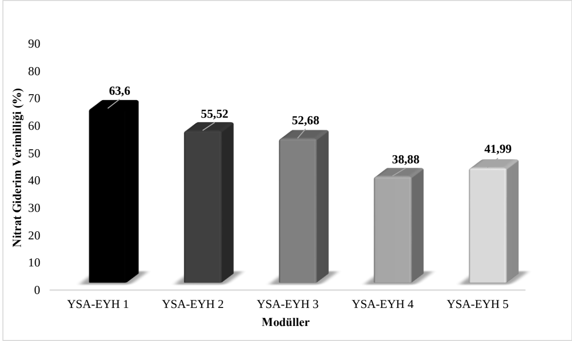
Şekil 3. 38. Yapay sulak alan ekolojik yakıt hücresi modüllerinin çıkış sularının araştırma periyodu içerisindeki ortalama nitrat giderim verimliliği (%)
