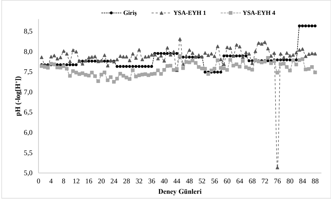
Şekil 3. 3. Yapay sulak alan ekolojik yakıt hücresi 4 modülünün çıkış suyunun araştırma periyodu içerisindeki giriş ve yapay sulak alan ekolojik yakıt hücresi 1 modülünün çıkış suyuna göre pH değişimi
