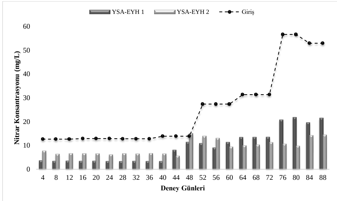
Şekil 3. 33. Yapay sulak alan ekolojik yakıt hücresi 2 modülünün çıkış suyunun araştırma periyodu içerisindeki giriş ve yapay sulak alan ekolojik yakıt hücresi 1 modülünün çıkış suyuna göre ortalama nitrat konsantrasyonu (mg/L) değişimi
