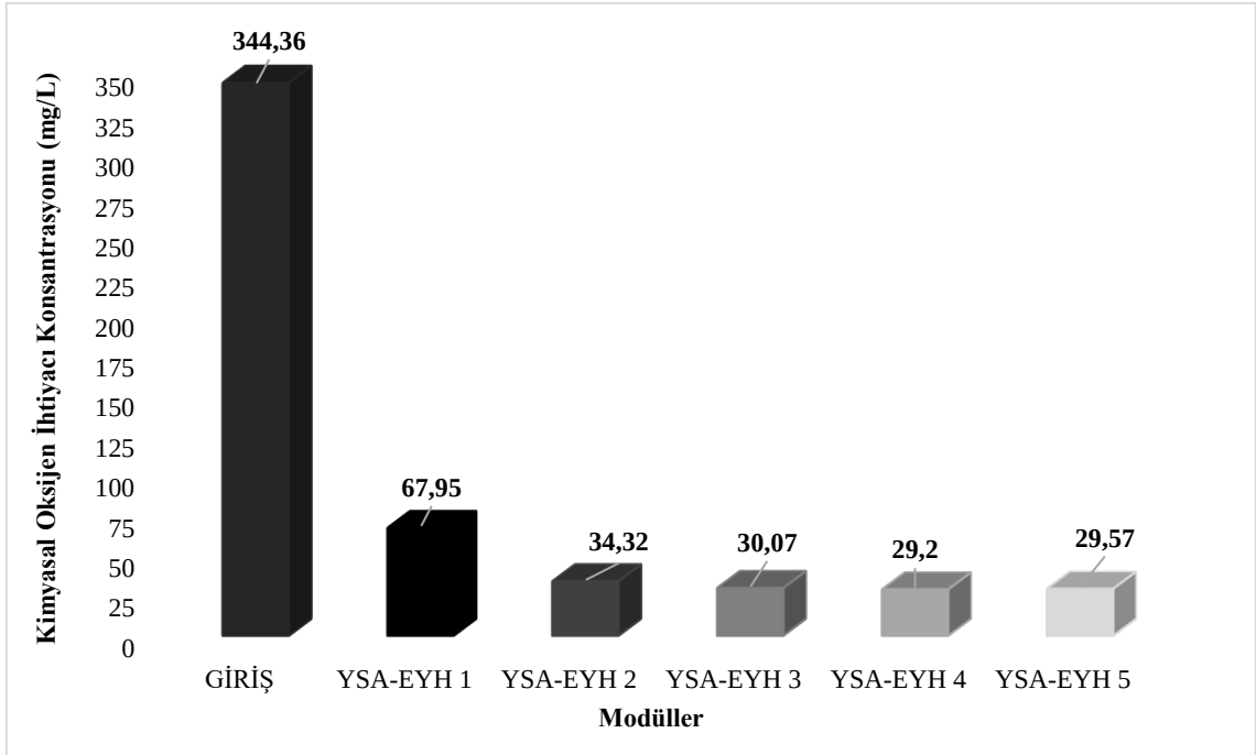
Şekil 3. 25. Yapay sulak alan ekolojik yakıt hücresi modüllerinin çıkış sularının araştırma periyodu içerisindeki ortalama kimyasal oksijen ihtiyacı konsantrasyonu (mg/L) değişimi
