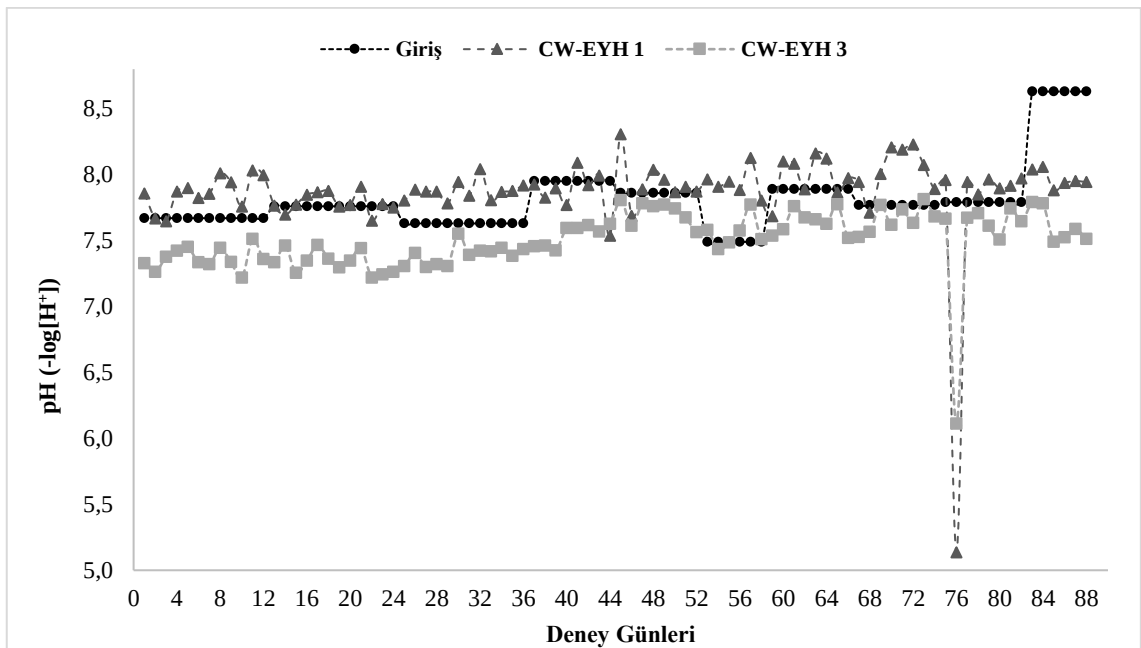
Şekil 3. 2. Yapay sulak alan ekolojik yakıt hücresi 3 modülünün çıkış suyunun araştırma periyodu içerisindeki giriş ve yapay sulak alan ekolojik yakıt hücresi 1 modülünün çıkış suyuna göre pH değişimi
