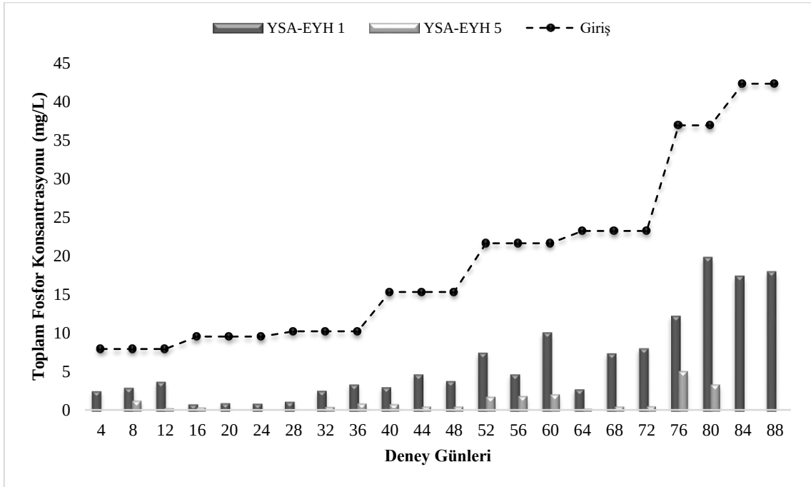
Şekil 3. 42. Yapay sulak alan ekolojik yakıt hücresi 5 modülünün çıkış suyunun araştırma periyodu içerisindeki giriş ve yapay sulak alan ekolojik yakıt hücresi 1 modülünün çıkış suyuna göre ortalama toplam fosfor konsantrasyonu (mg/L) değişimi
