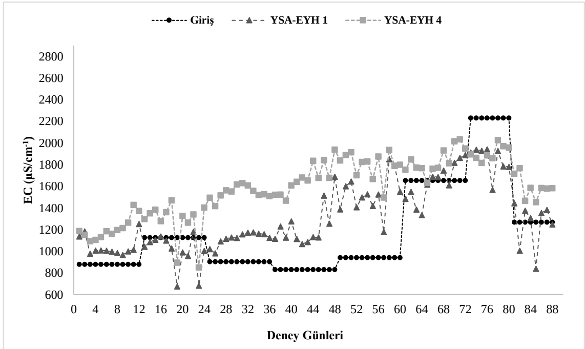
Şekil 3. 7. Yapay sulak alan ekolojik yakıt hücresi 4 modülünün çıkış suyunun araştırma periyodu içerisindeki giriş ve yapay sulak alan ekolojik yakıt hücresi 1 modülünün çıkış suyuna göre EC değişimi
