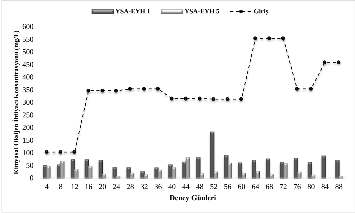
Şekil 3. 24. Yapay sulak alan ekolojik yakıt hücresi 5 modülünün çıkış suyunun araştırma periyodu içerisindeki giriş ve yapay sulak alan ekolojik yakıt hücresi 1 modülünün çıkış suyunu göre kimyasal oksijen ihtiyacı konsantrasyonu (mg/L) değişimi
