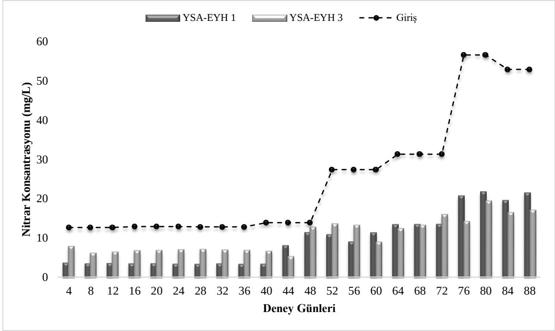
Şekil 3. 34. Yapay sulak alan ekolojik yakıt hücresi 3 modülünün çıkış suyunun araştırma periyodu içerisindeki giriş ve yapay sulak alan ekolojik yakıt hücresi 1 modülünün çıkış suyuna göre ortalama nitrat konsantrasyonu (mg/L) değişimi
