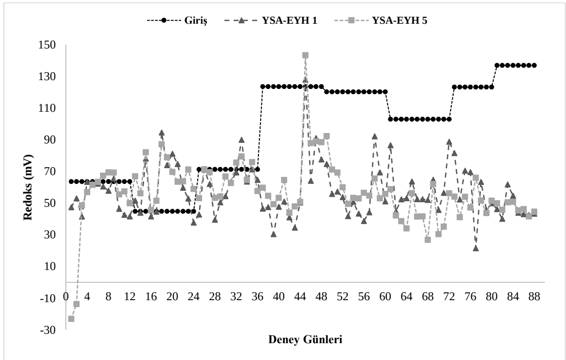
Şekil 3. 16. Yapay sulak alan ekolojik yakıt hücresi 5 modülünün çıkış suyunun araştırma periyodu içerisindeki giriş ve yapay sulak alan ekolojik yakıt hücresi 1 modülünün çıkış suyuna göre redoks (mV) değişimi
