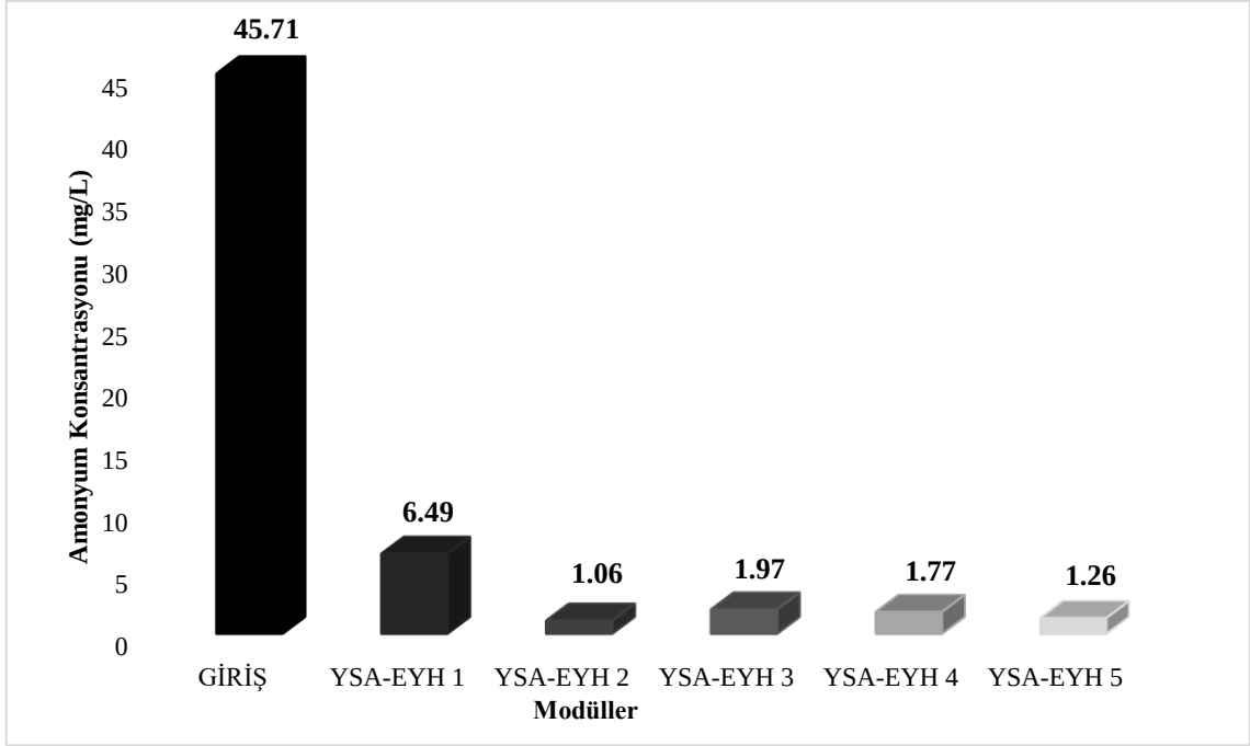
Şekil 3. 31. Yapay sulak alan ekolojik yakıt hücresi modüllerinin çıkış sularının araştırma periyodu içerisindeki ortalama kimyasal oksijen ihtiyacı konsantrasyonu (mg/L) değişimi
