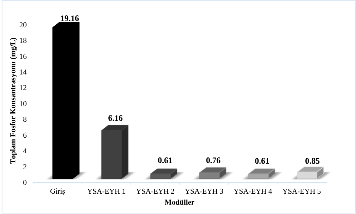
Şekil 3. 43. Yapay sulak alan ekolojik yakıt hücresi modüllerinin çıkış sularının araştırma periyodu içerisindeki ortalama toplam fosfor konsantrasyonu (mg/L) değişimi
