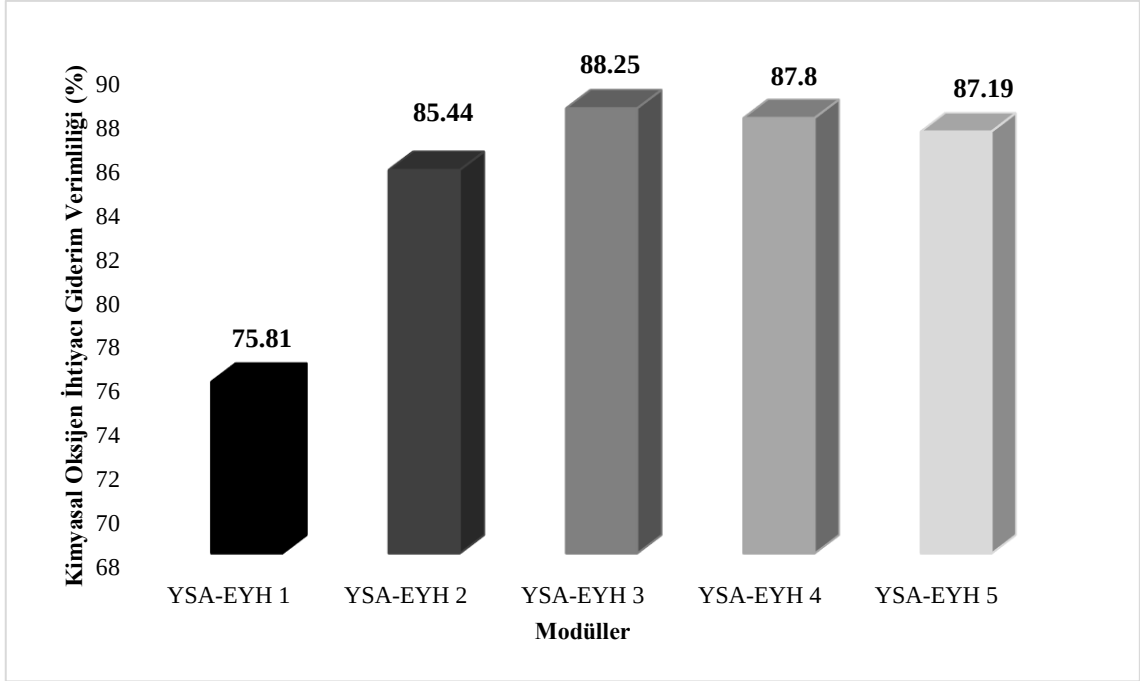
Şekil 3. 26. Yapay sulak alan ekolojik yakıt hücresi modüllerinin çıkış sularının araştırma periyodu içerisindeki ortalama kimyasal oksijen ihtiyacı giderim verimliliği (%)
