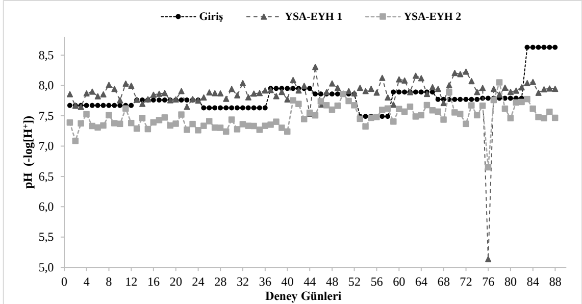
Şekil 3. 1. Yapay sulak alan ekolojik yakıt hücresi 2 modülünün çıkış suyunun araştırma periyodu içerisindeki giriş ve yapay sulak alan ekolojik yakıt hücresi 1 modülünün çıkış suyuna göre pH değişimi
