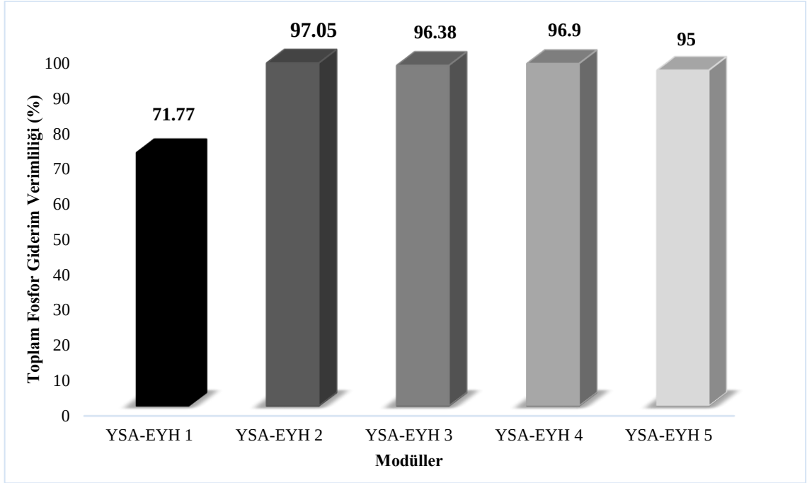
Şekil 3. 44. Yapay sulak alan ekolojik yakıt hücresi modüllerinin çıkış sularının araştırma periyodu içerisindeki ortalama toplam fosfor giderim verimliliği (%)
