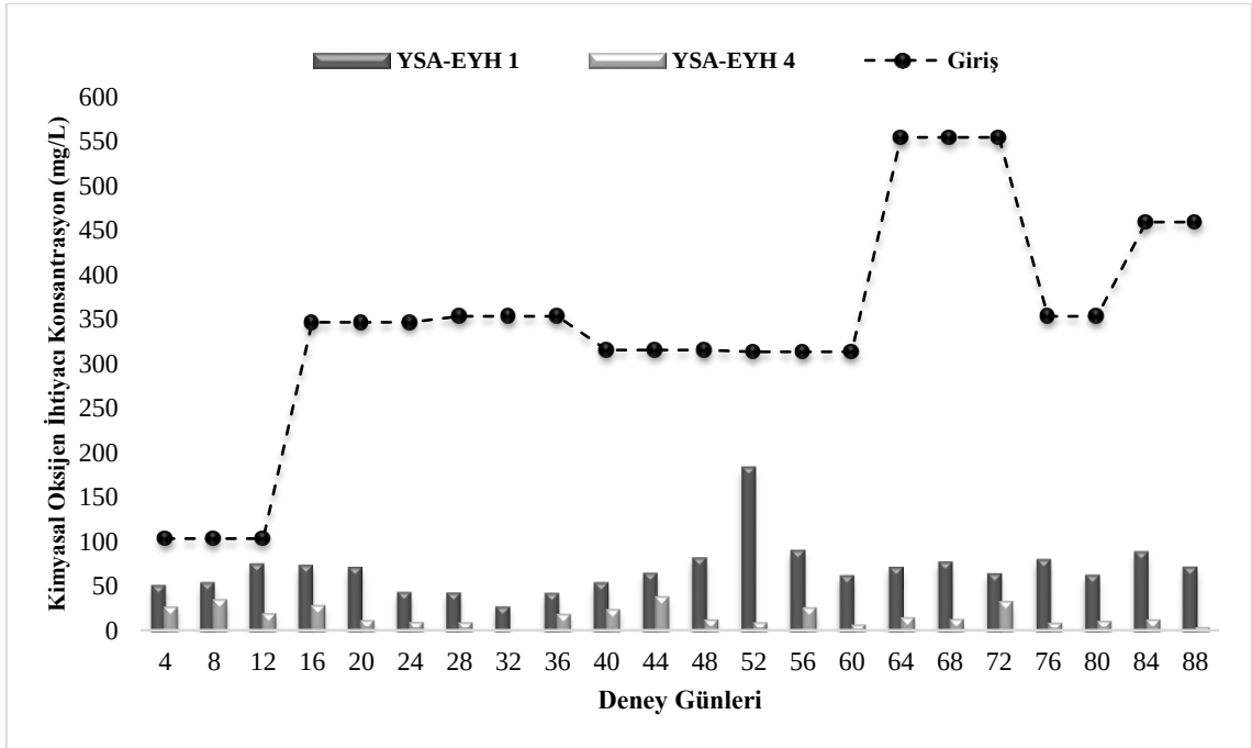
Şekil 3. 23. Yapay sulak alan ekolojik yakıt hücresi 4 modülünün çıkış suyunun araştırma periyodu içerisindeki giriş ve yapay sulak alan ekolojik yakıt hücresi 1 modülünün çıkış suyuna göre kimyasal oksijen ihtiyacı konsantrasyonu (mg/L) değişimi
