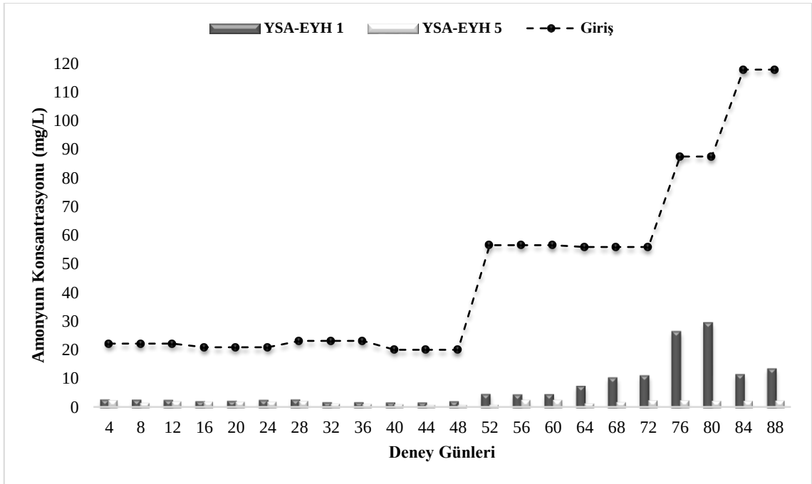
Şekil 3. 30. Yapay sulak alan ekolojik yakıt hücresi 5 modülünün çıkış suyunun araştırma periyodu içerisindeki giriş ve yapay sulak alan ekolojik yakıt hücresi 1 modülünün çıkış suyuna göre ortalama amonyum konsantrasyonu (mg/L) değişimi
