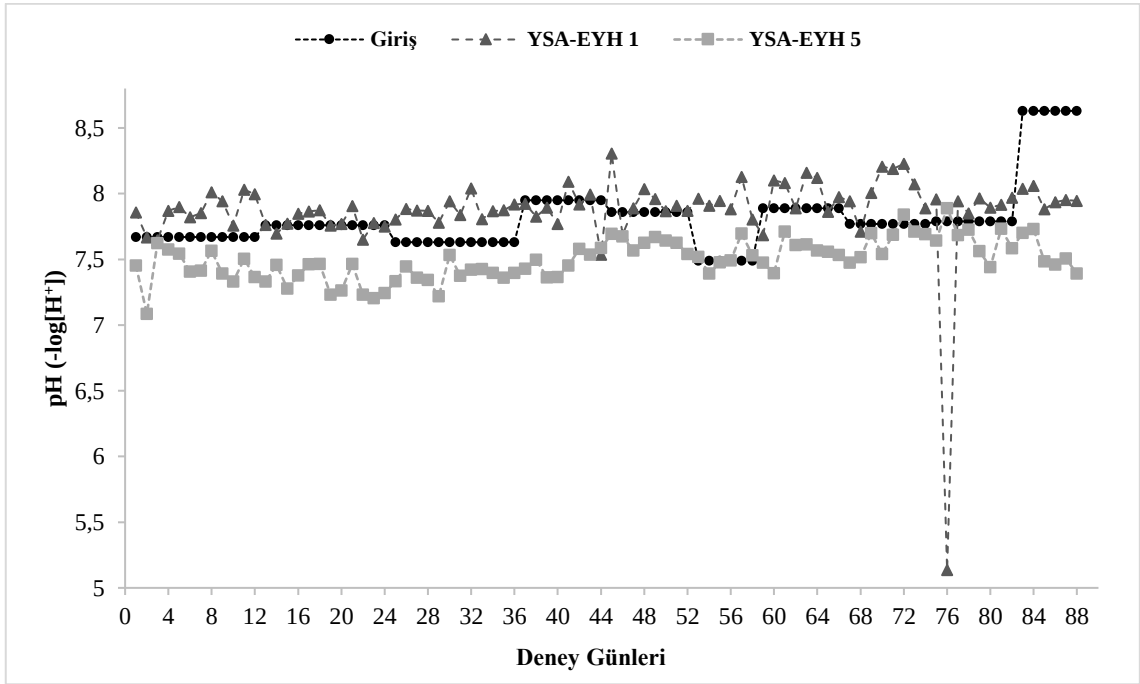
Şekil 3. 4. Yapay sulak alan ekolojik yakıt hücresi 5 modülünün çıkış suyunun araştırma periyodu içerisindeki giriş ve yapay sulak alan ekolojik yakıt hücresi 1 modülünün çıkış suyuna göre pH değişimi
