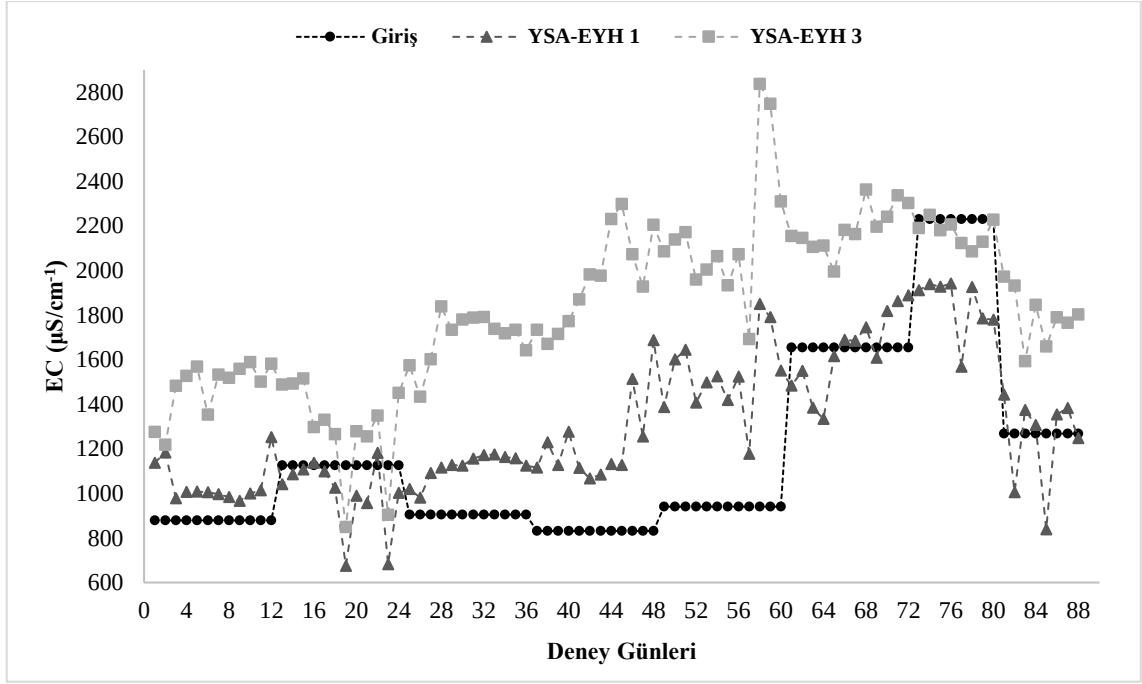
Şekil 3. 6. Yapay sulak alan ekolojik yakıt hücresi 3 modülünün çıkış suyunun araştırma periyodu içerisindeki giriş ve yapay sulak alan ekolojik yakıt hücresi 1 modülünün çıkış suyuna göre EC değişimi
