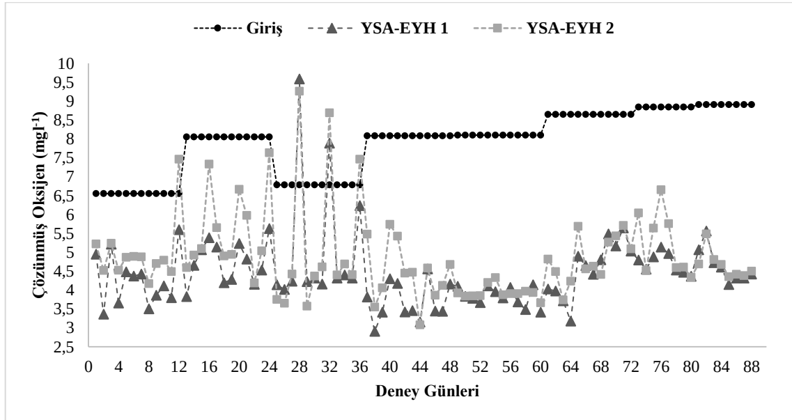
Şekil 3. 17. Yapay sulak alan ekolojik yakıt hücresi 2 modülünün çıkış suyunun araştırma periyodu içerisindeki giriş ve yapay sulak alan ekolojik yakıt hücresi 1 modülünün çıkış suyuna göre çözünmüş oksijen (mgL -1 ) değişimi
