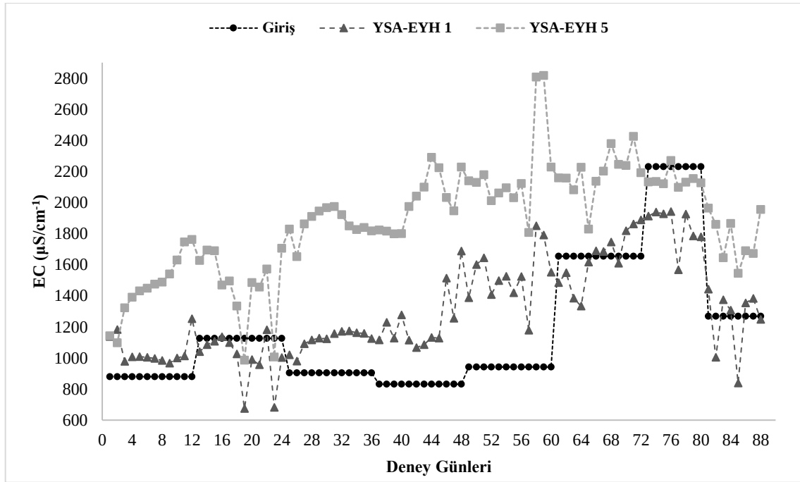
Şekil 3. 8. Yapay sulak alan ekolojik yakıt hücresi 5 modülünün çıkış suyunun araştırma periyodu içerisindeki giriş ve yapay sulak alan ekolojik yakıt hücresi 1 modülünün çıkış suyuna göre EC değişimi
