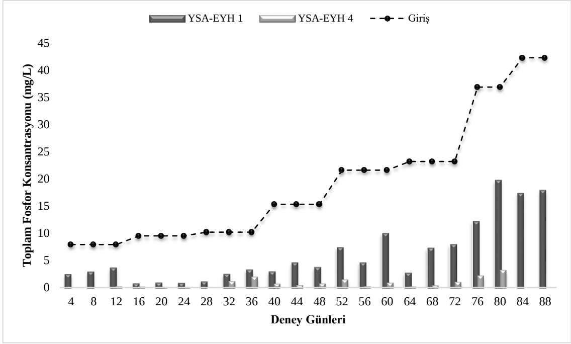
Şekil 3. 41. Yapay sulak alan ekolojik yakıt hücresi 4 modülünün çıkış suyunun araştırma periyodu içerisindeki giriş ve yapay sulak alan ekolojik yakıt hücresi 1 modülünün çıkış suyuna göre ortalama toplam fosfor konsantrasyonu (mg/L) değişimi
