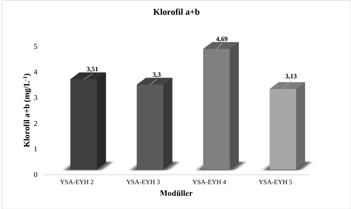
Şekil 3. 49. Yapay sulak alan ekolojik yakıt hücresi modüllerinde bulunan bitkilerin araştırma periyodu içerisindeki ortalama klorofil a+b değerleri
