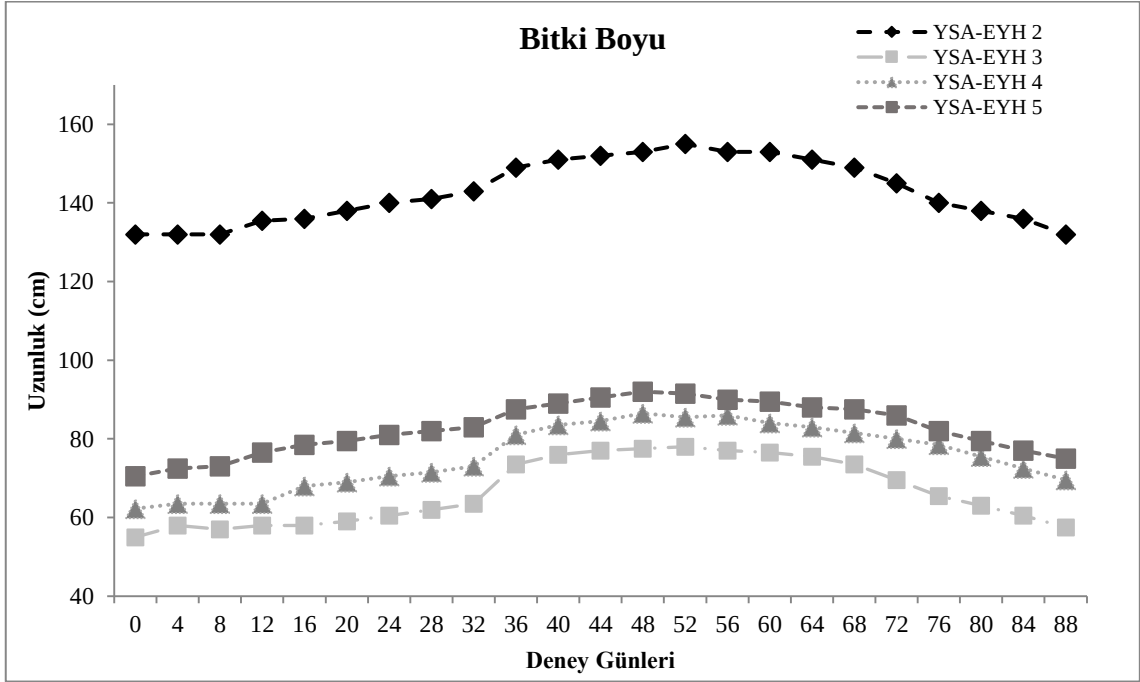
Şekil 3. 45. Yapay sulak alan ekolojik yakıt hücresi modüllerinde bulunan bitkilerin araştırma periyodu içerisindeki bitki boy uzunlukları (cm)
