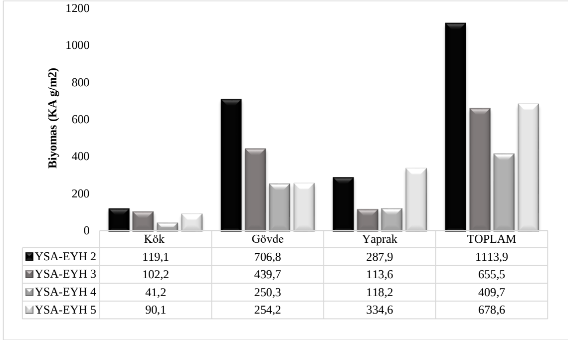
Şekil 3. 51. Yapay sulak alan ekolojik yakıt hücresi modüllerinden araştırma sonunda hasat edilen bitkilerin toprak altı, toprak üstü ve toplam bitki biyomasları
