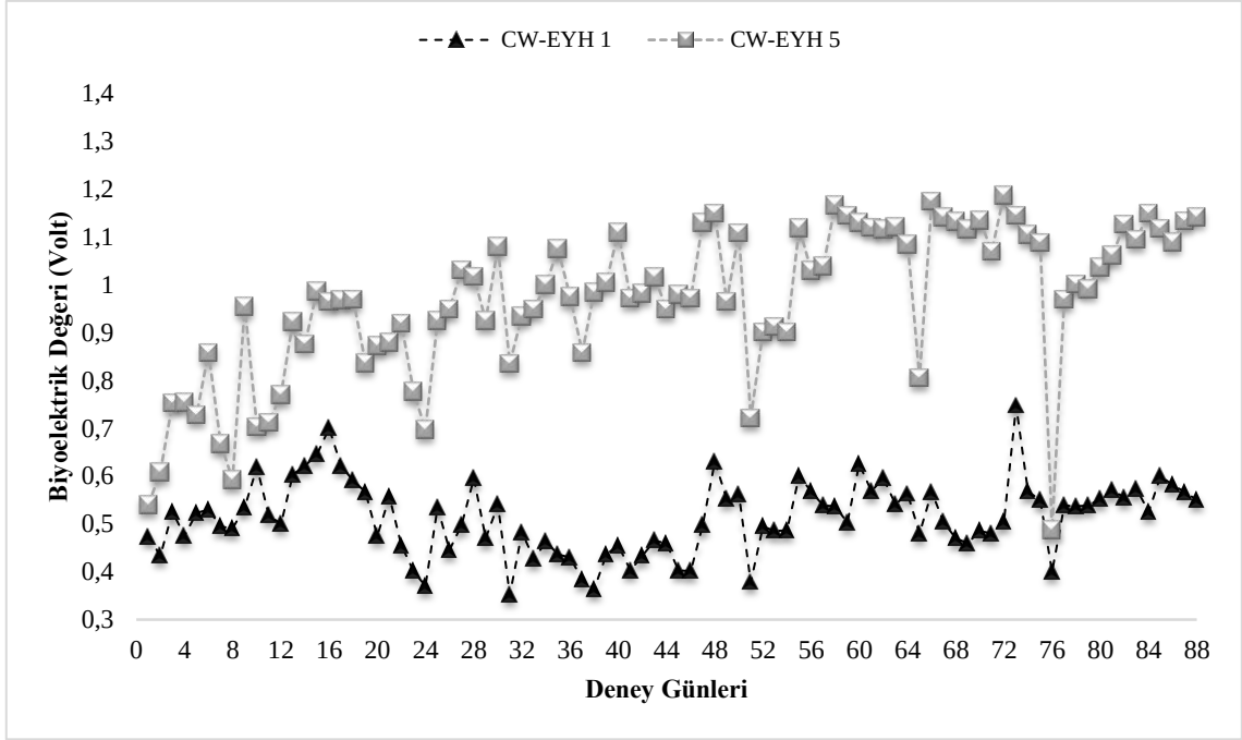
Şekil 3. 55. Araştırma periyodu içerisinde yapay sulak alan ekolojik yakıt hücresi 1 modülü ve yapay sulak alan ekolojik yakıt hücresi 5 modülünün biyoelektrik üretim değerleri(mV) değişimi
