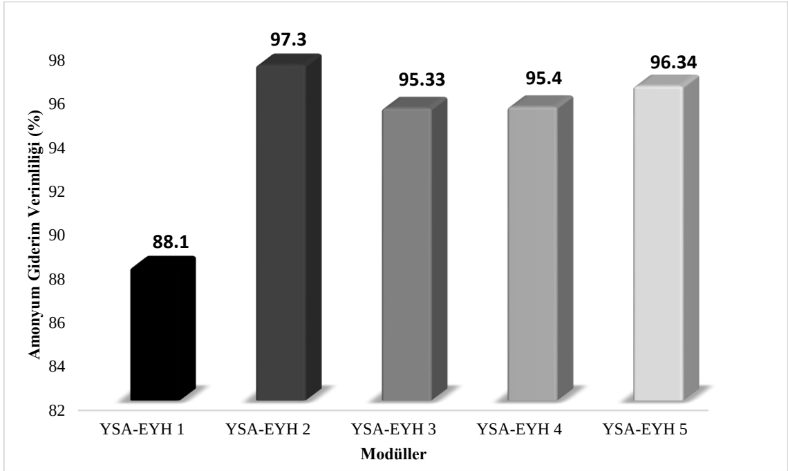
Şekil 3. 32. Yapay sulak alan ekolojik yakıt hücresi modüllerinin çıkış sularının araştırma periyodu içerisindeki ortalama amonyum giderim verimliliği (%)
