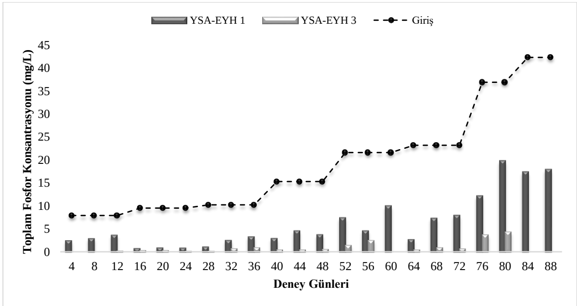
Şekil 3. 40. Yapay sulak alan ekolojik yakıt hücresi 3 modülünün çıkış suyunun araştırma periyodu içerisindeki giriş ve yapay sulak alan ekolojik yakıt hücresi 1 modülünün çıkış suyuna göre ortalama toplam fosfor konsantrasyonu (mg/L) değişimi
