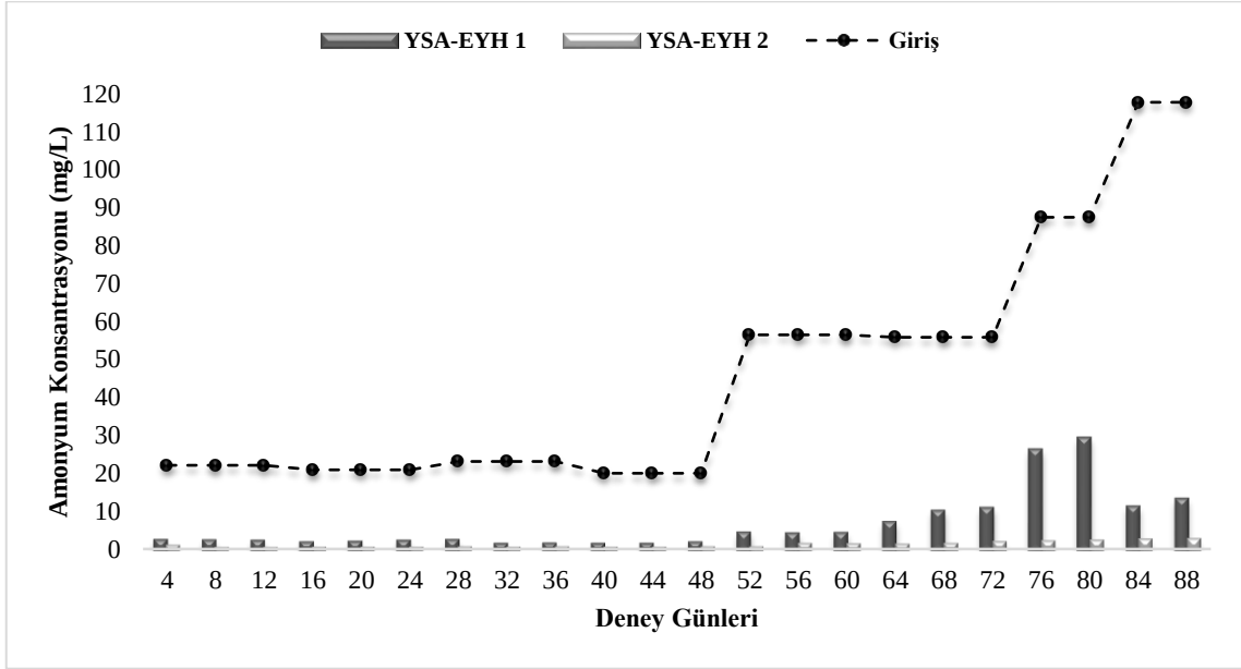
Şekil 3. 27. Yapay sulak alan ekolojik yakıt hücresi 2 modülünün çıkış suyunun araştırma periyodu içerisindeki giriş ve yapay sulak alan ekolojik yakıt hücresi 1 modülünün çıkış suyuna göre ortalama amonyum konsantrasyonu (mg/L) değişimi
