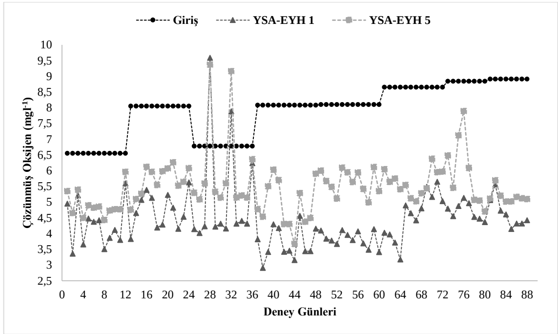
Şekil 3. 20. Yapay sulak alan ekolojik yakıt hücresi 5 modülünün çıkış suyunun araştırma periyodu içerisindeki giriş ve yapay sulak alan ekolojik yakıt hücresi 1 modülünün çıkış suyuna göre çözünmüş oksijen ( \text{mgL}^{-1} ) değişimi
