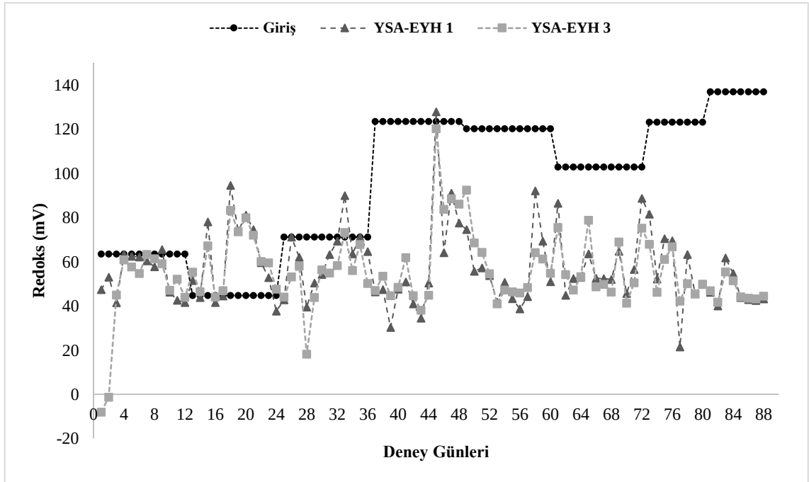
Şekil 3. 14. Yapay sulak alan ekolojik yakıt hücresi 3 modülünün çıkış suyunun araştırma periyodu içerisindeki giriş ve yapay sulak alan ekolojik yakıt hücresi 1 modülünün çıkış suyuna göre redoks (mV) değişimi
