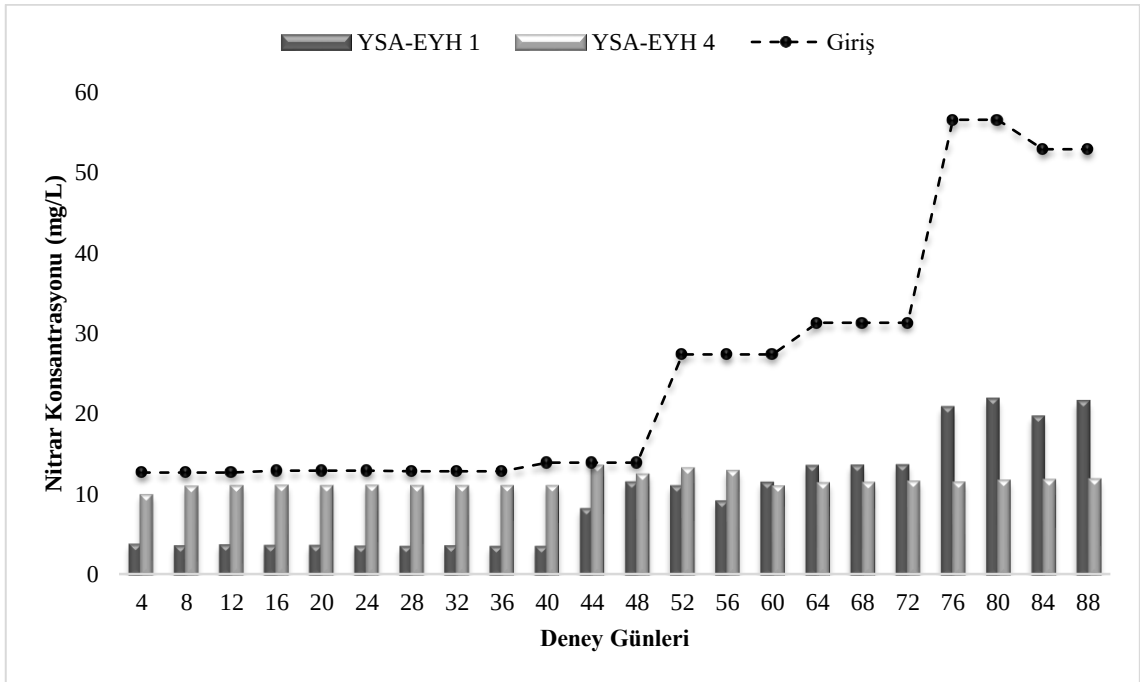
Şekil 3. 35. Yapay sulak alan ekolojik yakıt hücresi 4 modülünün çıkış suyunun araştırma periyodu içerisindeki giriş ve yapay sulak alan ekolojik yakıt hücresi 1 modülünün çıkış suyuna göre ortalama nitrat konsantrasyonu (mg/L) değişimi
