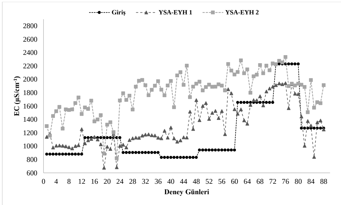
Şekil 3. 5. Yapay sulak alan ekolojik yakıt hücresi 2 modülünün çıkış suyunun araştırma periyodu içerisindeki giriş ve yapay sulak alan ekolojik yakıt hücresi 1 modülünün çıkış suyuna göre EC değişimi
