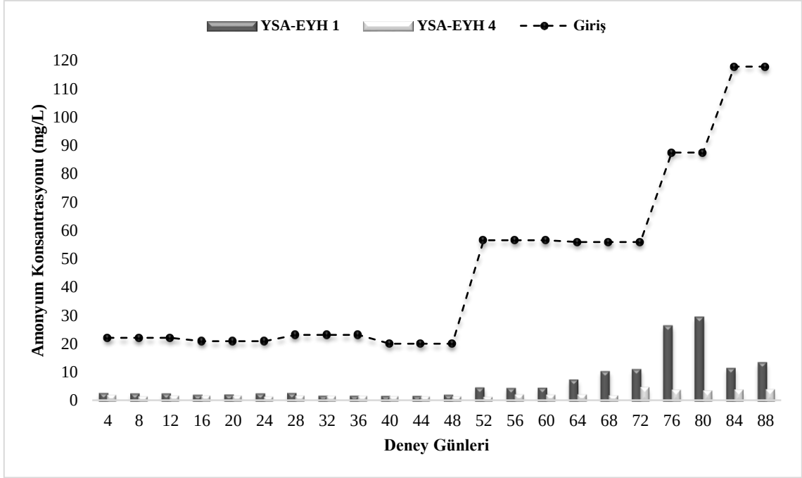
Şekil 3. 29. Yapay sulak alan ekolojik yakıt hücresi 4 modülünün çıkış suyunun araştırma periyodu içerisindeki giriş ve yapay sulak alan ekolojik yakıt hücresi 1 modülünün çıkış suyuna göre ortalama amonyum konsantrasyonu (mg/L) değişimi
