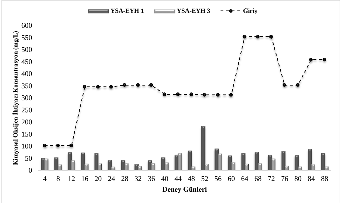
Şekil 3. 22. Yapay sulak alan ekolojik yakıt hücresi 3 modülünün çıkış suyunun araştırma periyodu içerisindeki giriş ve yapay sulak alan ekolojik yakıt hücresi 1 modülünün çıkış suyuna göre kimyasal oksijen ihtiyacı konsantrasyonu (mg/L) değişimi
