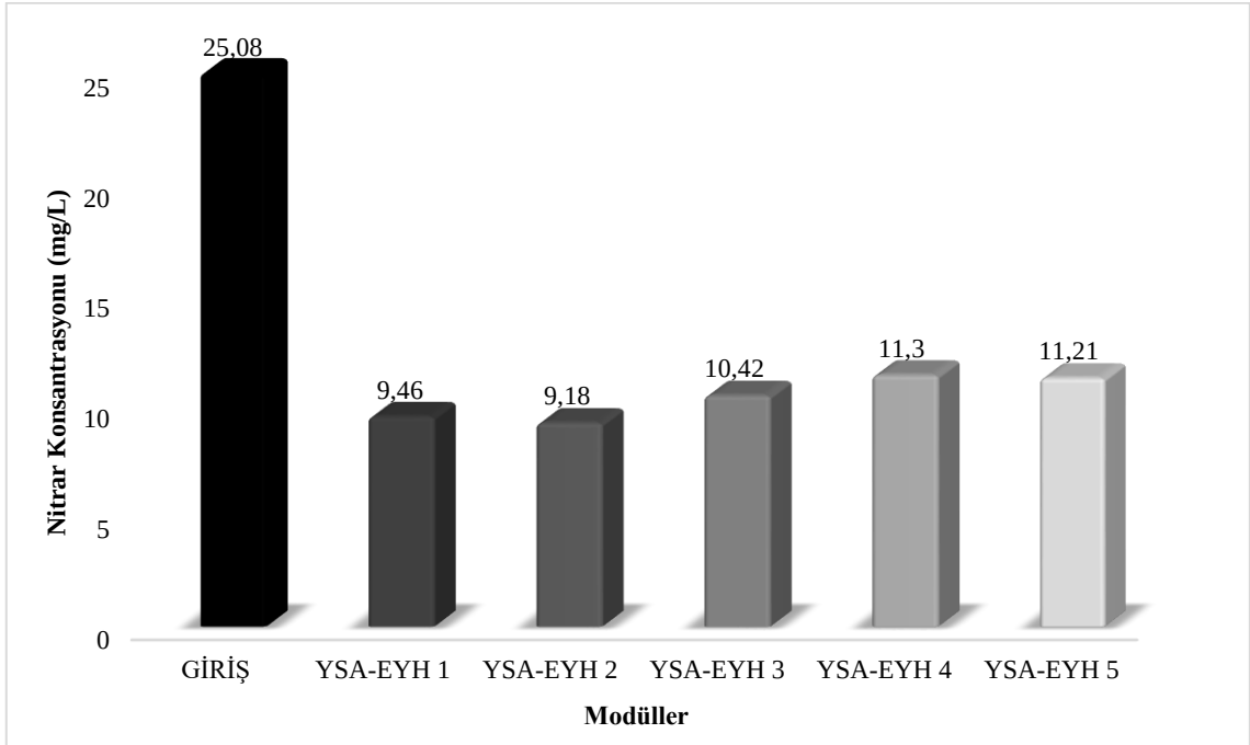
Şekil 3. 37. Yapay sulak alan ekolojik yakıt hücresi modüllerinin çıkış sularının araştırma periyodu içerisindeki ortalama nitrat konsantrasyonu (mg/L) değişimi
