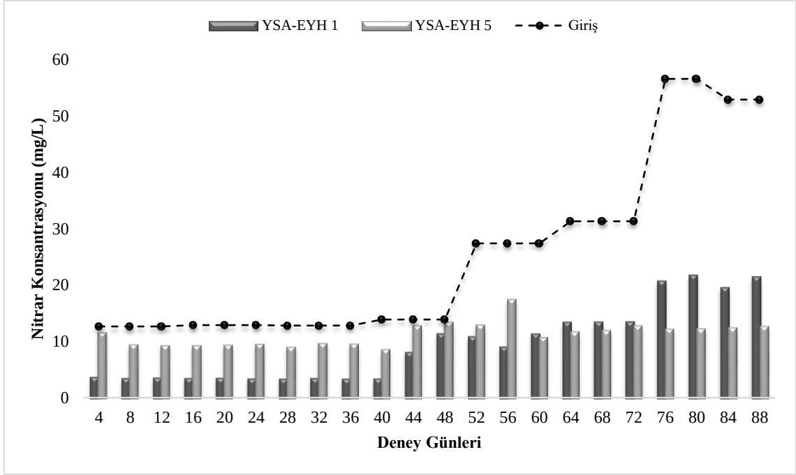
Şekil 3. 36. Yapay sulak alan ekolojik yakıt hücresi 5 modülünün çıkış suyunun araştırma periyodu içerisindeki giriş ve yapay sulak alan ekolojik yakıt hücresi 1 modülünün çıkış suyuna göre ortalama nitrat konsantrasyonu (mg/L) değişimi
