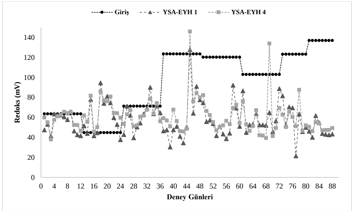
Şekil 3. 15. Yapay sulak alan ekolojik yakıt hücresi 4 modülünün çıkış suyunun araştırma periyodu içerisindeki giriş ve yapay sulak alan ekolojik yakıt hücresi 1 modülünün çıkış suyuna göre redoks (mV) değişimi
