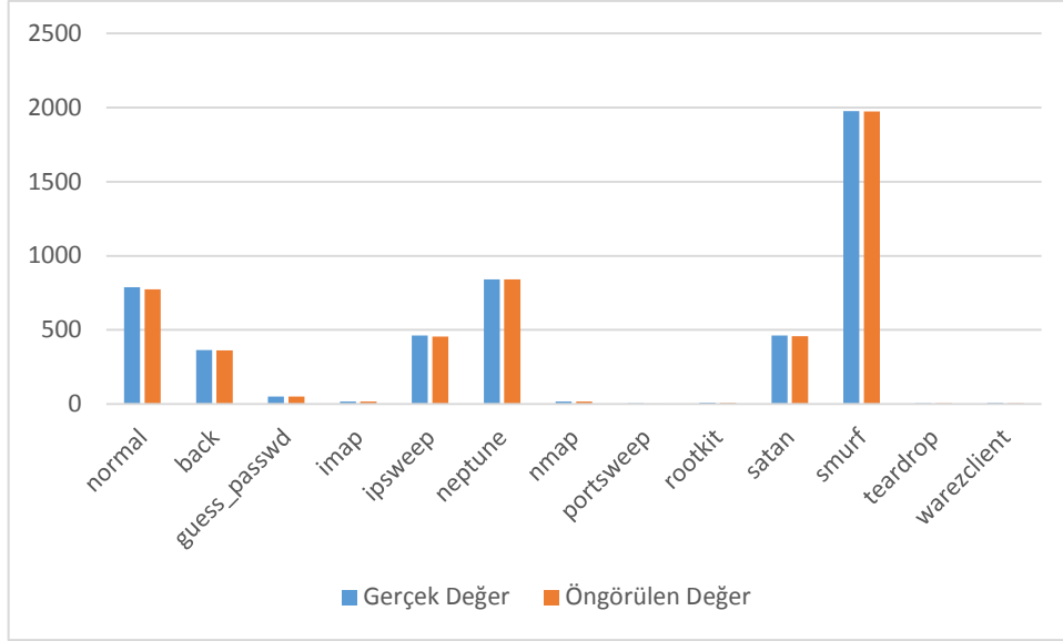
Şekil 7.9. J48 algoritması için service , src_bytes , dst_bytes , wrong_fragment , count , srv_count , diff_srv_rate , dst_host_diff_srv_rate , dst_host_same_src_port_rate , dst_host_srv_diff_host_rate özelliklerine göre gerçek değer ve öngörülen değerlerin dağılım grafiği
