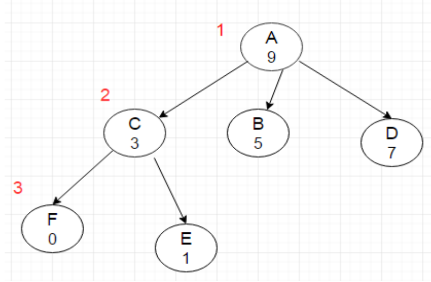
Şekil 7.7. Açgözlü En İyi İlk Arama Algoritması
