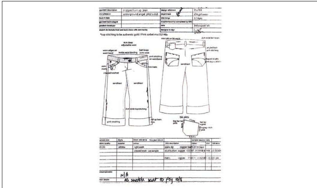
Şekil 5.4. Örnek teknik föy-4 [8]
