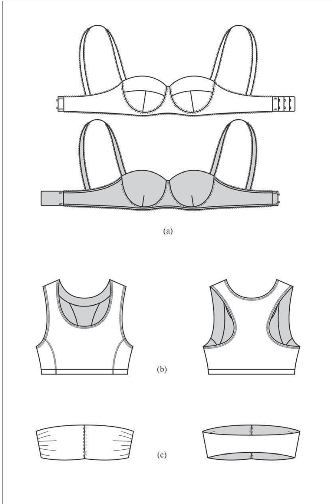
Şekil 4.45. (a) Sutyen, (b) Sporcu sutyeni, (c) Askısız sutyen teknik çizimi; ön-arka görüşleri
