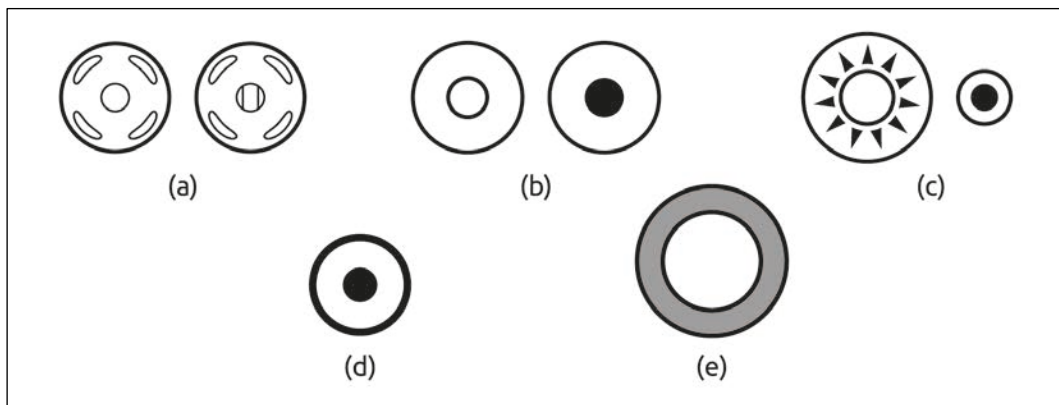
Şekil 5.16. Çıt çıt, mıknatıs çıt çıt, rivet, perçin ve kuşgözü teknik çizimleri
