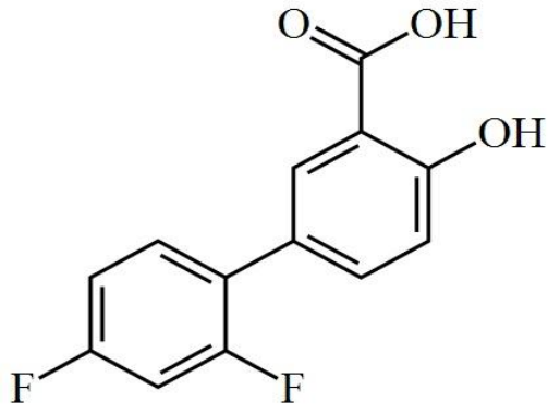
Şekil 14. DİF'in moleköl yapısı
