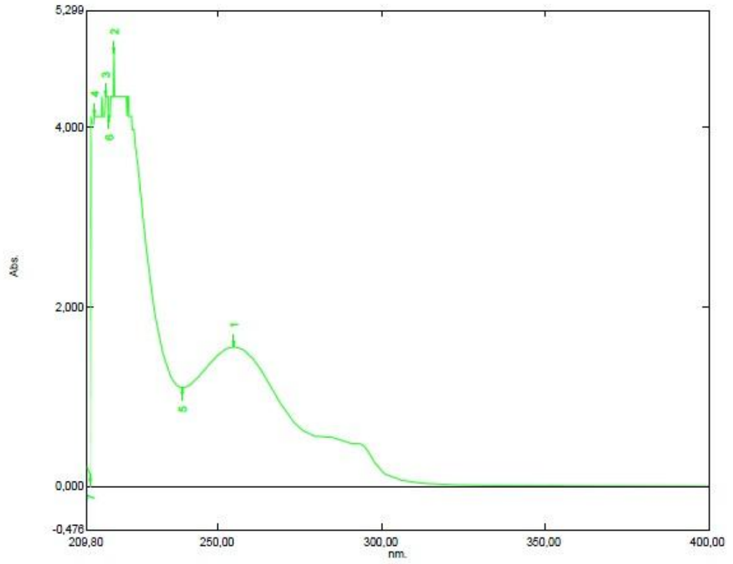
Şekil 4. 1.01 \times 10^{-4} M ARP spektrumu (1: 254.60 nm, 2: 218.00 nm)
