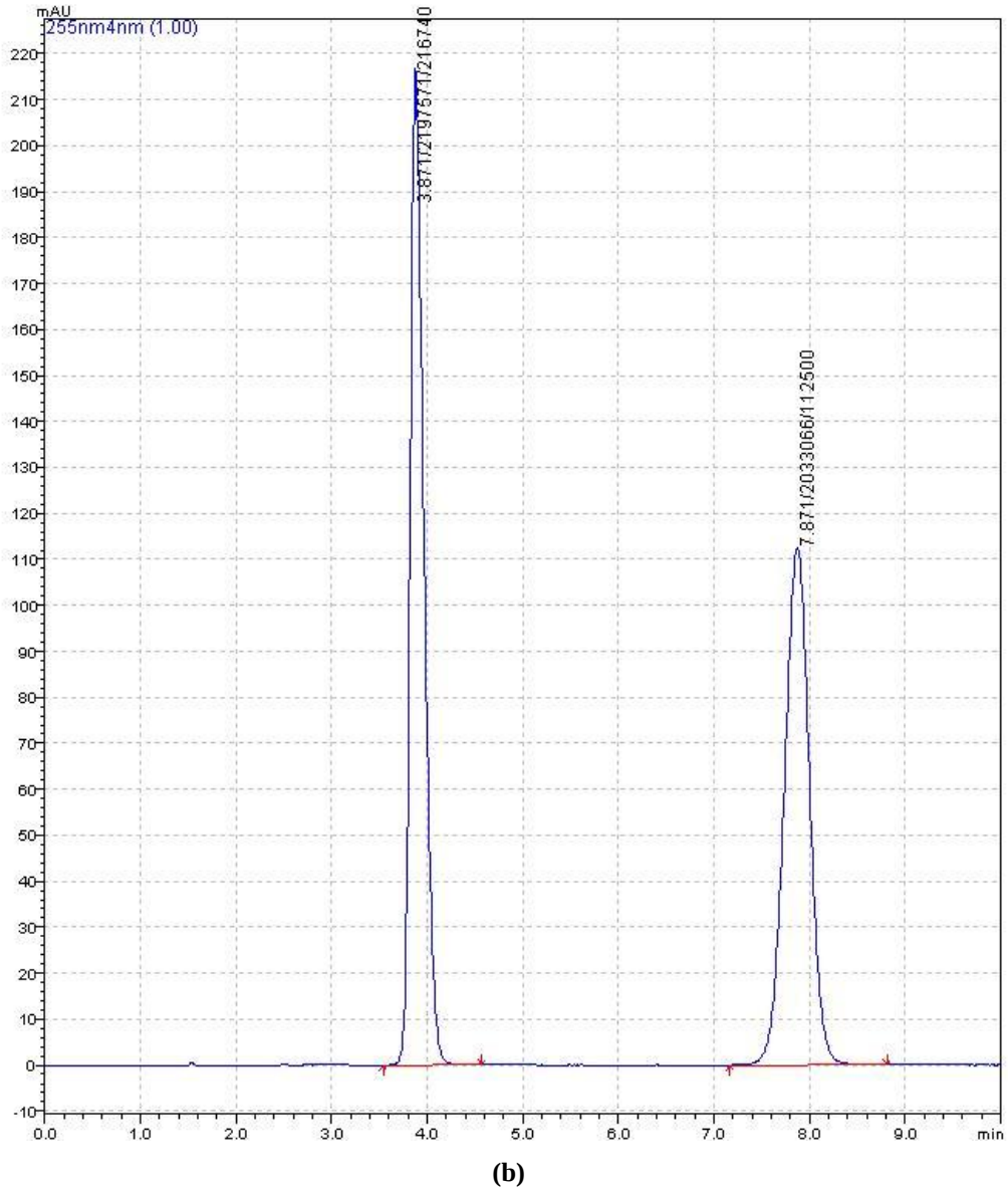
Şekil 15. ARP ve DİF'in 10^{-3} M derişimine sahip çözeltilerinin MeOH:Tampon (65:35, h/h) mobil fazında, 1 mL/dk (a) ve 0.8 mL/dk (b) akış hızlarında eş zamanlı analizi sonucu 255 nm dalga boyunda elde edilen kromatogramları
