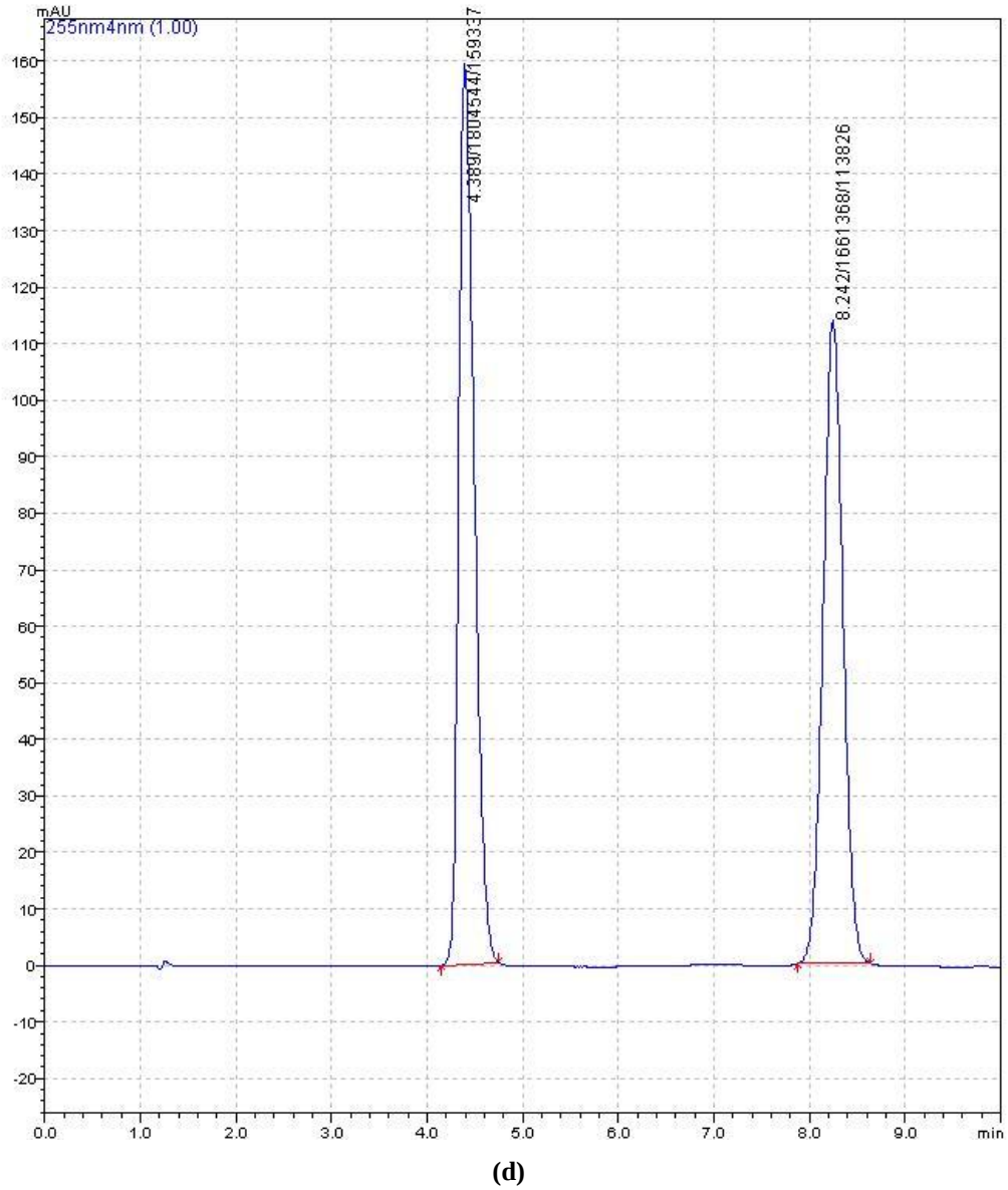
Şekil 16. ARP ve DİF'in 10^{-3} M derişimine sahip çözeltilerinin, sırasıyla deęişken bileşimli hareketli faz yöntemiyle, 1 mL/dk akış hızında eş zamanlı analizleri sonucu 255 nm dalga boyunda elde edilen kromatogramları
