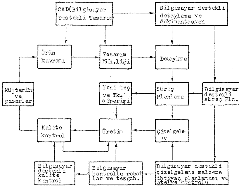
Şekil 2.6 CAM 'ın Ürün çevrimi (GROOWER, ZIMMERS, 1984).
