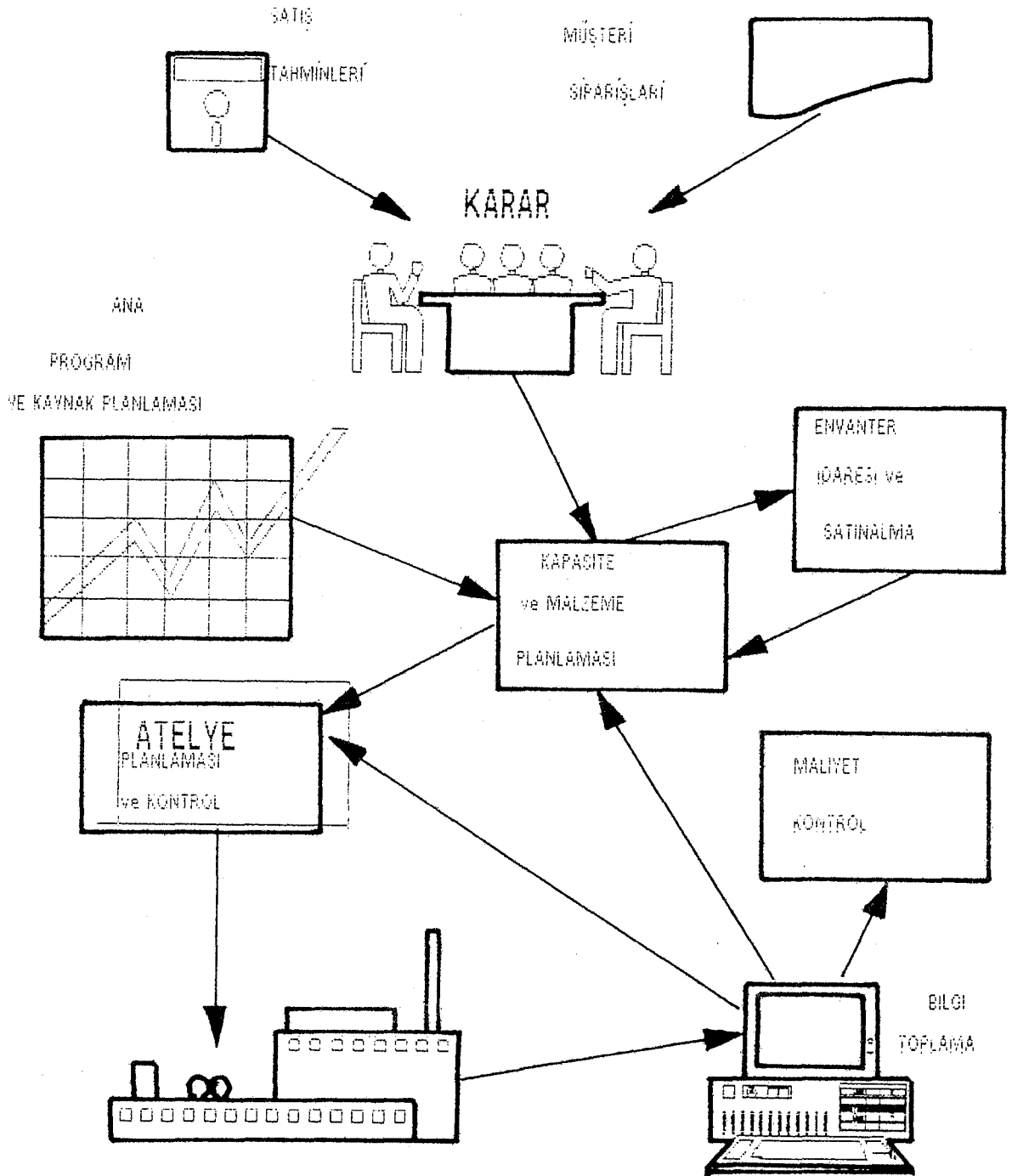
Şekil 2.16 Production IV imalat planlama sistemi genel yapısı ve elemanları
