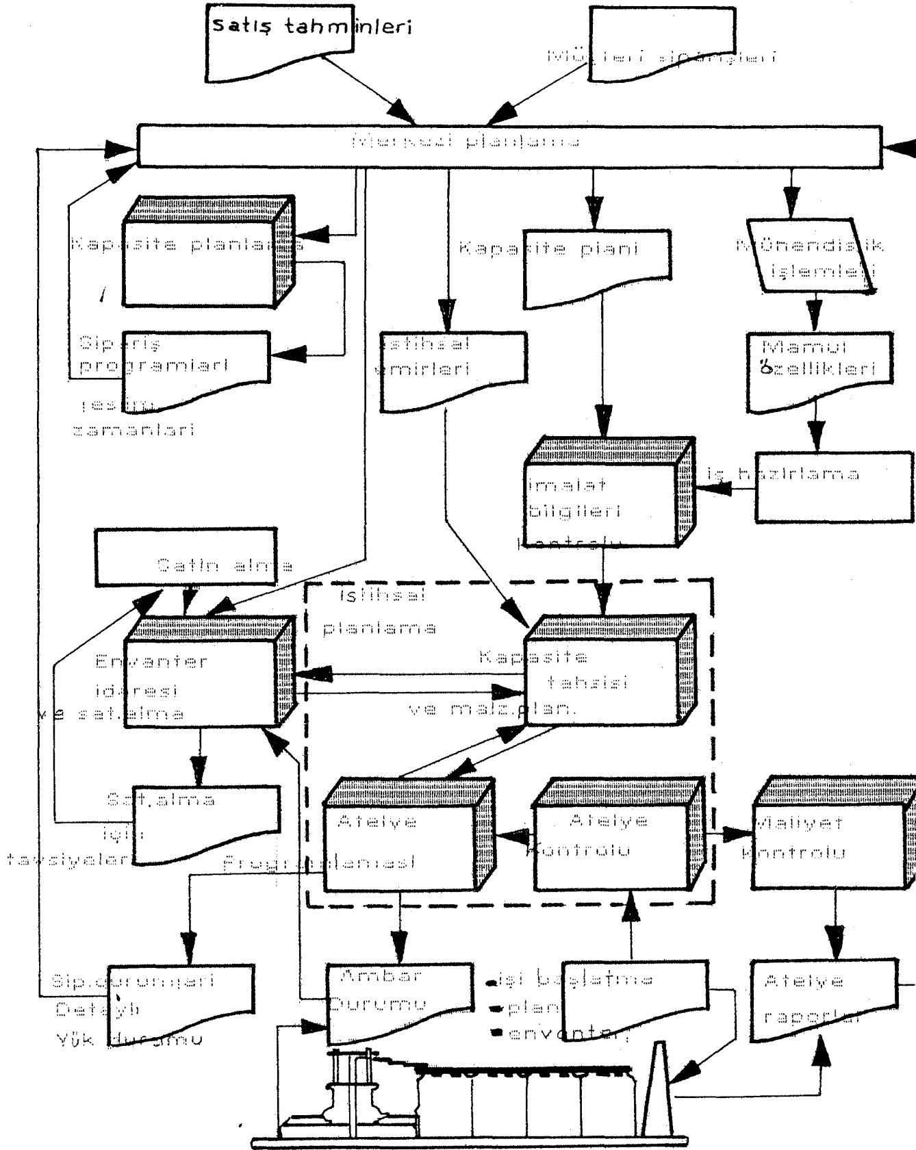
Şekil 2.17 Production IV imalat planlama sistemi ana şeması
