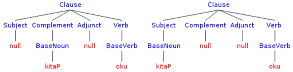
Şekil 7.2. İlişkisel Modeller İçin Örnek Sözdizimsel Çözümlemeler
