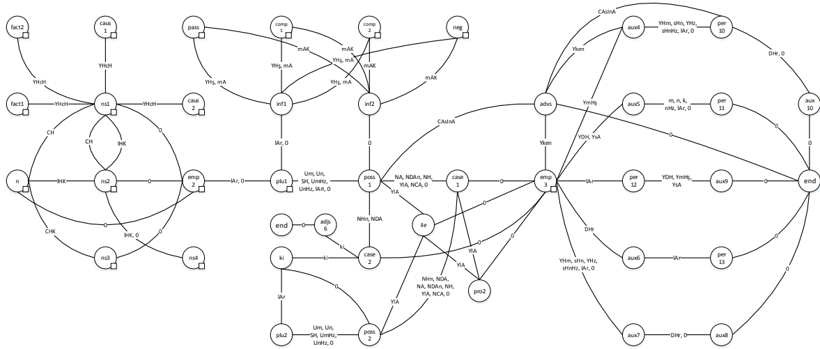
Şekil 4.5. Türkçe Ad Morfotaktikleri
