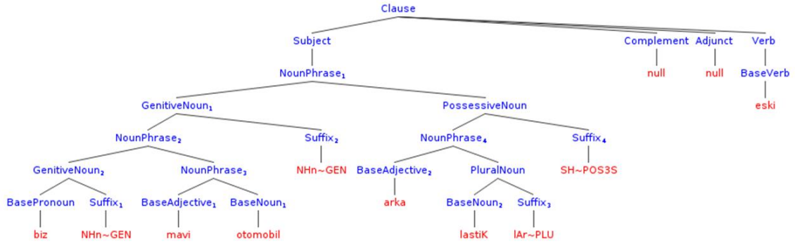
Şekil 7.1. OBBD ve Öbek Olasılık Modeli İçin Bir Örnek Sözdizimsel Çözümleme
