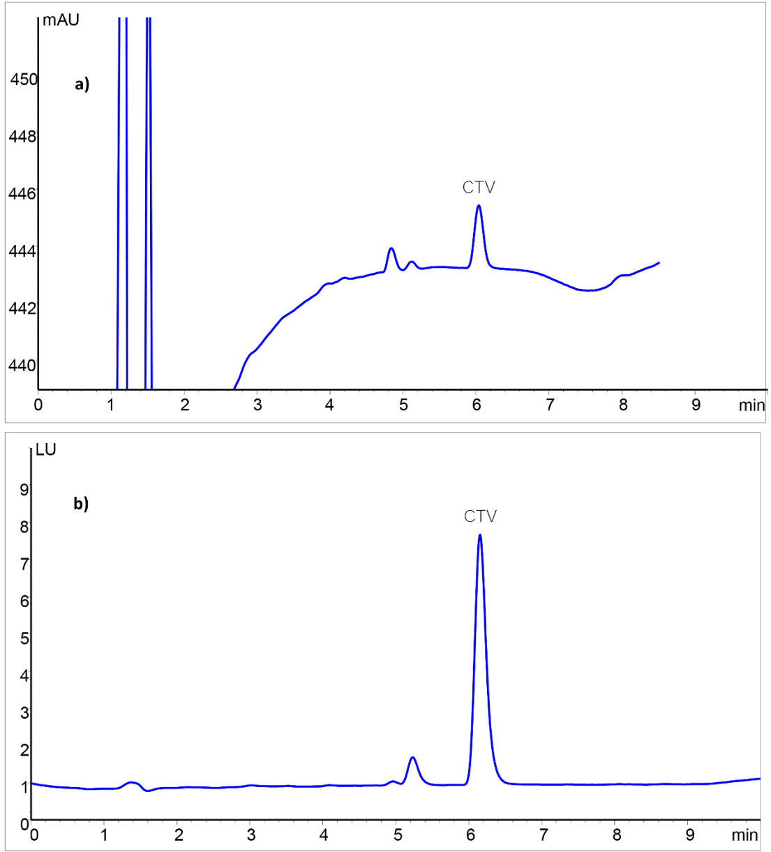
Şekil 4.10. 100 ng/ml CTV standardının optimum UHPLC-FLD koşullarında a) 220 nm'de UV dedektör ile, b) \lambda_{uy}:220 nm, \lambda_{yay}:340 nm dalga boyu değerlerinde floresans dedektör ile elde edilen kromatogramları
