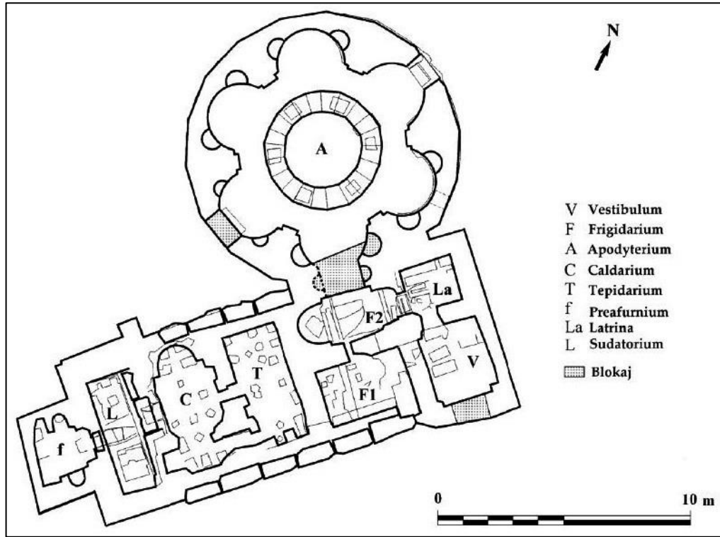
Görsel 4. Hamam Yapısının Genel Planı
