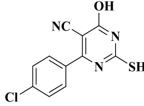
Şekil 5.15. 4-Hidroksi-2-merkaptto -6-(4-klorofenil)pirimidin-5-karbonitril yapısı
