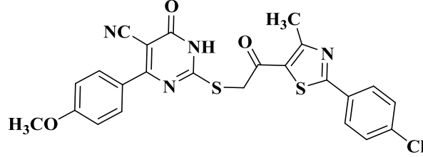
Şekil 5.41. Bileşik 19'un kimyasal yapısı
