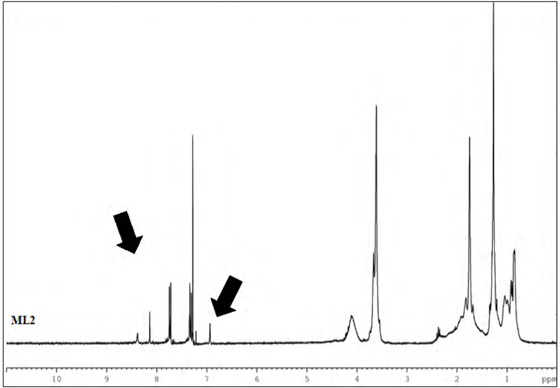
Şekil 5.15. Eudragit® RS 100 ile hazırlanan nanopartiküllerin ve saf maddelerin 1 H-NMR analiz spektrumları
