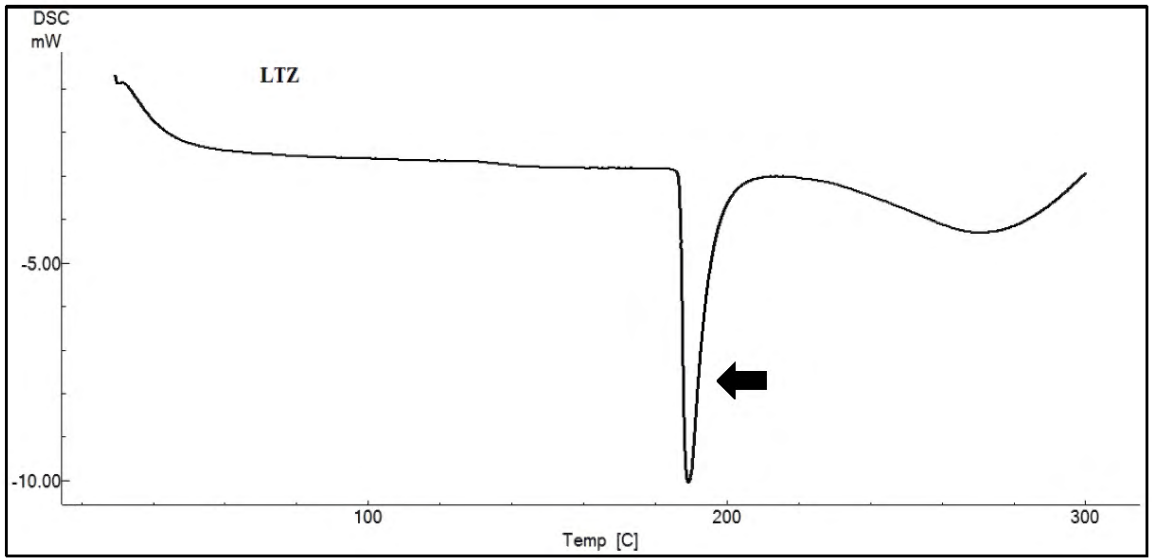
Şekil 5.17. (Devam) Kollidon® SR ile hazırlanan formülasyonların ve kullanılan saf maddelerin DSC analizlerine ait termogramlar
