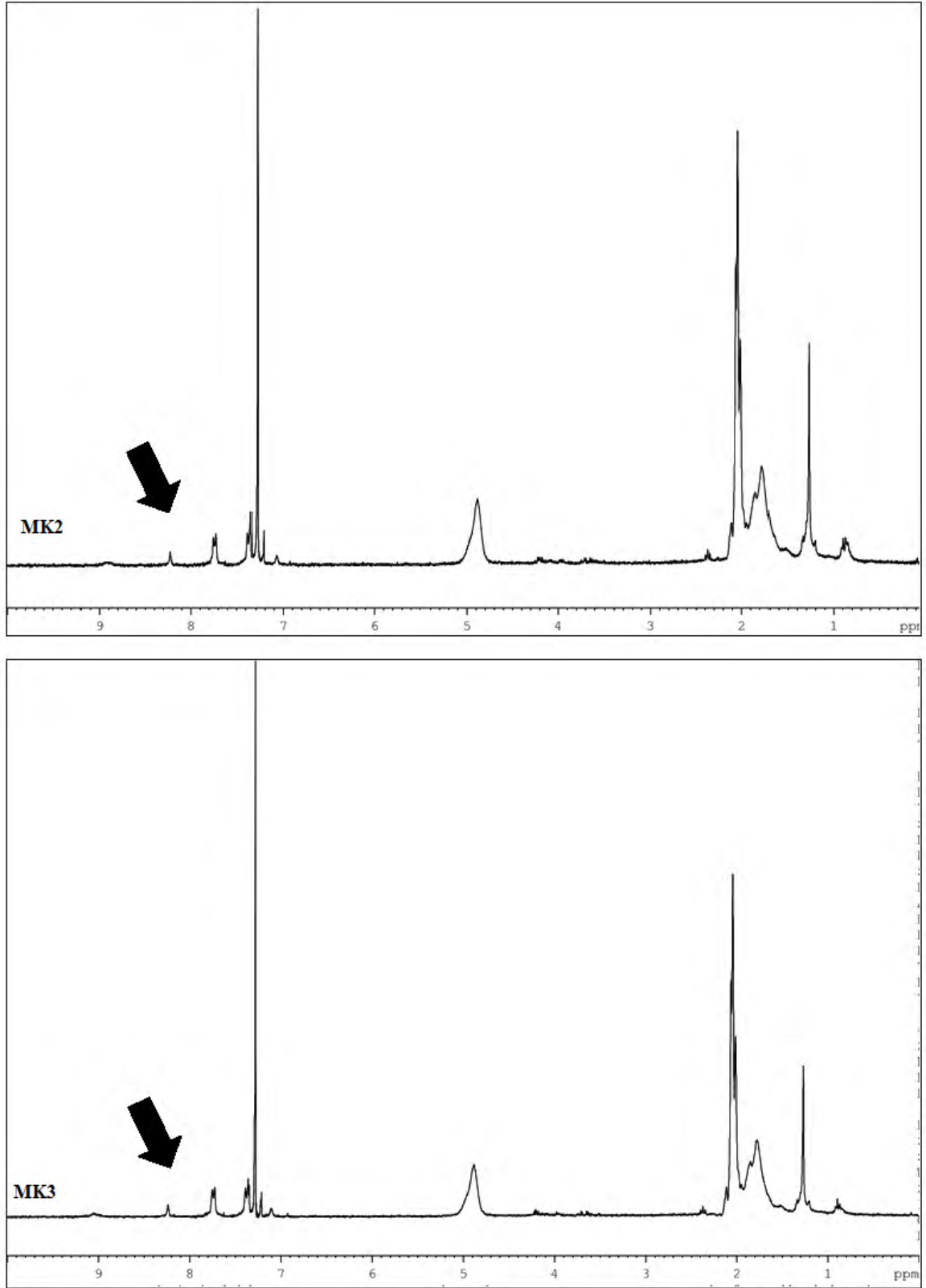
Şekil 5.19. (Devam) Kollidon® SR ile hazırlanan nanopartiküllerin ve saf maddelerin ^1\text{H} -NMR analiz spektrumları
