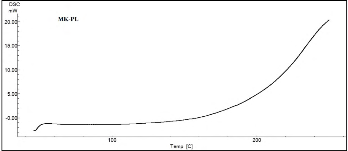
Şekil 5.17. (Devam) Kollidon® SR ile hazırlanan formülasyonların ve kullanılan saf maddelerin DSC analizlerine ait termogramlar
