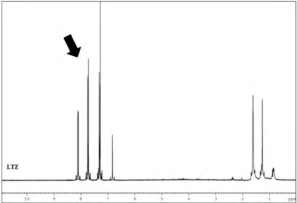
Şekil 5.19. (Devam) Kollidon® SR ile hazırlanan nanopartiküllerin ve saf maddelerin 1 H-NMR analiz spektrumları
