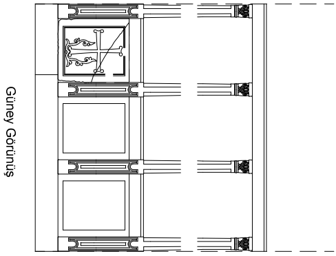
Çizim 152-Orta Bizans Dönemi Templon Restitüsü II
