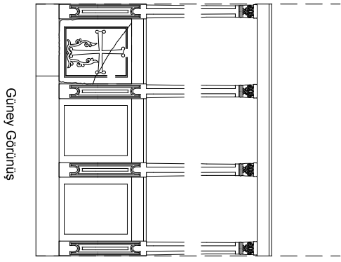
Çizim 149-Orta Bizans Dönemi Templon Restitüsyonu I
