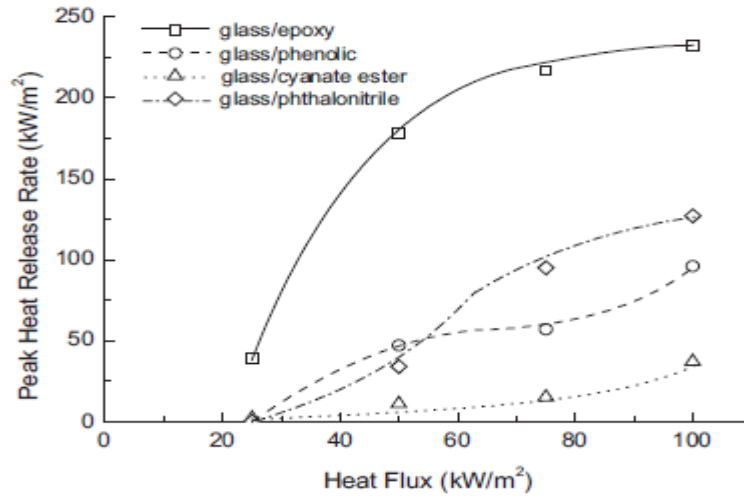
Şekil 6.6. Çeşitli cam/termoset polimer lamineler için pik HRR'de ısı akısının etkisi
