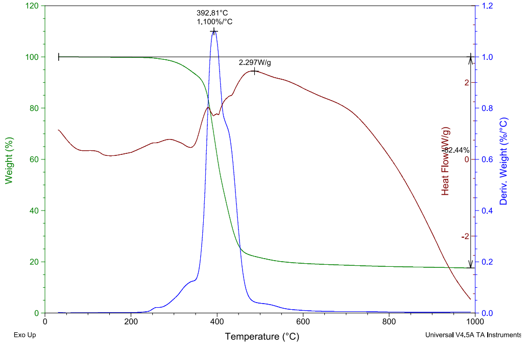
Şekil 10.17. %20ATH (E7), katkılanırılmış epoksi reçineye ait özet TGA sonucu
