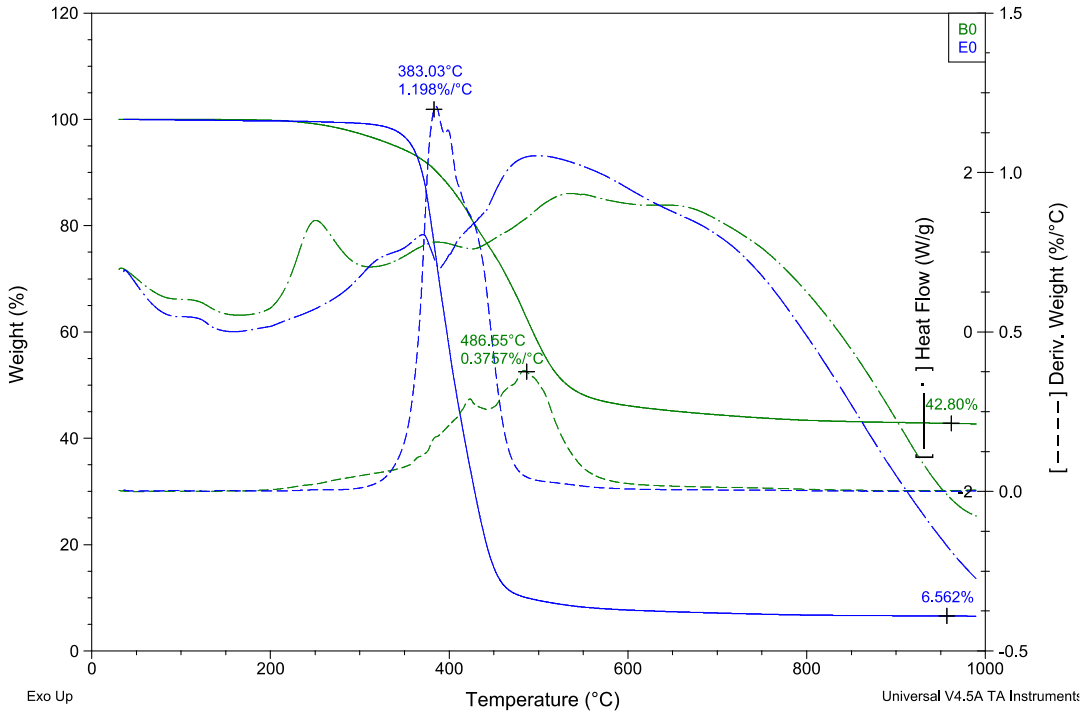
Şekil 10.3. Epoksi (E0) ve benzoksazin (B0) laminelerin karşılaştırmalı TGA sonuçları
