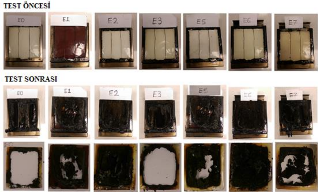
Şekil 10.32. Duman yoğunluğu testine tabi tutulmuş numunelerin görselleri
