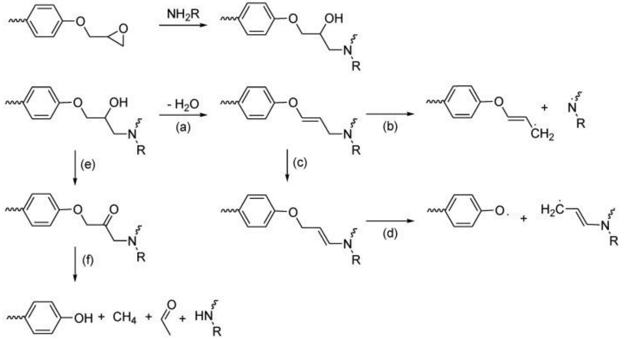
Şekil 5.10. Epoksi reçinelerin termal dekompozisasyon şeması[1]
