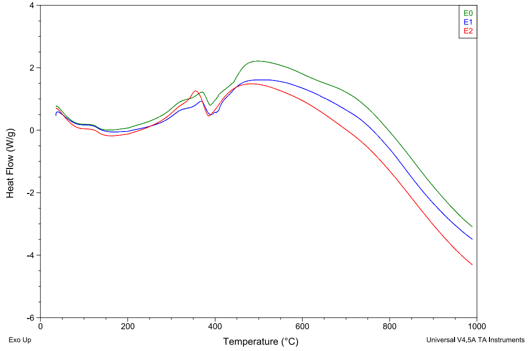
Şekil 10.8. %2 RP(E1) ve %2 APP(E2) kimyasallarından oluşan fosfor tabanlı güç tutuşur katkıları kullanarak üretilen epoksi laminelerin ısı salınımı sonuçları
