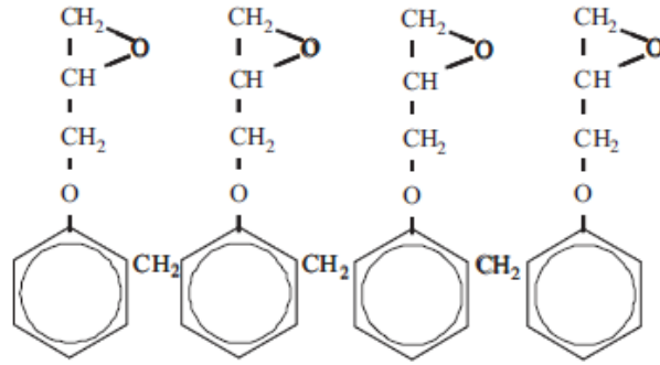
Şekil 5.9. Epoksi novolak reçinenin temsili yapısı
