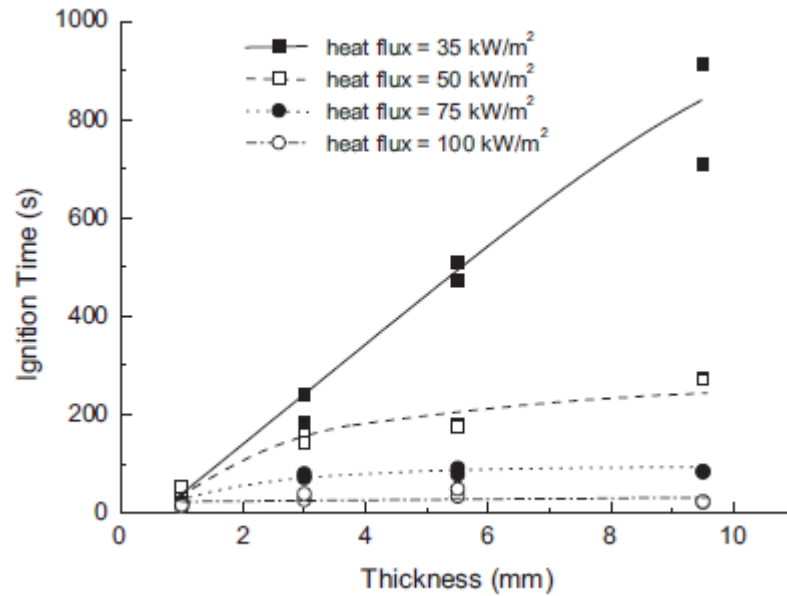
Şekil 6.4. Cam/fenolik plakaların tutuşma süresinde kalınlığın etkisi
