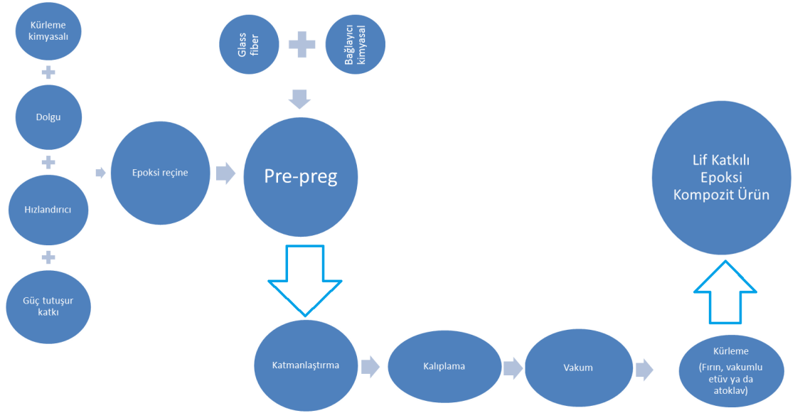
Şekil 5.1: Elyaf takviyeli kompozitlerin üretim şeması [1]
