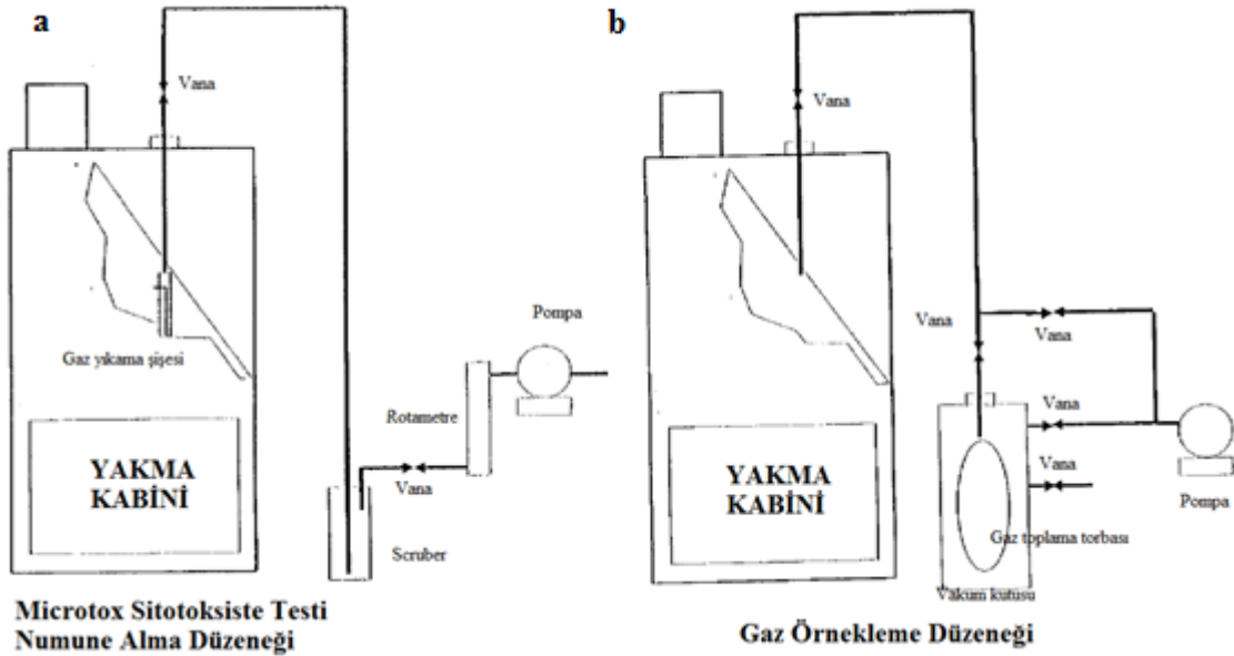
Şekil 9.2. Gaz numunelerinin alınmasında kullanılan test düzenekleri a: toksisite ölçümü, b: gaz analizleri
