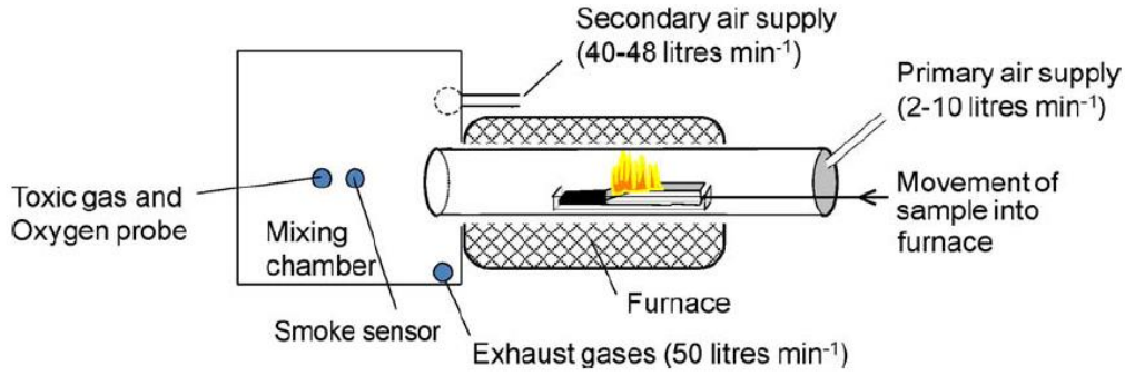
Şekil 8.3. Stec and Hull Toksik Kabini [70]
