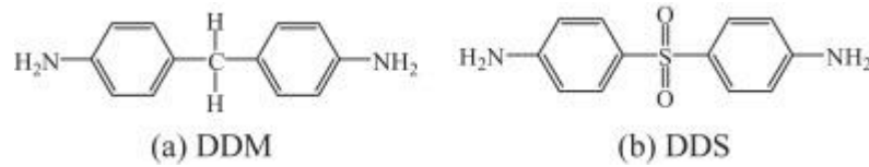
Şekil 5.20. 4,4’-diaminodifenil metan (DDM) ve 4,4’-diaminodifenil sülfonun (DDS) kimyasal yapıları[46]
