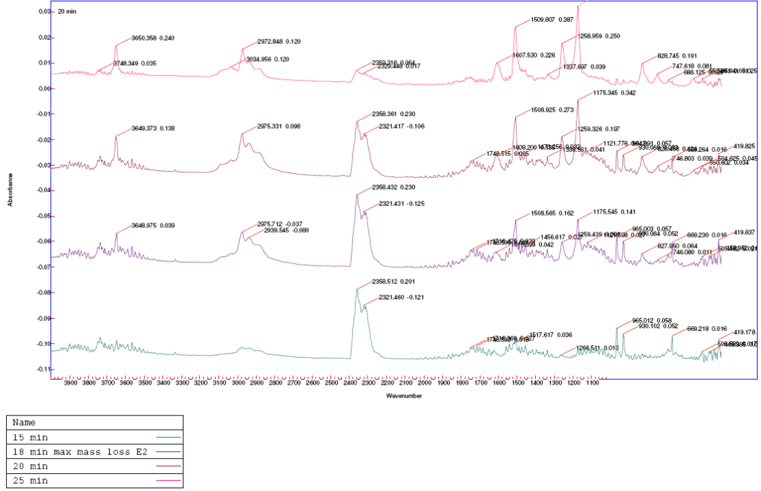
Şekil 10.24. E2 numunesi maksimum kütle kaybı noktalarında ekstrakte edilmiş FTIR specturmları
