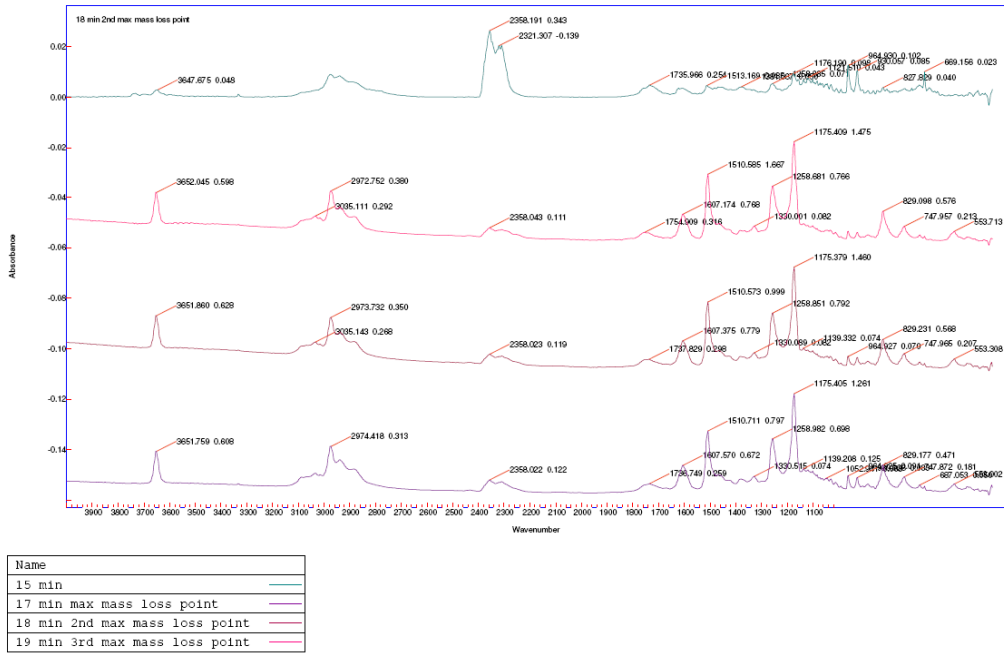
Şekil 10.23. E1 numunesi maksimum kütle kayıp noktalarında ekstrakte edilmiş FTIR spectrurları
