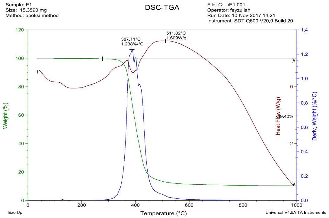
Şekil 10.4. %2 RP(E1) katkılandırılmış epoksi reçineye ait özet TGA sonucu
