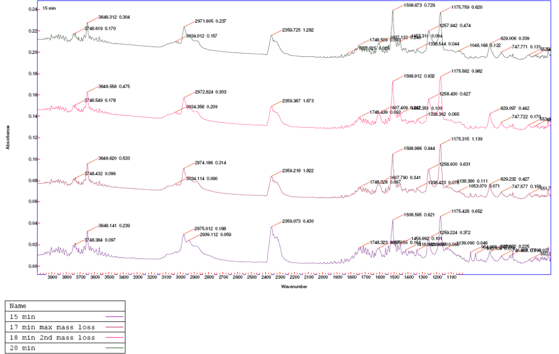
Şekil 10.25. E3 numunesi maksimum kütle kaybı noktalarında ekstrakte edilmiş FTIR specturmları
