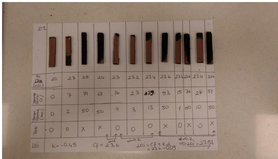
Şekil 10.29. E1 kırmızı fosfor katkılı numunesinin görsel LOİ sonuçları
