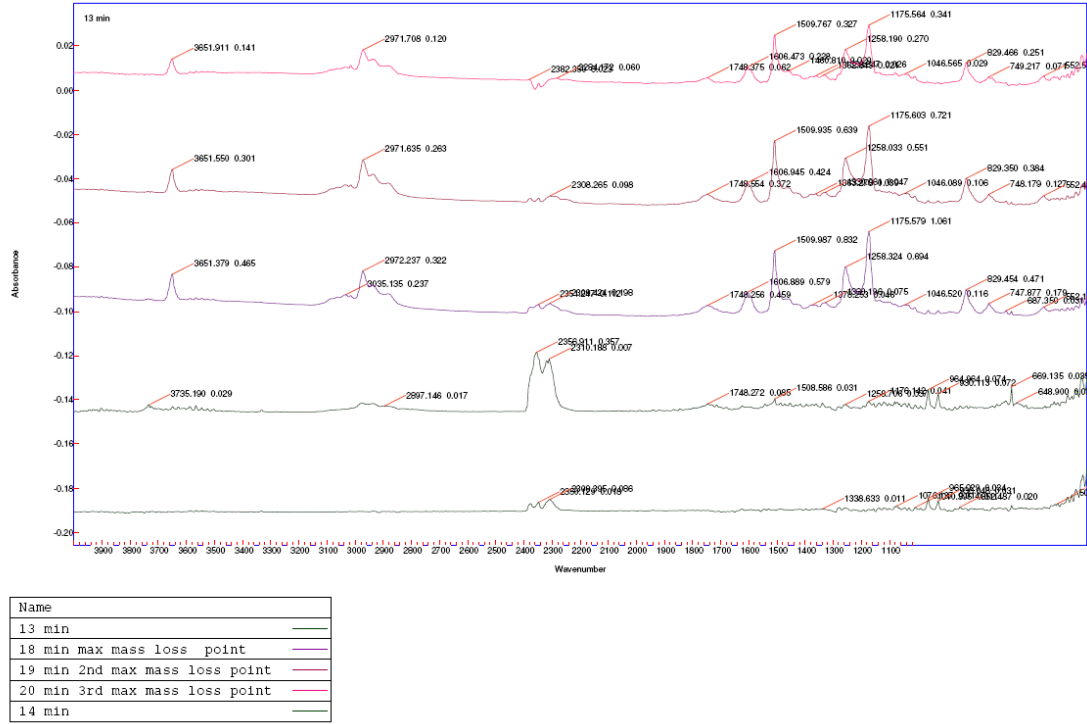
Şekil 10.26. E5 numunesi maksimum kütle kaybı noktalarında ekstrakte edilmiş FTIR specturmları
