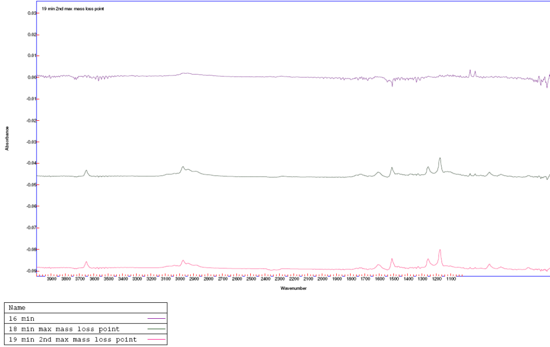
Şekil 10.28. E7 numunesi maksimum kütle kaybı noktalarında ekstrakte edilmiş FTIR spektrumları
