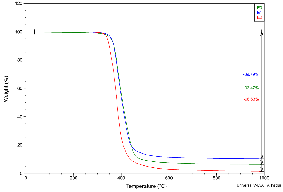
Şekil 10.6. %2 RP(E1) ve %2 APP(E2) kimyasallarından oluşan fosfor tabanlı güç tutuşur katkıları kullanılarak üretilen epoksi laminelerin kütle kaybı sonuçları
