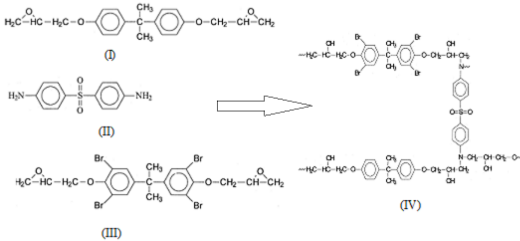
Şekil 8.1. Bisfenol A (DGBBA) / tetrabromobisfenol A (DGE BTBA) diglisidileterlerinden ve 4,4'-diaminodifenilsülfol (DDS) kütleme kimyasalı ile hazırlanan BER oluşum mekanizması [68]
