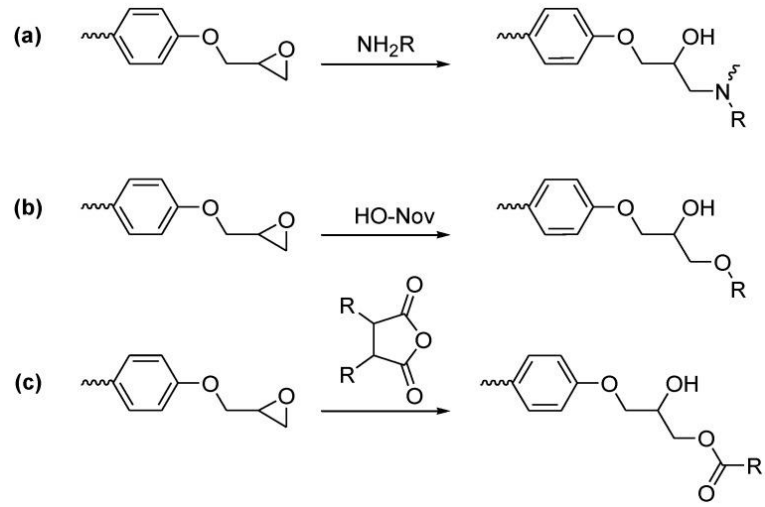
Şekil 5.12. Epoksi reçine sertleştiricileri (a) amin, (b) fenol-novolak veya (c) anhidrid kullanılarak oluşturulan bağlar [1]
