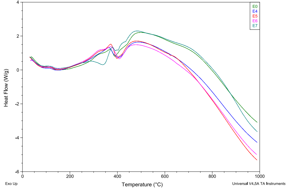
Şekil 10.20. İkinci grup tabanlı güç tutuşur karkılar ile sinerjistik olarak kullanılan ATH, SbO 3 ve ZnB katkıları kullanılarak üretilen epoksilaminelerin diferansiyel ısı salınımı sonuçları
