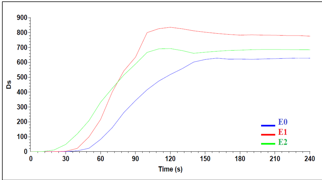
Şekil 10.30. Fosfor tabanlı katkı malzemelerinin duman yoğunluğu değerlerine olan etkisi
