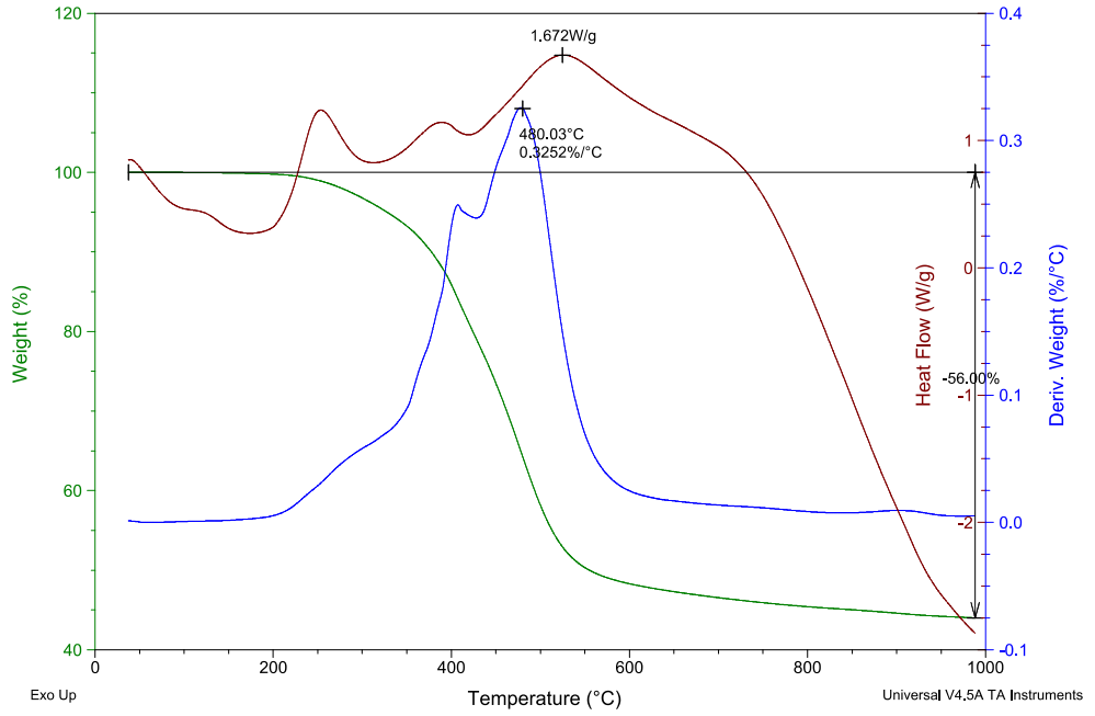
Şekil 10.10. %2 APP (B2) katkılandırılmış benzoksazin reçineye ait özet TGA sonucu
