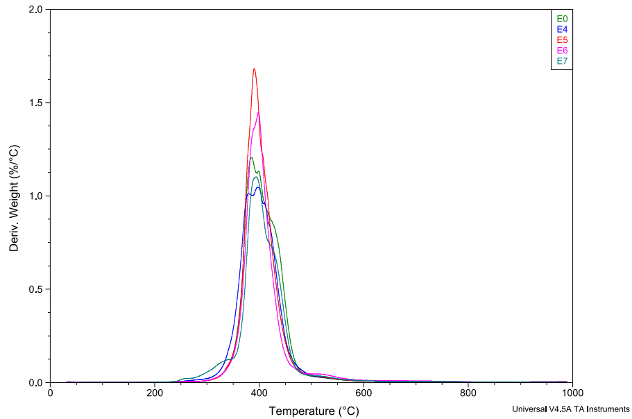
Şekil 10.19. İkinci grup tabanlı güç tutuşur karkılar ile sinerjistik olarak kullanılan ATH, \text{SbO}_3 ve ZnB katkıları kullanılarak üretilen epoksilaminelerin diferansiyel kütle kaybı sonuçları
