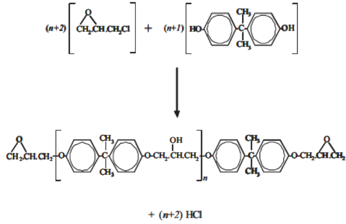
Şekil 5.5. Epoksi reçinelerin üretimi(bifenol A'nın diglisidil eteri)
