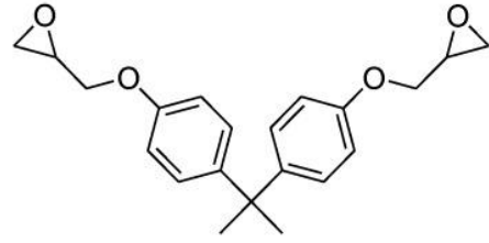
DGEBA
