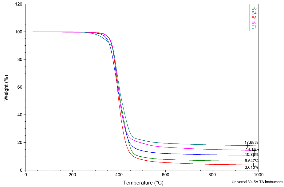
Şekil 10.18. İkinci grup tabanlı güç tutuşur karkılar ile sinerjistik olarak kullanılan ATH, \text{SbO}_3 ve ZnB katkıları kullanılarak üretilen epoksilaminelerin kütle kaybı sonuçları
