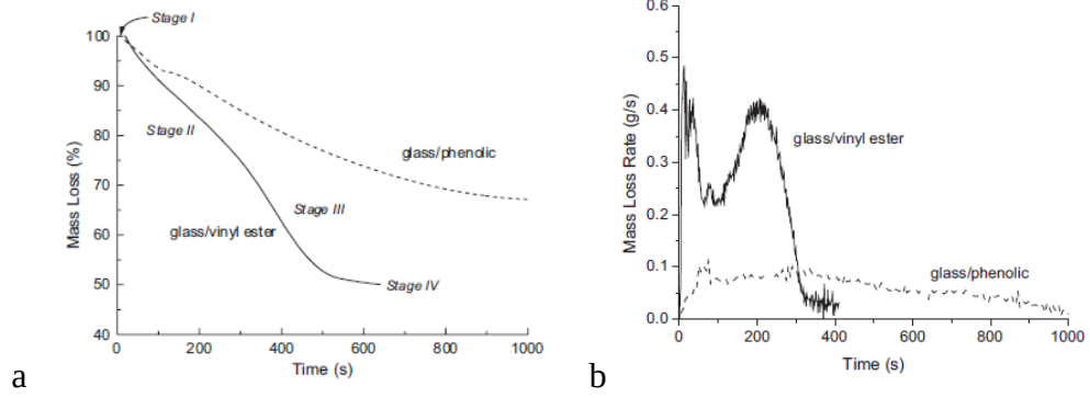
 ekil 6.7. Cam/vinil ester ve cam/fenolik lamineler i in k t le kaybı (a) ve k t le kayıp hızı(b) eęrileri
