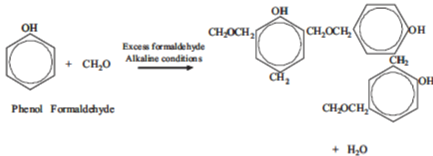
Şekil 5.3. Fenolik resol tipli reçinelerin hazırlanması ve yapısı
