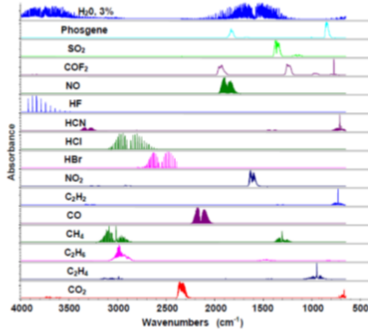
Şekil 7.1. Toksik gazların FTIR spektrumunda yer aldığı spesifik dalga boyu bantları
