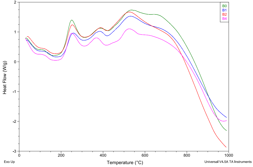
Şekil 10.13. %2 RP ve % 2 APP kimyasallarından oluşan fosfor tabanlı güç tutuşur katkıları kullanılarak üretilen benzozkazin laminelerindiferansiyel ısı salımı sonuçları
