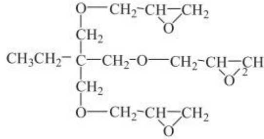
Şekil 5.16. Üç fonksiyonlu epoksi reçine (trimethylol propane-N-triglycidyl ether) kimyasal yapısı[46]
