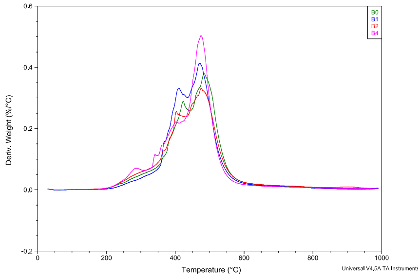
Şekil 10.12. %2 RP ve % 2 APP kimyasallarından oluşan fosfor tabanlı güç tutuşur katkıları kullanılarak üretilen benzzokzazin laminelerin diferansiyel kütle kaybı sonuçları
