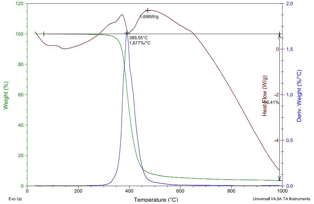
Şekil 10.15. %2 SbO3(E5) katkılanırılmış epoksi reçineye ait özet TGA sonucu
