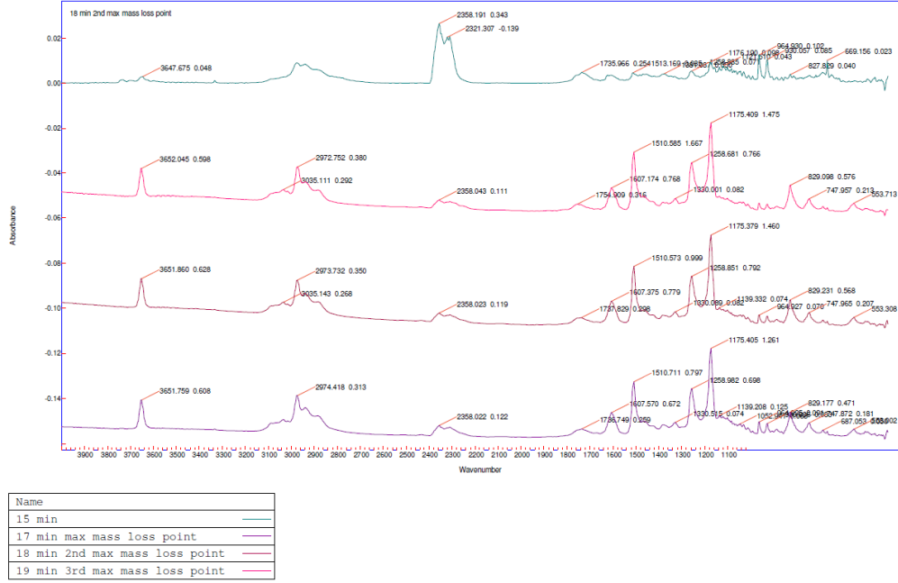
Şekil 10.22. E0 numunesi maksimum kütle kayıp noktalarında ekstrakte edilmiş FTIR spectrurları
