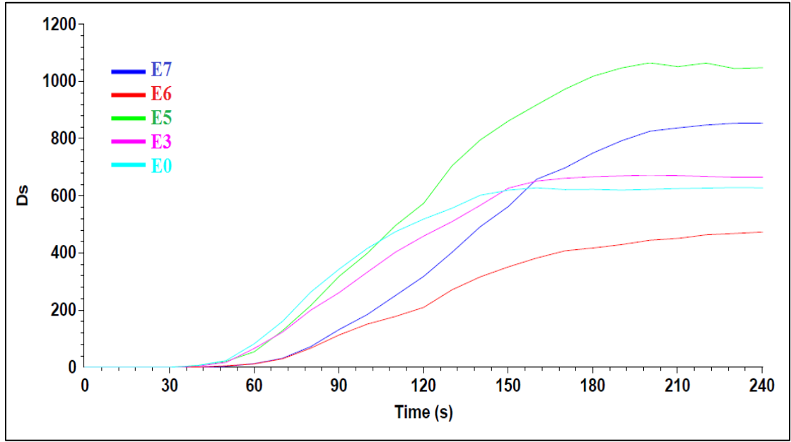
Şekil 10.31. Metal tabanlı katkı malzemelerinin duman yoğunluğu değerlerine olan etkisi
