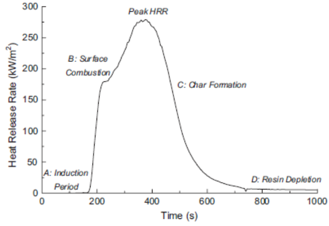
Şekil 6.5. 50 kW/m 2 ısı akısında cam/vinil eter kompozitler için ısı salınım hızı profili
