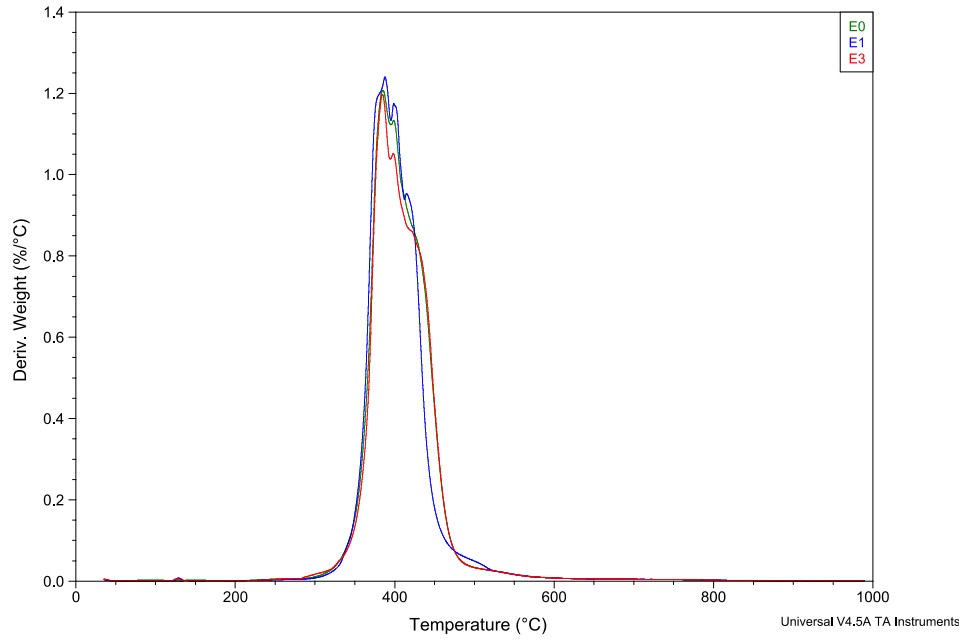
Şekil 10.7. %2 RP(E1) ve %2 APP(E2) kimyasallarından oluşan fosfor tabanlı güç tutuşur katkıları kullanılarak üretilen epoksi laminelerin diferansiyel kütle kaybı sonuçları
