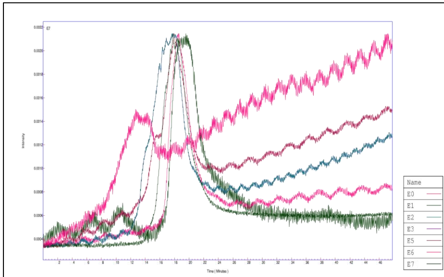
Şekil 10.21. Epoksi laminelerin TG analizinde termal bozumları süresince kayıt edilen FTIR spectrumları
