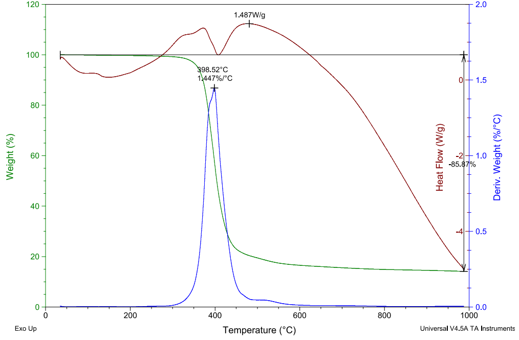
Şekil 10.16. %2 ZnB( E6) katkılanırılmış epoksi reçineye ait özet TGA sonucu
