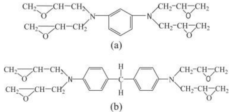
Şekil 5.17. Tetrafonksiyonel epoksi reçine kimyasal yapısı[46]
