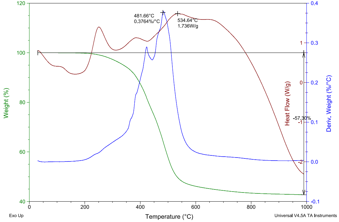
Şekil 10.2. Güç tutuşur katkılandırılmamış benzoksazin reçine (B0) TGA sonucu
