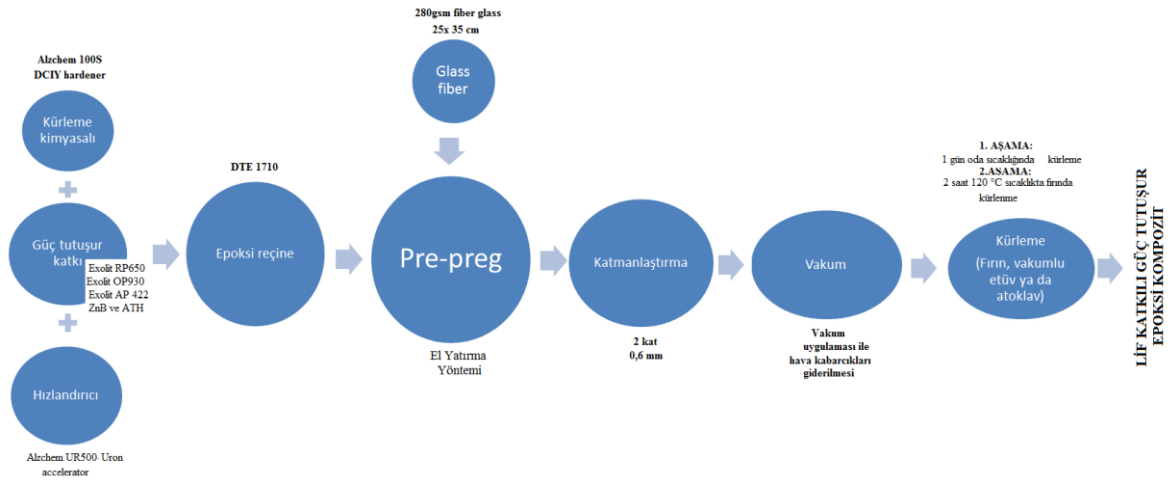
Şekil 9.1. Kompozit üretim şeması
