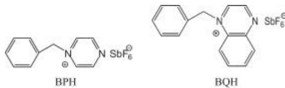
Şekil 5.22. N-benzilpirazinyum heksafluoroantimonat (BPH) ve N-benzilkuinoksalinyum heksafluoroantimonat (BQH) kimyasal yapıları [46]
