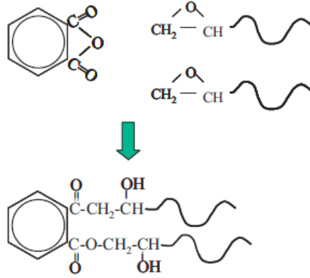
Şekil 5.8. Epoksi reçineler: anhidrit sertleştirici-basitleştirilmiş reaksiyon
