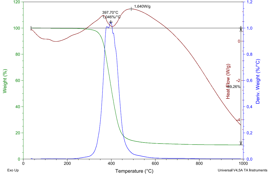
Şekil 10. 14. %2 ATH (E4) katkılanırılmış epoksi reçineye ait özet TGA sonucu
