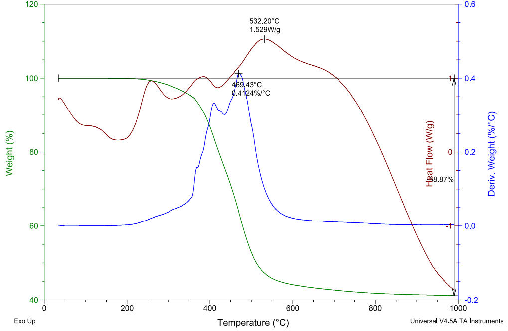
Şekil 10.9. %2 RP (B1) katkılandırılmış benzoksazin reçineye ait özet TGA sonucu
