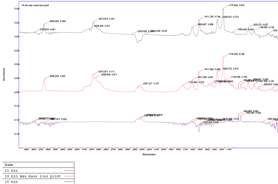
Şekil 10.27. E6 numunesi maksimum kütle kaybı noktalarında ekstrakte edilmiş FTIR specturmları
