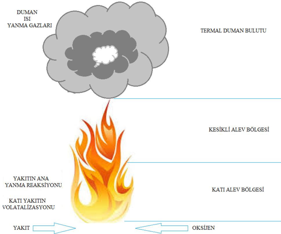
Şekil 6.1. Türbülanslı duman bulutu içerisindeki farklı zonların (bölgelerin) şematik gösterimi
