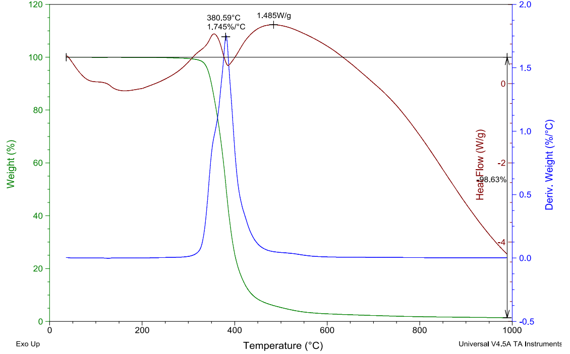
Şekil 10.5. %2 APP(E2) katkılандırılmış epoksi reçineye ait özet TGA sonucu
