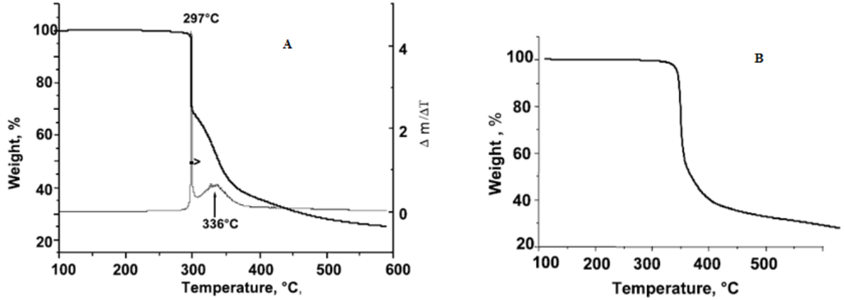
Şekil 8.2. %20 Br içeren BER termal bozunum eğrisi A: HRTG, B: TG [68]
