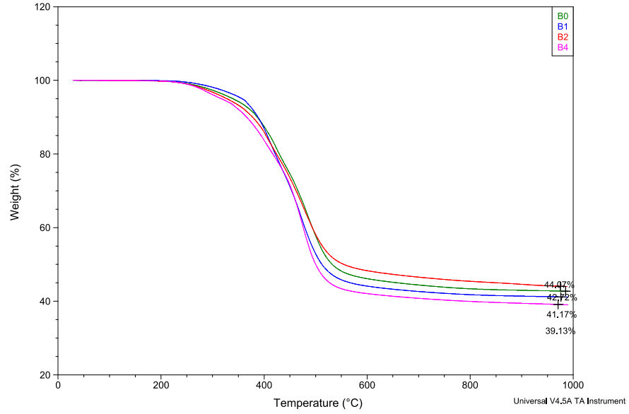
Şekil 10.11. %2 RP ve % 2 APP kimyasallarından oluşan fosfor tabanlı güç tutuşur katkıları kullanılarak üretilen benzzokzazin laminelerin kütle kaybı sonuçları
