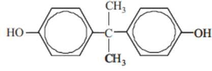
Şekil 5.4. Bisfenol A
