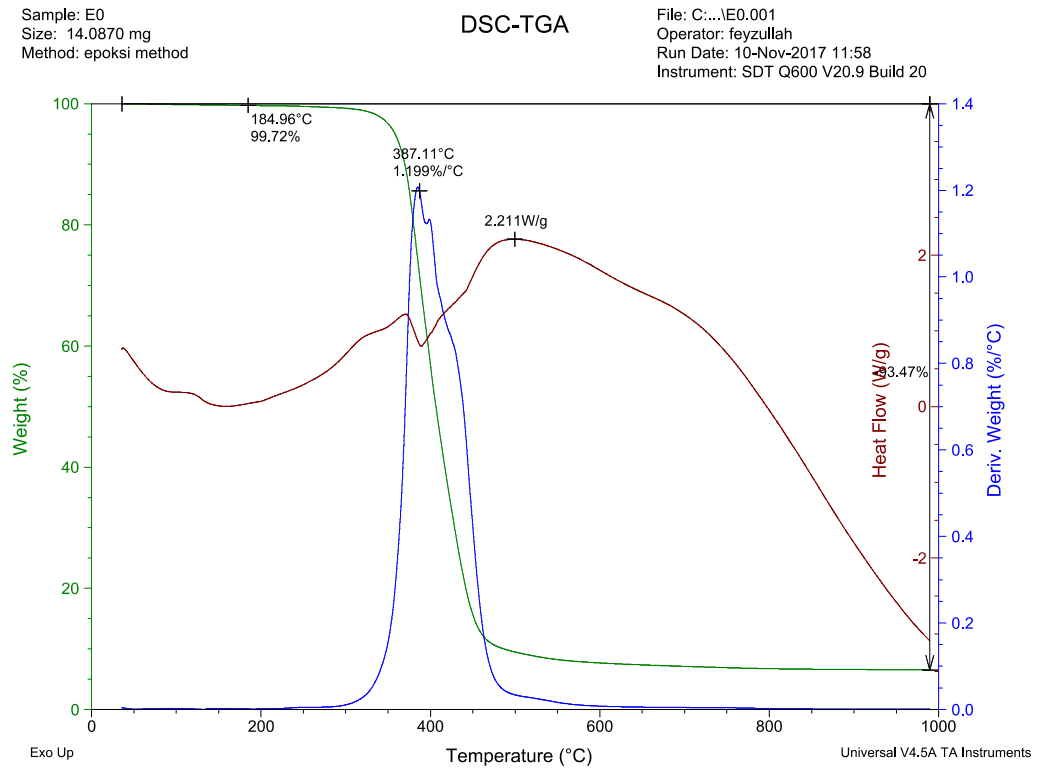
Şekil 10.1. Güç tutuşur katkılandırılmamış epoksi reçine (E0) TGA sonucu
