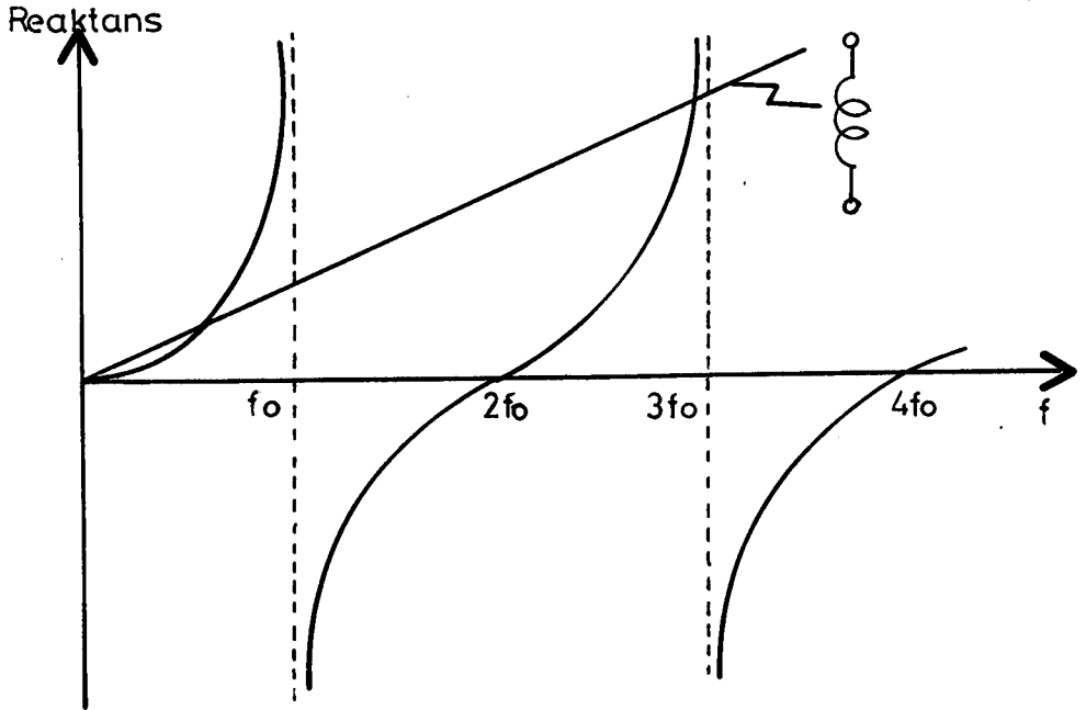
Şekil 4.4 Sonu kısa devre kayıpsız iletim hattının ve bir bobinin reaktansının frekansa göre değişimi
