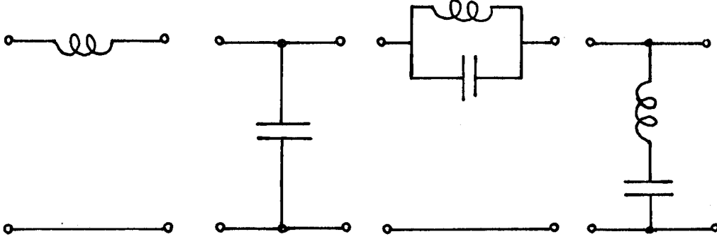
Şekil 3.3 Alçak geçiren devre elemanları
