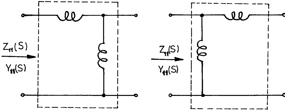
Şekil 3.5 Band geçiren tipinde iki kapılı devreler.
