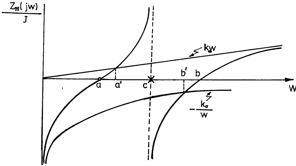
Şekil 3.2 Z_{11} Reaktans fonksiyonunun frekansa göre değişimi
