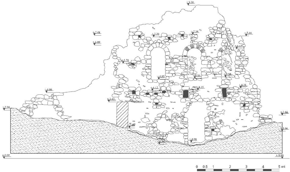
Çizim 12. Peristyl'in doğu duvarı
