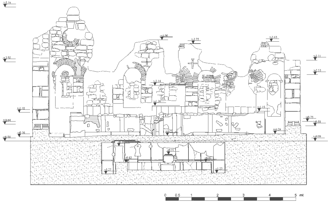
Çizim 13. Peristyl kuzey-güney kesiti batıya bakış
