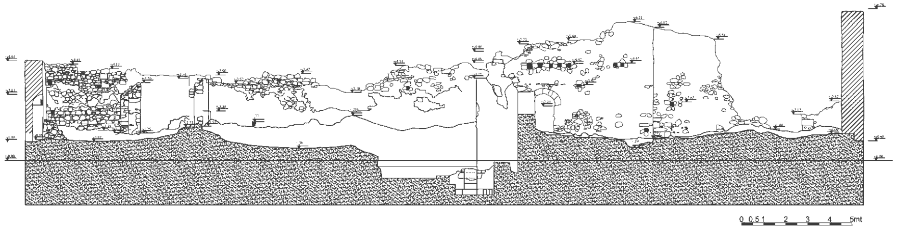
Çizim 8. Vaftizhane doğu-batı kesiti kuzeye bakış
