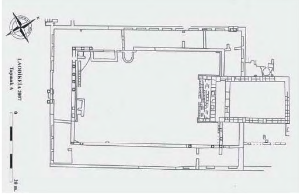
A) Laodikeia Antik Kenti, Tapınak A plânı.
