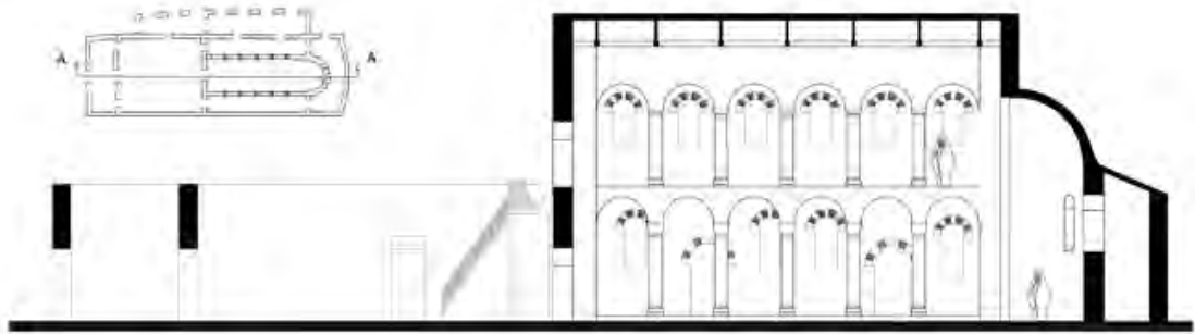
B) S5-IX sektöründe yer alan kilisenin kesit restitüsyonu.
