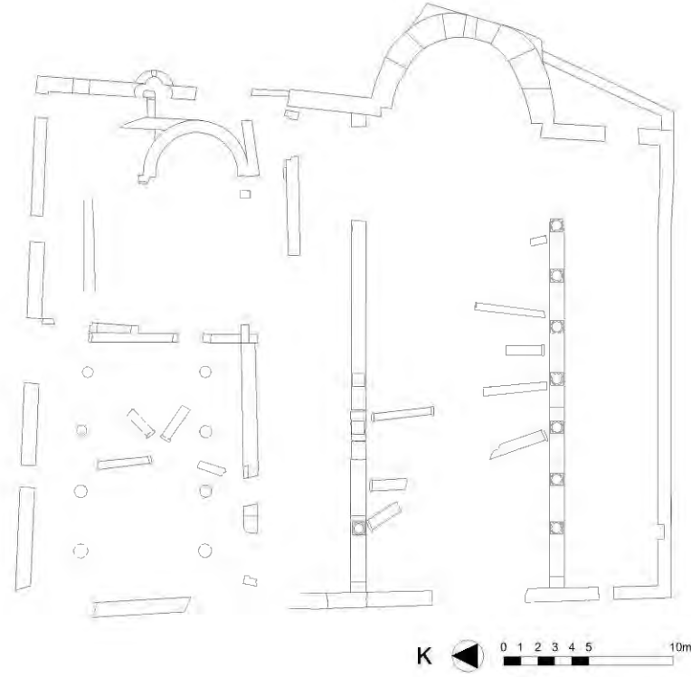
A) S5-V sektöründeki kilisenin plânı. (Liman Bazilikası)
