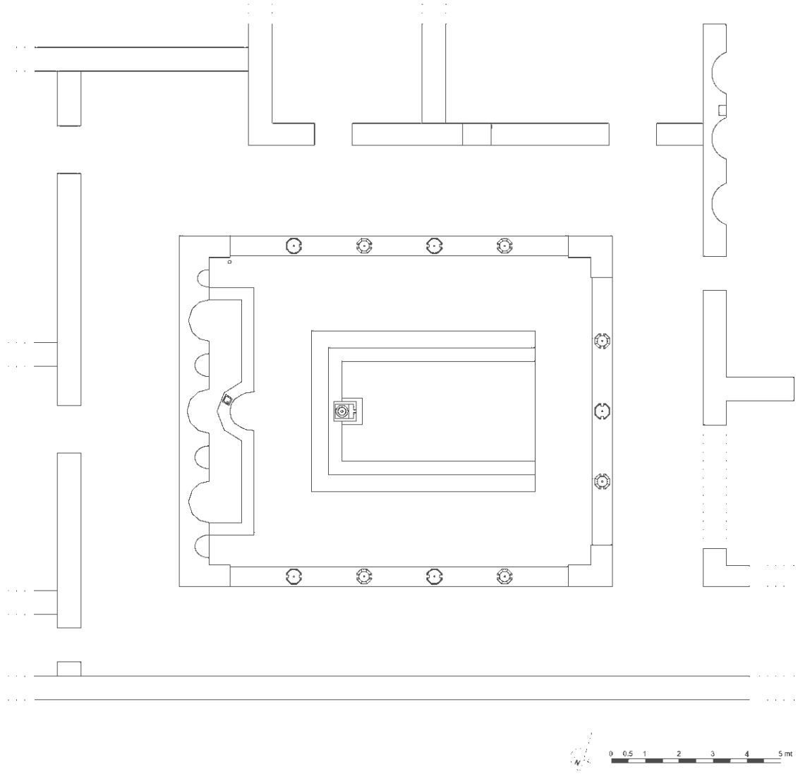
Çizim 23. Peristyl plân restitüsyonu
