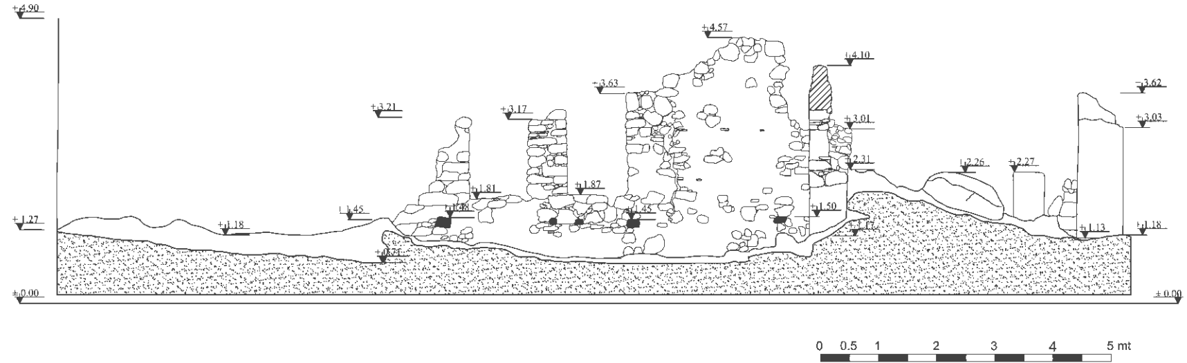
Çizim 6. Kilise güney ek mekânı doğu-batı kesiti güneye bakış
