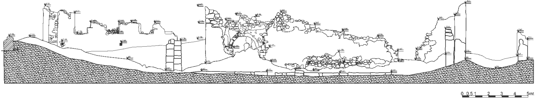
Çizim 3. Kilise doğu-batı kesiti güneye bakış
