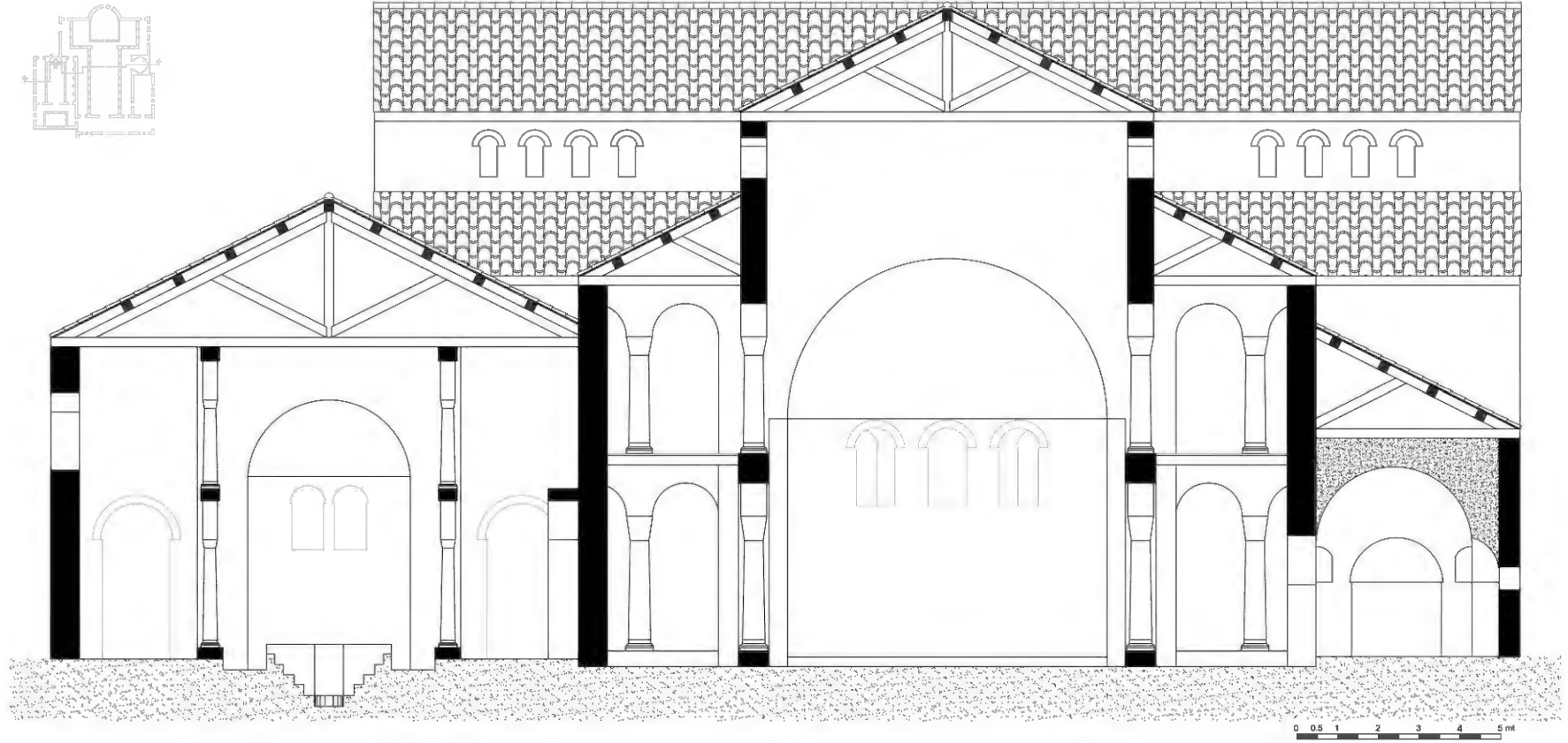
Çizim 20. Kilise ve vaftizhane kuzey-güney kesit restitüsyonu
