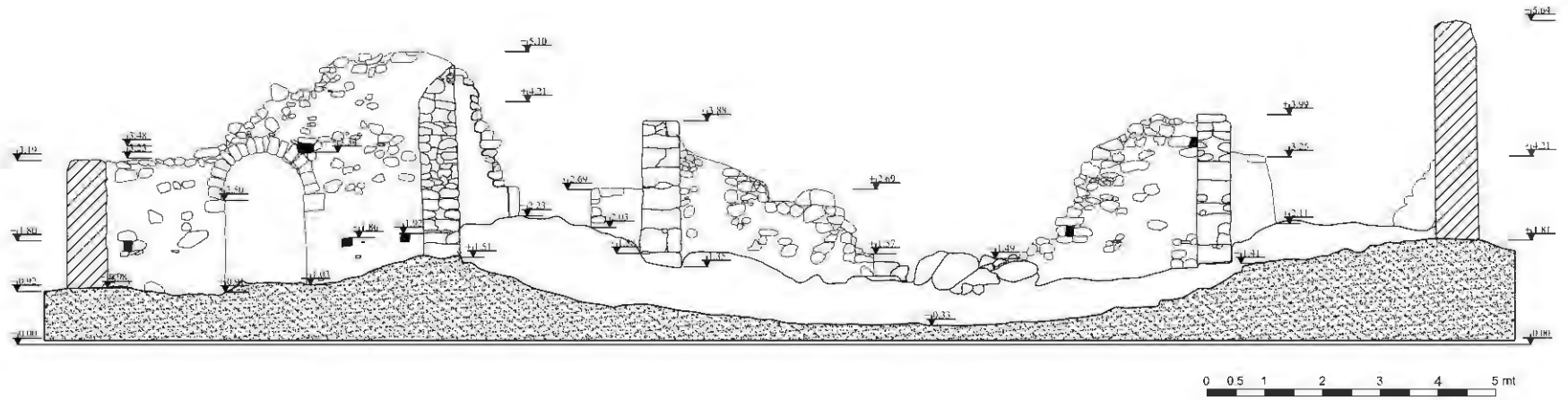
Çizim 2. Kilise kuzey-güney kesiti batıya bakış
