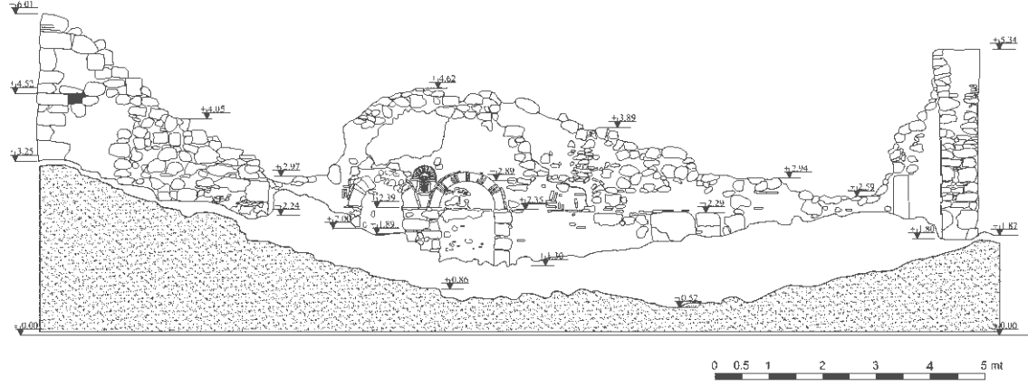
Çizim 11. Triclinium ana mekânı doğu duvarı
