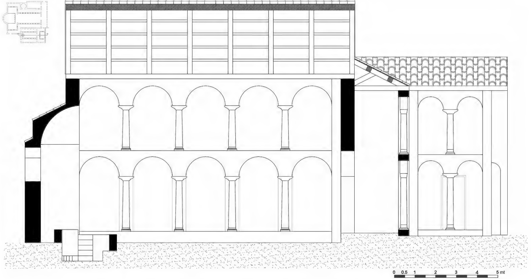
Çizim 22. Vaftizhane doğu-batı kesit restitüsyonu
