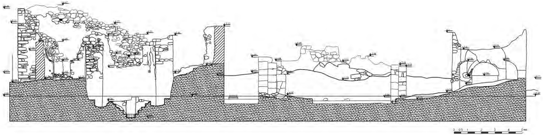
Çizim 1. Kilise ve vaftizhane kuzey-güney kesiti doğuya bakış
