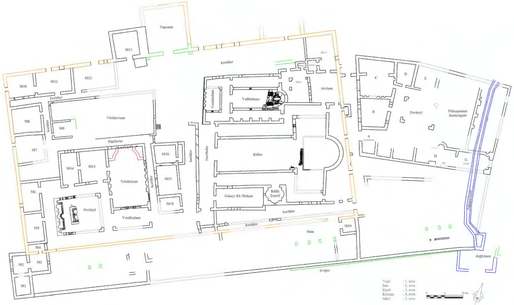
Plân 5. Episkopeion içerisinde tespit edilen inşa evreleri
