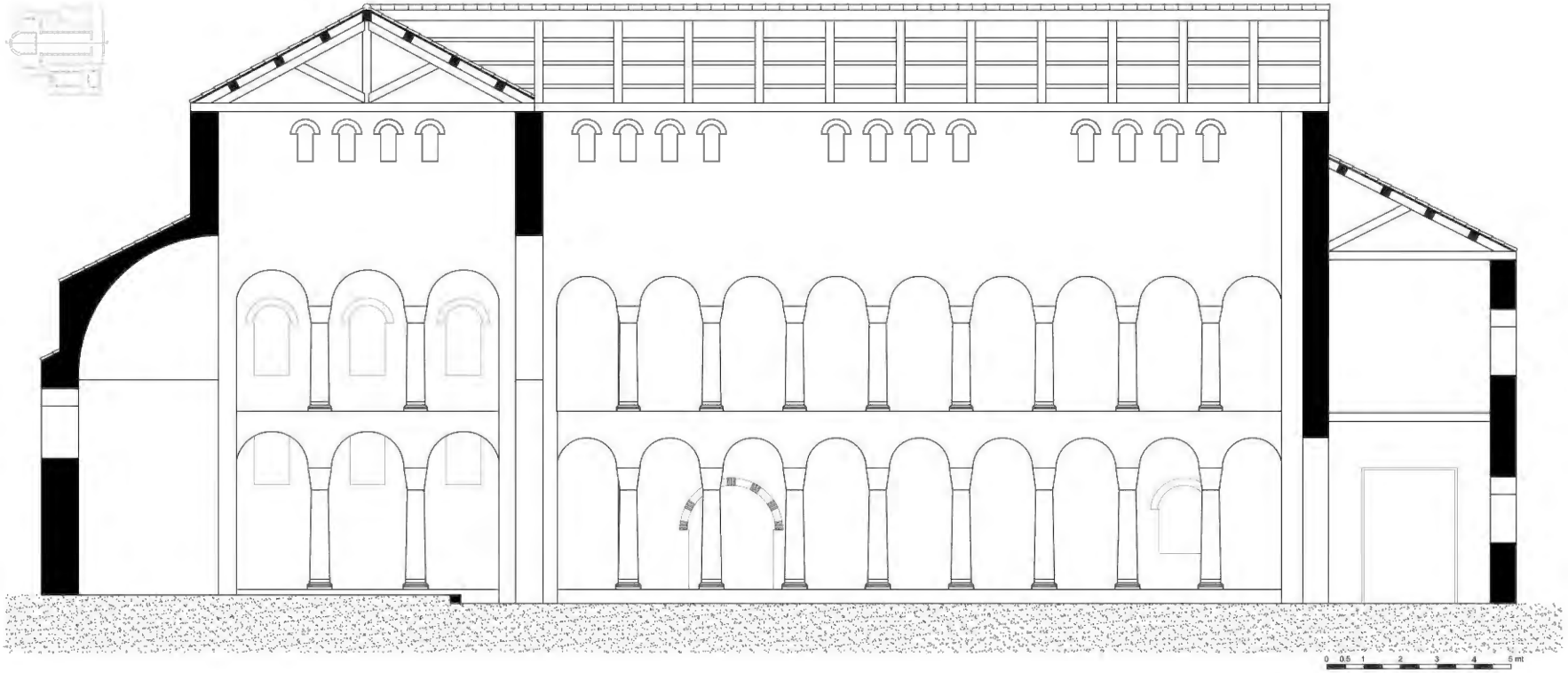
Çizim 21. Kilise doğu-batı kesit restitüsyonu
