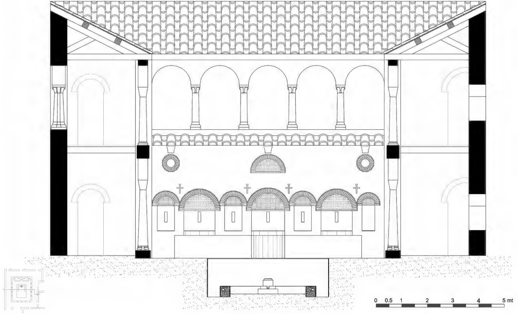
Çizim 25. Peristyl kuzey-güney kesit restitüsyonu
