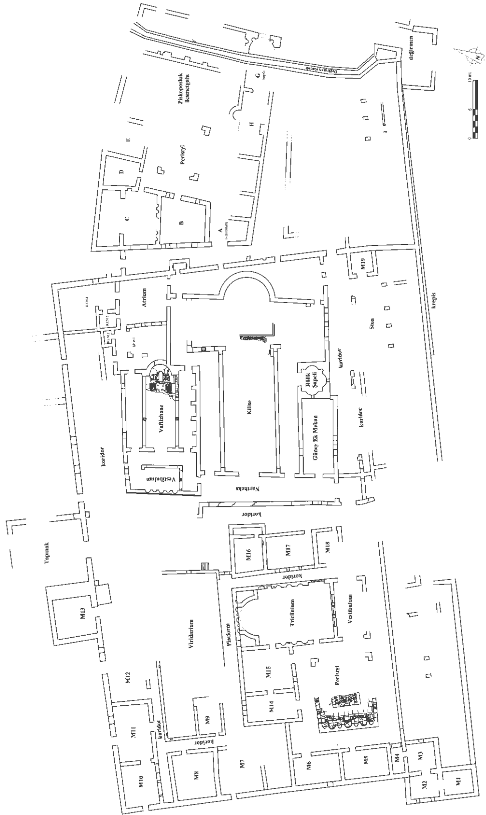
Şekil 21. Episkopeion röleve plânı
