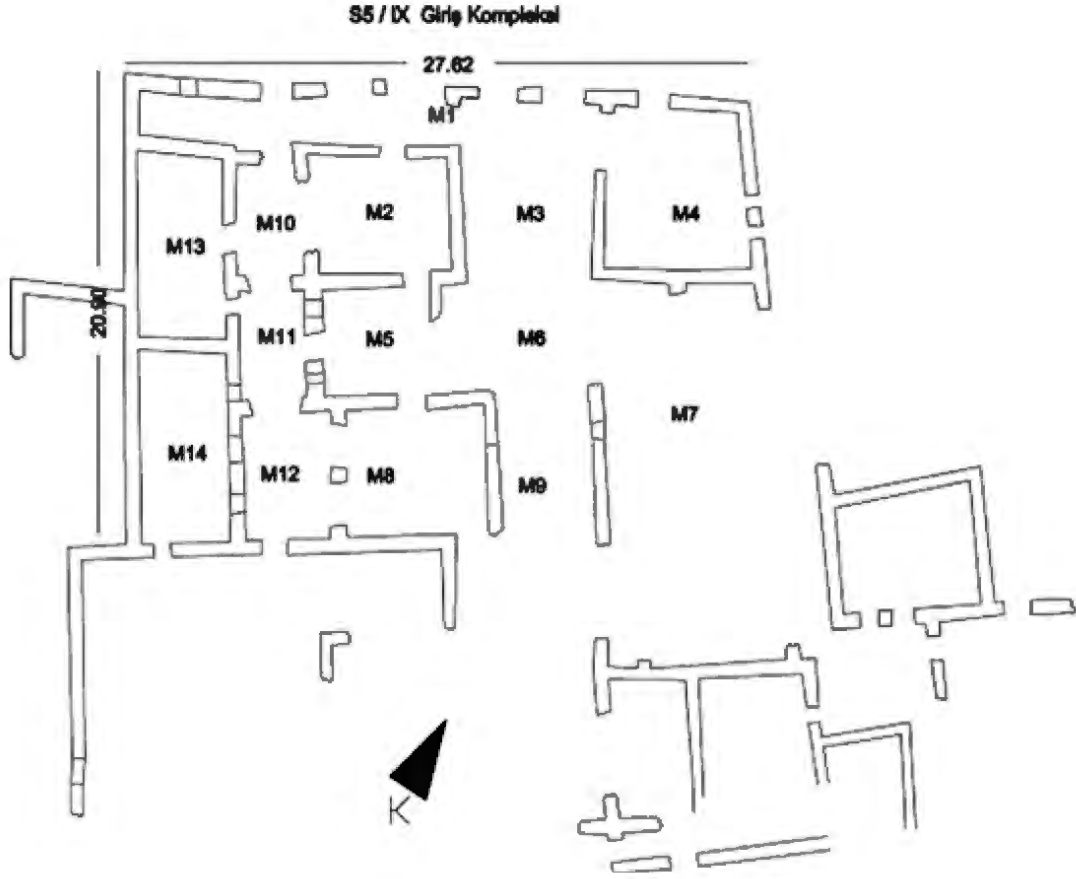
A) Giriş Kompleksi'nin plânı.
