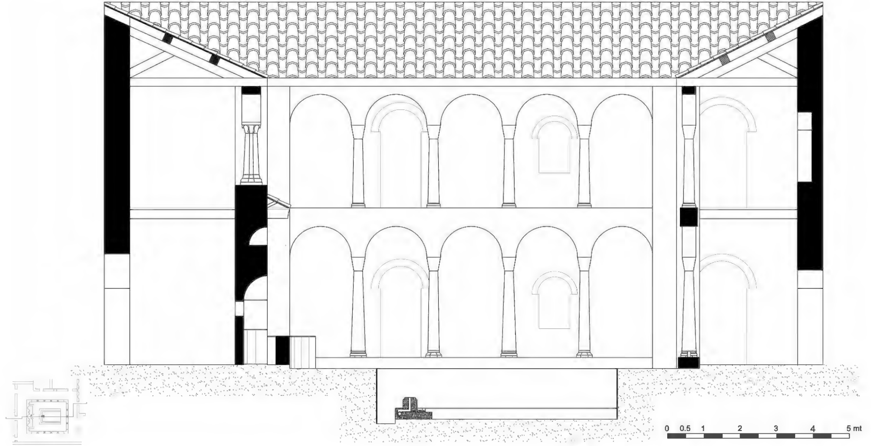
Çizim 24. Peristyl doğu-batı kesit restitüsyonu
