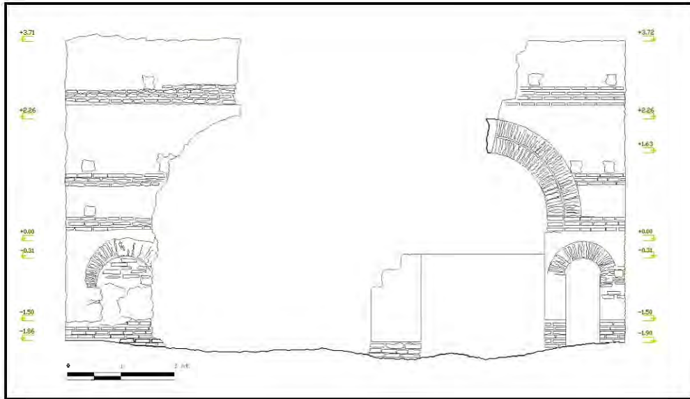
B) Vespasianus Hamamı tepidarium güney iç cephe çizimi.
