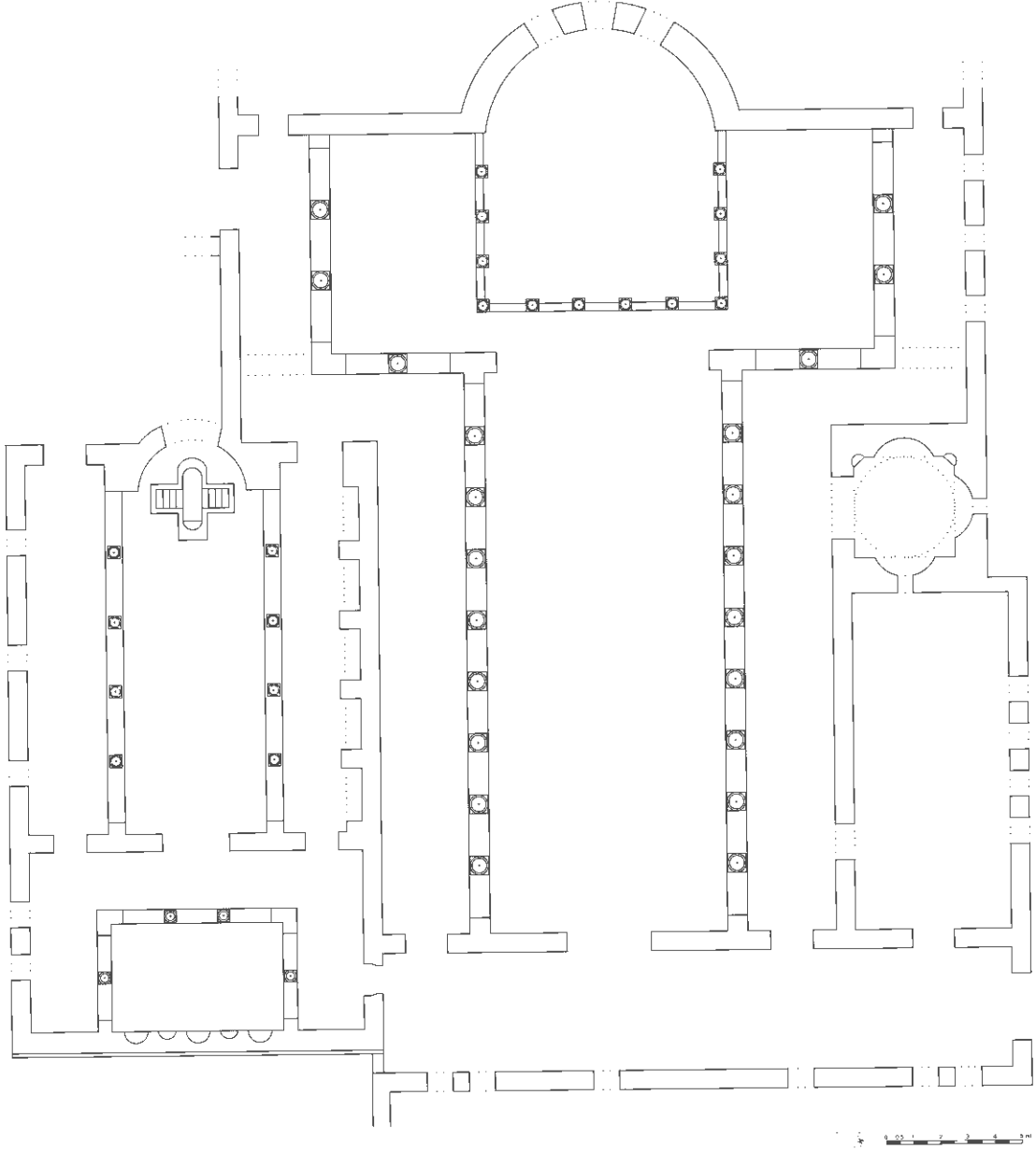
Çizim 19. Kilise ve vaftizhane plân restitüsyonu
