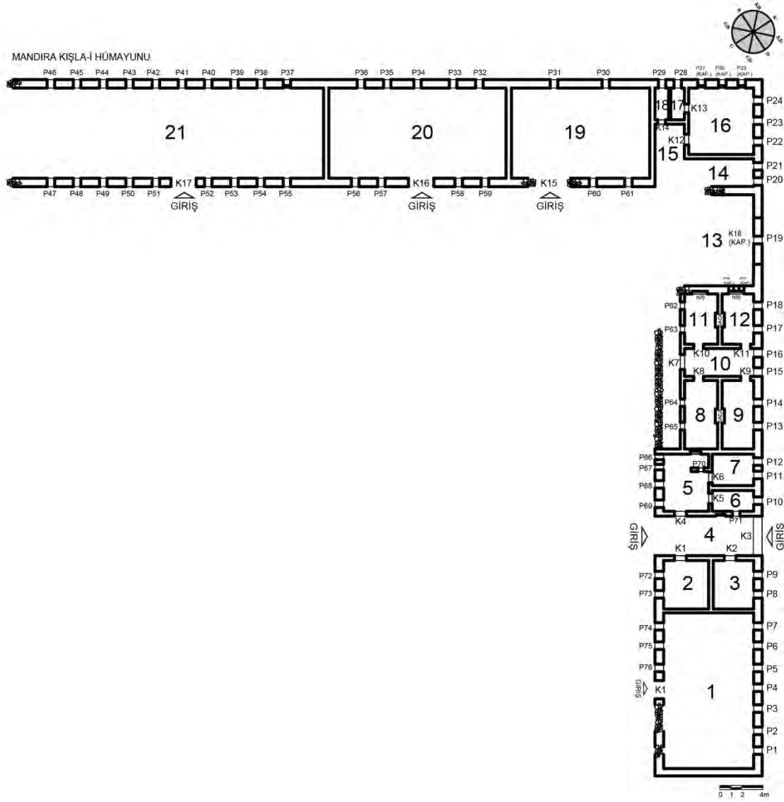
Şekil 3. 44. Mandıra Kışla-i Hümayunu'nun plan krokisi (25.07.2018) (Çizen: Ece GÜLER).
