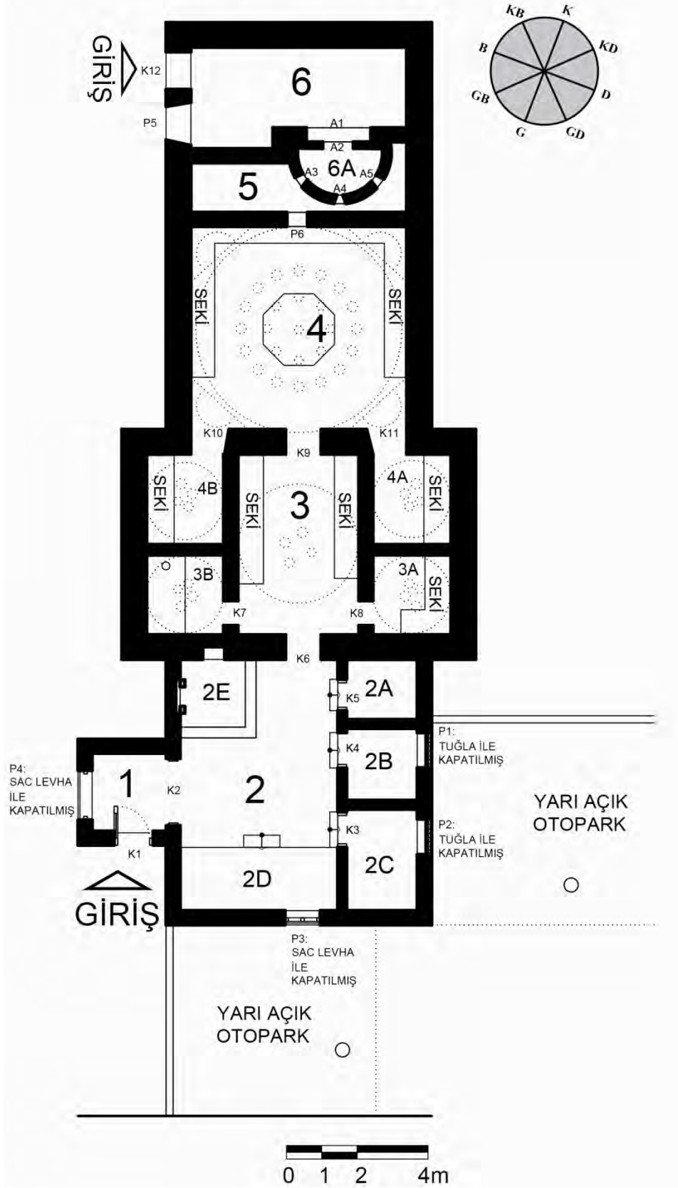
Şekil 3. 32. Mahmudiye mevkiinde bulunan hamamın plan krokisi (25.07.2018) (Çizen: Ece GÜLER).
