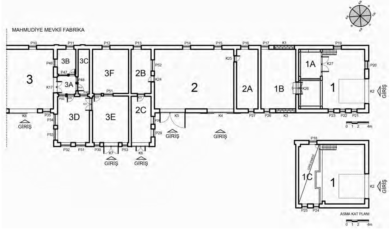
Şekil 3. 27. Mahmudiye mevkiinde bulunan fabrikanın plan krokisinde gösterilen 1, 2 ve 3 numaralı mekânlar (25.07.2018) (Çizen: Ece GÜLER).
