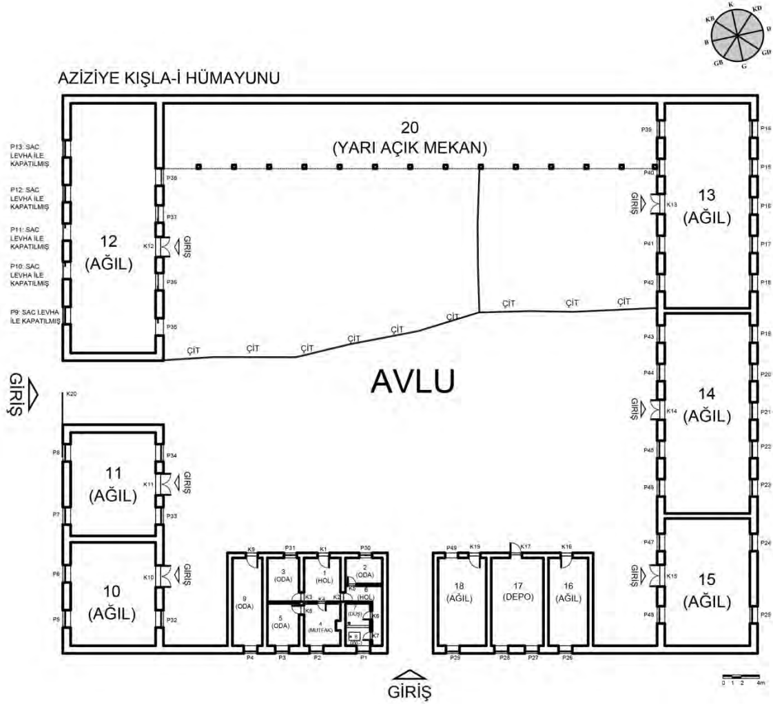
Şekil 3. 35. Aziziye Kışla-i Hümayunu'nun plan krokisi (25.07.2018) (Çizen: Ece Güler).
