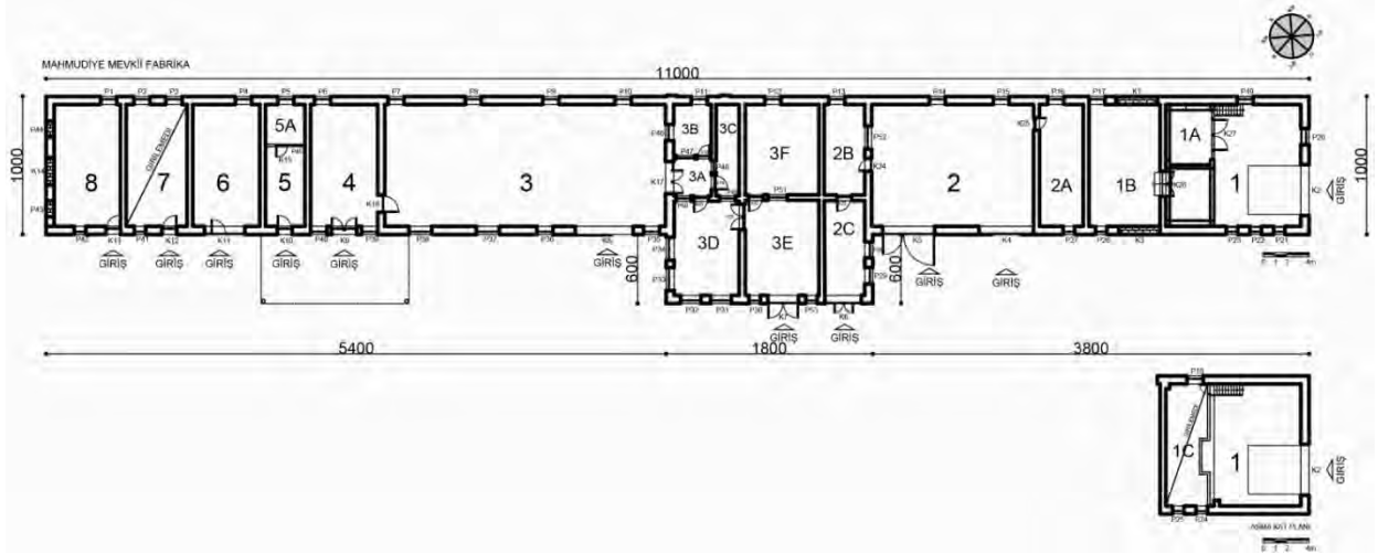
Şekil 3. 25. Mahmudiye mevkiinde bulunan fabrikanın plan krokisi (25.07.2018) (Çizen: Ece GÜLER).
