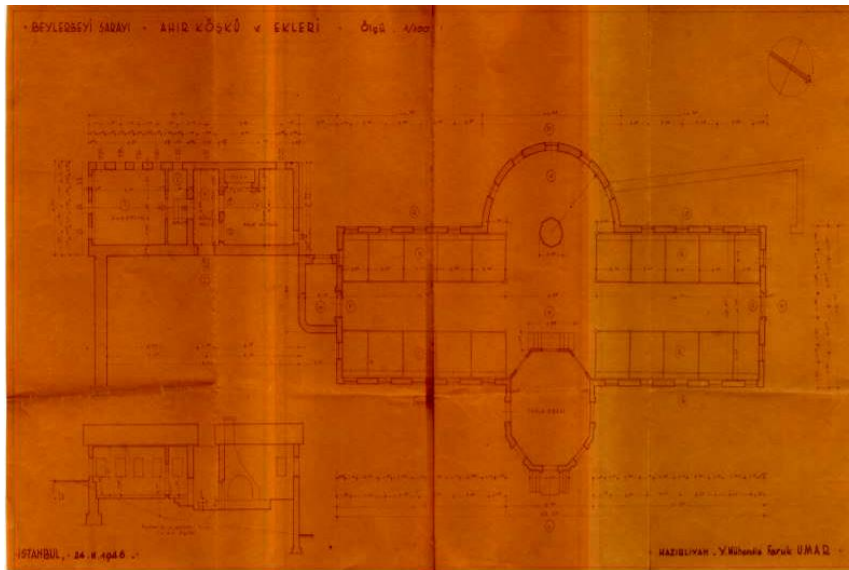
Görsel 2. 7. Beylerbeyi Sarayı'nda bulunan has ahır, samanlık ve mutfağın 1946 yılına ait planı (Göncü, 2006, s. 162)
