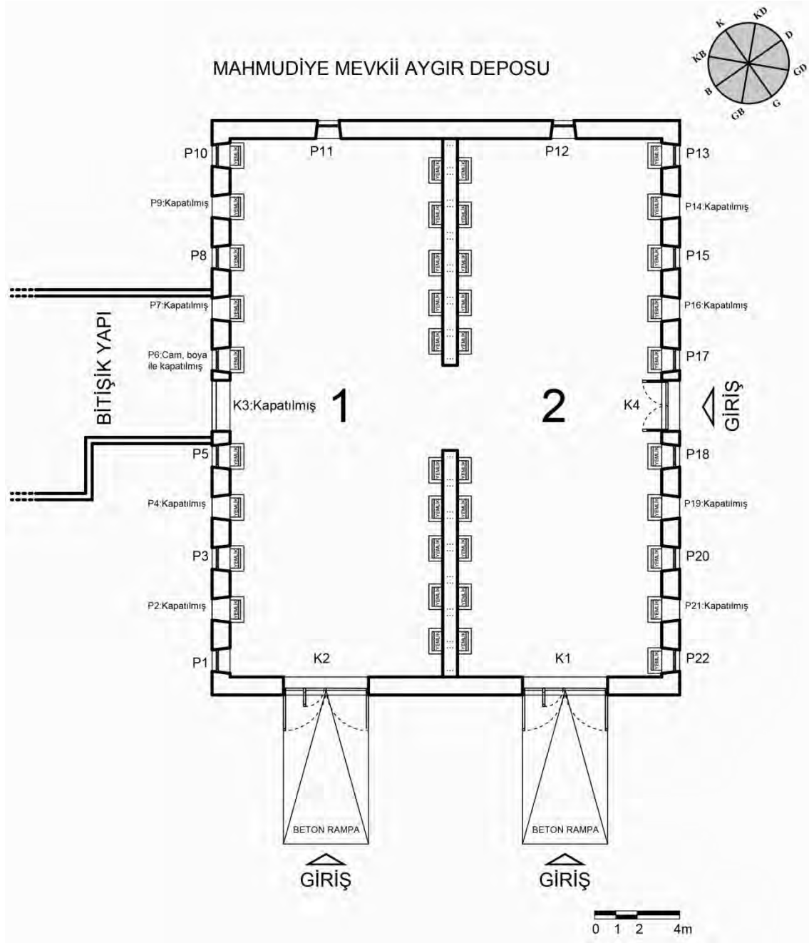
Şekil 3. 23. Mahmudiye mevkiinde bulunan aygır deposunun plan krokisi (25.07.2018) (Çizen: Ece GÜLER).
