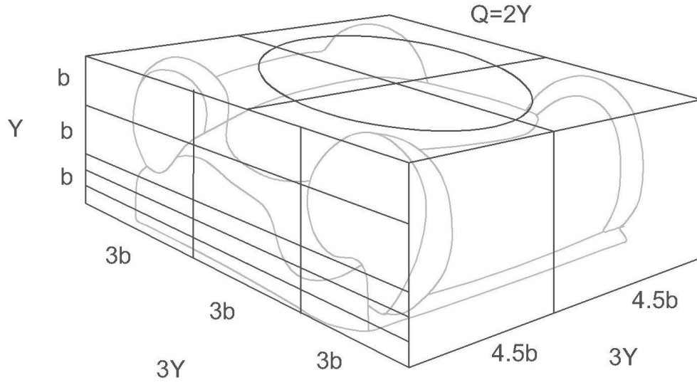
Çizim-3.2: Standart Prokonnesos Üretimi Antik Çağ İon Sütun Başlığı Oranları
