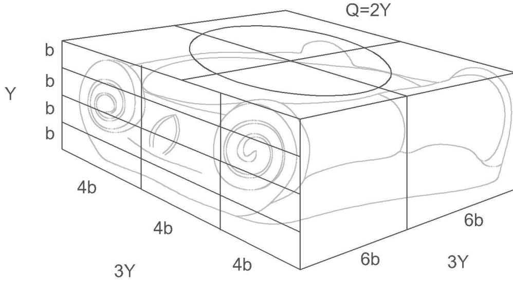
Çizim-3.3: Standart Prokonnesos Üretimi Geç Antik Çağ İon Sütun Başlığı Oranları
