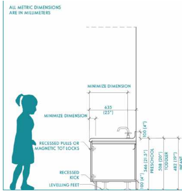
Görsel 2.13. Lavabo ve çocuk ilişkisi (LGA Architectural Partners. 2016. s.58.)
