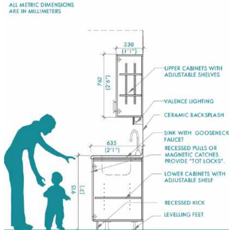
Görsel 2.14. Yetişkin lavabosu ve çocuk ilişkisi (LGA Architectural Partners. 2016. s.56.)
