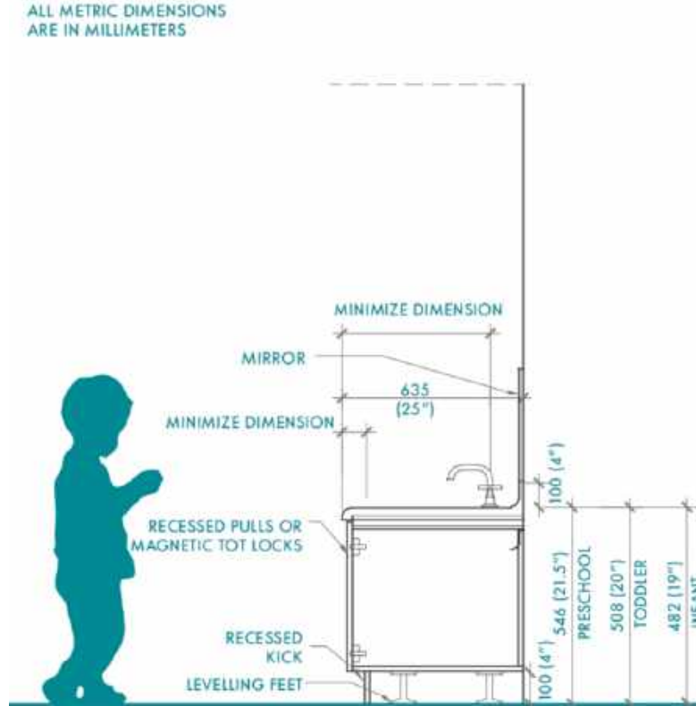
Görsel 2.15. El yıkama alanı ve çocuk ilişkisi (LGA Architectural Partners. 2016. s.71.)
