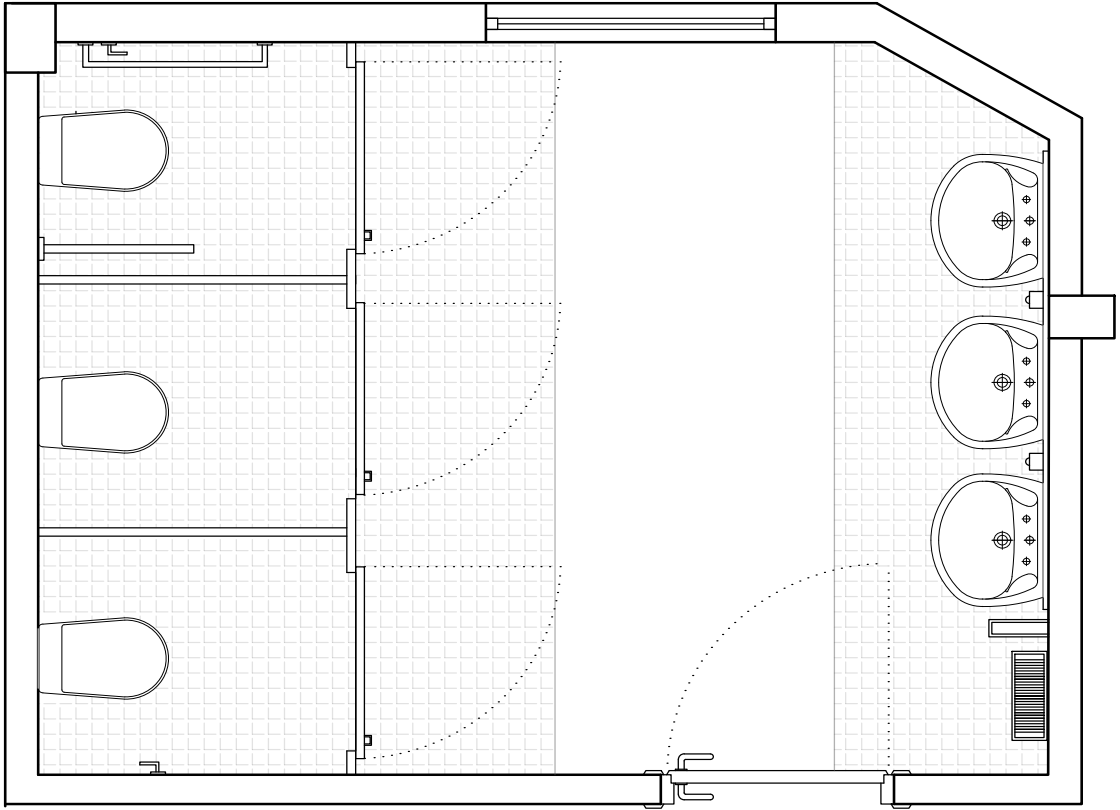
Görsel 4.13. Altın Çocuk Akademi Sümer tuvalet alanı ölçeksiz uygulama eskiz planı
