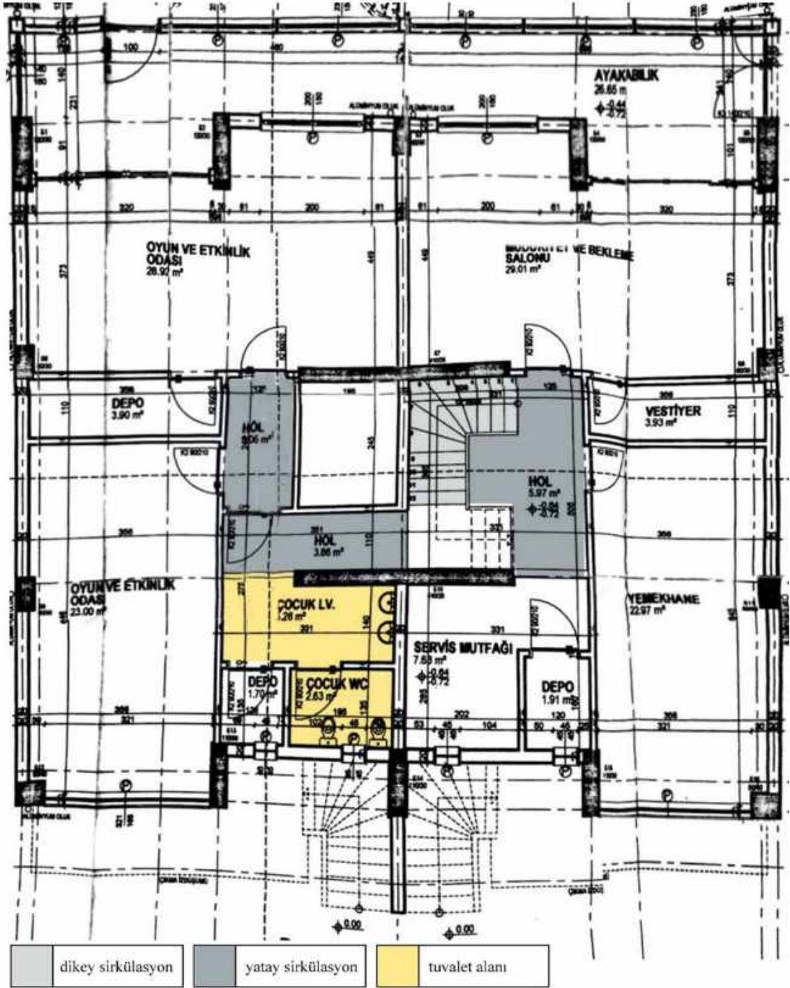
Görsel 4.1. Batıkent Altın Çocuk Akademi giriş kat planı
