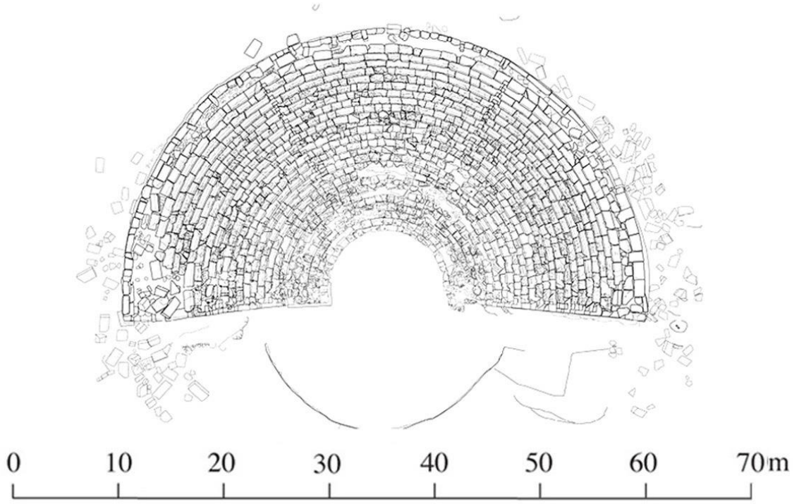
Görsel 70: Antiphellos Tiyatrosu Planı.
