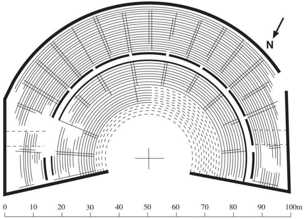
Görsel 68: Letoon Tiyatrosu Planı.
