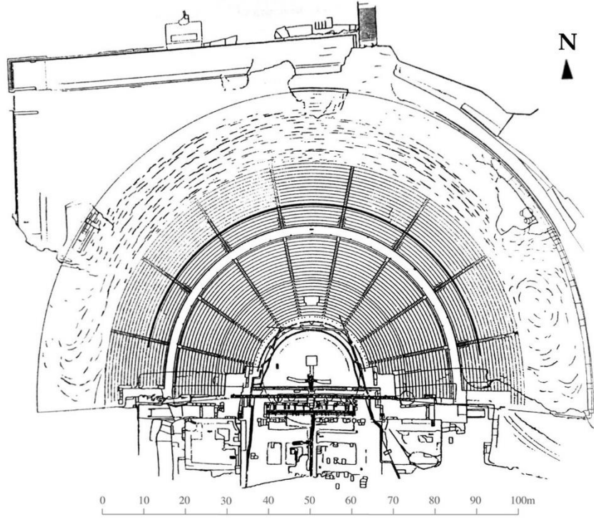
Görsel 46: Syrakusai Tiyatrosu Planı.
