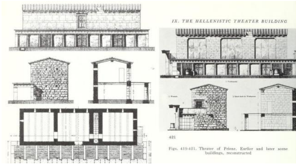
Görsel 73: Hellenistik Dönem, Erken ve Geç Evreli Priene Skene Yapısı.
