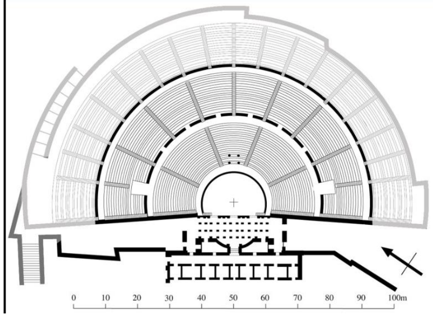
Görsel 57: Miletos Tiyatrosu Planı.
