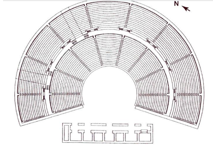
Görsel 59: Kaunos Tiyatrosu Planı.
