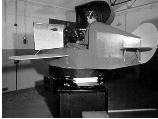
Şekil 3.1. Link Trainer uçuş simülatörü 9
