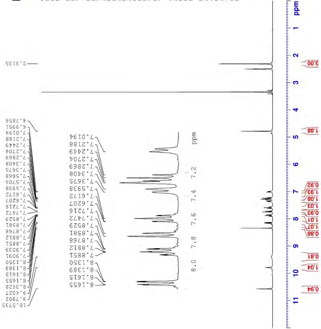
Şekil 5.20. Bileşik 4c'ye ait ^1\text{H} NMR spektrumu
