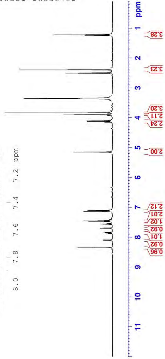
Şekil 5.76. Bileşik 8j'ya ait 1 H NMR spektrumu
