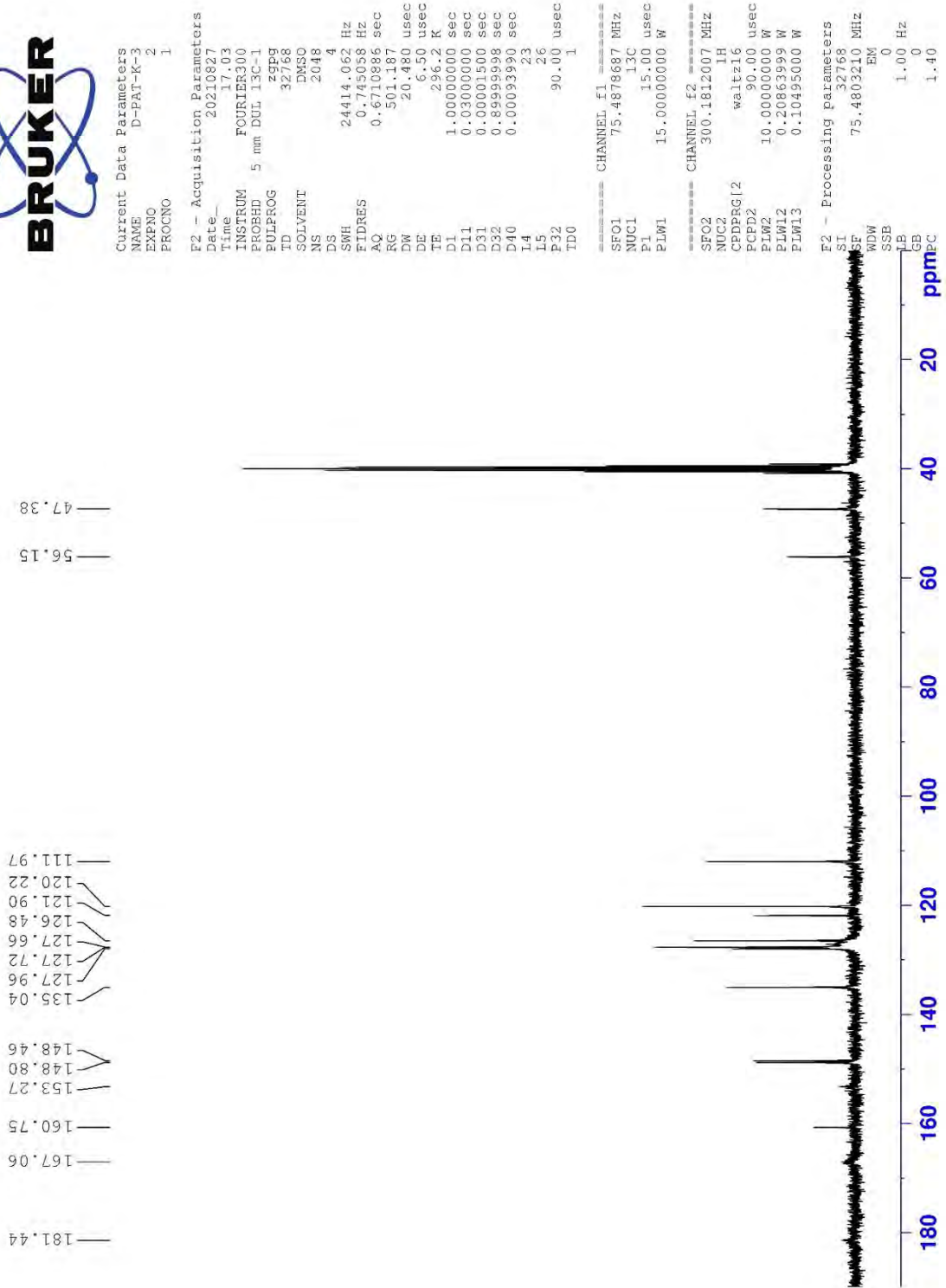
Şekil 5.15. Bileşik 4c'ye ait ^{13}\text{C} NMR spektrumu
