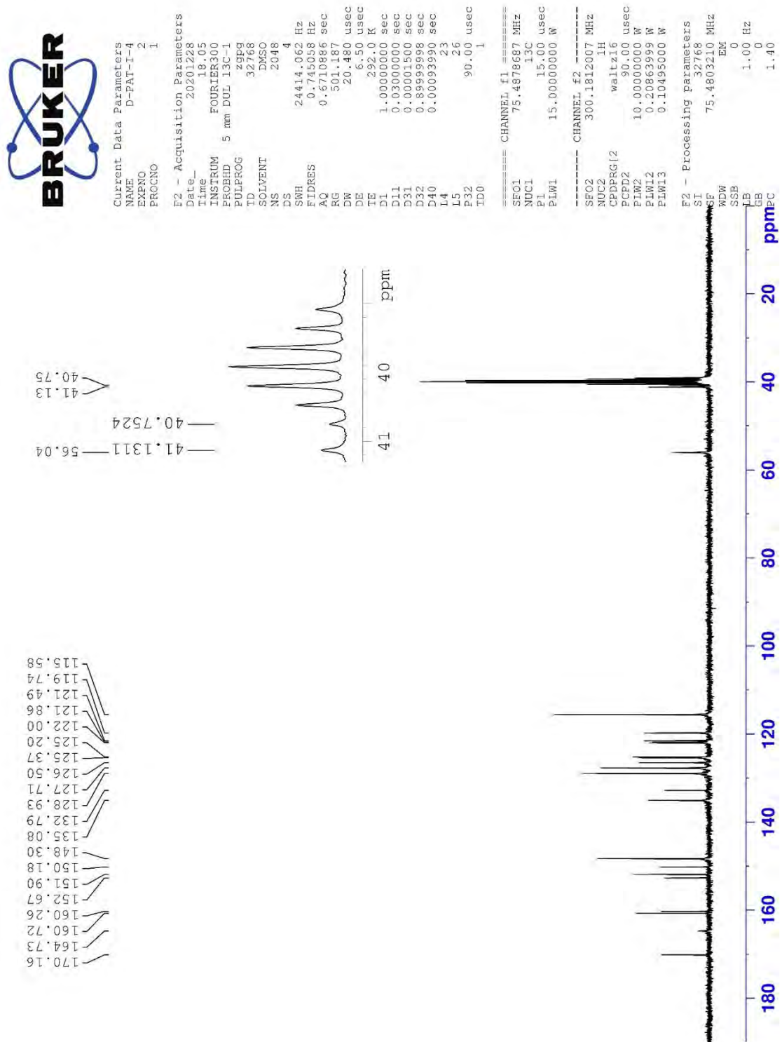
Şekil 5.59. Bileşik 8d'ya ait ^{13}\text{C} NMR spektrumu
