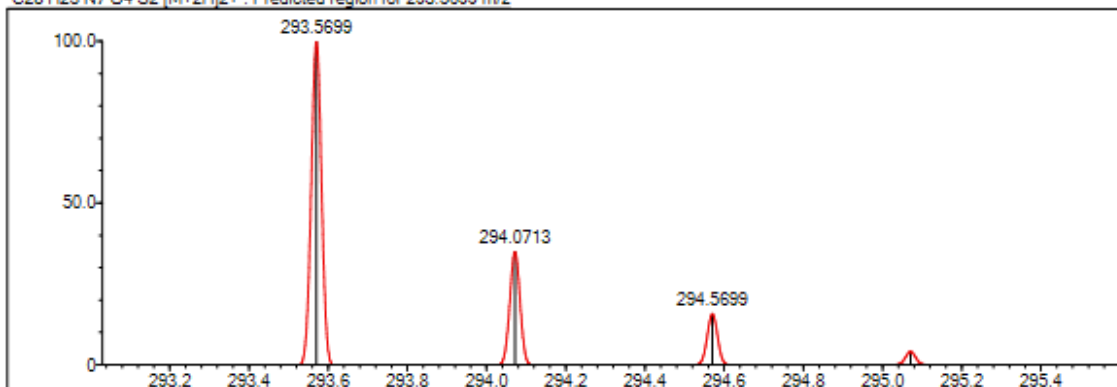
Şekil 5.66. Bileşik 8f'ya ait HRMS spektrumu
