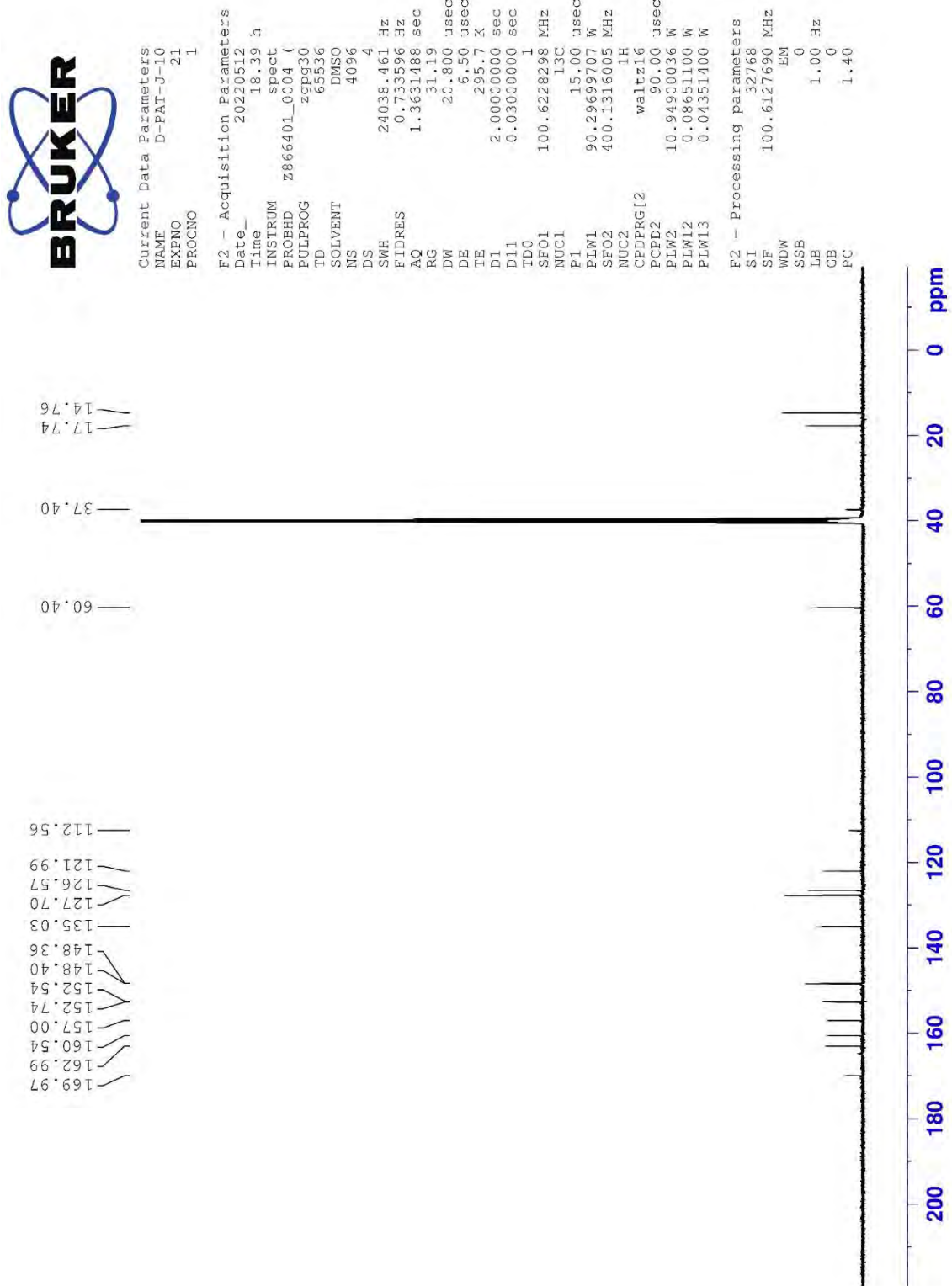
Şekil 5.110. Bileşik 8u'ya ait ^{13}\text{C} NMR spektrumu
