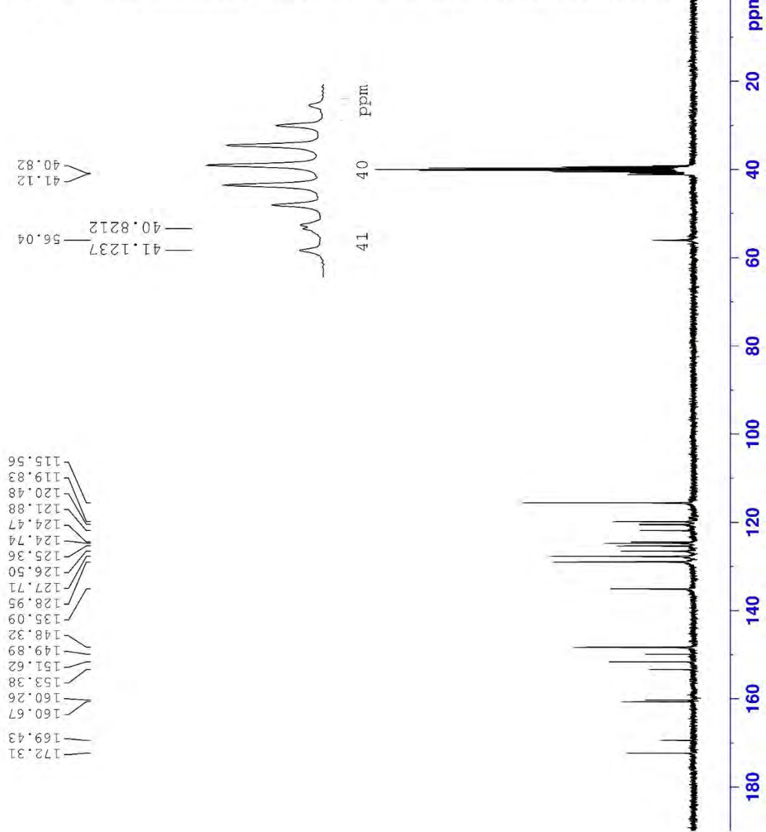
Şekil 5.53. Bileşik 8b'ya ait ^{13}\text{C} NMR spektrumu
