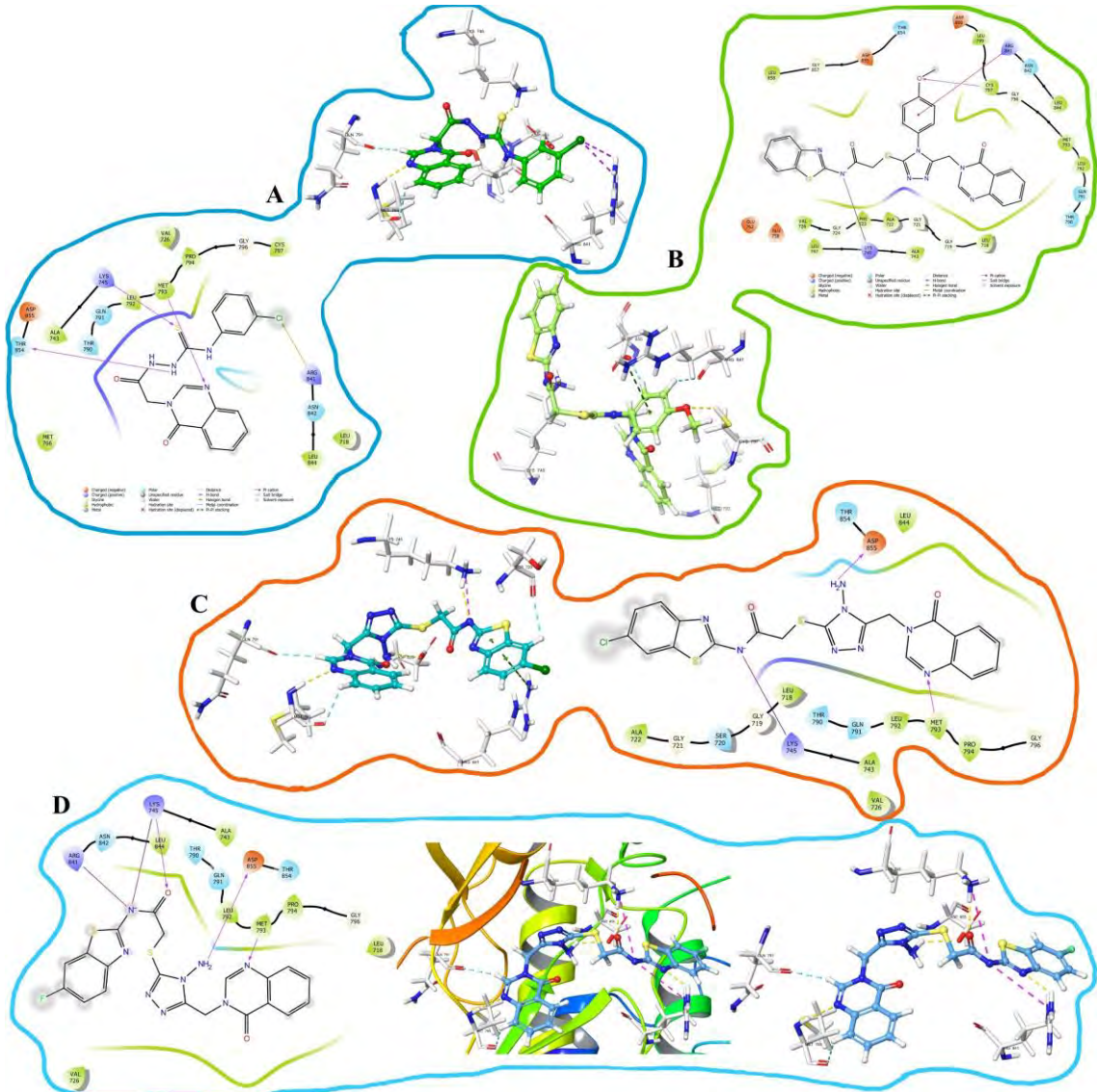
Şekil 5.132. EGFR proteini üzerindeki yerleştirme çalışması (PDBID: 2ITY)
