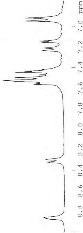
Şekil 5.115. Bileşik 13a'ya ait ^1\text{H} NMR spektrumu
