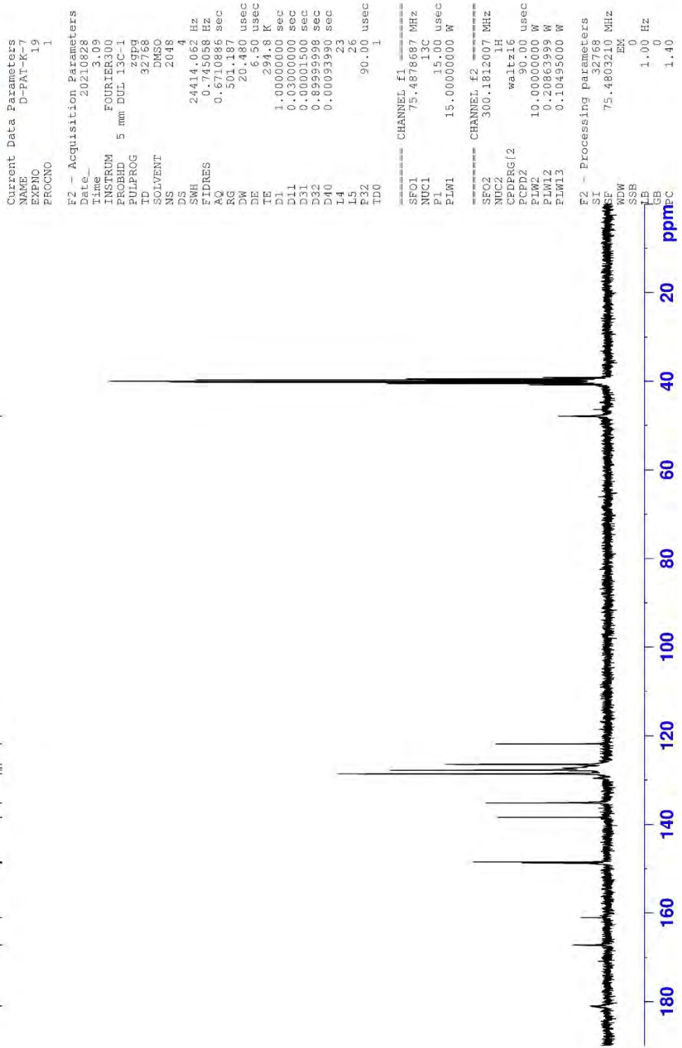
Şekil 5.27. Bileşik 4g'ye ait ^{13}\text{C} NMR spektrumu
