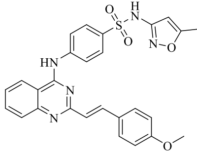
Şekil 2.9. Kinazolin ve N -arilsülfonilamit içeren apoptoz indükleyici EGFR inhibitörleri
