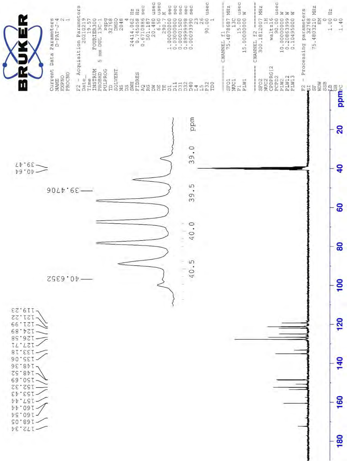
Şekil 5.92. Bileşik 80'ya ait ^{13}\text{C} NMR spektrumu
