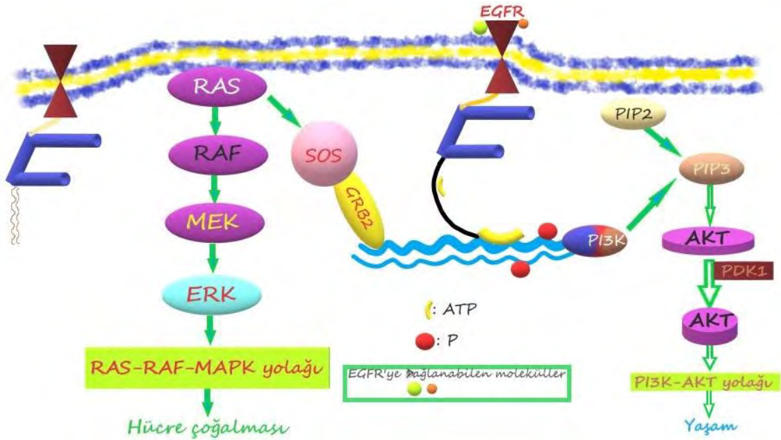
Şekil 2.1. EGFR yolağının şematik özeti
