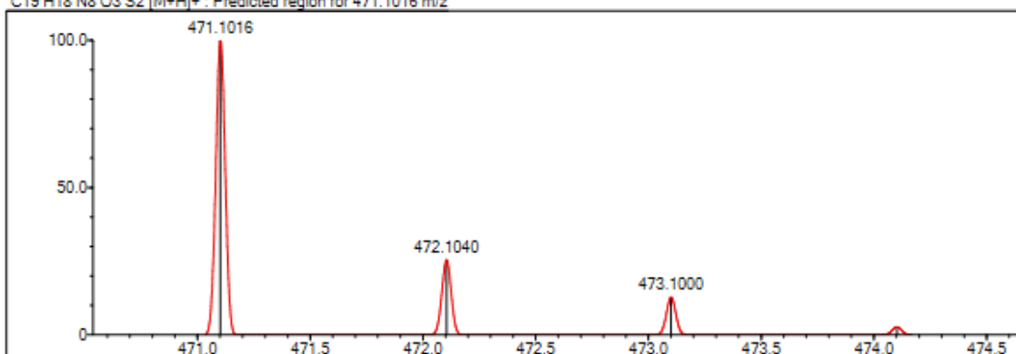
Şekil 5.108. Bileşik 8t'ya ait HRMS spektrumu
