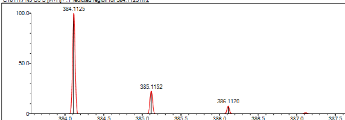
Şekil 5.10 Bileşik 4a'ya ait HRMS spektrumu
