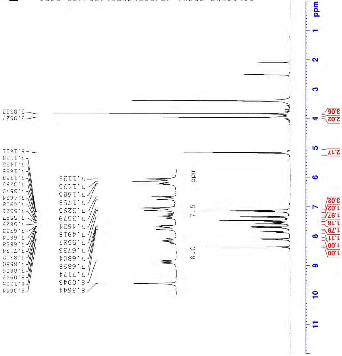
Şekil 5.52. Bileşik 8b'ya ait ^1\text{H} NMR spektrumu
