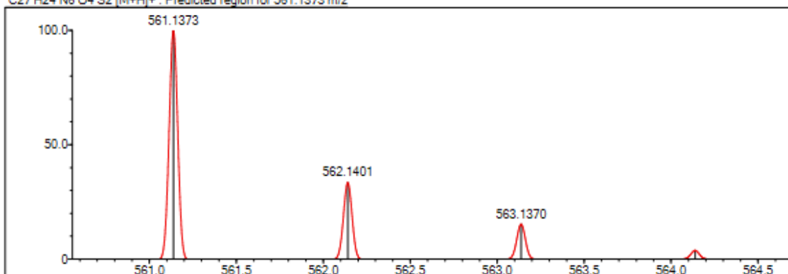
Şekil 5.123. Bileşik 13c'ye ait 1 H NMR spektrumu
