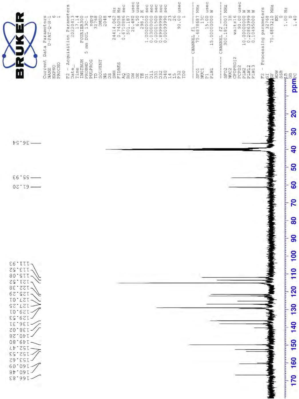
Şekil 5.116. Bileşik 13a'ya ait ^1\text{H} NMR spektrumu
