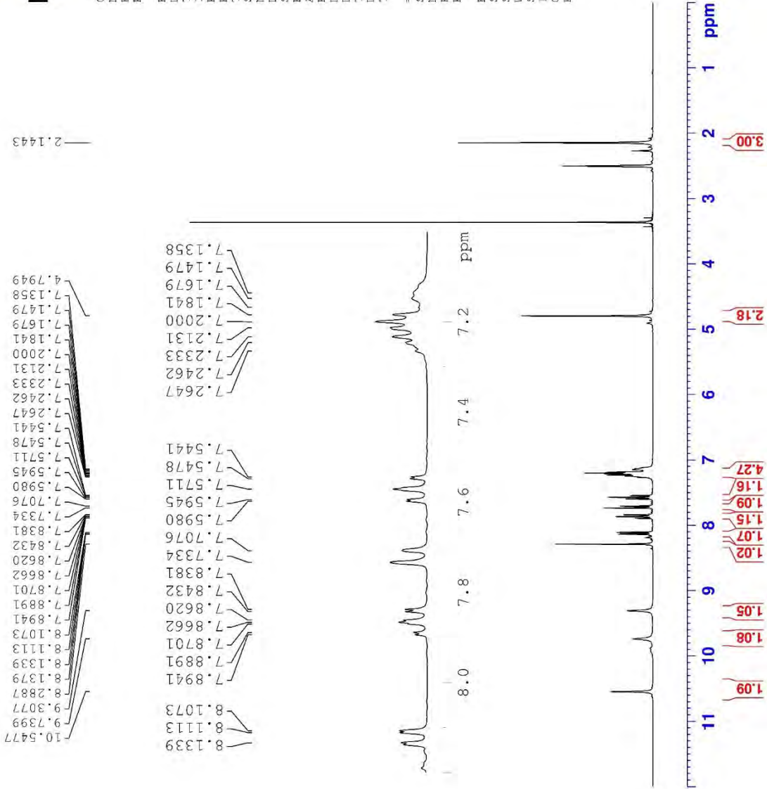
Şekil 5.23. Bileşik 4f'ye ait ^1\text{H} NMR spektrumu
