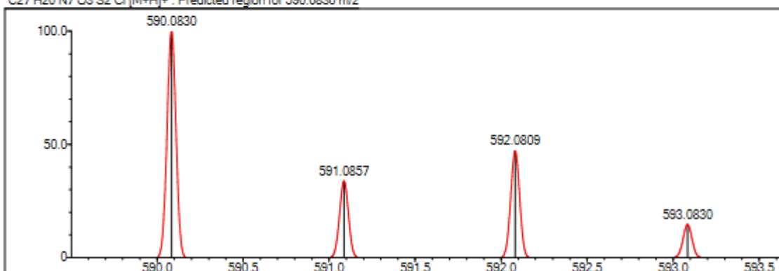
Şekil 5.54. Bileşik 8b'ya ait HRMS spektrumu
