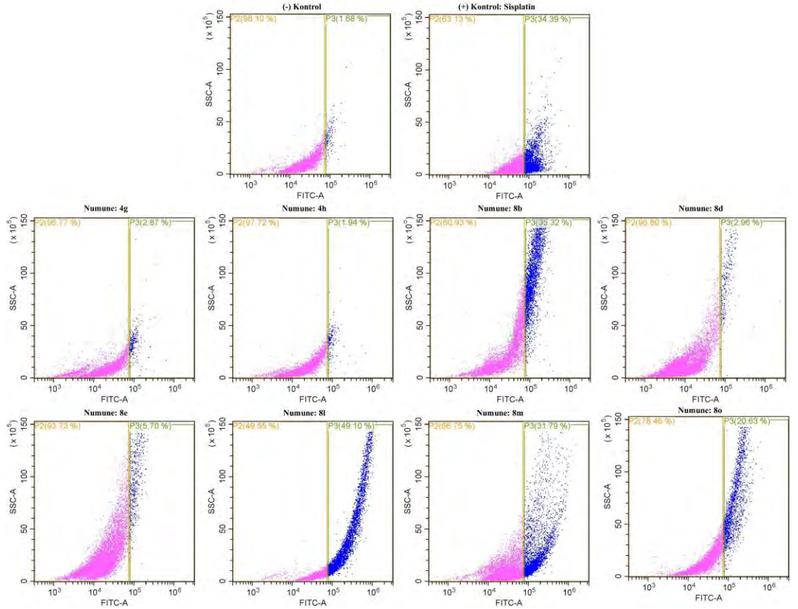
Şekil 5.128. Aktif bileşiklerin ve kontrollerin kaspaz-3 aktivasyon sonuçlarına ait kadrantlar*
