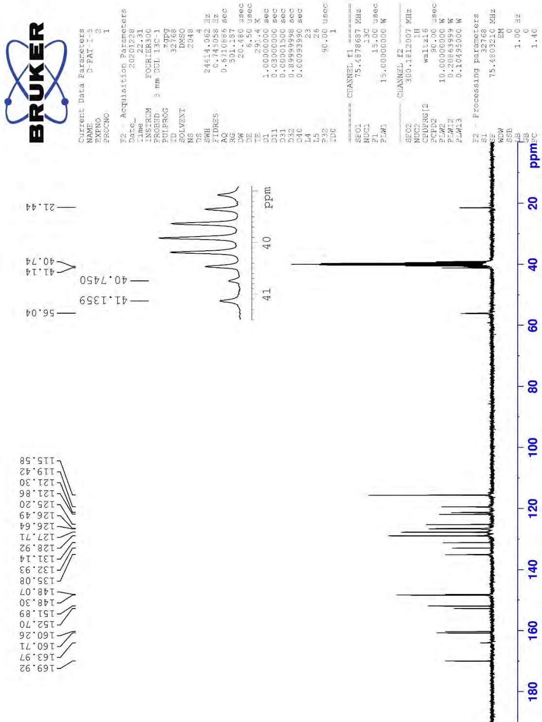
Şekil 5.62. Bileşik 8e'ya ait ^{13}\text{C} NMR spektrumu
