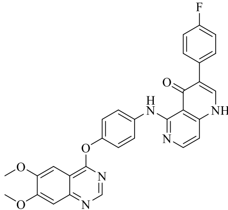
Şekil 2.8. Kinolin ve kinazolin kökenli 1,6-naftiridinon türevlerinden en aktif bulunan analog
