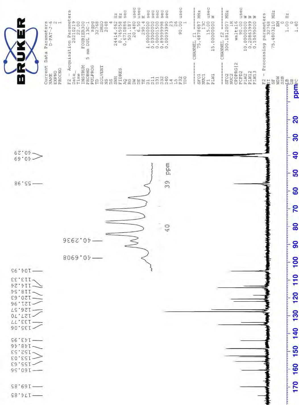
Şekil 5.98. Bileşik 8q'ya ait ^{13}\text{C} NMR spektrumu
