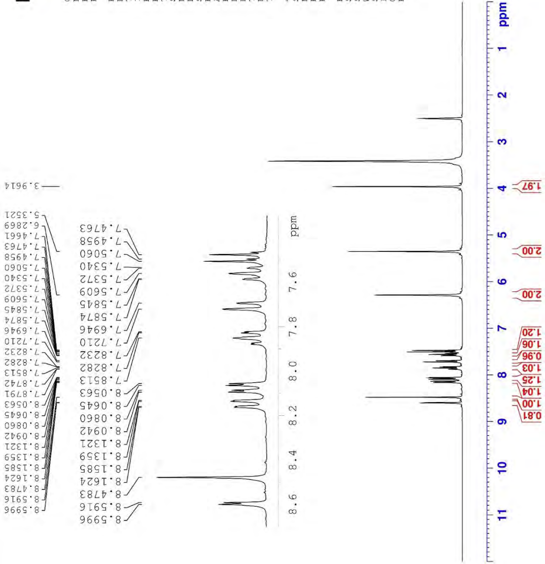
Şekil 5.88. Bileşik 8n'ya ait ^1\text{H} NMR spektrumu
