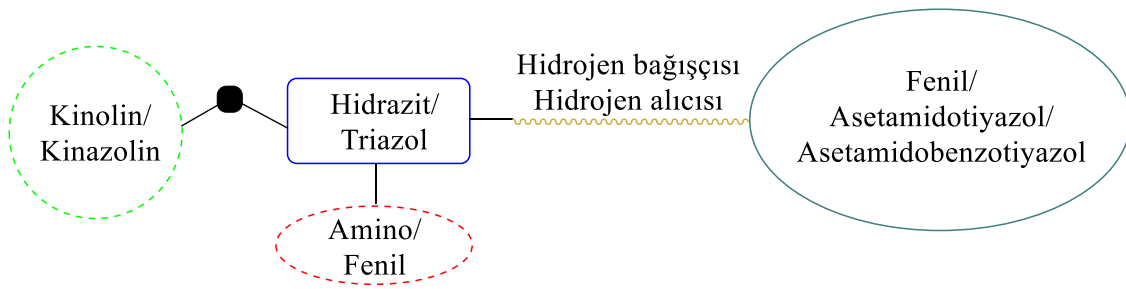
Şekil 5.134. Yapı etki ilişkisine ait diyagramı
