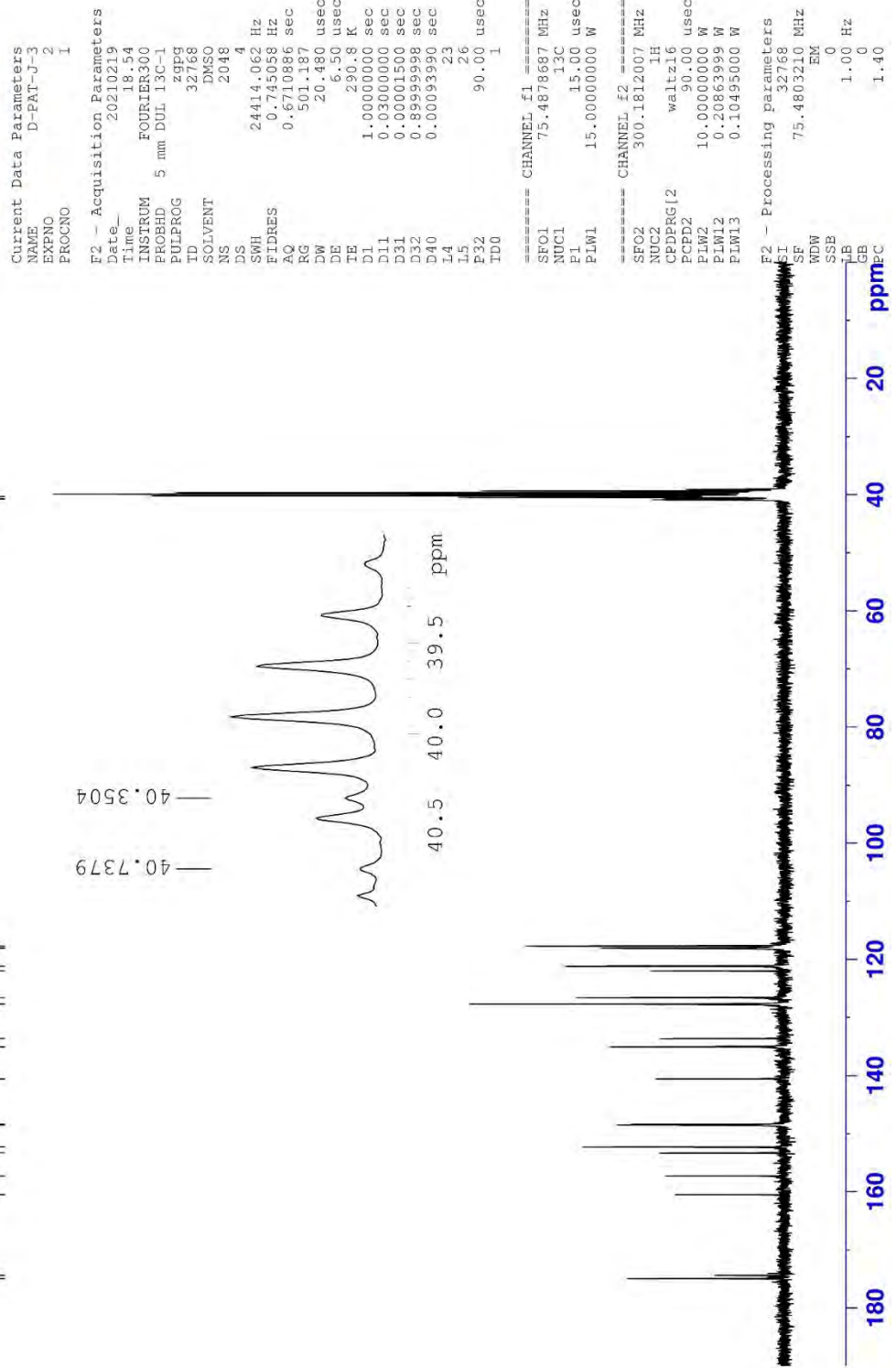
Şekil 5.89. Bileşik 8n'ya ait ^{13}\text{C} NMR spektrumu
