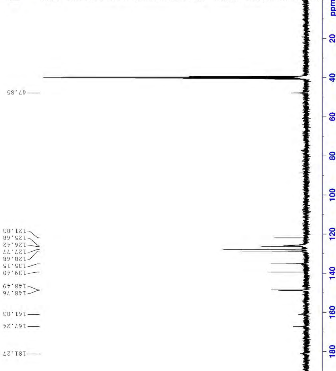
Şekil 5.39. Bileşik 4k'ye ait ^{13}\text{C} NMR spektrumu
