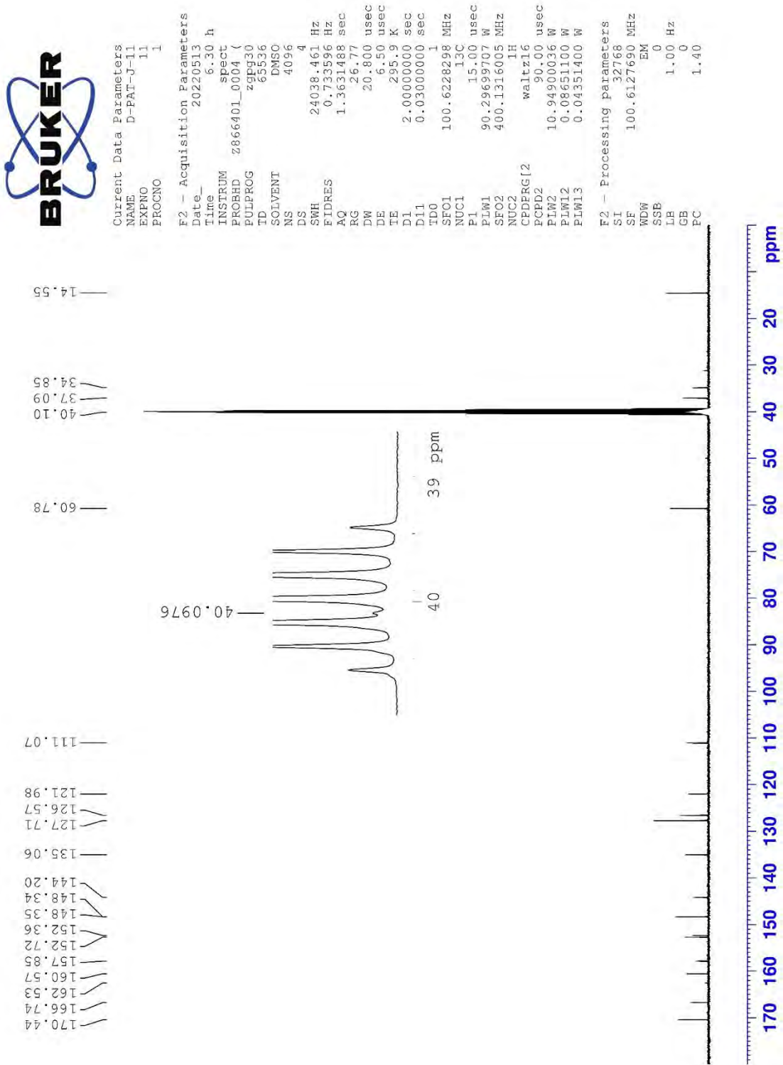
Şekil 5.113. Bileşik 8v'ya ait 13 C NMR spektrumu
