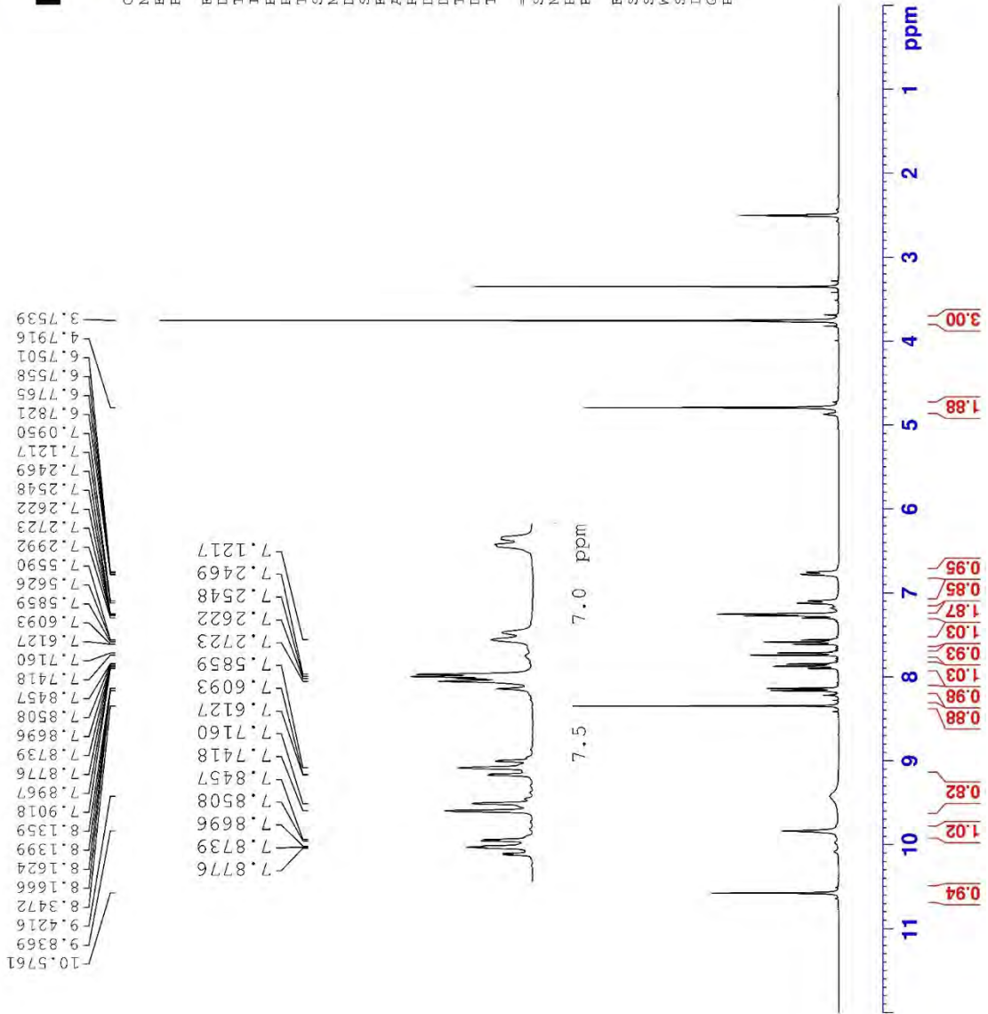
Şekil 5.11. Bileşik 4b'ya ait ^1\text{H} NMR spektrumu
