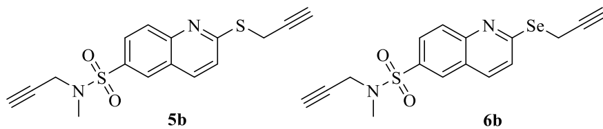
Şekil 2.13. 6-( N -metil- N -allil sülfonamit)-2-(alliltiyoksi/allilselanil)kinolin analogları
