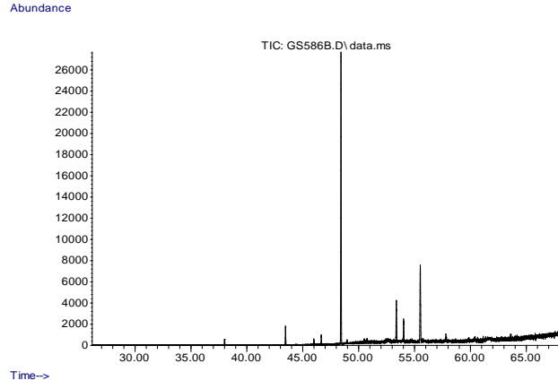
Şekil 4.21. Sumçanka Çeşidi Sap Sabit Yağ Asitleri Metil Ester Kromatogramı
