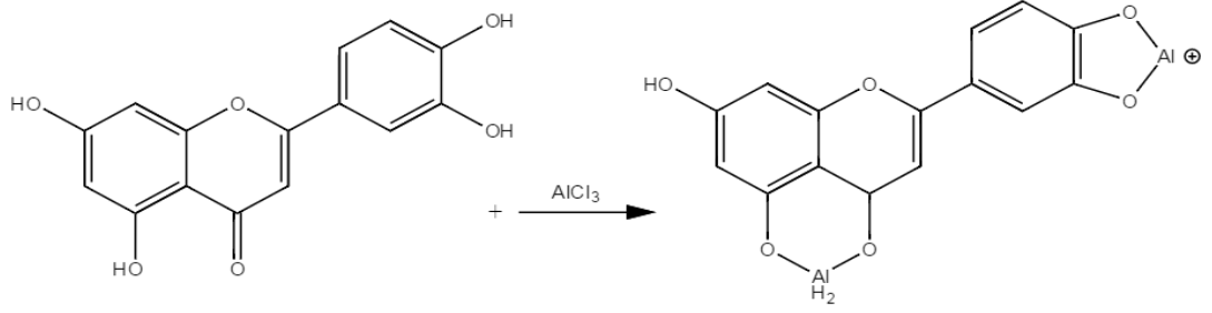
Şekil 2.3. Rutin'in AlCl_3 ile Oluşturduğu Kompleks
