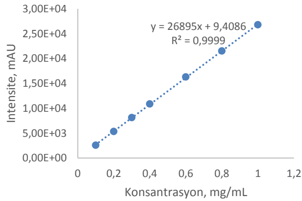
Şekil 5.3. Rutin'in Kalibrasyon Eğrisi
