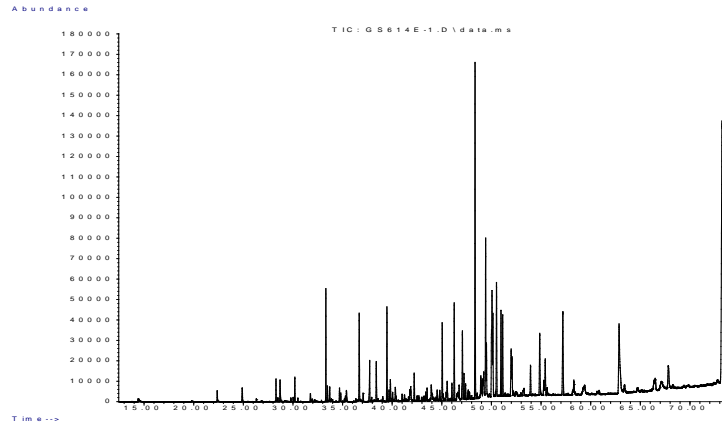
Şekil 4.10. F. esculentum Güneş Çeşidi Kavuzu Uçucu Bileşenlerin Kromatografik Profili (MSD-SPME Yöntemi ile)
