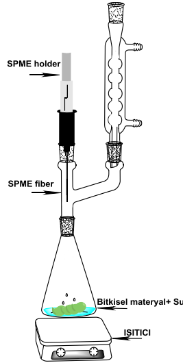
Şekil 3.7. MSD-SPME İşlemi İçin Kullanılan Düzenek
