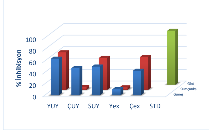
Şekil 5.5. F. esculentum Uçucu Yağ ve Ekstrelerinin Ellman Metodunda AChE İnhibisyonlarının Karşılaştırılması. YUY: Yaprak Uçucu Yağı, ÇUY: Çiçek Uçucu Yağı, SUY: Sap Uçucu Yağı, YEx: Yaprak Ekstresi, ÇEx: Çiçek Ekstresi, GInt: Galantamin.
