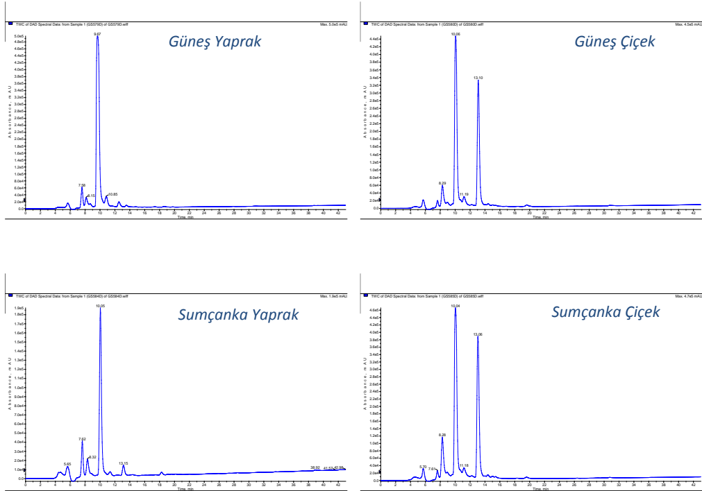
Şekil 4.15. Çeşitlerin Yaprak ve Çiçeklerinin LC-MS Kromatogramları
