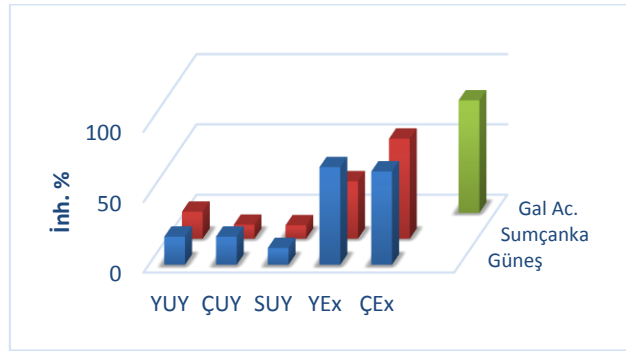
Şekil 5.1. Güneş ve Sumçanka Çeşitlerine Ait DPPH Radikalini Süpürme Etkisi. YUY: Yaprak Uçucu Yağı, ÇUY: Çiçek Uçucu Yağı, SUY: Sap Uçucu Yağı, YEx: Yaprak Ekstresi, ÇEx: Çiçek Ekstresi, Gal.Ac.; Gallik Asit.
