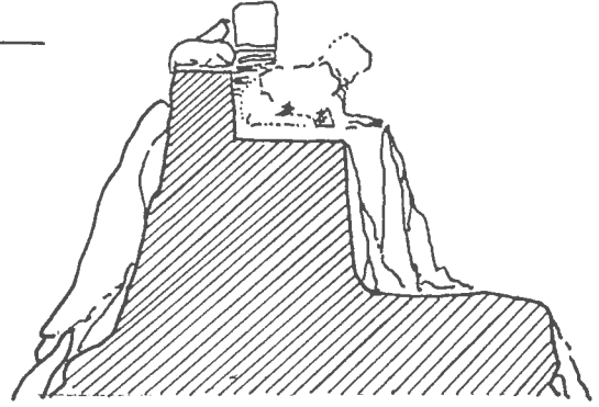
YANDAN GÖRÜNÜŞ
