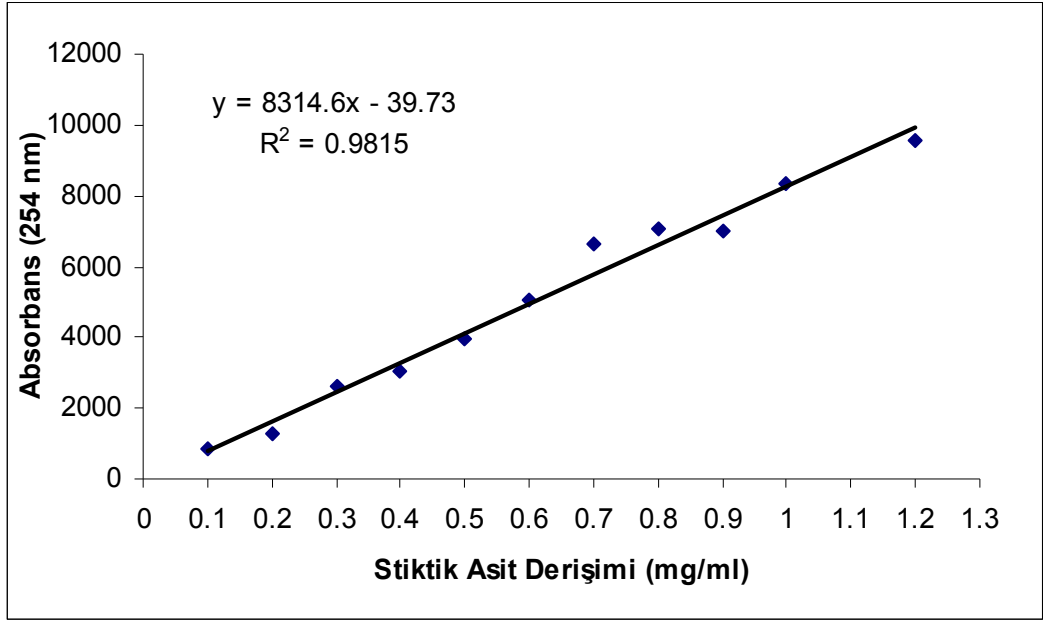
Şekil 3.3. Stiktik asitin kalibrasyon grafiğı
