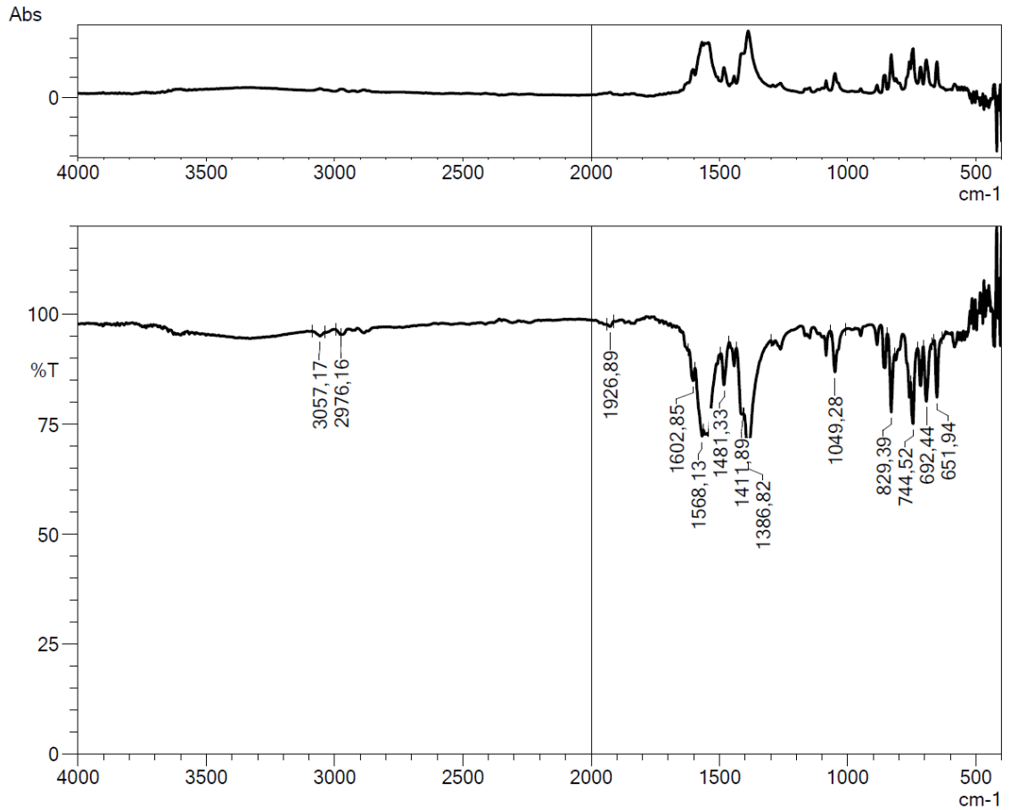
Şekil 5.9. Bileşik A5'e ait IR spektrumu
