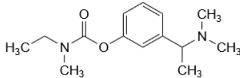
Şekil 2.11. Rivastigmin bileşiği
