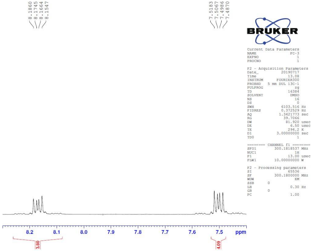
Şekil 5.7. Bileşik A3'e ait NMR spektrumları
