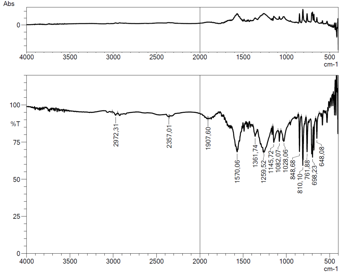
Şekil 5.8. Bileşik A4'e ait IR spektrumu
