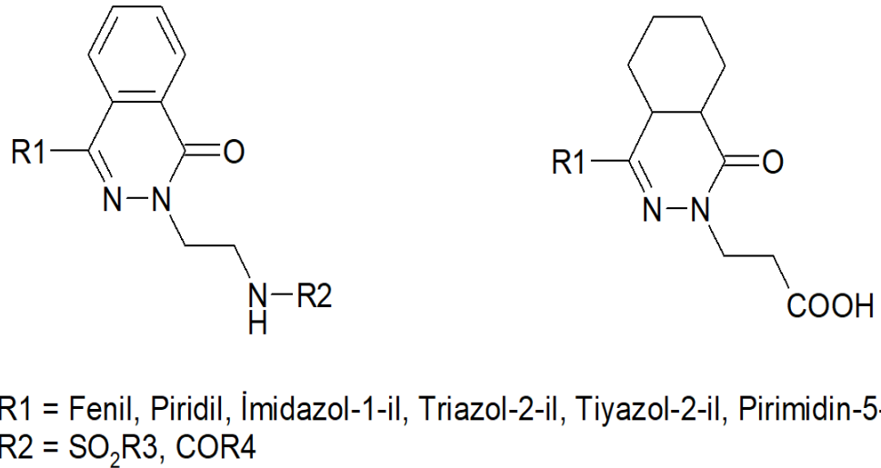
Şekil 2.24. Çalışmalar sonucu elde edilen farklı sübstitüsyonlar içeren ftalazinon türevleri
