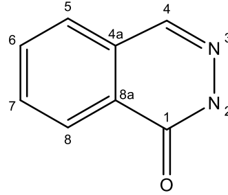
Şekil 2.15. 1(2H)-Ftalazinon Numaralandırması
