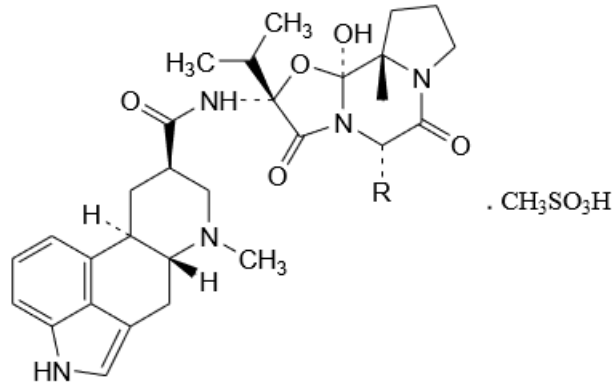
Şekil 2.3. Kodergokrin bileşiği
