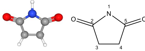
Şekil 2.29. Pirolidin-2,5-dion halkası numaralandırması, 2D ve 3D görüntüsü
