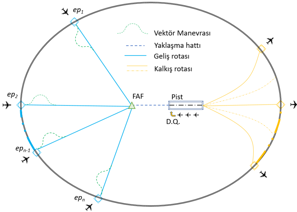
Şekil 3.1. Jenerik bir terminal manevra sahası (TMA) konfigürasyonu
