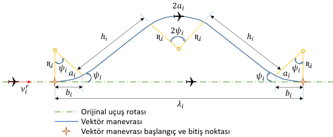
Şekil 3.5. Vektör manevrası
