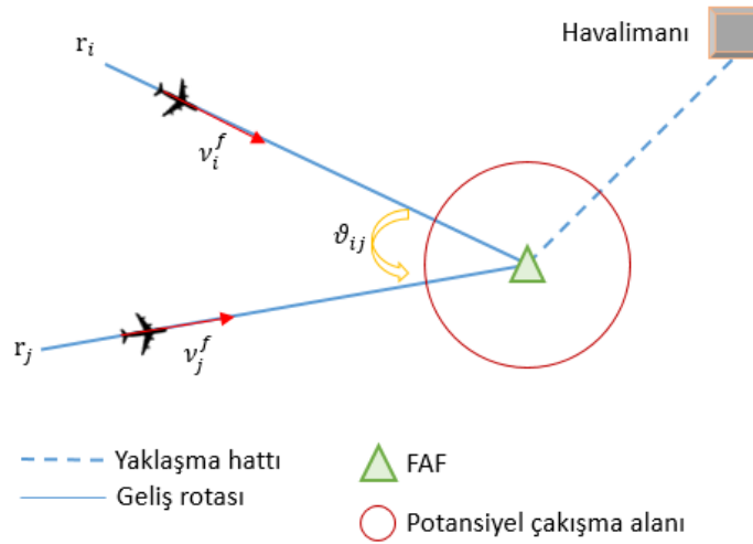
Şekil 3.4. Kesişen rotaların geometrisi
