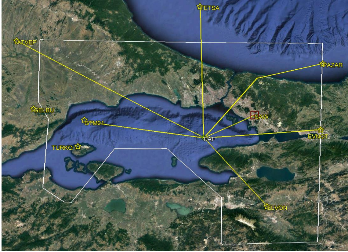
Şekil 3.7. İstanbul TMA ve Sabiha Gökçen Havalimanı(LTFJ) harita görünümü [43]
