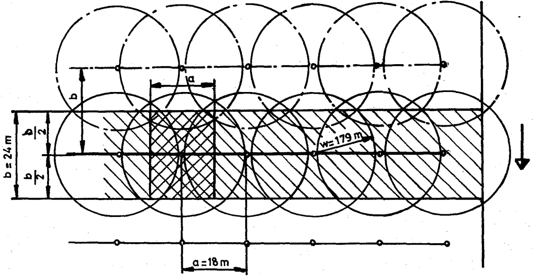
Şekil 3.11. Dörtgen bağlantı sisteminde yağmurlama alanı (Karmeli,1987)
