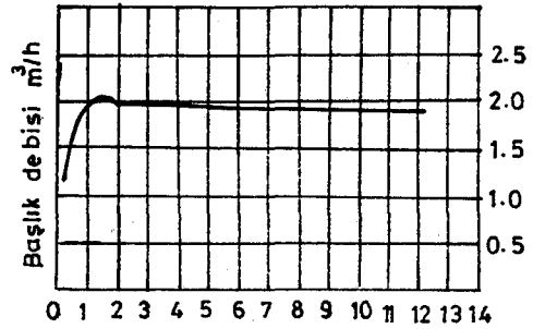
Bir basınç dengeleyicisi işletme eğrisi
