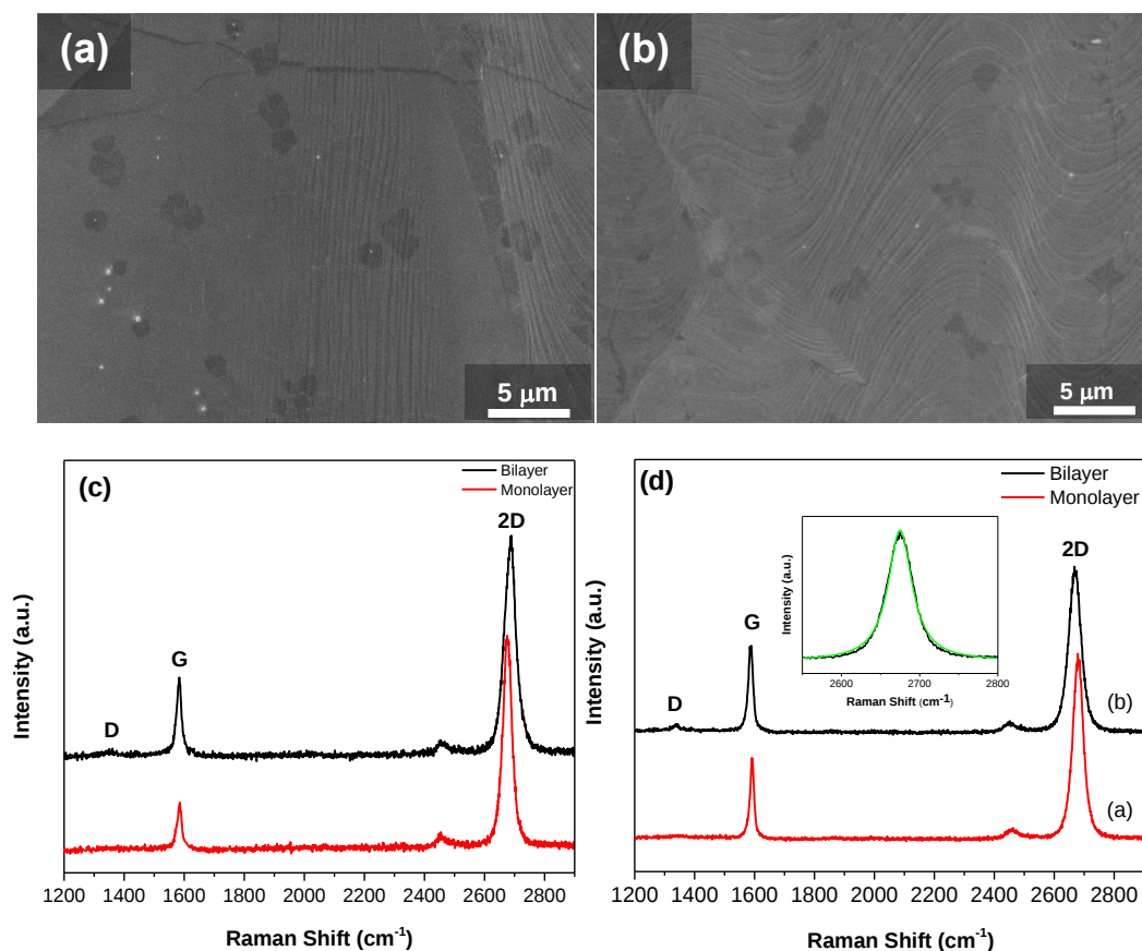
Figure A.8. Images MEB-FEG de graphène synthétisé sur les feuilles de cuivre B1 (a) et B2 (b) . La feuille B1 été nettoyée par de l'acide acétique pendant 10 minutes puis soumise à une CVD mettant en œuvre 200 sccm d'Ar seul au départ Ar puis un mélange de 100 sccm H 2 /20 sccm CH 4 pendant la croissance du graphène pour une durée de 5 min et une pression de 0,5 torr pendant tout le processus. La feuille de cuivre B2 a été nettoyée par de l'acide nitrique pendant 1 min puis soumise à une CVD mettant en œuvre 200 sccm Ar/100 sccm H 2 au départ, puis 100 sccm H 2 /17 sccm de CH 4 pendant la croissance du graphène, et 0,3 torr et 0,2 torr pendant les étapes de réduction puis de recuit. (c), (d) Spectres Raman correspondant aux échantillons montrés en (a) et (b), enregistrés à différents emplacements.
