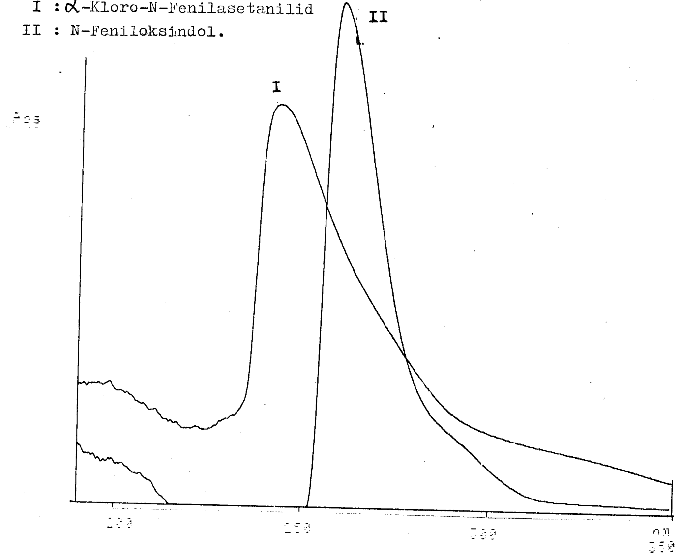
Şekil 2.11 \alpha -Kloro-N-Fenilasetanilid'in halka kapanmasının U.V. spektrumu
