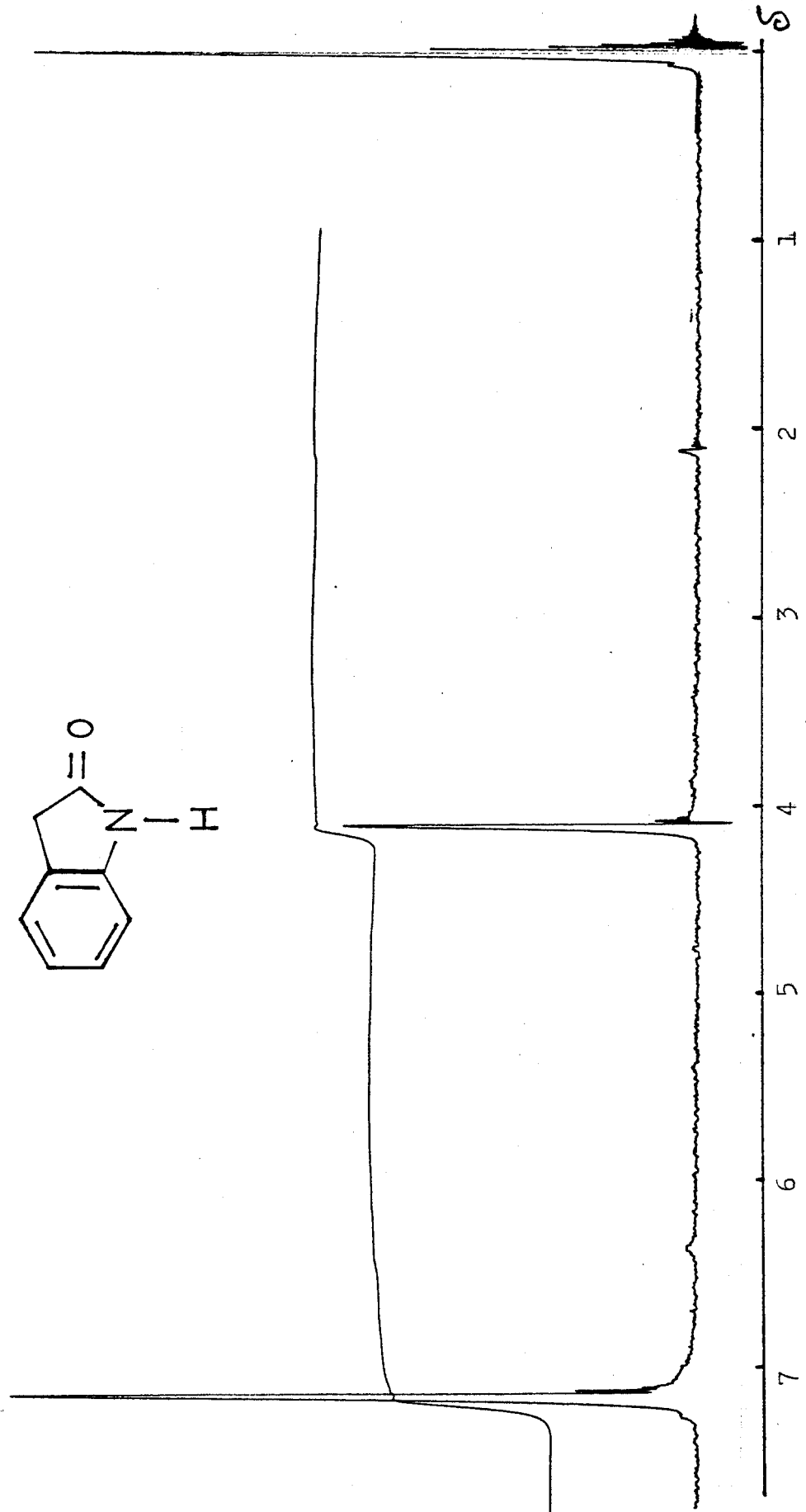
Şekil 2.10 Oksindolün N.M.R. spektrumu (CF 3 COOH içinde).
