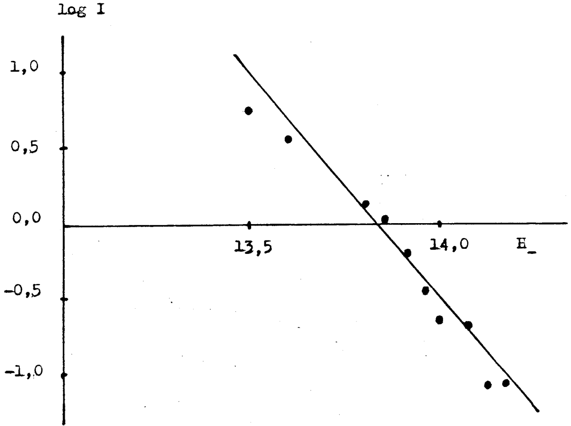
Şekil 2. 21 Oksindol'un proton verme sabitinin saptanması.
