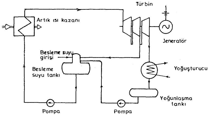
Şekil 3.4. Döner fırın gazının by-pass edilmesiyle elektrik enerjisi üretimi (Mohrenstecher'den, 1986)
