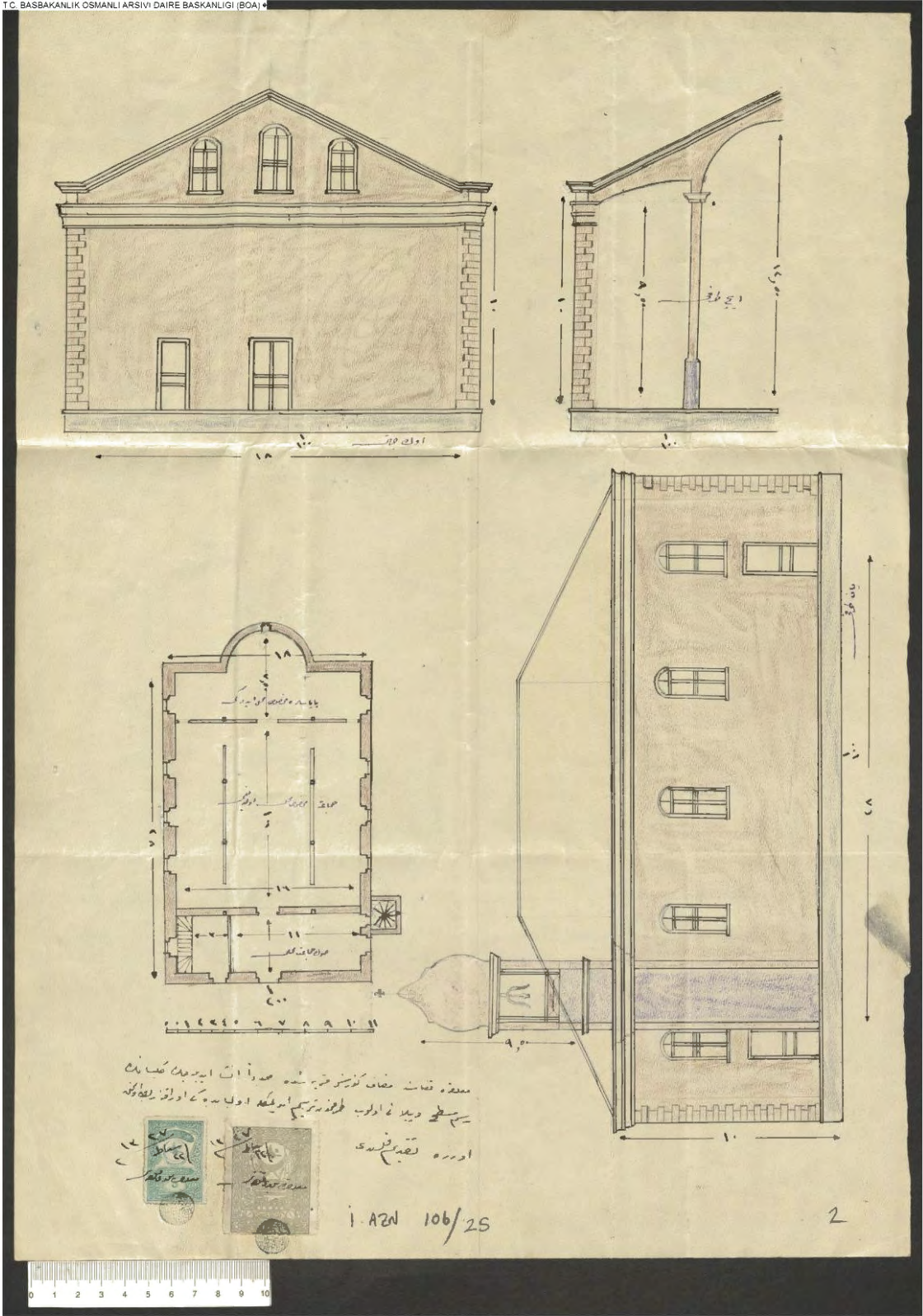
Belge 32: Malkara Gözsüz Köyü'nde harap durumda bulunan Rum Kilisesi'nin Proje Çizimleri (BOA, İ.AZN.106-25, H.15.06.1330/M.01.06.1912)
