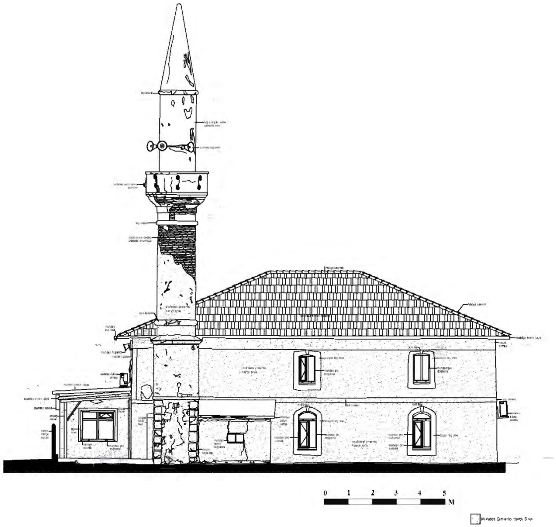
Çizim 74: Saray Büyükyoncalı Aziziye Camii Güneybatı Cephe Rölöve (İbrahim Uran Badur'dan)
