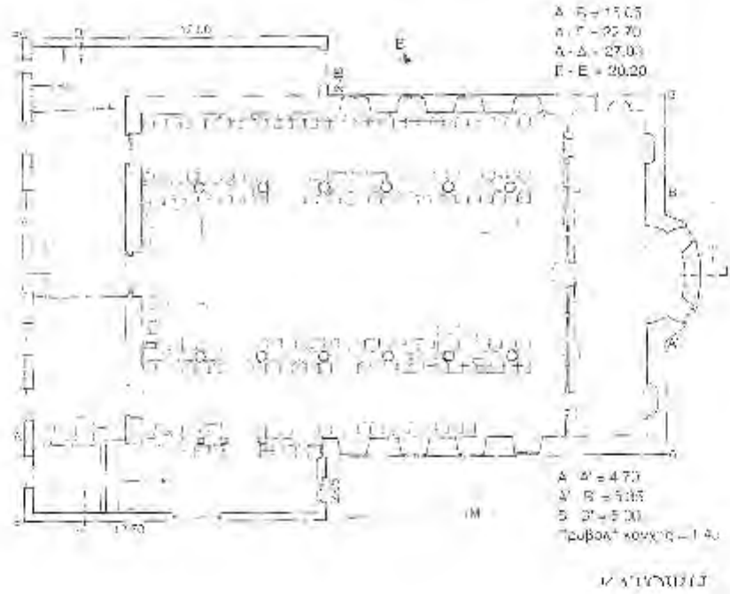
Çizim 131: Dimetoka Agios Athanasios (Άγιος Αθανάσιος) Kilisesi Zemin Kat Planı (Theodoros Kyrkudis'ten)
