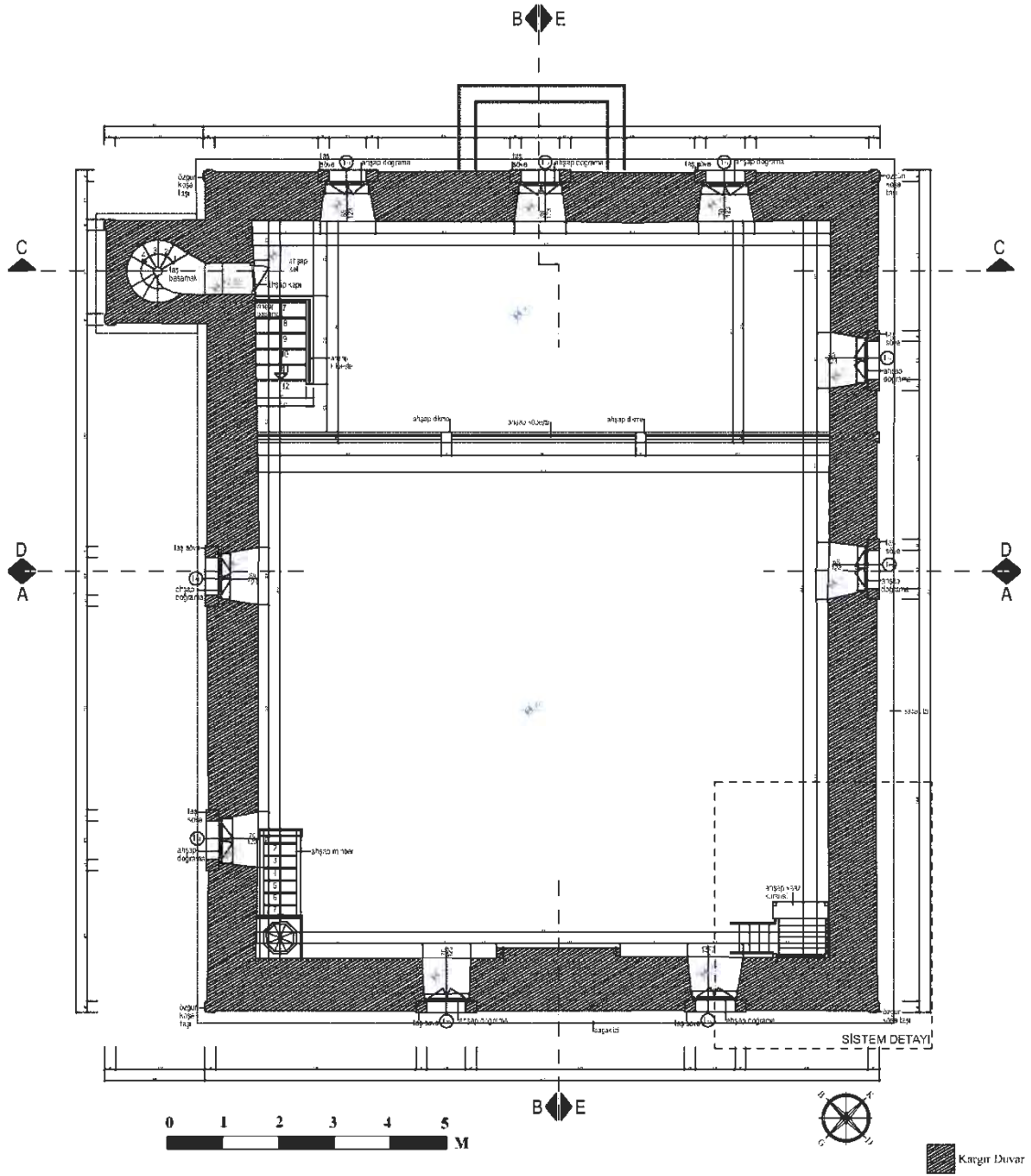
Çizim 76: Saray Büyükyoncalı Aziziye Camii Asma Kat Planı Restorasyon (İbrahim Uran Badur'dan)
