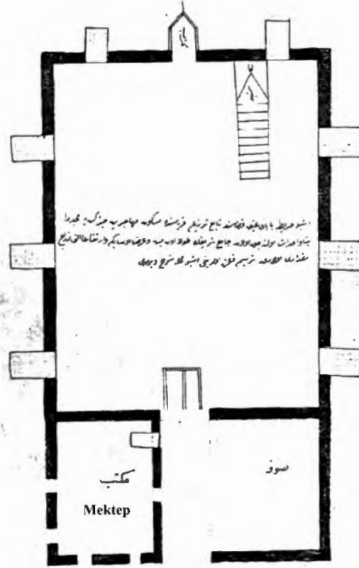
Çizim 2: Terzili Köyü Zemin Kat Planı (F. Kocacık'dan)
