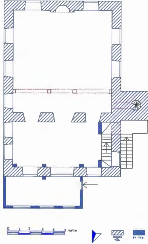
Çizim 5: Edirne Havsa Yolageldi Köyü Zemin Kat Planı (Halil İbrahim Eryılmaz'dan)
