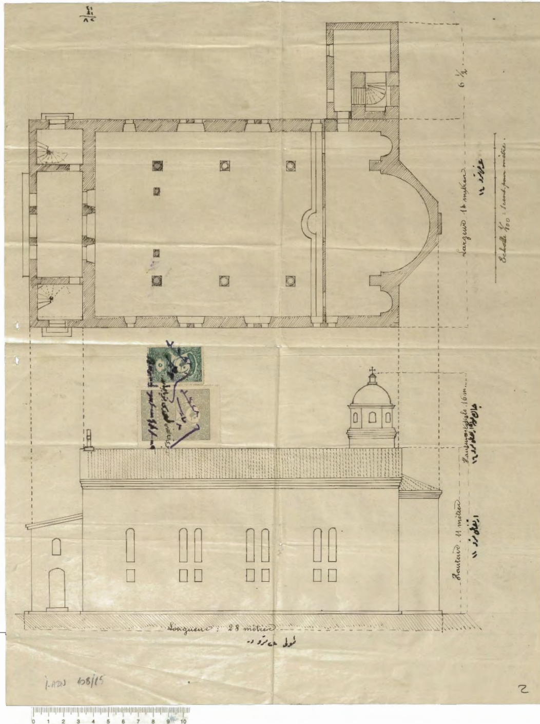
Belge 28: Malkara'nın Yukarı Rum Mahallesi Katolikleri İçin Yapılacak Kargir Kilisenin Çizimleri (BOA, İ.AZN. 108-15, H.05.11.1330/M.16.10.1912)
