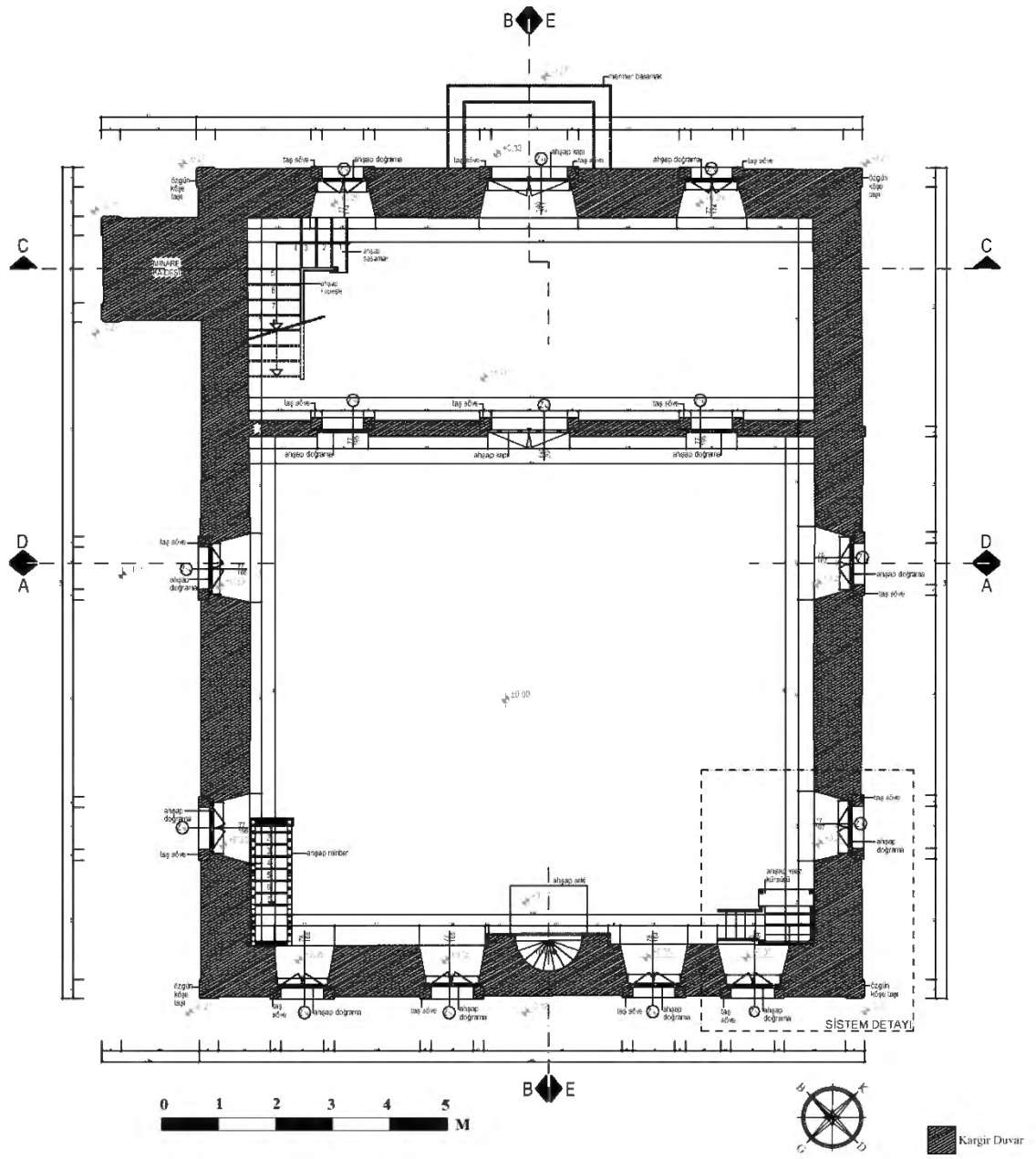
Çizim 75: Saray Büyükyoncalı Aziziye Camii Zemin Kat Planı Restorasyon (İbrahim Uran Badur'dan)
