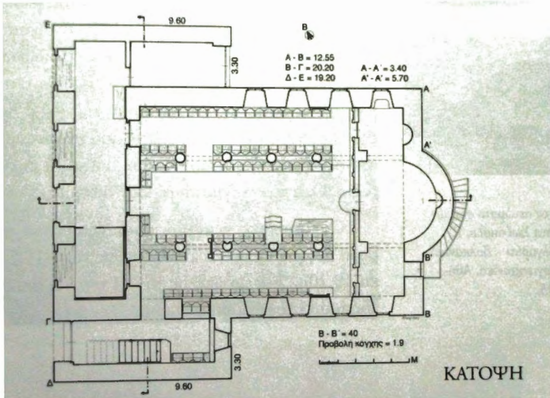
Çizim 133: Dimetoka Sotiros Hristou (Σωτήρος Χριστού) Kilisesi Zemin Kat Planı (Yılmaz Büktel'den)
