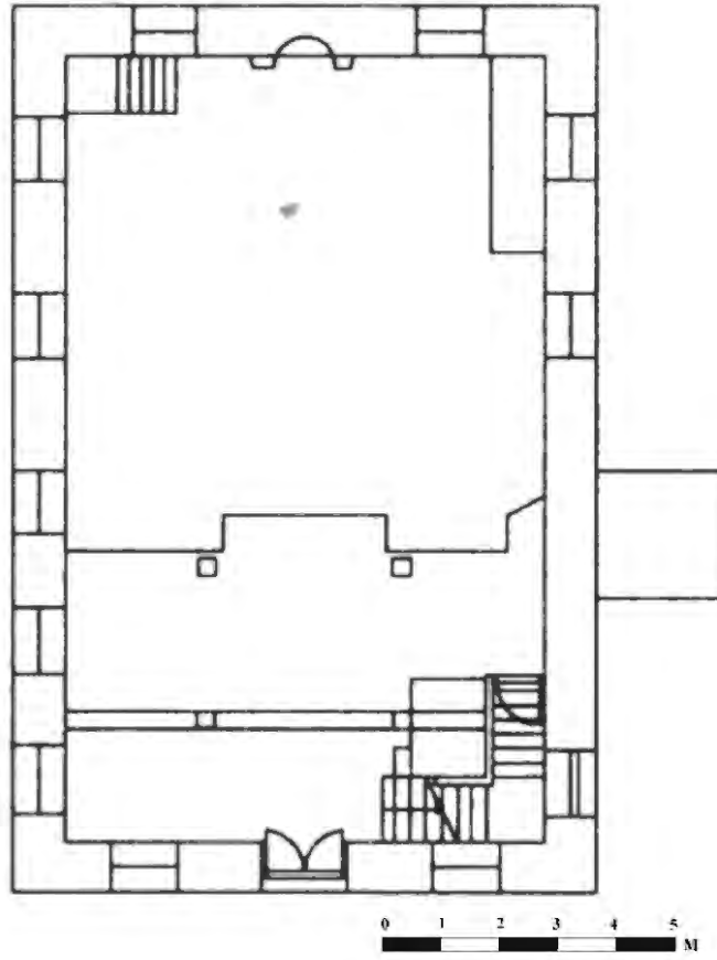
Çizim 7: Silivri Alipaşa Mahallesi Camii Zemin Kat Planı (Sezgi Giray Küçük'ten)
