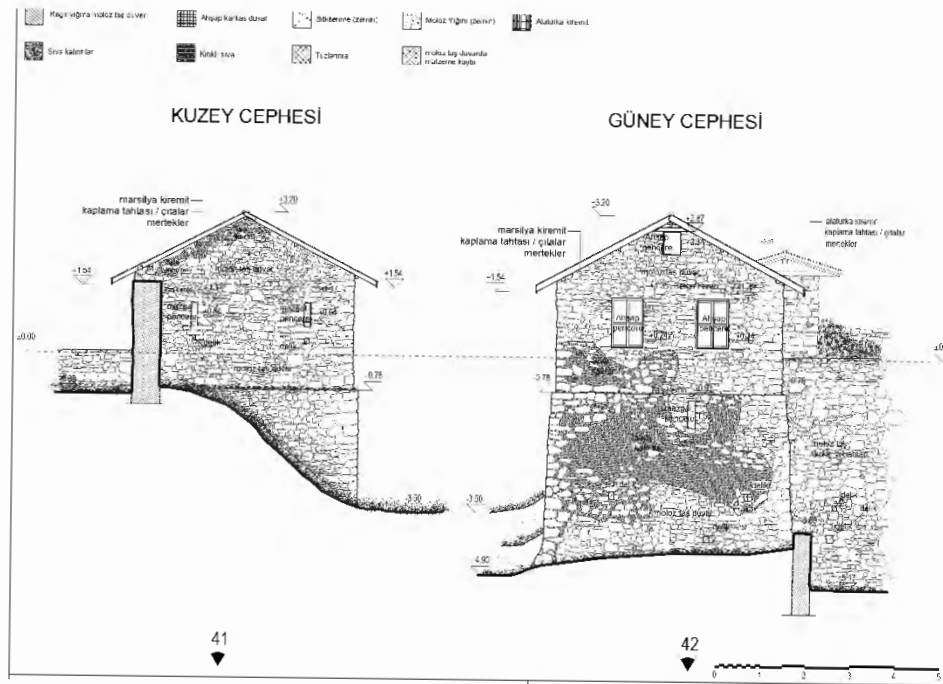
Çizim 124: Hoşköy Ioannis Theologos Manastırı Yetimhane Kuzey ve Güney Cepheleri Rölöve (Arşimet İnşaat)
