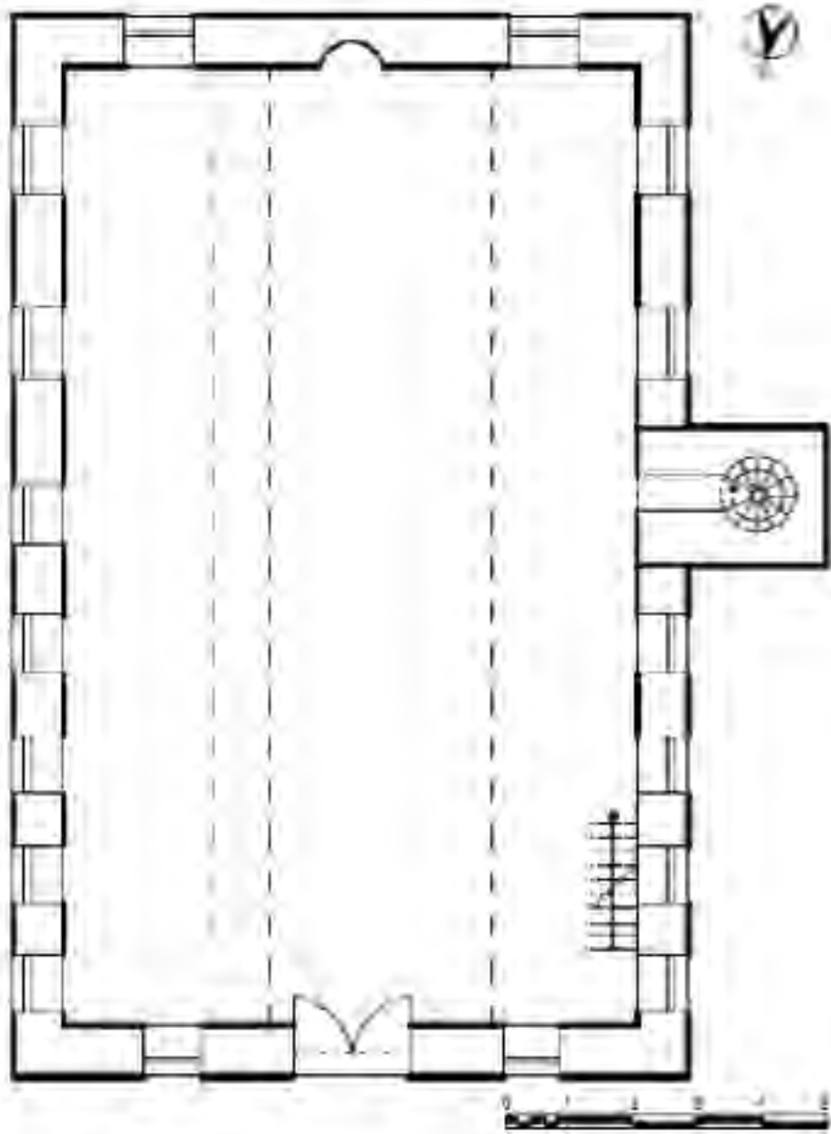
Çizim 41: Günümüze Ulaşmayan İpsala Aliço Pehlivan Köyü Camii Zemin Kat Planı (Murat Karademir'den)
