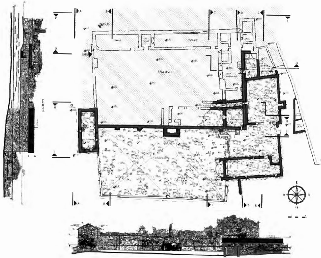
Çizim 123: Hoşköy Ioannis Theologos Manastırı Zemin Kat Planı Rölöve (Arşimet İnşaat)
