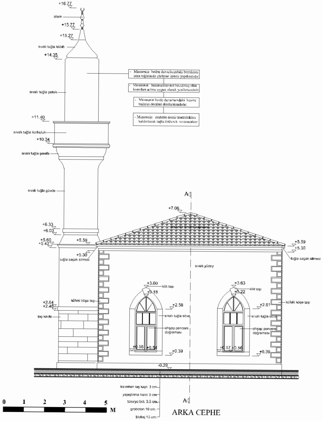
Çizim 19: Tekirdağ Saray Kurtdere Camii Güneydoğu Cephe Restorasyon (İbrahim Uran Badur'dan)
