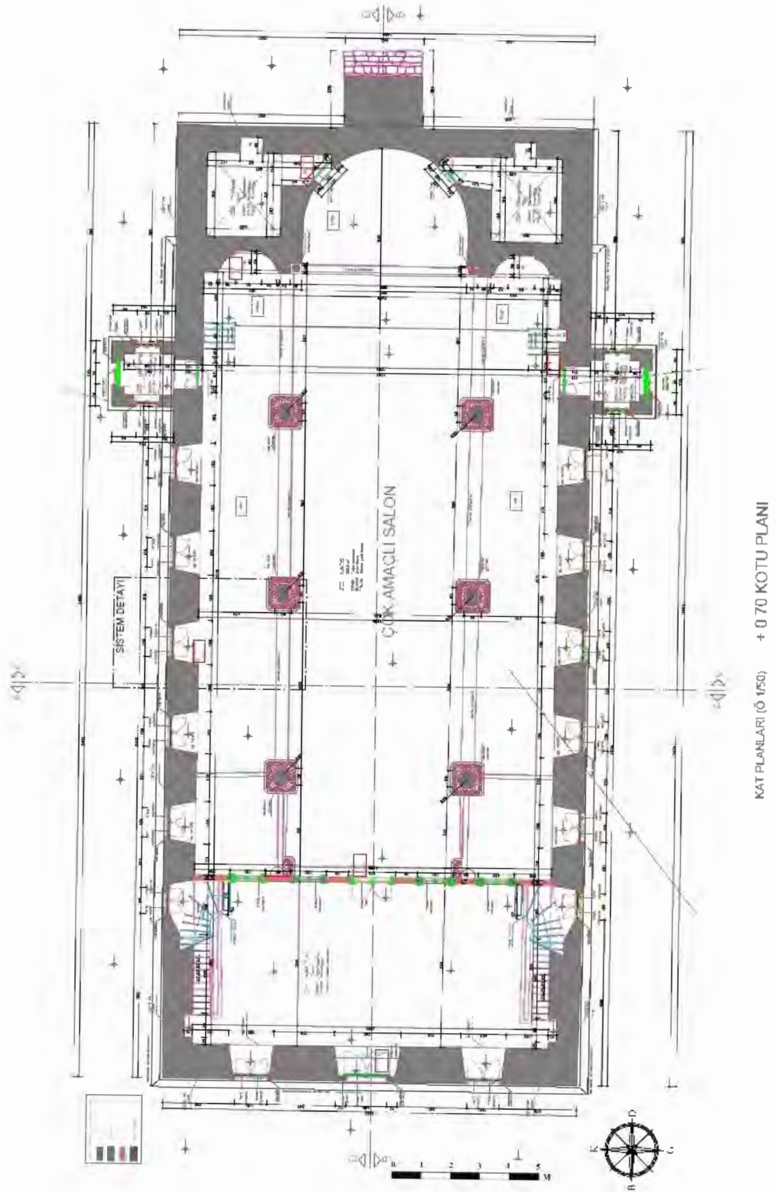
Çizim 95: Malkara Surp Toros Kilisesi Zemin Kat Planı Restorasyon (Taksim Yapı Mimarlık)
