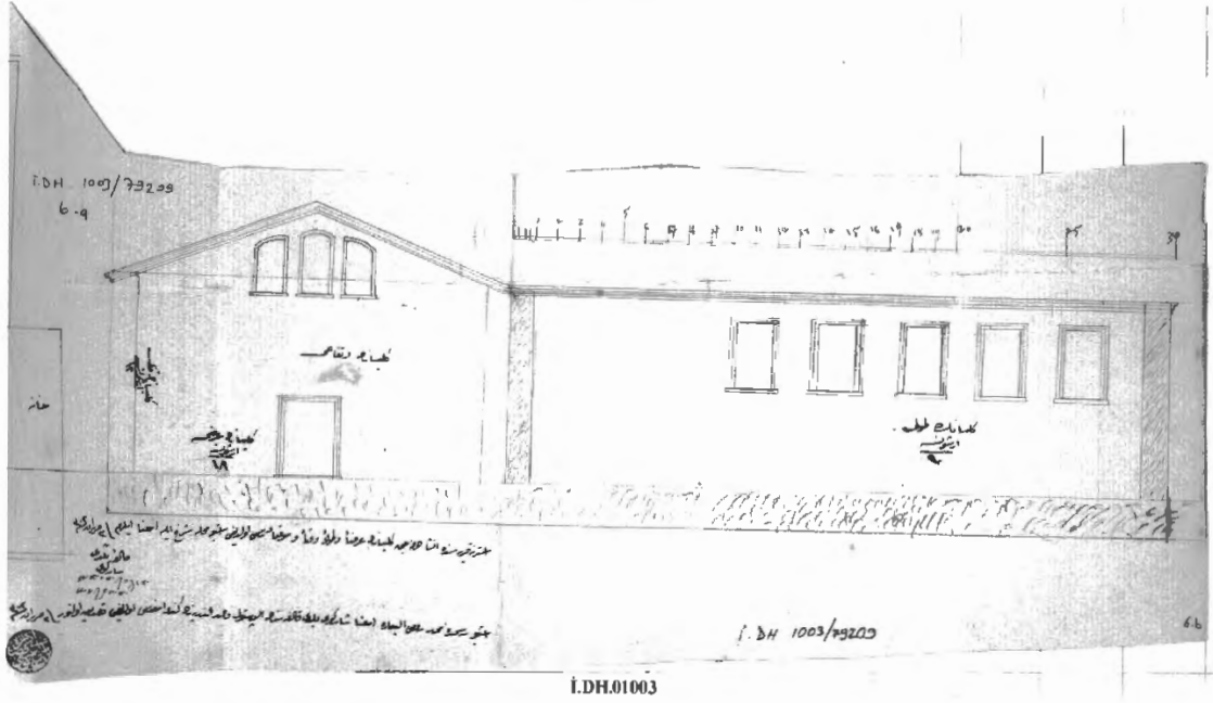
Belge 14: Gelibolu Sancağı Dahilinde Şarköy Kazasına Bağlı İsterir (Sterna) Karyesinde İnşa Edilecek Rum Kilisesinin Proje Çizimleri (BOA, İ.DH..1003-79209, H.20.12.1303/M.19.09.1886)
