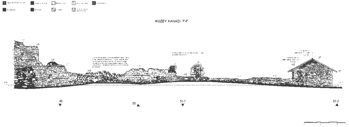
Çizim 125: Hoskoy Ioannis Theologos Manastırı Kuzey Cephe Rölöve (Arşimet İnşaat)
