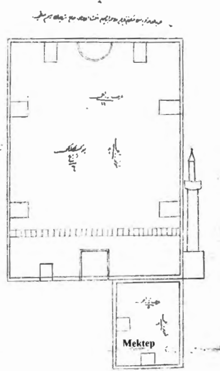
Çizim 4: Arab Hoca Köyü Zemin Kat Planı (F. Kocacık''dan)
