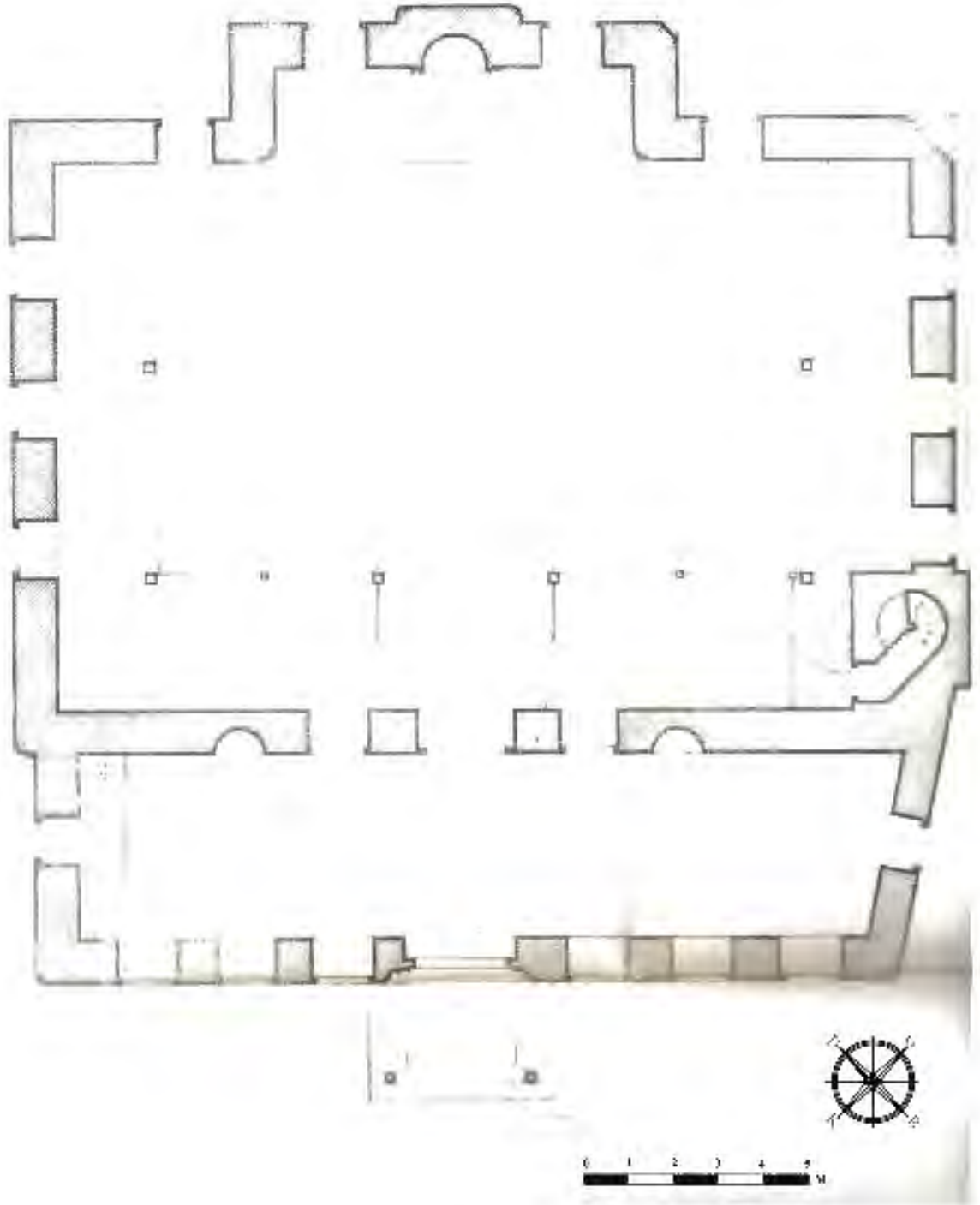
Çizim 42: Tekirdağ Süleymanpaşa Eski Camii Zemin Kat Planı (Mehmet Tuncel'den)
