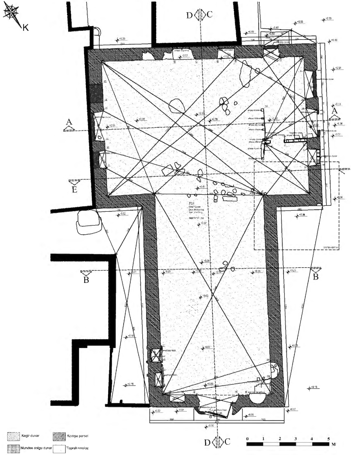
Çizim 111: Şarköy Eriklice Aziz Theotokos Rum Kilisesi Zemin Kat Planı Rölöve (Pasa Mimarlık)
