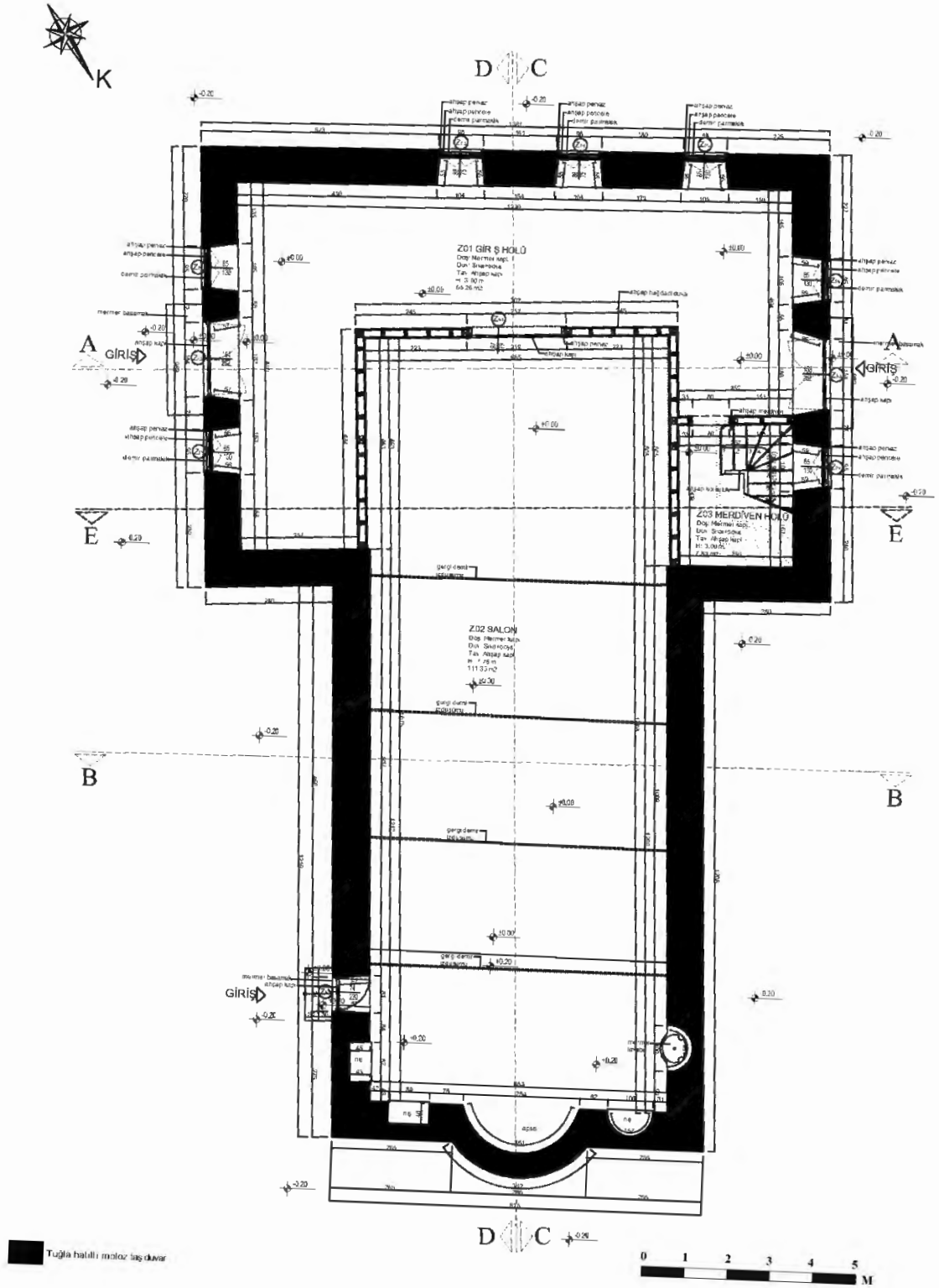
Çizim 117: Şarköy Eriklice Aziz Theotokos Rum Kilisesi Zemin Kat Planı Restorasyon (Pasa Mimarlık)
