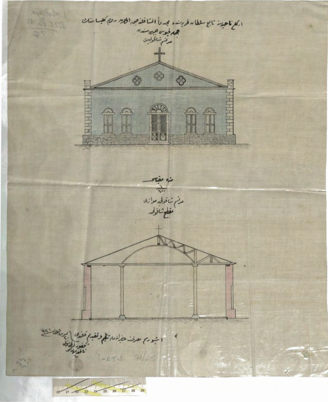
Belge 40: Ereğli Sultan (Sultanköy) Köyü'nde Kilise İnşasına Dair Cephe ve Kesit Çizimi (BOA, İ.AZN.71-25, H.11.03.1325/M.24.04.1907
