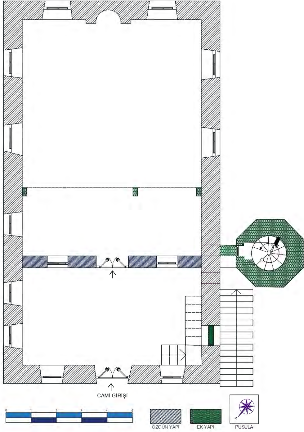
YANIKAĞIL CAMİSİ ZEMİN KAT PLANI
