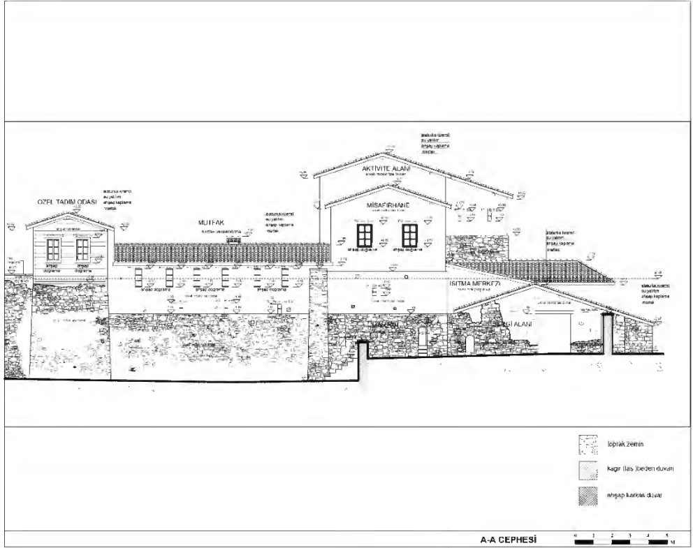
Çizim 129: Hoşköy Ioannis Theologos Manastırı Doğu Cephe Restorasyon (Arşimet İnşaat)
