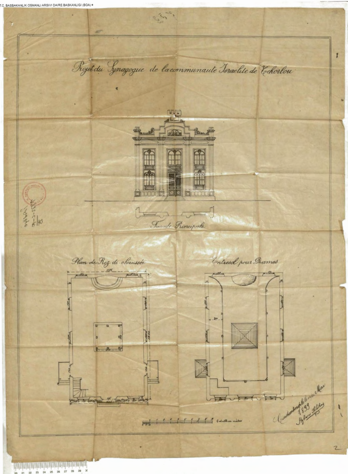
Belge 11: Çorlu 'da Yeniden İnşa Edilecek Havranın Proje Çizimleri (BOA, İ..AZN. 57-15, H.10.06.1322/M.22.08.1904)
