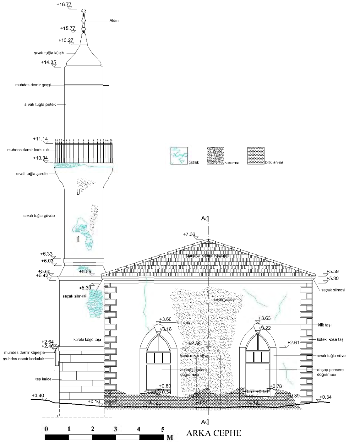
Çizim 13: Tekirdağ Saray Kurtdere Camii Güneydoğu Cephe Rölöve (İbrahim Uran Badur'dan)
