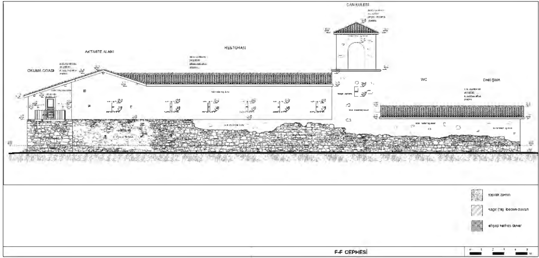
Çizim 130: Hoşköy Ioannis Theologos Manastırı Batı Cephe Restorasyon (Arşimet İnşaat)
