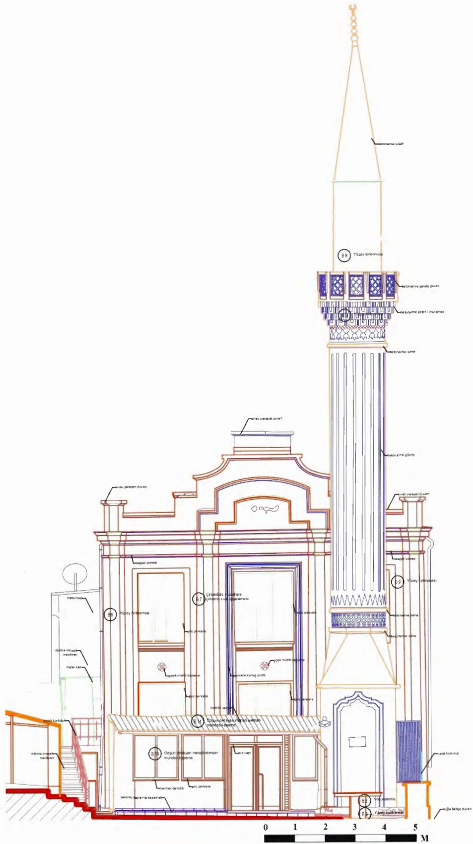
Çizim 84: Tekirdağ Çorlu Sinagogu (Yeni Camii) Kuzeybatı Cephe Rölöve (SM Restorasyon)
