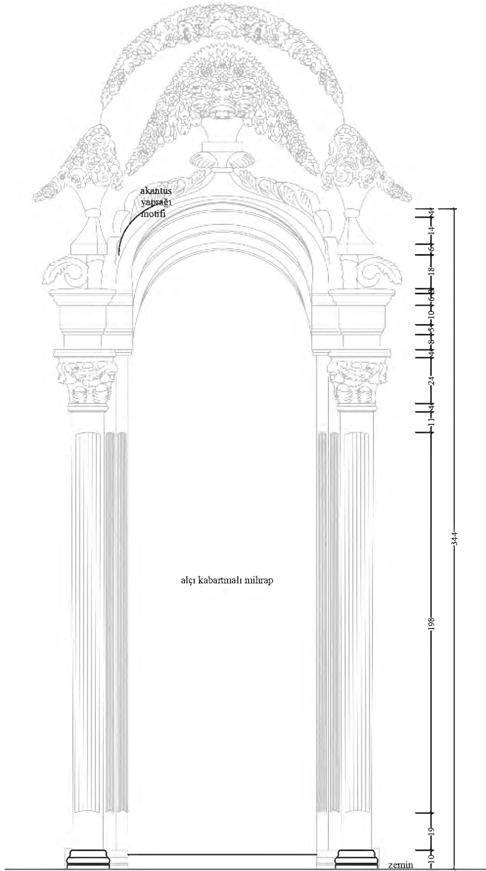
Çizim 55: Tekirdağ Süleymanpaşa Orta Camii Mihrap Detayı (Ani Mimarlık)
