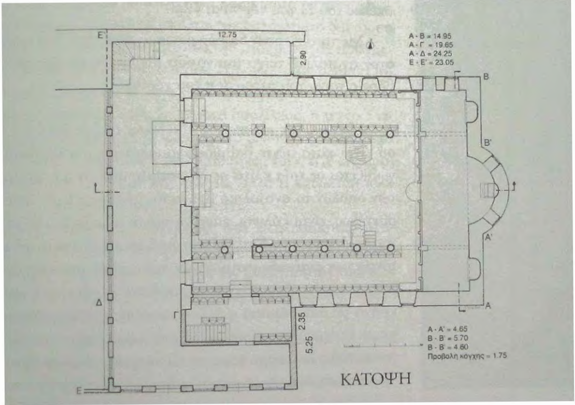
Çizim 134: Sofulu Agios Athanasios (Άγιος Αθανάσιος) Kilisesi Zemin Kat Planı (Yılmaz Büktel'den)
