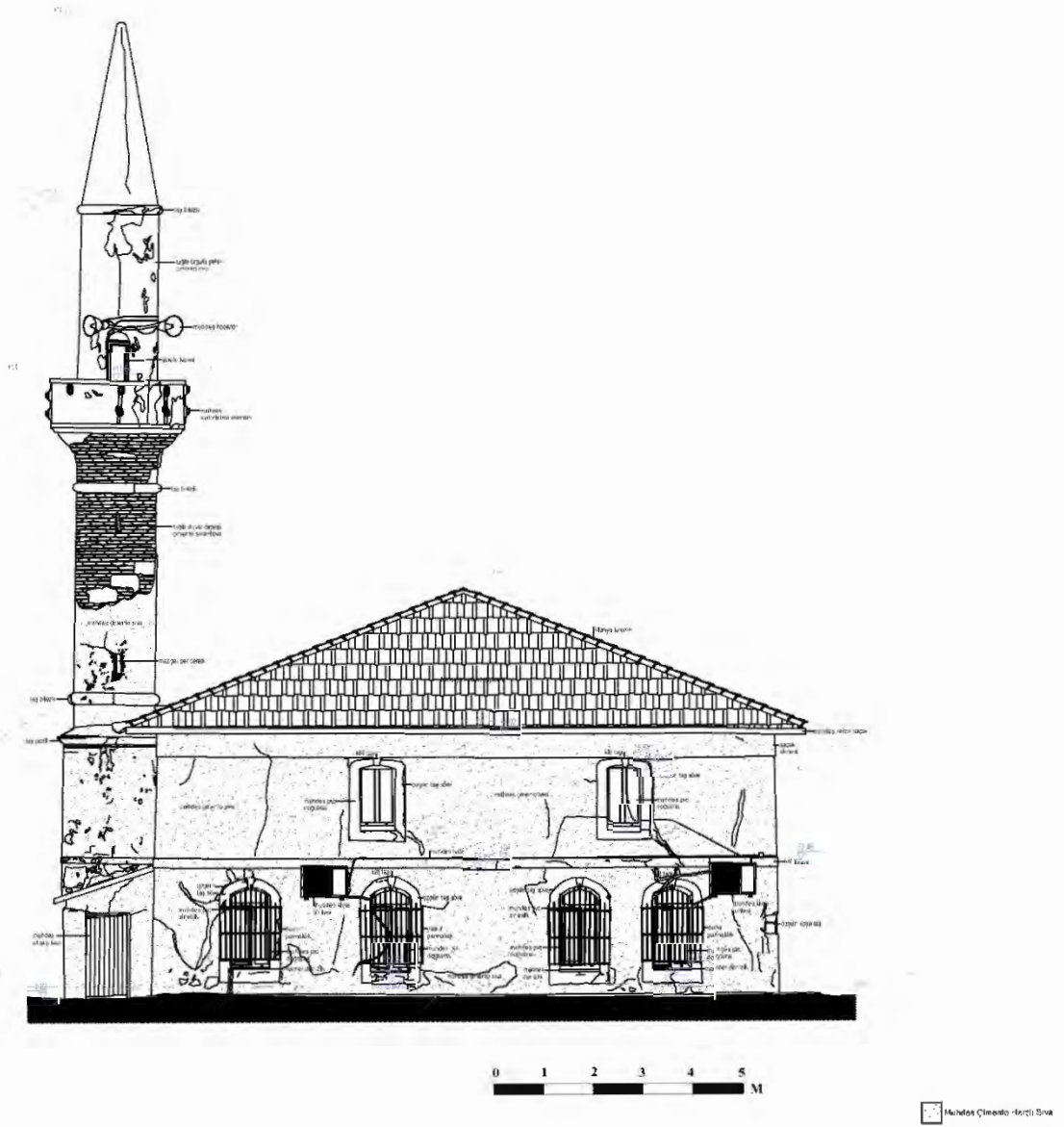
Çizim 73: Saray Büyükyoncalı Aziziye Camii Güneydoğu Cephe Rölöve (İbrahim Uran Badur'dan)
