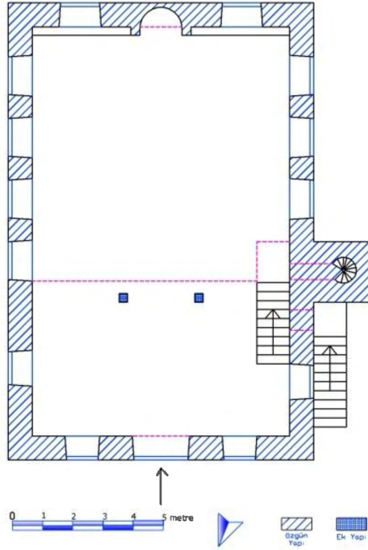
Çizim 6: Kırklareli Babaeski Ağayeri Camii Zemin Kat Planı (Halil İbrahim Eryılmaz'dan)
