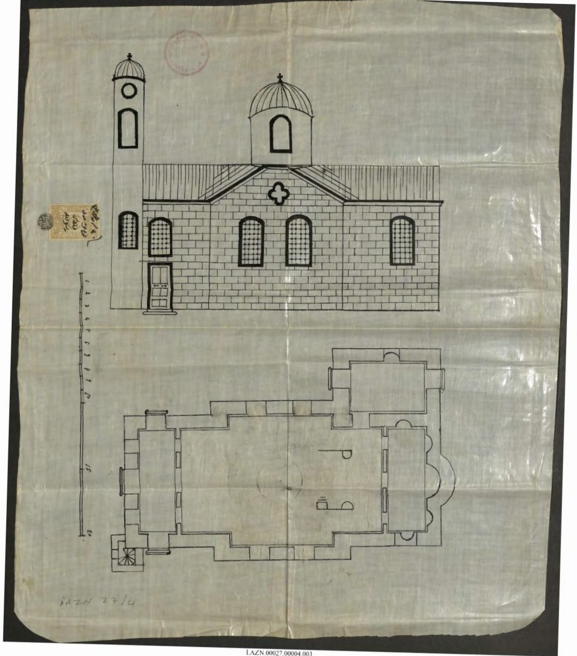
Belge 36: Hayrabolu kazasına Bağlı Hasköy Köyü Sınırları İçinde Bulunan Ayazma Yakınında Bulunan Eski Kilisenin Temelleri üzerine İnşa Edilecek Yeni Kilisenin Mimari Çizimleri (BOA, LAZN.27-4, H.04.03.1315/M.03.08.1897)
