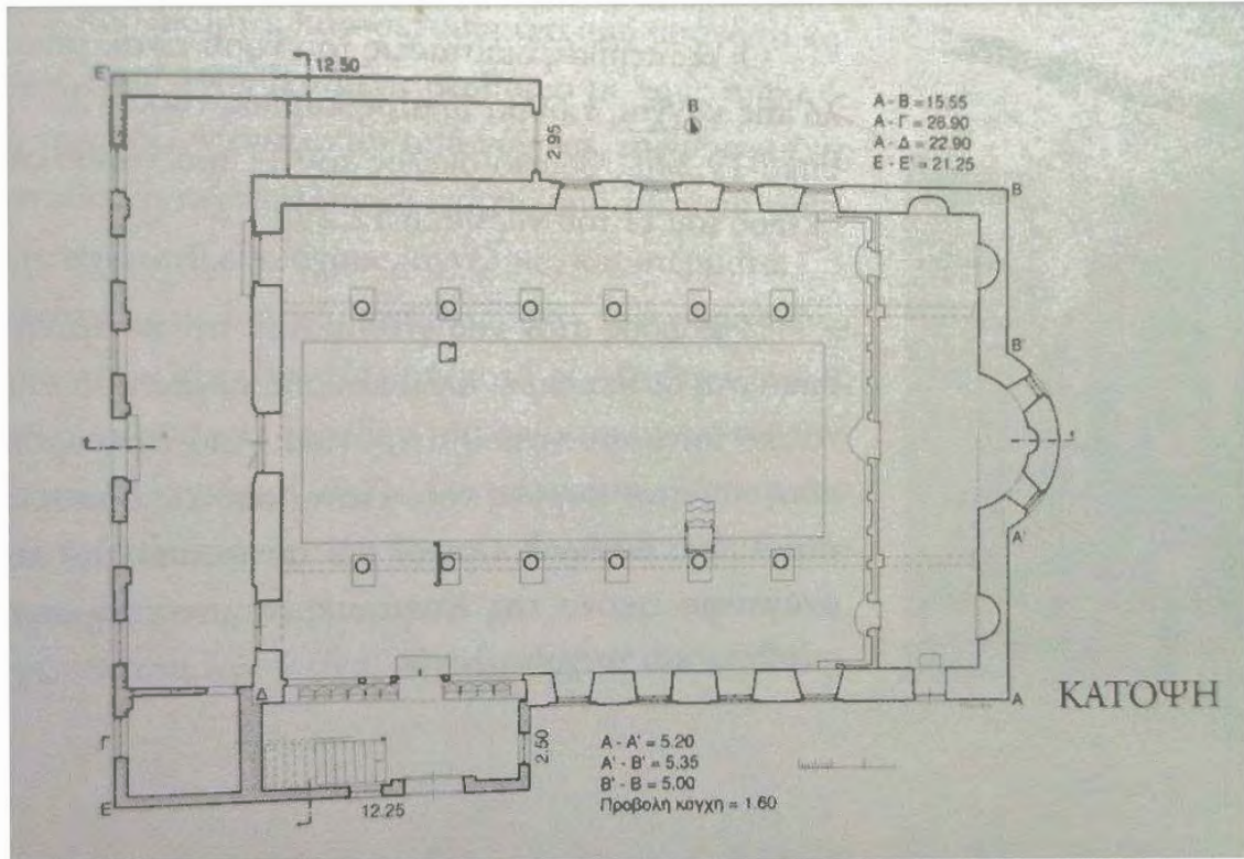
Çizim 132: Dimetoka Kimiseos Theotokou (Κοιμήσεως Θεοτόκου) Kilisesi Zemin Kat Planı (Yılmaz Büktel'den)
