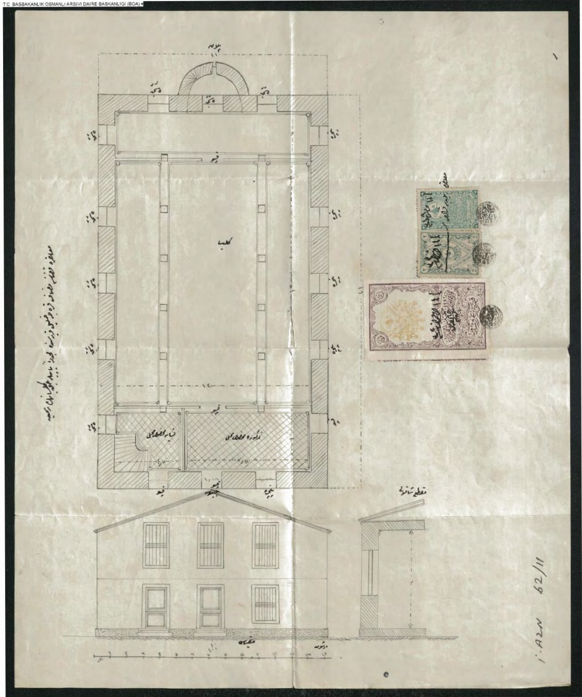
Belge 22: Malkara'ya Bağlı Karaca Halil Köyü'nde Aya Yani Kilisesinin İnşasına Dair Proje Çizimleri (BOA, İ.AZN. 62-11, H.07.06.1323/M.09.08.1905)
