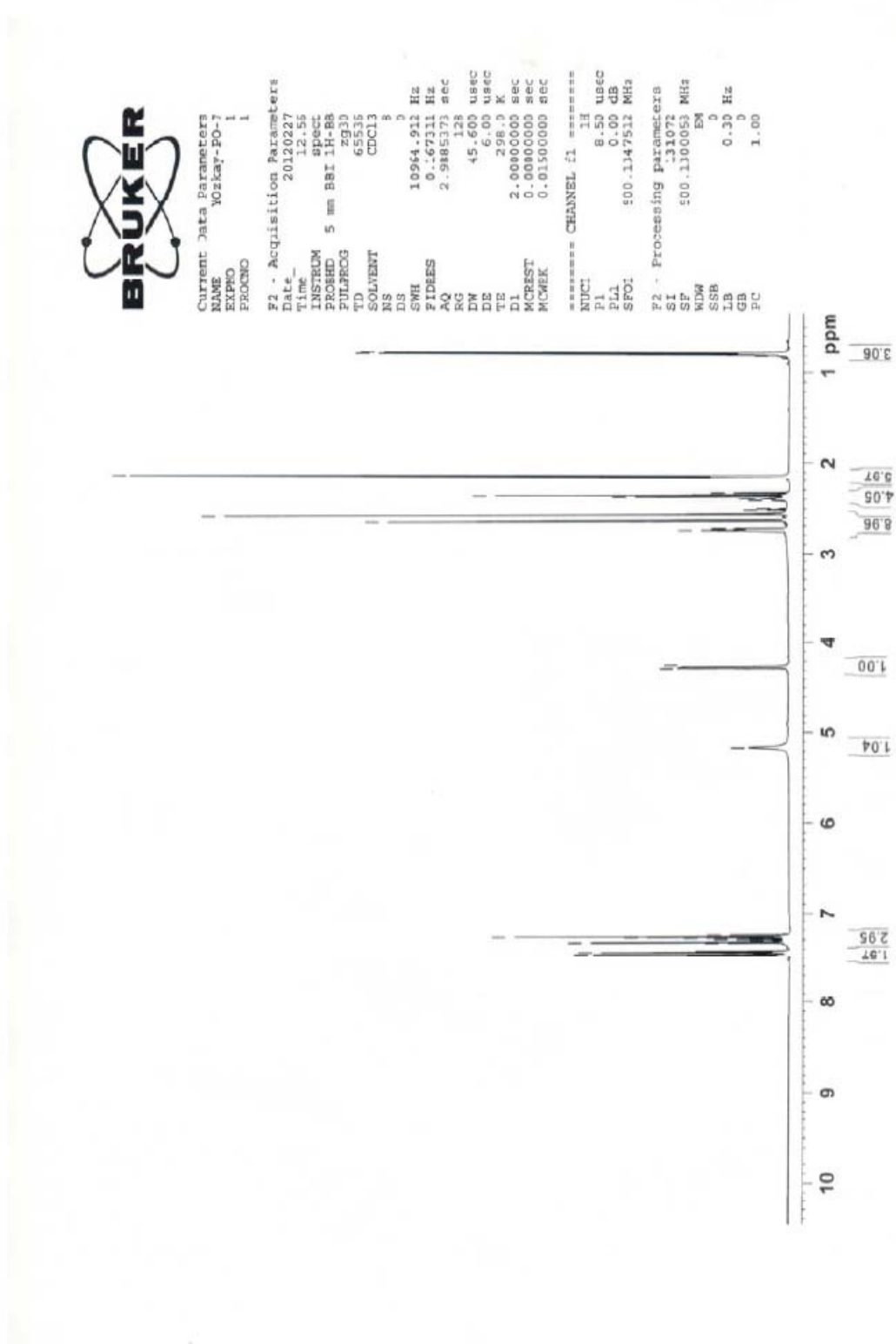
Ek-4. C4 kodlu bileşiğe ait ^1\text{H} -NMR spektrumu
