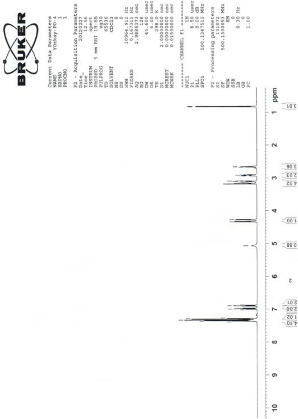
Ek-8. C8 kodlu bileşiğe ait ^1\text{H} -NMR spektrumu
