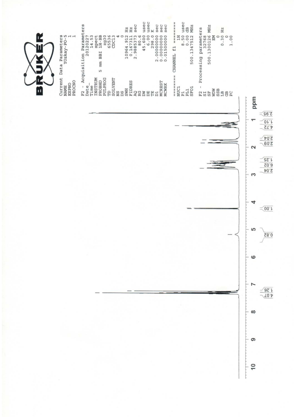
Ek-5. C5 kodlu bileşiğe ait ^1\text{H} -NMR spektrumu
