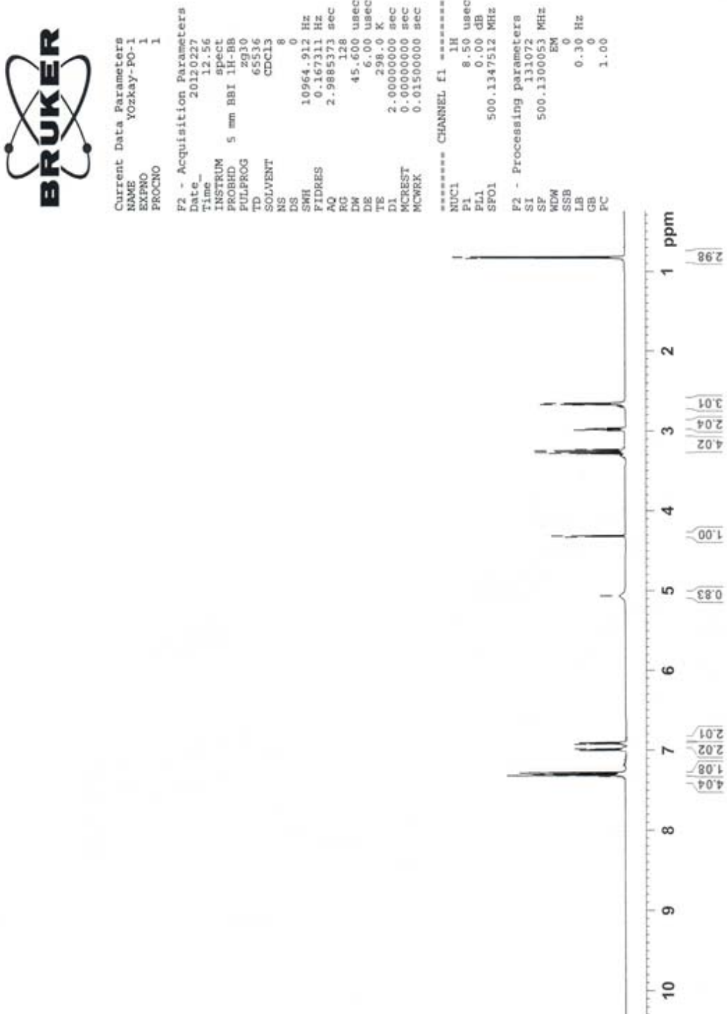
Ek-9. C9 kodlu bileşiğe ait ^1\text{H} -NMR spektrumu
