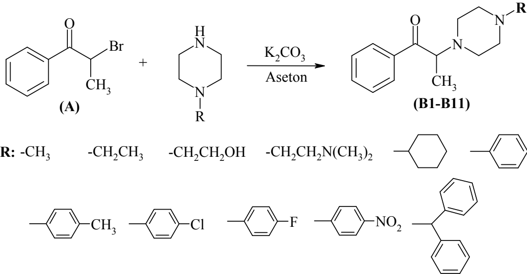
Şekil 9. 1-Fenil-2-(4-süstitüepiperazin-1-il)propanon türevlerinin (B1-B11) genel sentez yöntemleri
