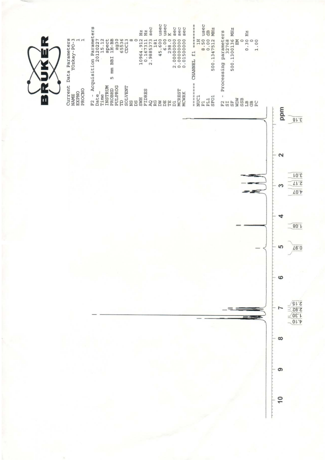
Ek-6. C6 kodlu bileşiğe ait ^1\text{H} -NMR spektrumu
