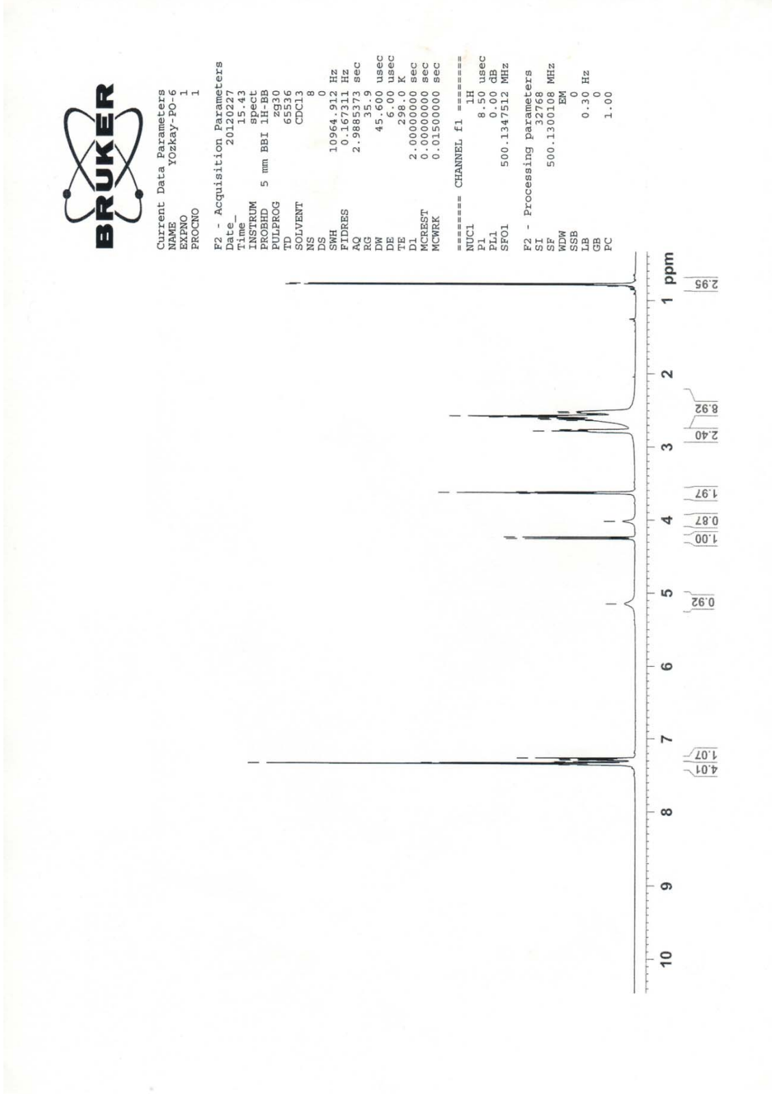
Ek-3. C3 kodlu bileşiğe ait ^1\text{H} -NMR spektrumu
