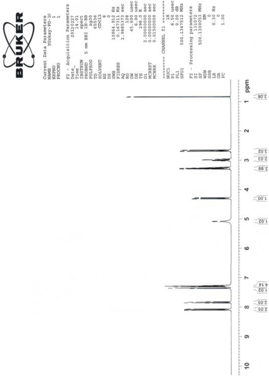
Ek-10. C10 kodlu bileşiğe ait ^1\text{H} -NMR spektrumu
