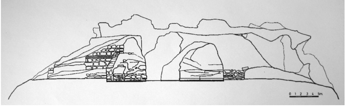
PLAN 4. Karacahisar Kalesi doğudaki giriş kapısı cephe rölövesi
