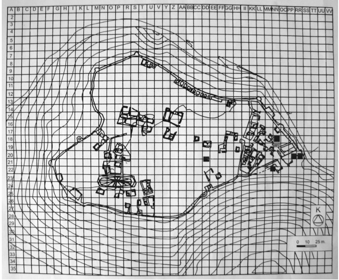
PLAN 1. Karacahisar Kalesi topografik planı
